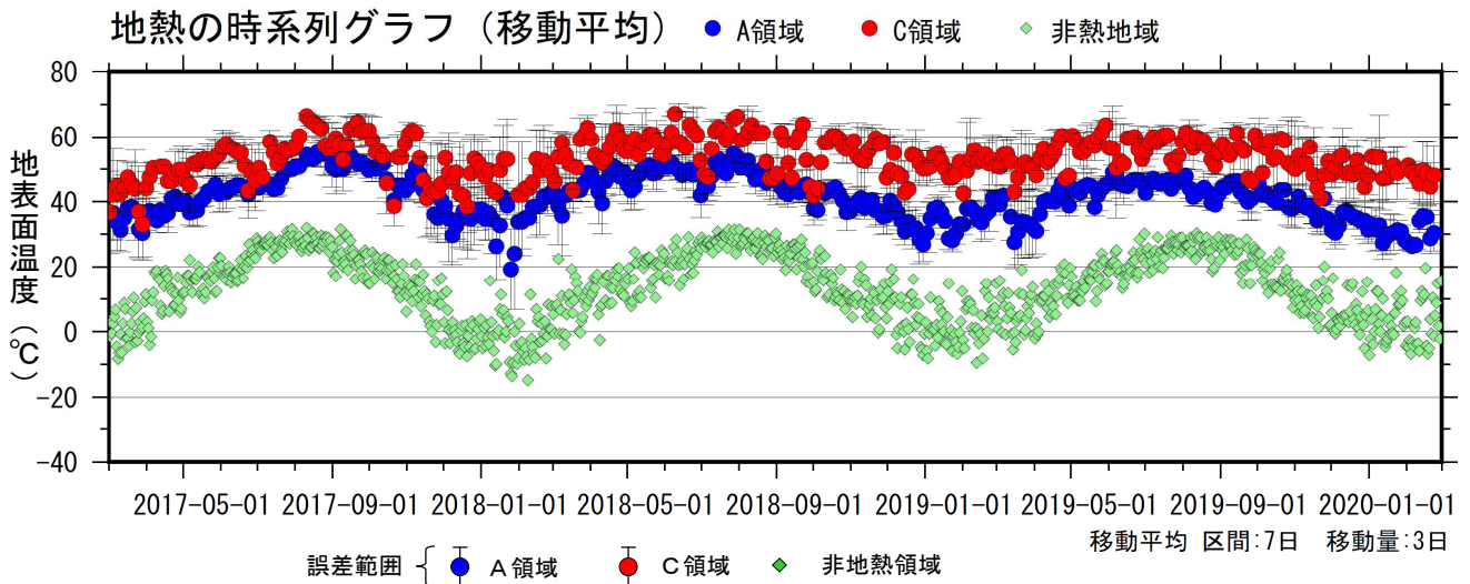
図2-2 九重山 星生山北尾根の赤外熱映像装置による日別最高温度の7日間移動平均値 (2017年3月～2020年2月)
