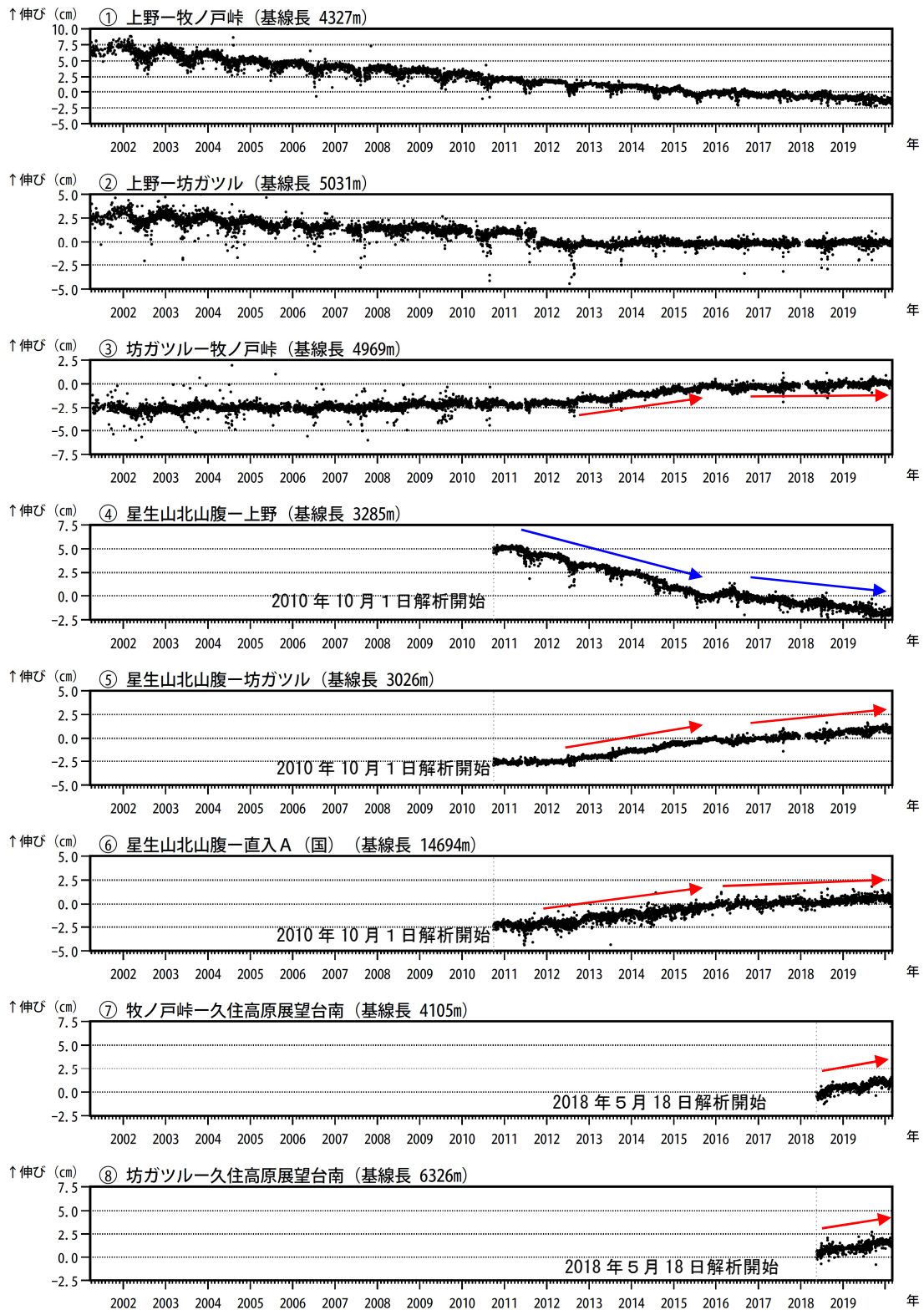
図8 九重山 GNSS連続観測による基線長変化（2001年4月～2020年2月）
