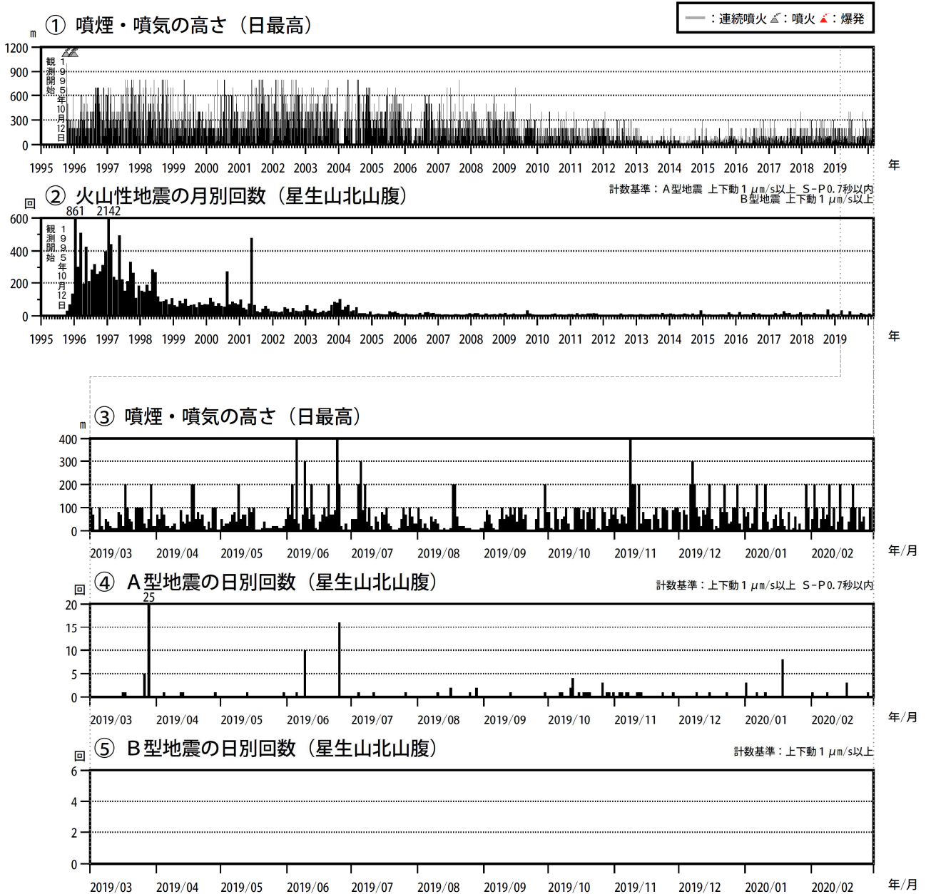
図3 九重山 火山活動経過図（1995年1月～2020年2月）
