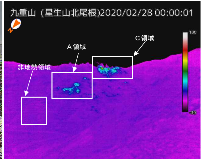
図2-1 九重山 地熱域の様相
