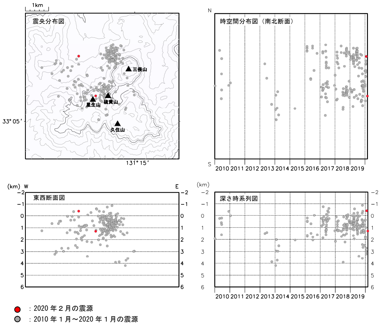
図 4-2 九重山 震源分布図（硫黄山付近の火山性地震）（2010年1月～2020年2月）
