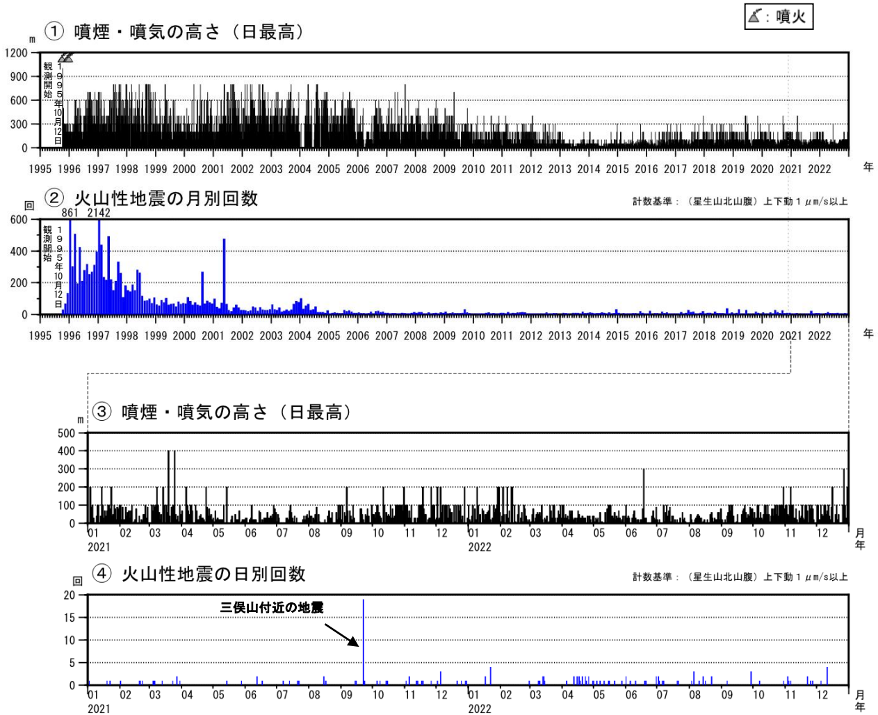
図3 九重山 火山活動経過図（1995年1月～2022年12月）
