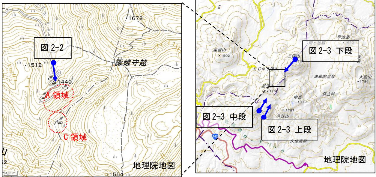
図 2-1 九重山 現地調査観測・機上観測位置及び撮影方向
