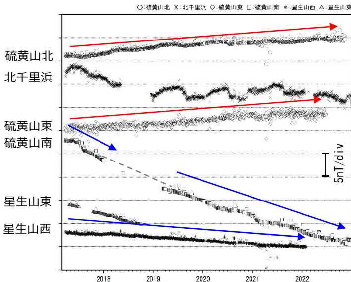
図 5-1 九重山 連続観測による全磁力の変化 (2017年3月~2022年12月31日)
