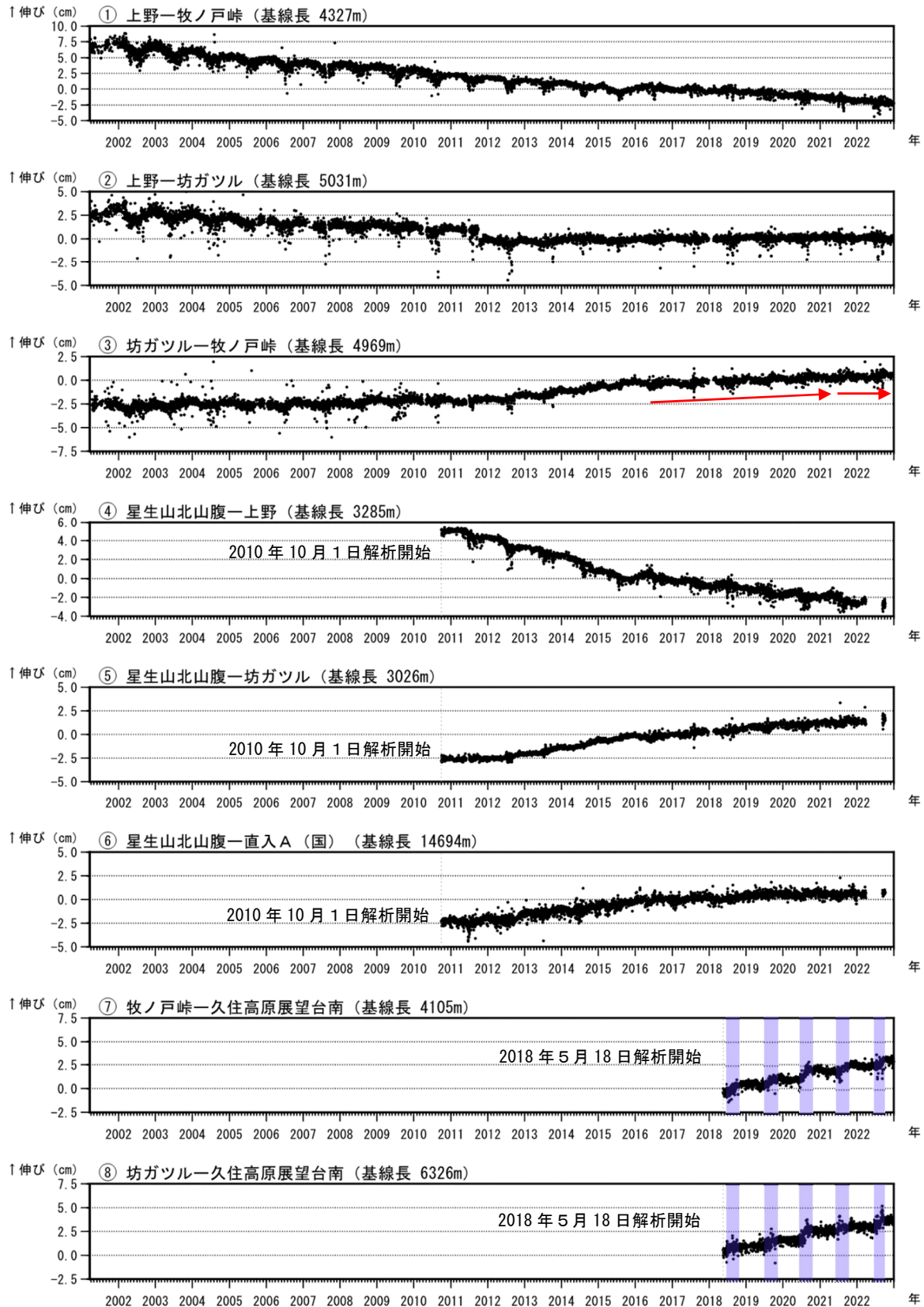
図6 九重山 GNSS連続観測による基線長変化 (2001年4月~2022年12月)
