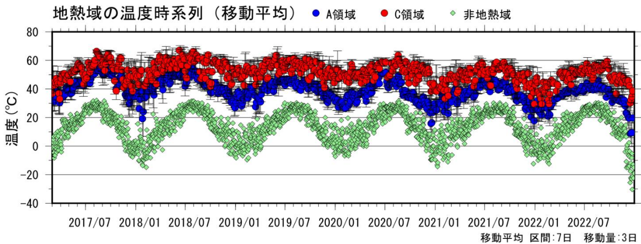
図 1-2 九重山 星生山北尾根の赤外熱映像装置による日別最高温度 (2017年3月~2022年12月)
