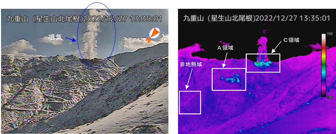
図 1-1 九重山 硫黄山の噴気及び地熱域の状況 (12月27日 星生山北尾根監視カメラ)
