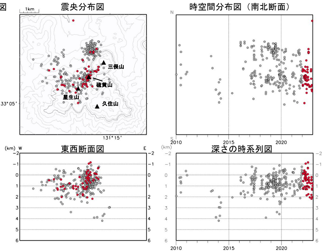
図4 九重山 震源分布図 ①広域図②狭域図 (2010年1月～2022年12月)
