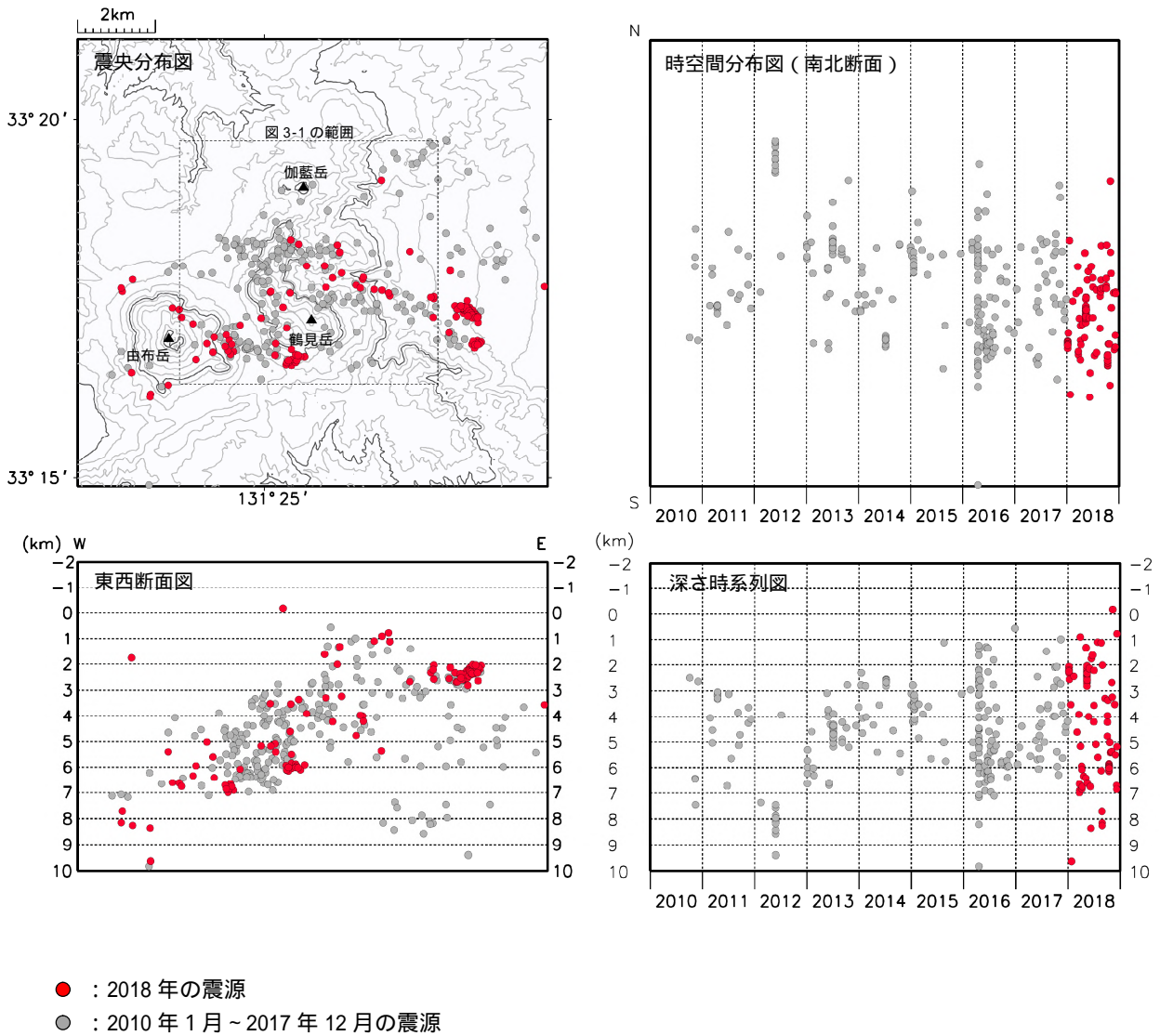
図 3-2 鶴見岳・伽藍岳 震源分布図（広域）（2010 年 1 月 ~ 2018 年 12 月）
