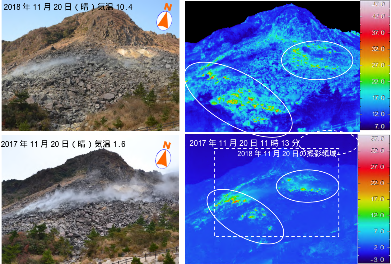
図 6 鶴見岳・伽藍岳 伽藍岳噴気地帯の赤外熱映像装置による地表面温度分布 ( 図中の白丸は伽藍岳噴気地帯の熱異常域を示す ) 前回 ( 2017年11月20日 ) の観測と比較して噴気の状態や熱異常域の分布に特段の変化は認められませんでした。
