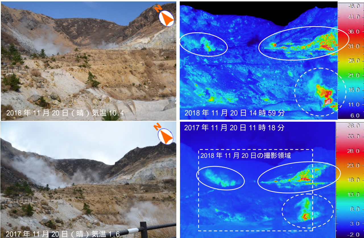
図 5 鶴見岳・伽藍岳 伽藍岳噴気地帯の赤外熱映像装置による地表面温度分布
