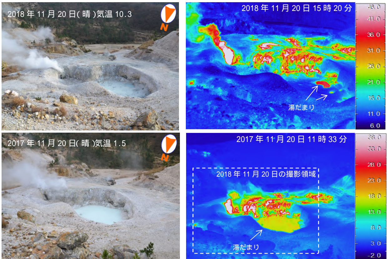
図 7 鶴見岳・伽藍岳 伽藍岳泥火山の赤外熱映像装置による地表面温度分布 泥火山内部の湯だまりは、量が減少し、水温が上昇していました。噴気の状態や熱異常域の分布については、前回 ( 2017年11月20日 ) の観測と比較して特段の変化は認められませんでした。
