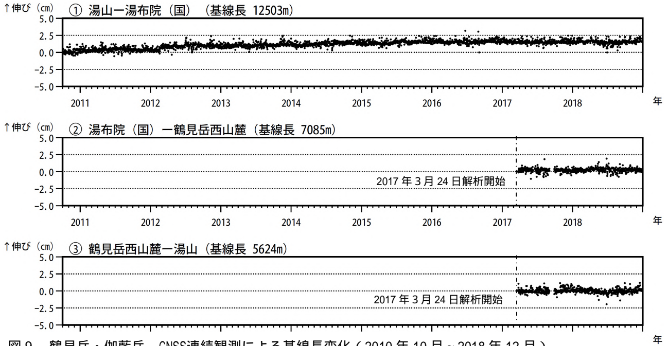
図 9 鶴見岳・伽藍岳 GNSS連続観測による基線長変化 (2010年10月~2018年12月) GNSS連続観測では、火山活動によると考えられる特段の変化は認められませんでした。
