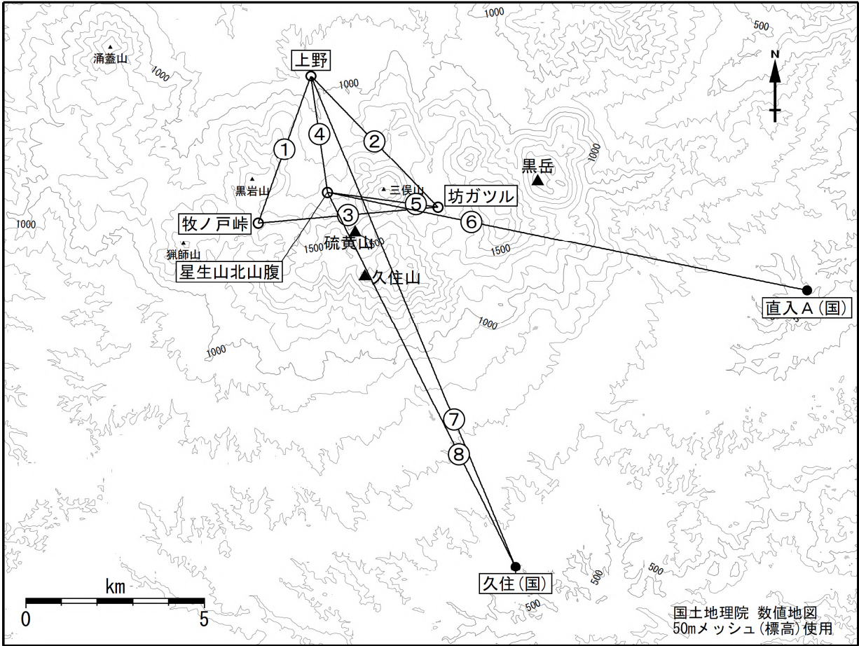
図 11 九重山 GNSS 連続観測点と基線番号
