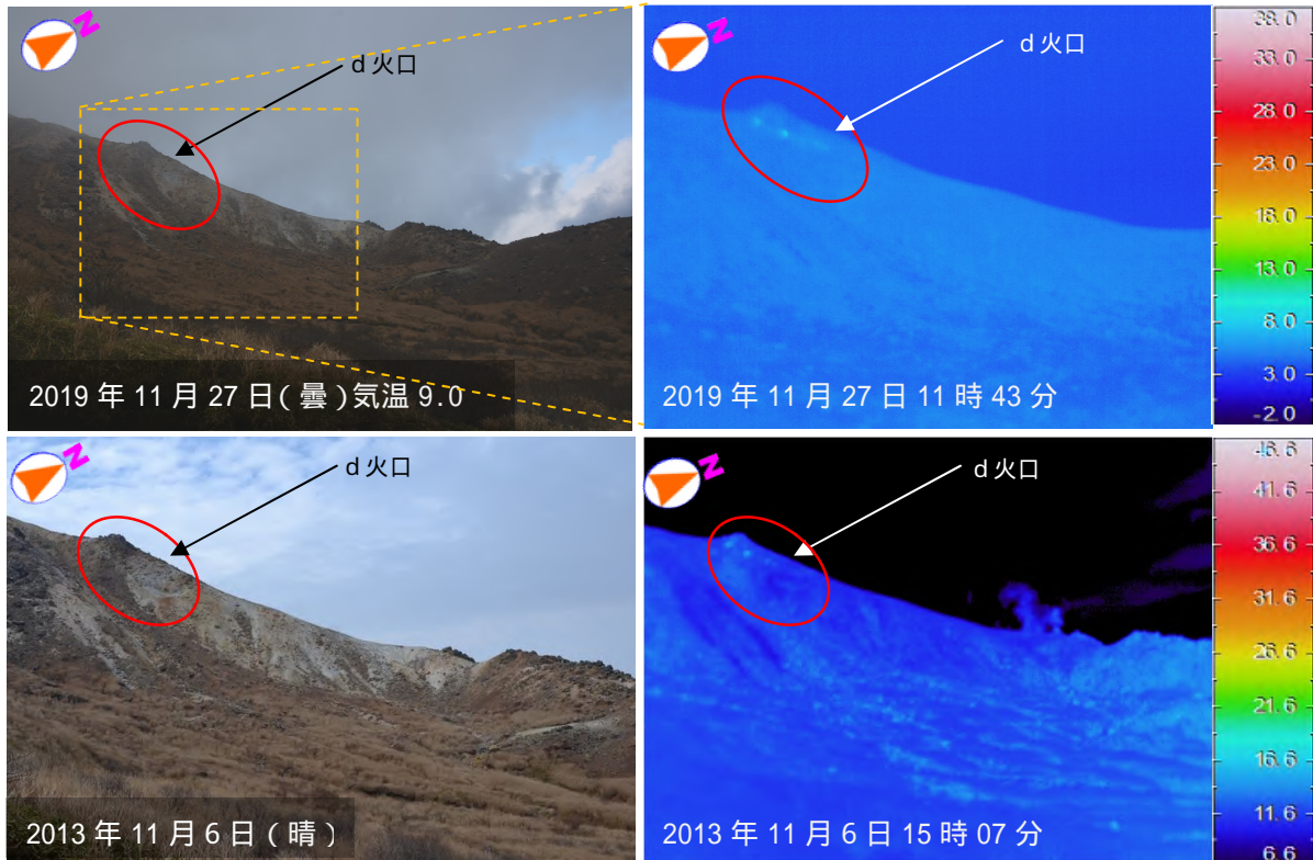
図 4-3 九重山 D領域の可視画像及び地表面温度分布の変化
