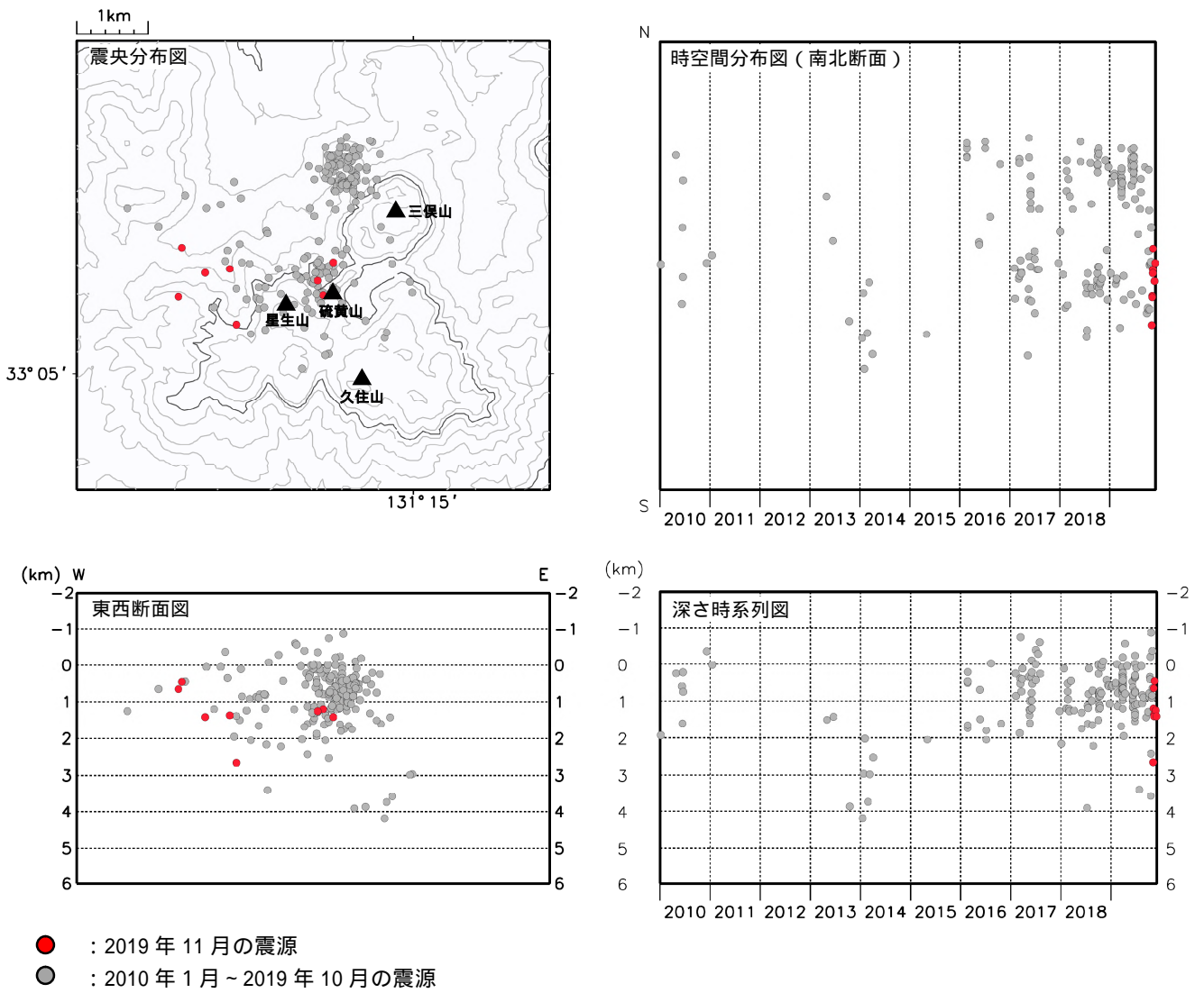
図 6-1 九重山 震源分布図（硫黄山付近の火山性地震）（2010年1月～2019年11月）
