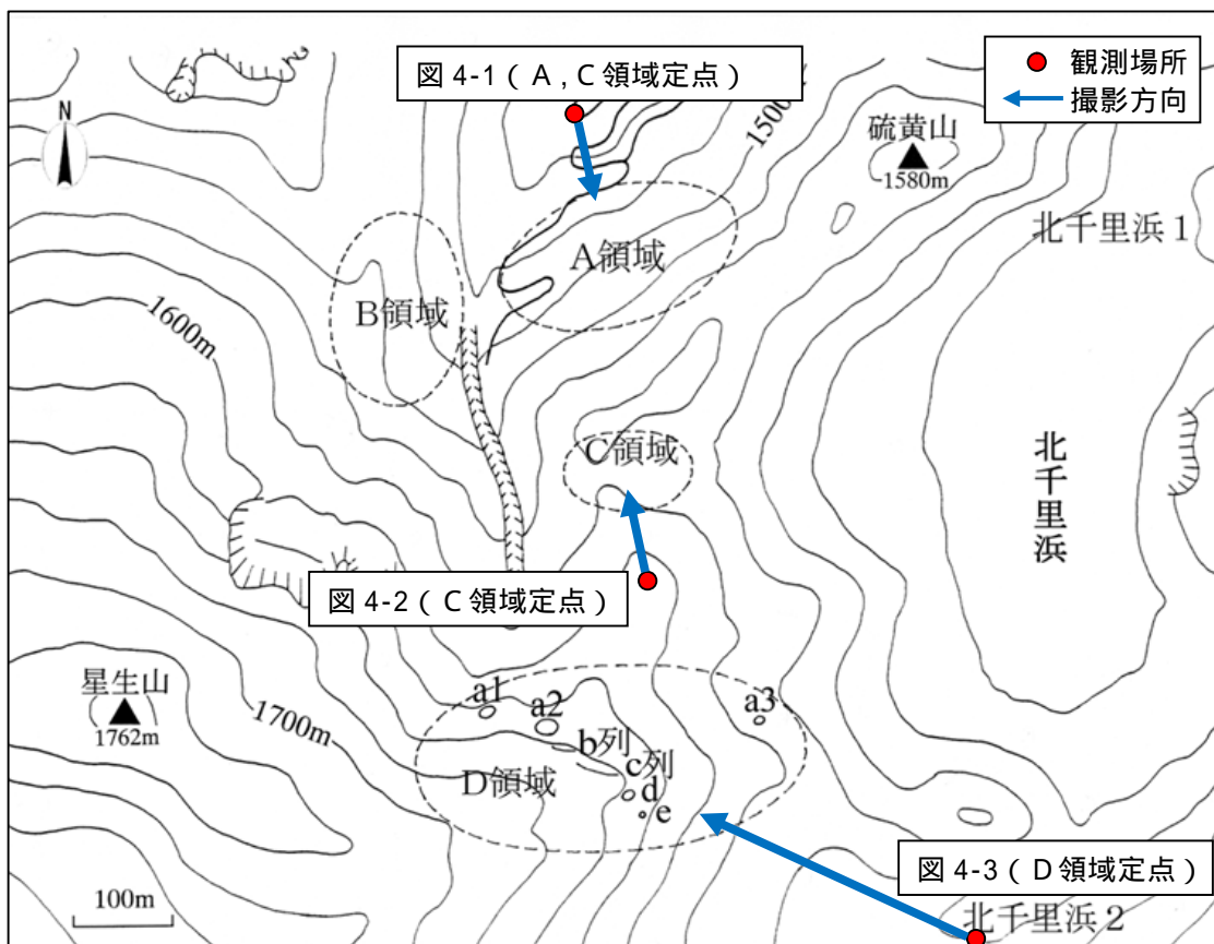
図 3 九重山 図 4 の観測位置及び撮影方向
