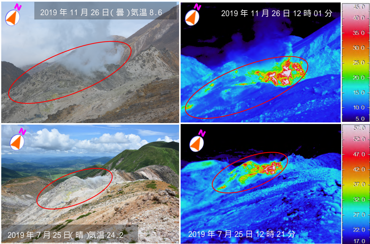
図 4-2 九重山 噴気地帯C領域の可視画像及び地表面温度分布
