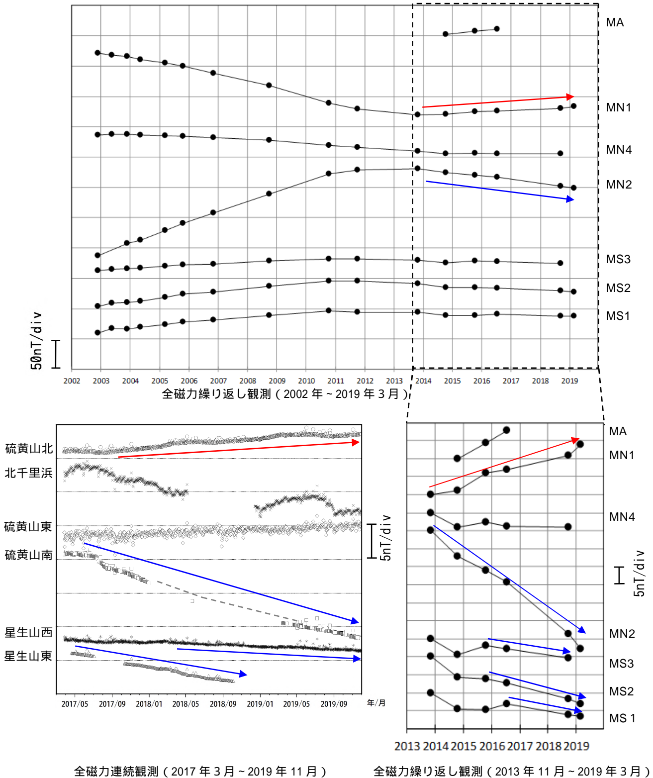
図7 九重山 連続観測及び繰り返し観測による全磁力の変化
