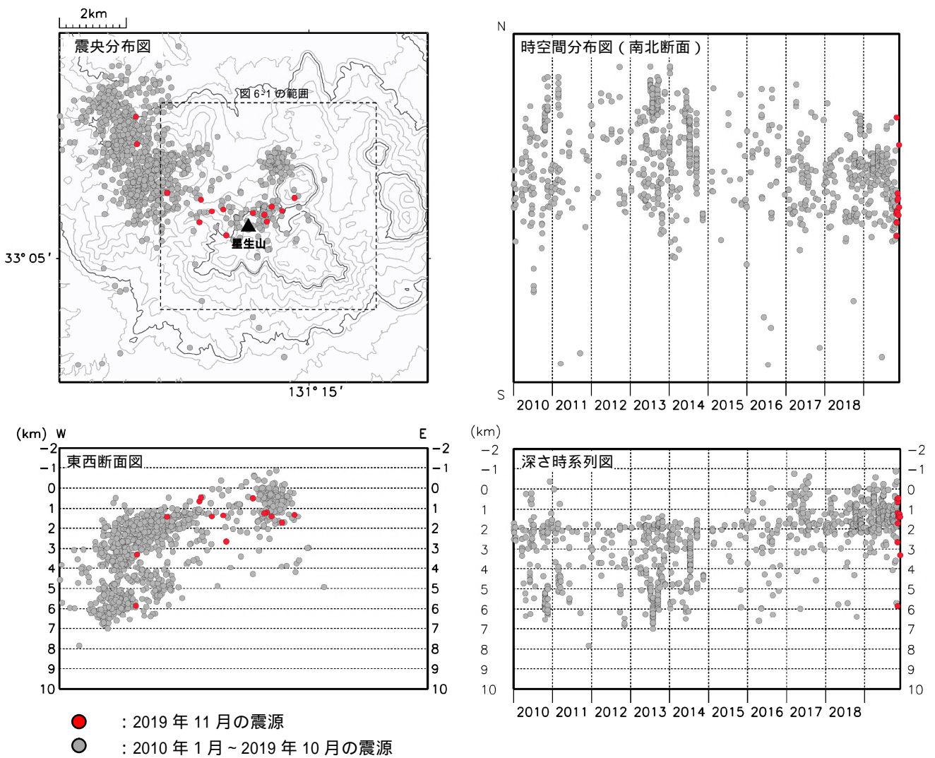
図 6-2 九重山 震源分布図（広域）（2010年1月～2019年11月）
