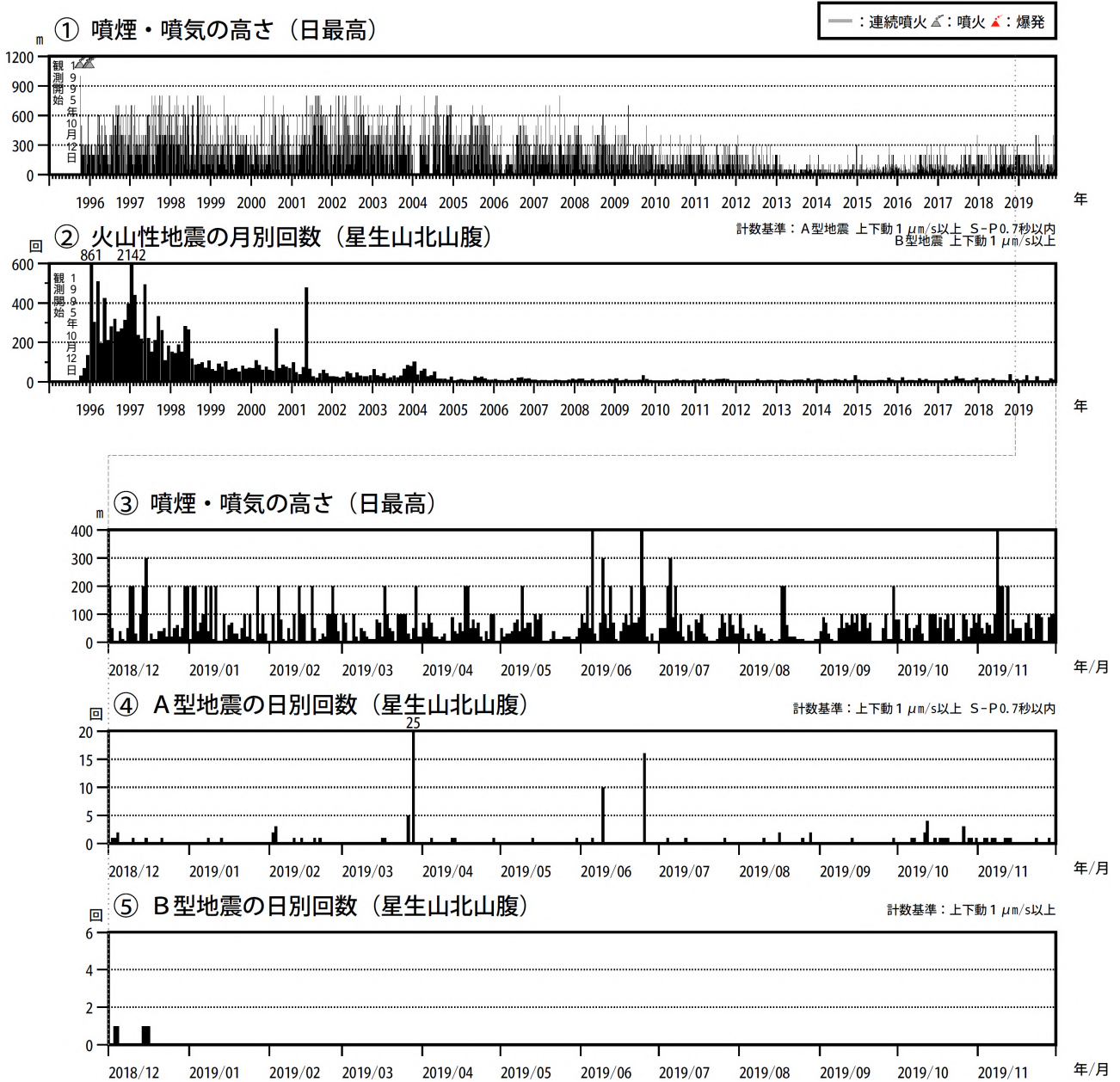
図5 九重山 火山活動経過図（1995年11月～2019年11月）
