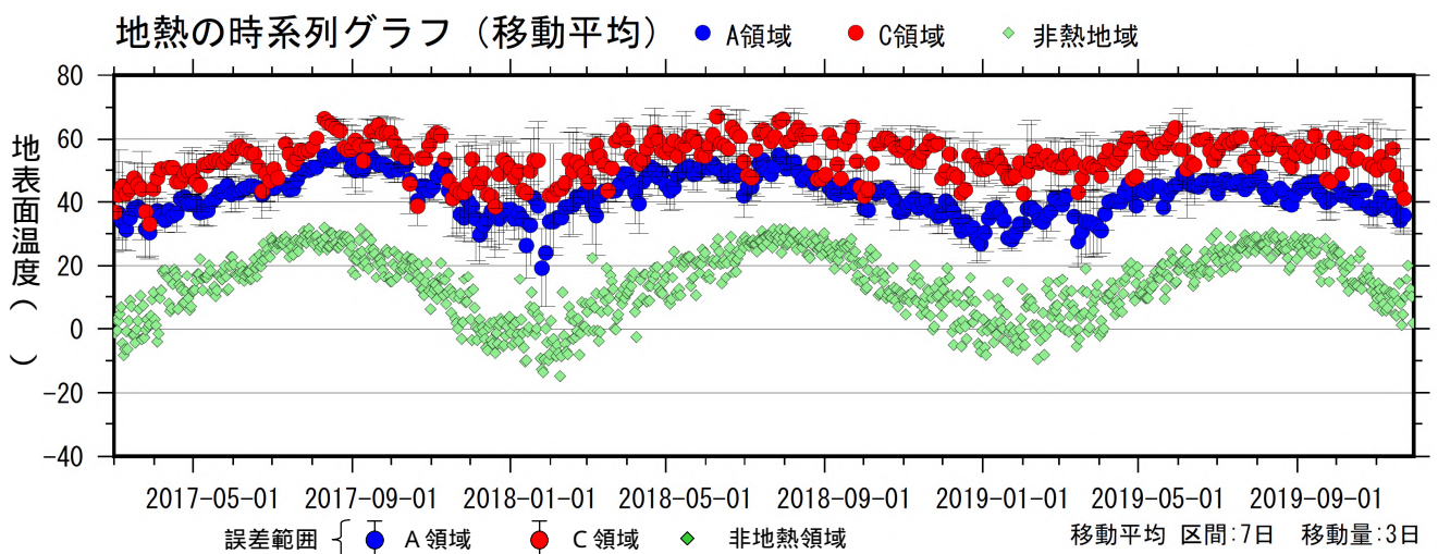
図 2-2 九重山 星生山北尾根の赤外熱映像装置による日別最高温度の 7 日間移動平均値 （2017 年 3 月～2019 年 11 月）
