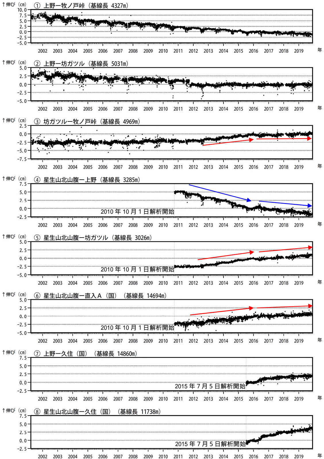
図 10 九重山 GNSS 連続観測による基線長変化（2001 年 3 月～2019 年 11 月）
