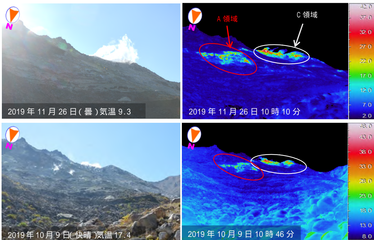
図 4-1 九重山 噴気地帯 A 領域 C 領域の可視画像及び地表面温度分布
