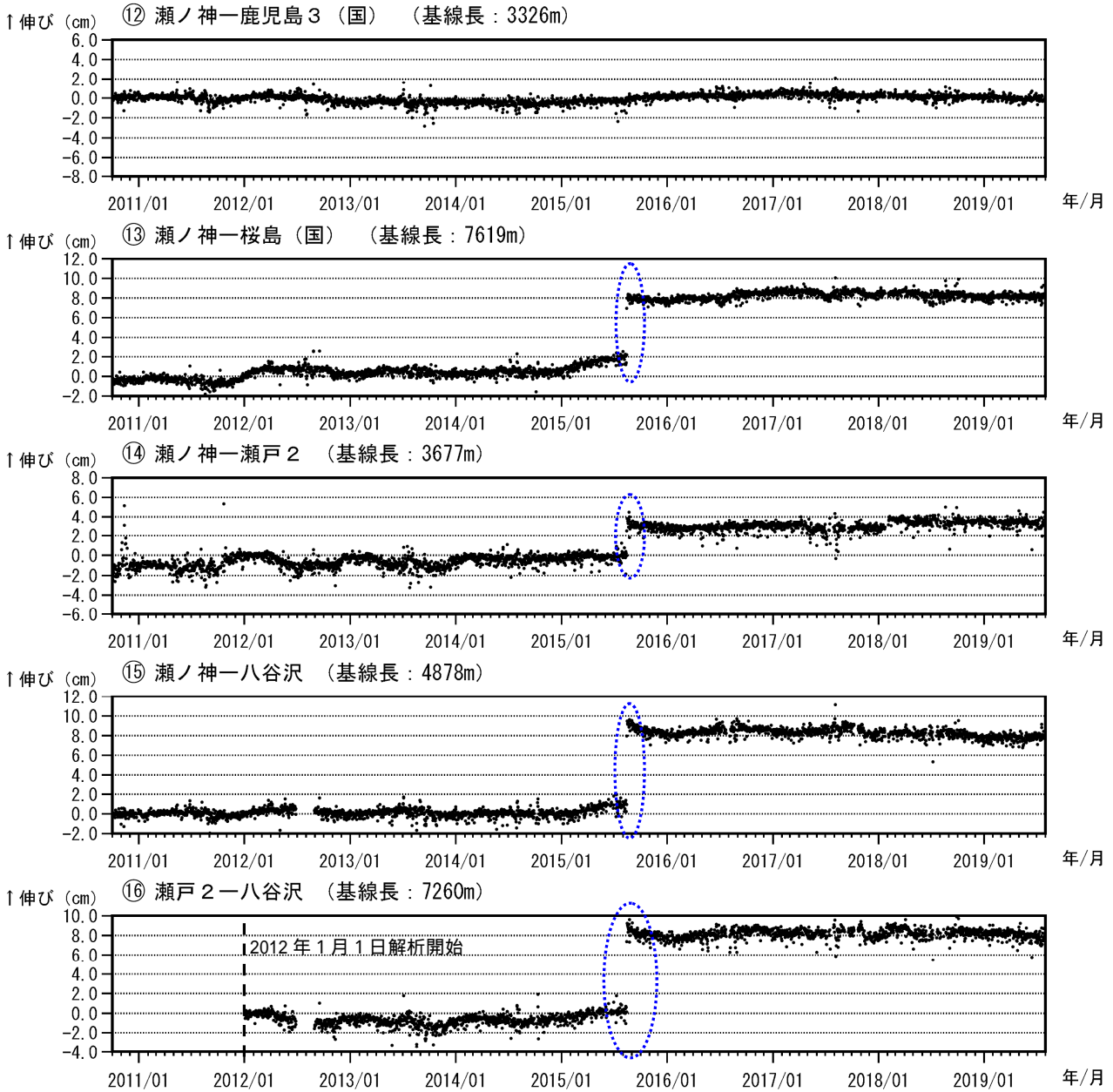
図 7-3 桜島 GNSS 連続観測による基線長変化 (2010 年 10 月 ~ 2019 年 7 月)
