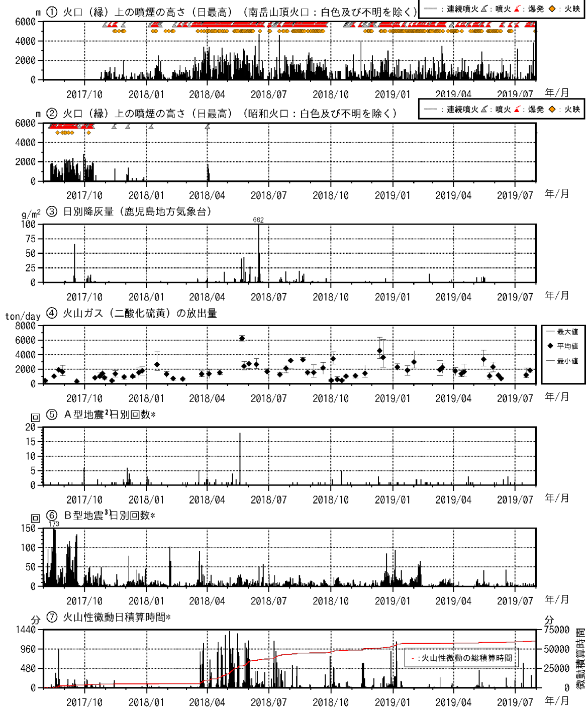
図4 桜島 最近2年間の活動経過図（2017年8月～2019年7月）
