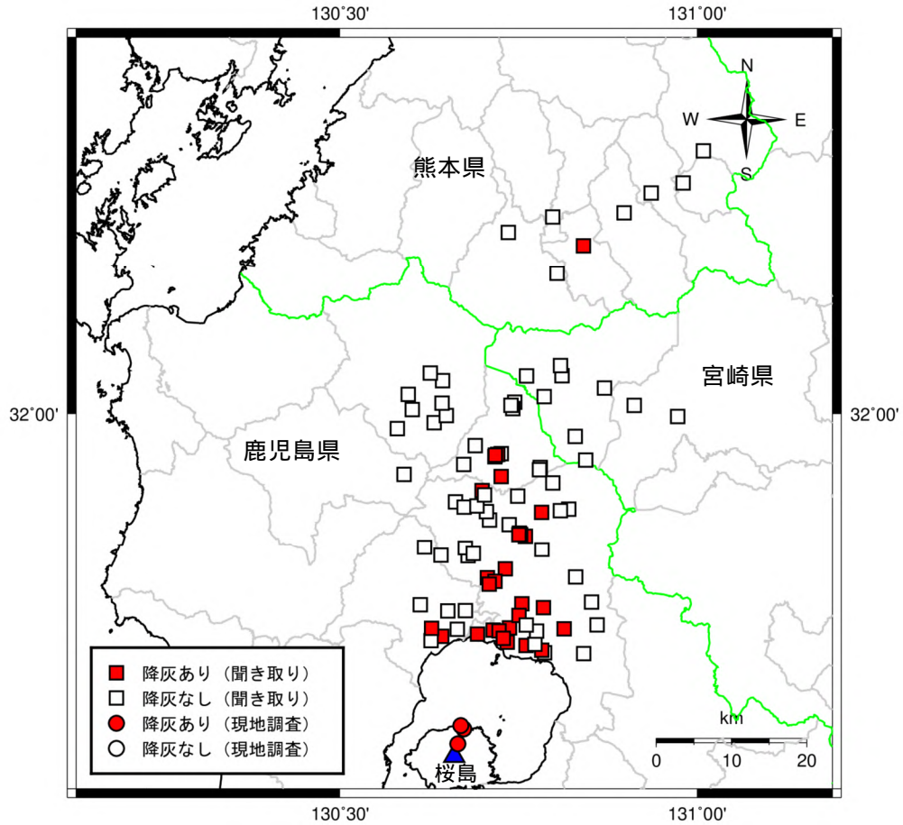
図 2-1 桜島 28 日の噴火による降灰の状況
