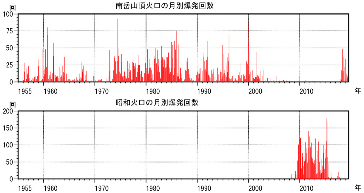
図 3-1 桜島 南岳山頂火口（上図）と昭和火口（下図）の月別爆発回数 （1955年1月～2019年7月）
