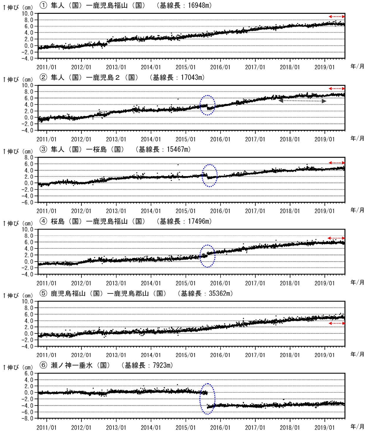
図 7-1 桜島 GNSS 連続観測による基線長変化（2010 年 10 月～2019 年 7 月）
