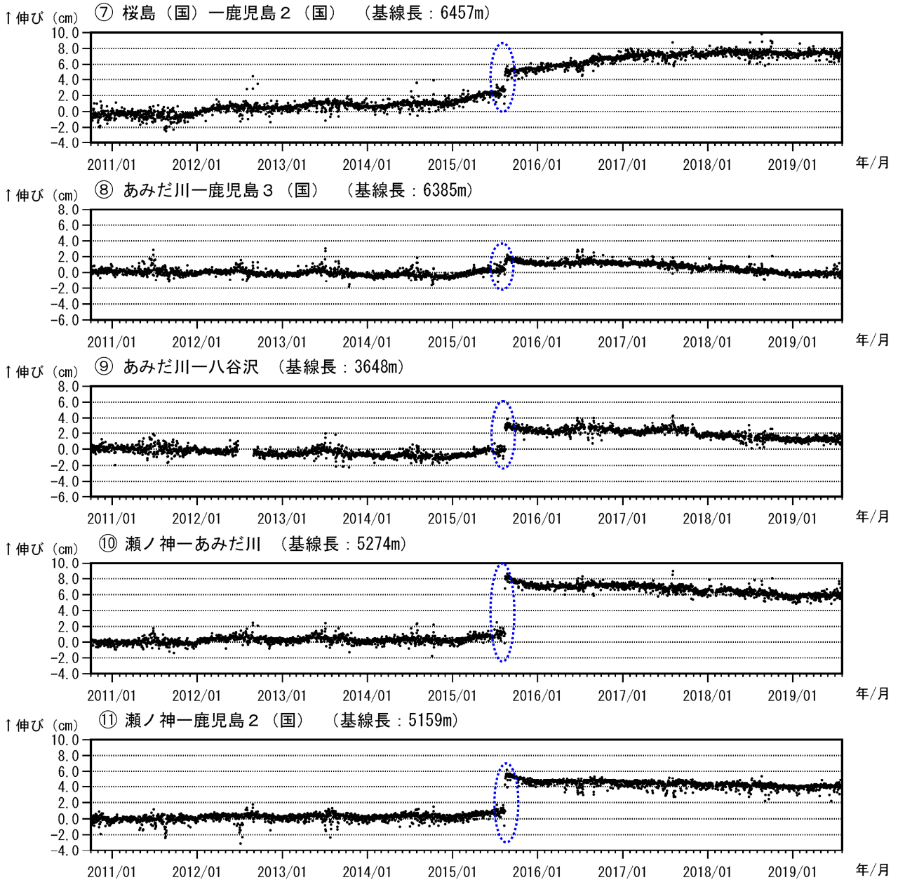
図 7-2 桜島 GNSS 連続観測による基線長変化（2010 年 10 月～2019 年 7 月）
