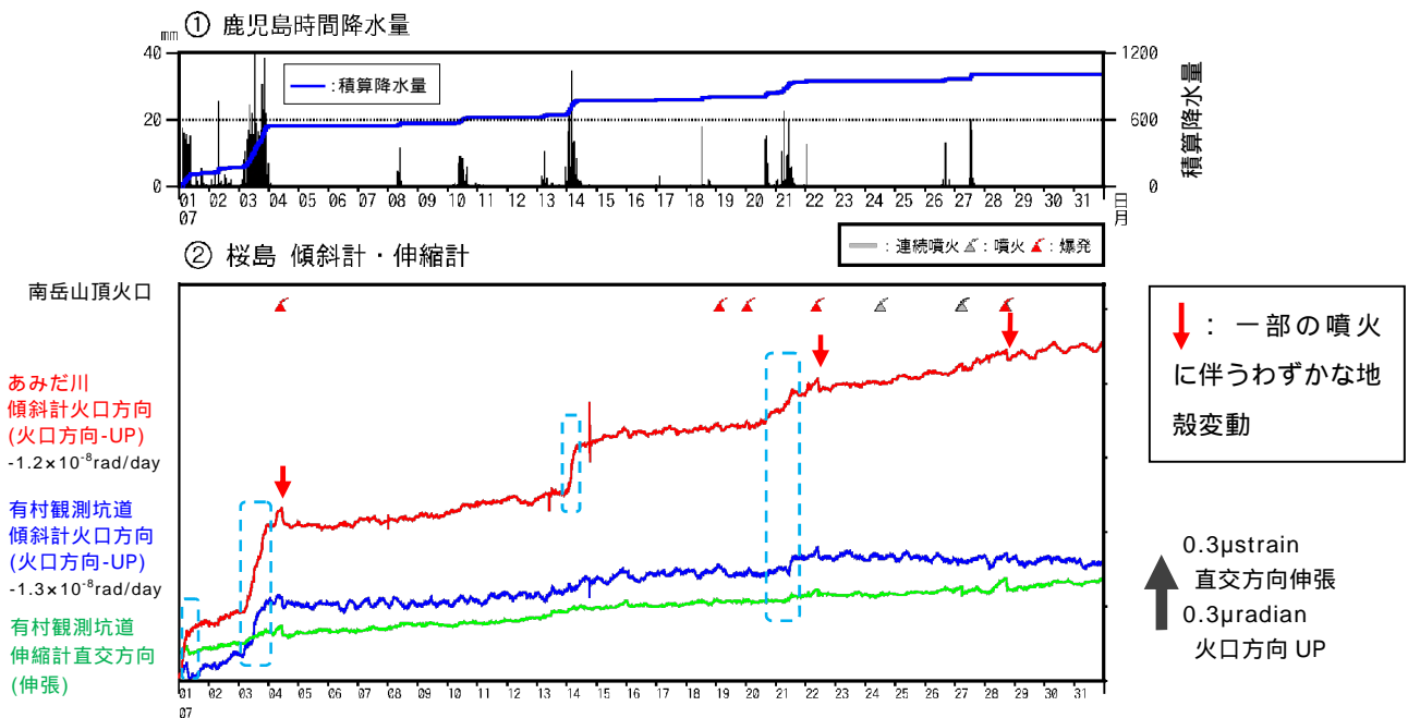
図6 桜島 傾斜計及び伸縮計による地殻変動の状況（2019年7月1日～7月31日）
