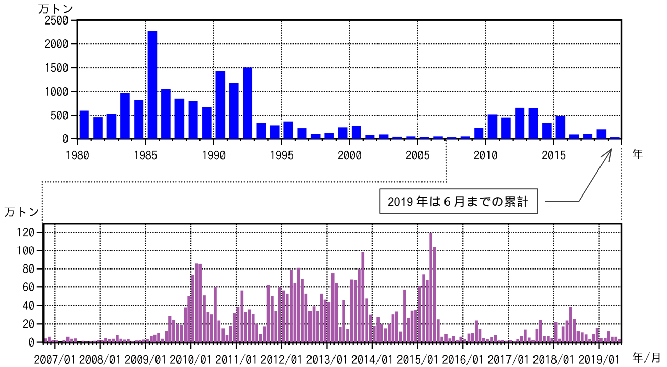
図9 桜島 鹿児島県が実施している降灰の観測データから推定した火山灰の総噴出量 （上段：1980年1月～2019年6月の年別値、下段：2006年10月～2019年6月の月別値）
