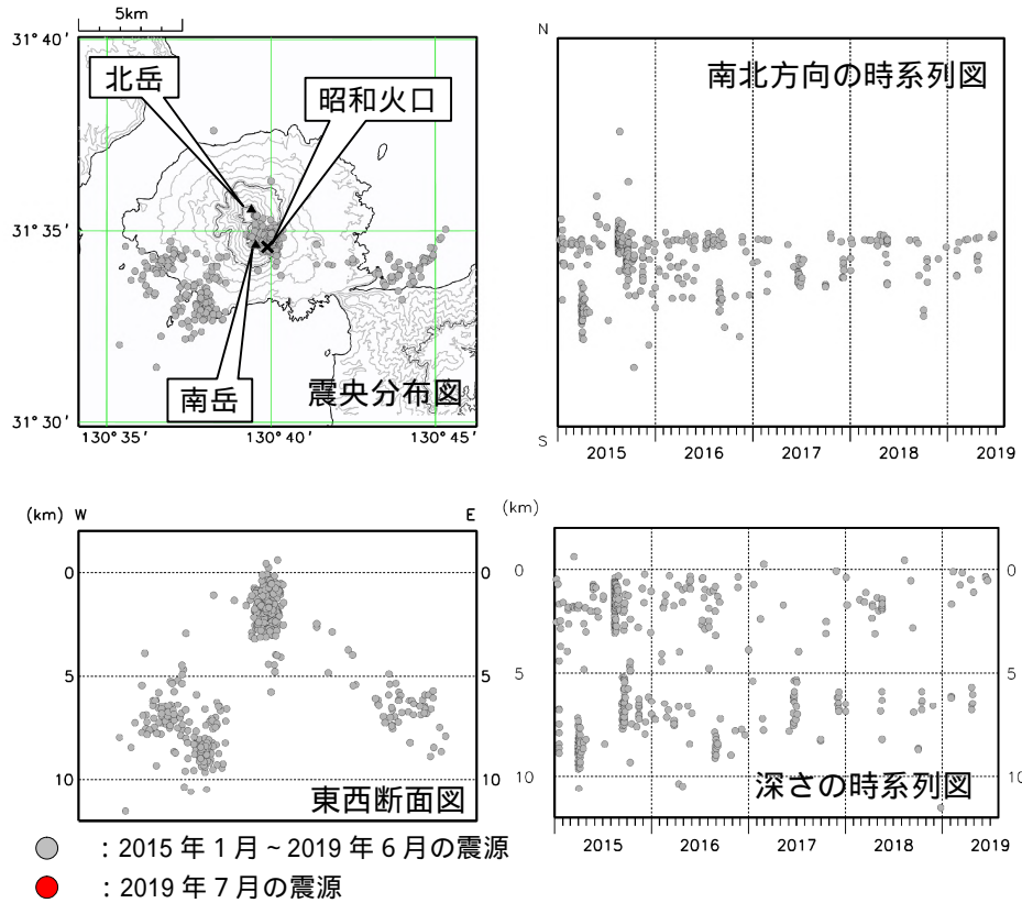
図5 桜島 震源分布図（2015年1月～2019年7月）
