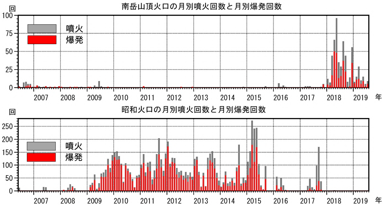
図 3-2 桜島 南岳山頂火口（上図）と昭和火口（下図）の月別噴火回数と月別爆発回数 （2006年6月～2019年7月）
