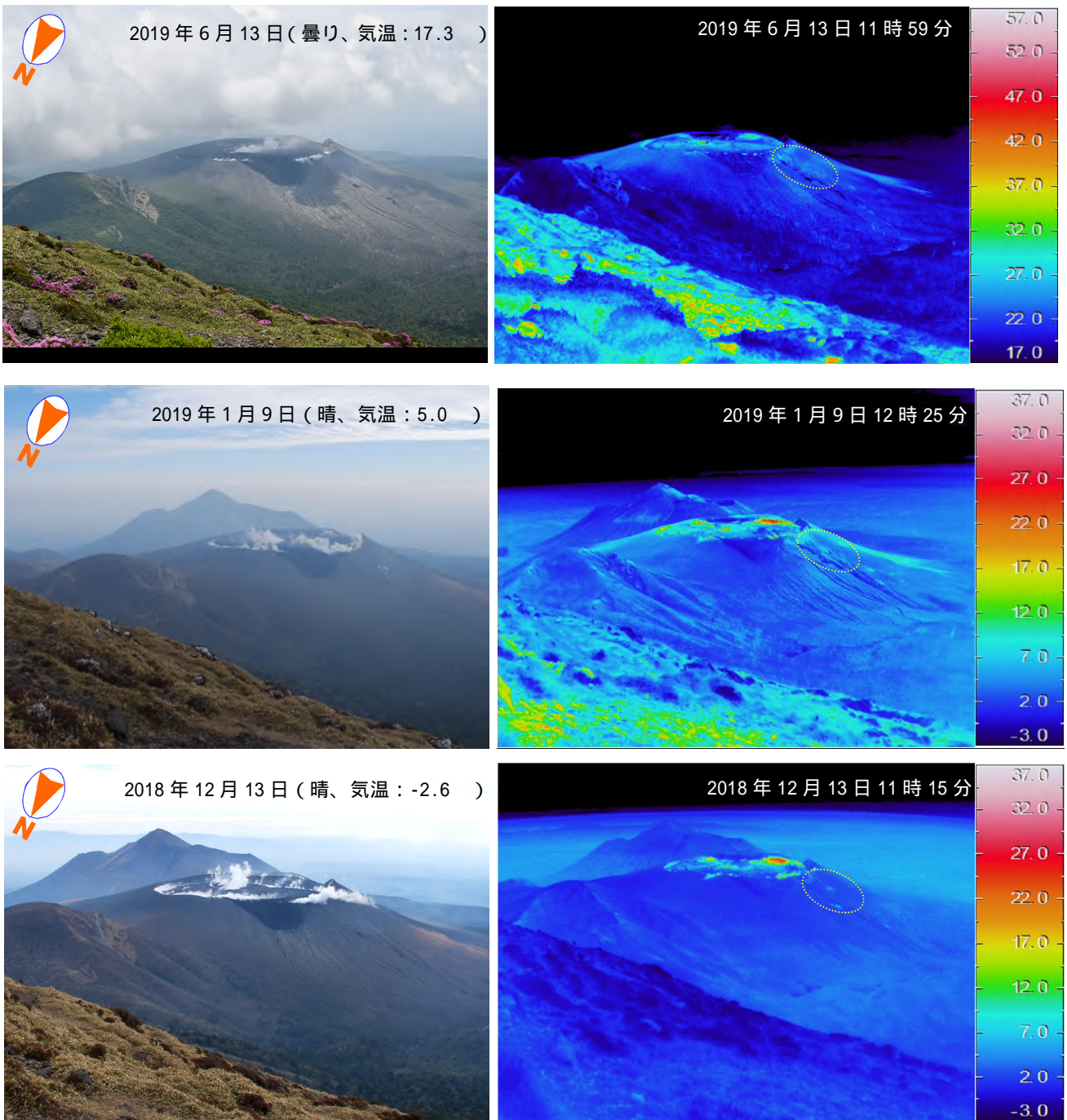
図3 霧島山（新燃岳） 火口内及び西側斜面の状況（韓国岳から観測）
