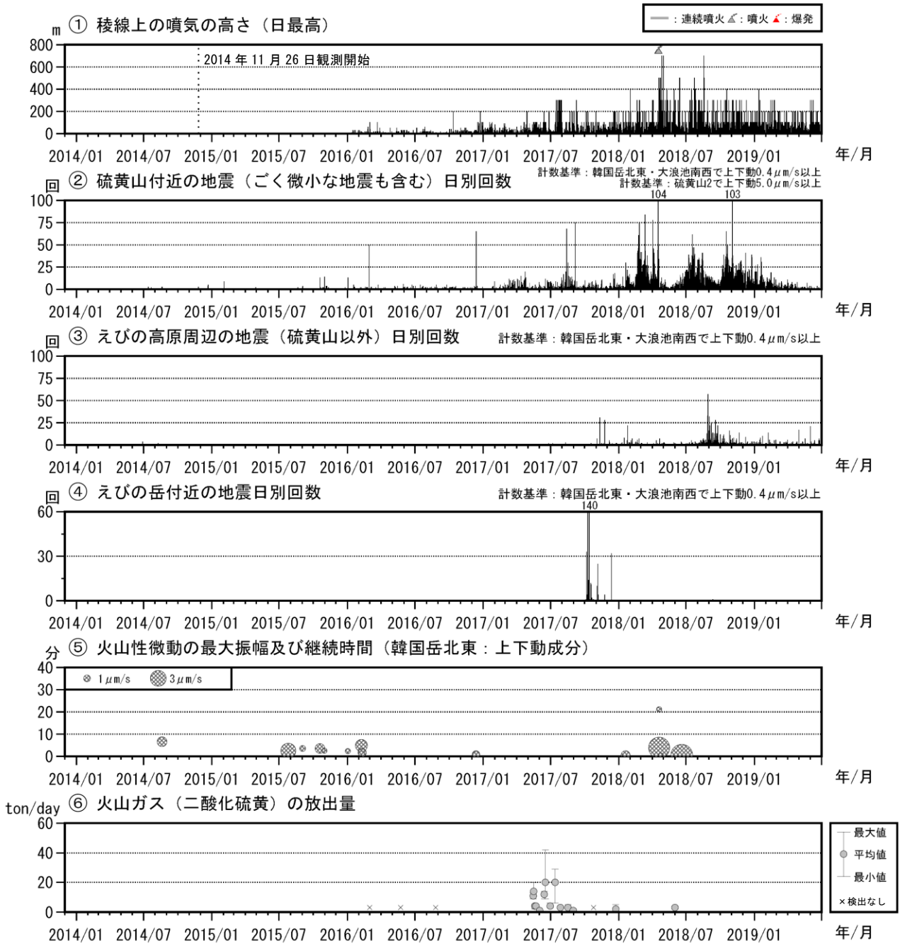
図6 霧島山（えびの高原（硫黄山）周辺）火山活動経過図（2013年12月～2019年6月）
