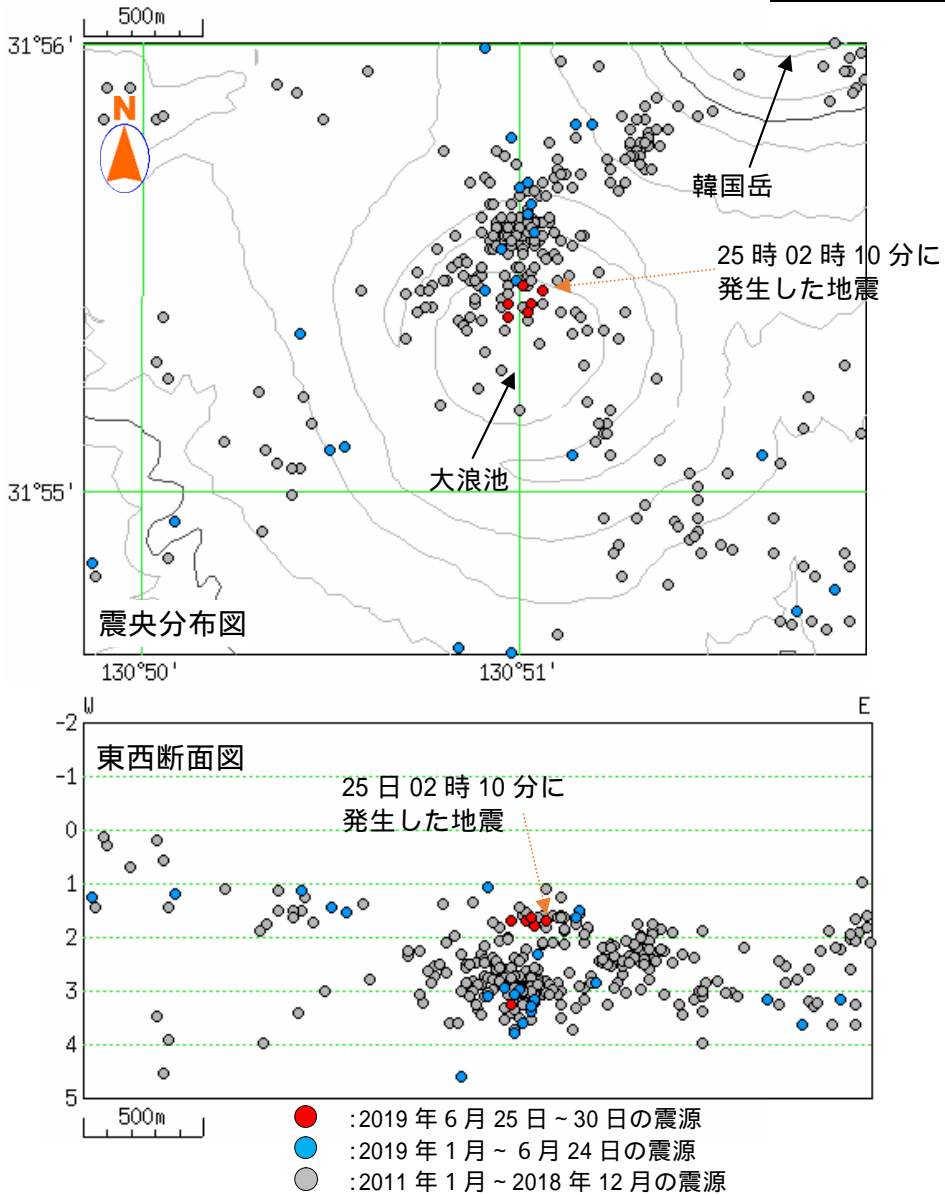
図2 霧島山 震源分布図（2011年1月～2019年6月）
