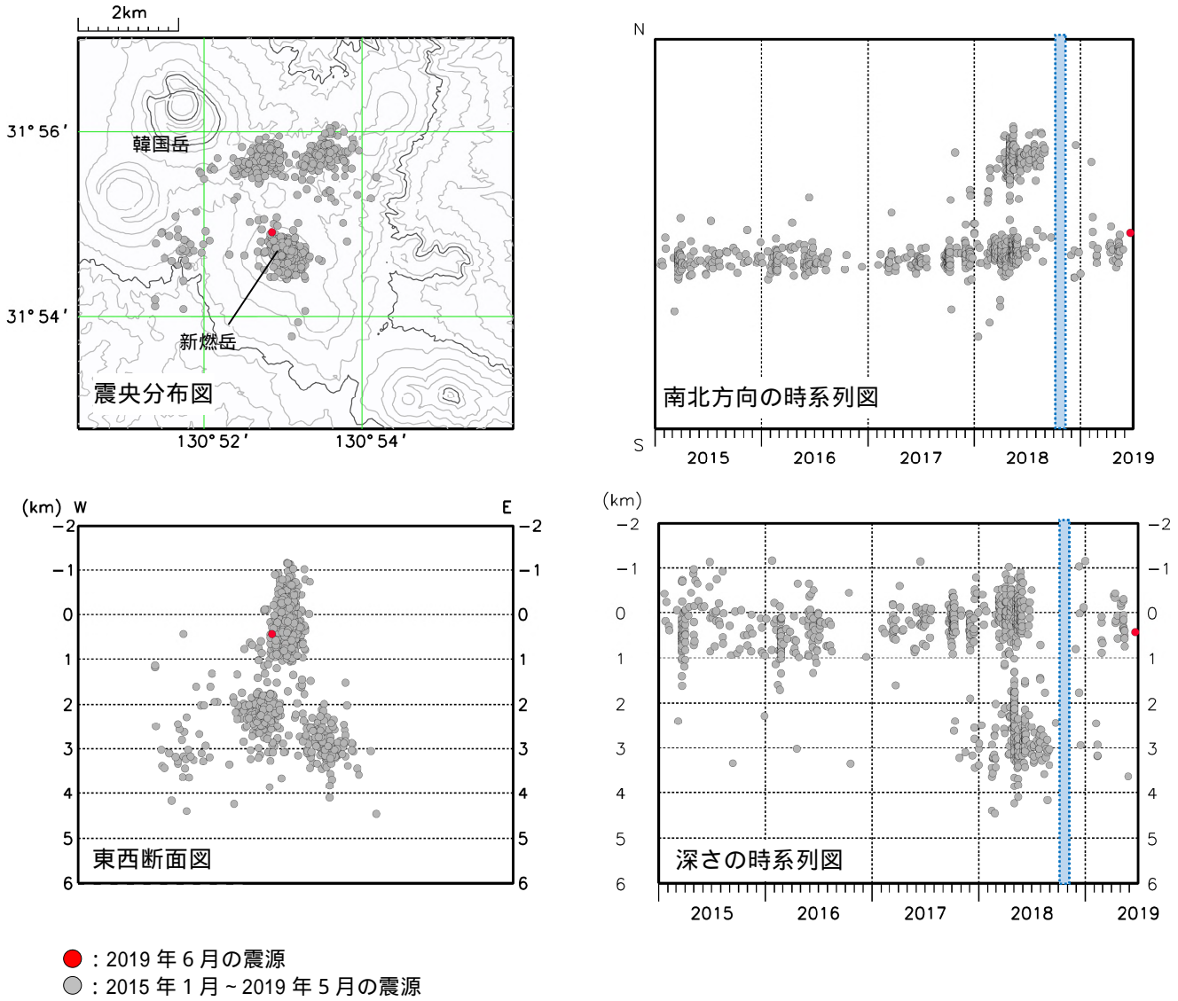
図6 霧島山（新燃岳） 震源分布図（2015年1月～2019年6月）
