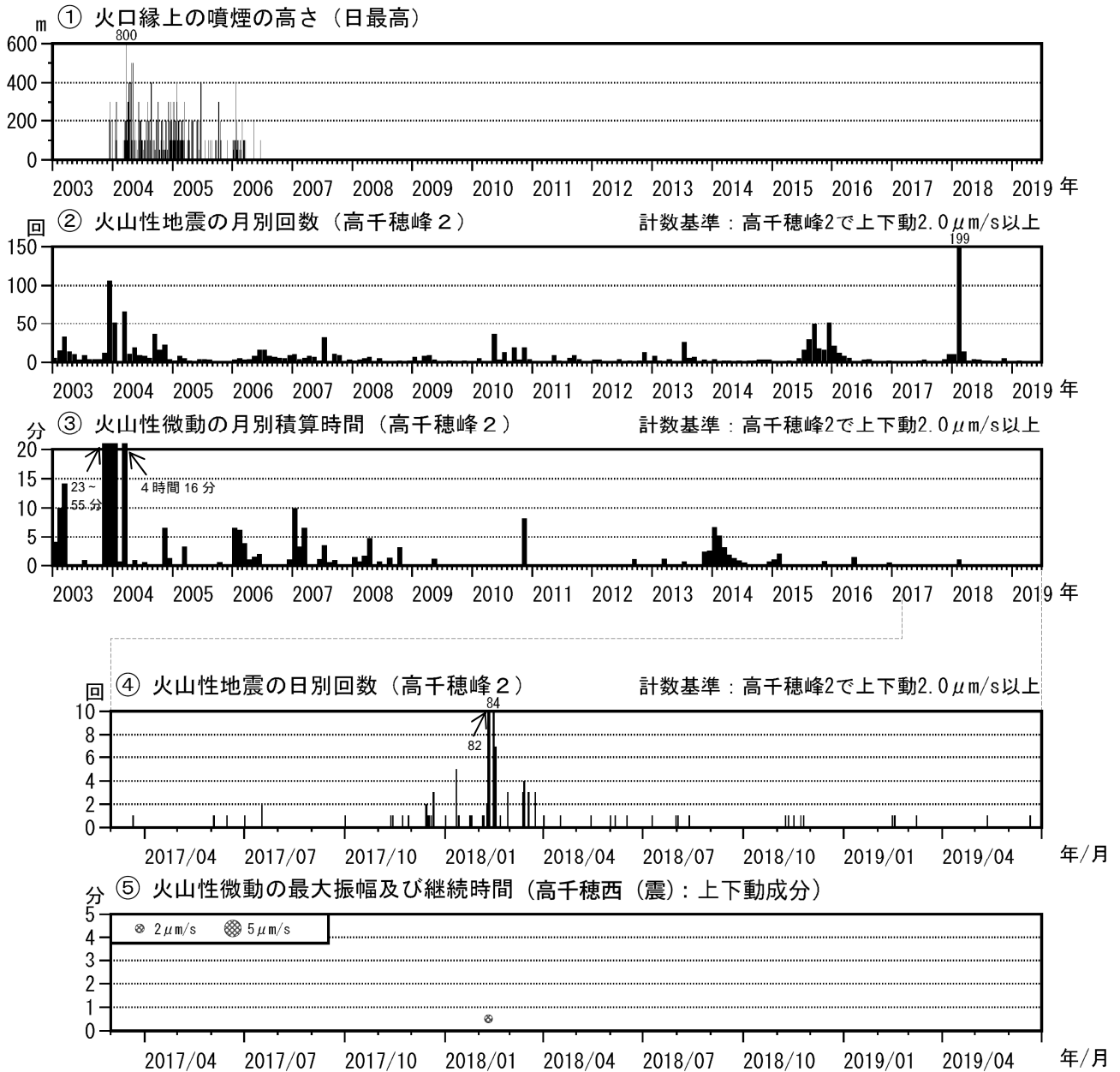
図2 霧島山（御鉢） 火山活動経過図（2003年1月～2019年6月）
