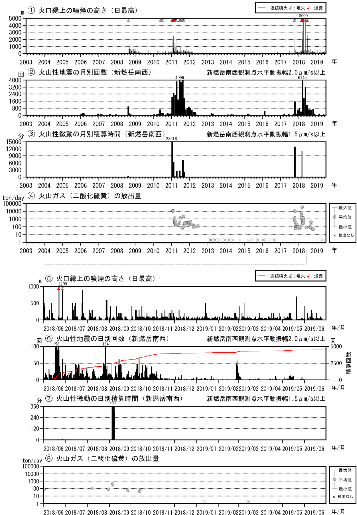
図4 霧島山（新燃岳） 火山活動経過図（2003年1月～2019年6月）
