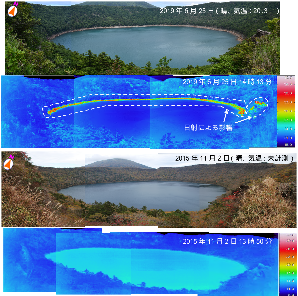
図4 霧島山 大浪池の火口湖及びその周辺の状況(2019年6月25日、大浪池火口縁から観測) 25日に大浪池で実施した現地調査では噴気等は観測されず、2015年11月2日の調査と比較して、大浪池の火口湖及びその周辺の状況に特段の変化は認められませんでした。 大浪池の水面の高さは、季節によって変動がみられています。25日は前回観測時(2015年11月2日)よりも水位が低くなっていたため、湖岸沿いに日射の影響が見られています。
