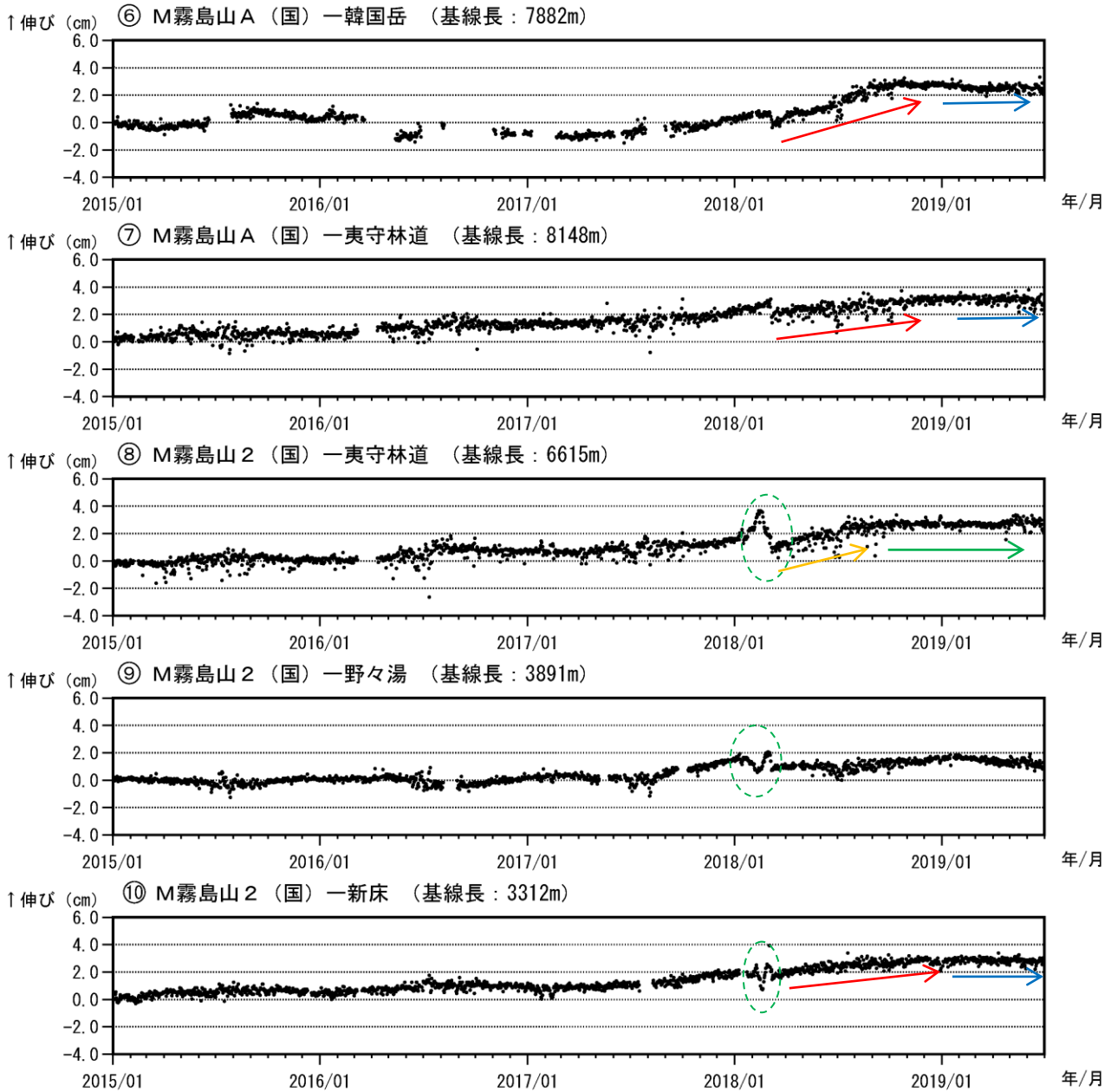
図 8-2 霧島山（えびの高原（硫黄山）周辺） GNSS 連続観測による基線長変化 (2015年1月～2019年6月)
