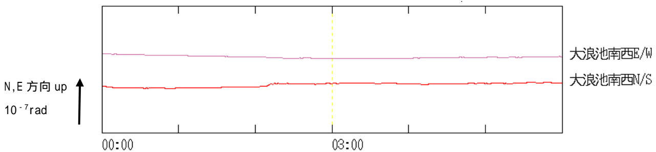
図3 霧島山 大浪池南西観測点の傾斜変動（2019年6月25日00時～06時、分値）
