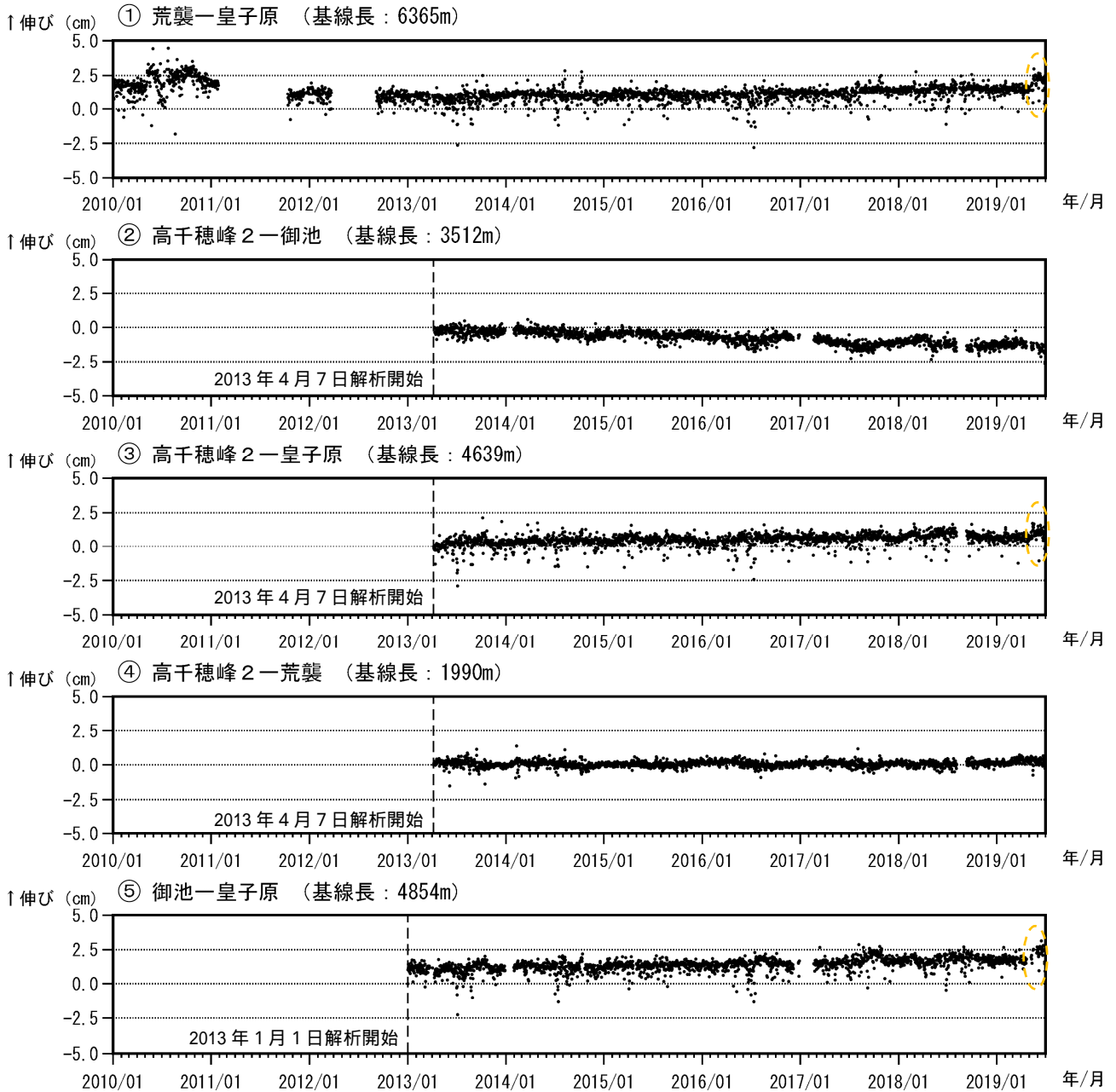
図4 霧島山（御鉢） GNSS連続観測による基線長変化（2010年1月～2019年6月）
