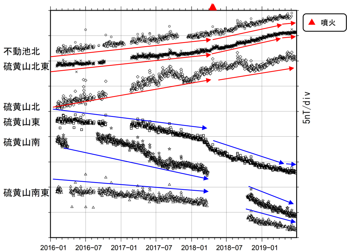
図 12 霧島山（えびの高原（硫黄山）周辺） 全磁力観測点で観測された全磁力変動 （2016 年 2 月～2019 年 6 月）
