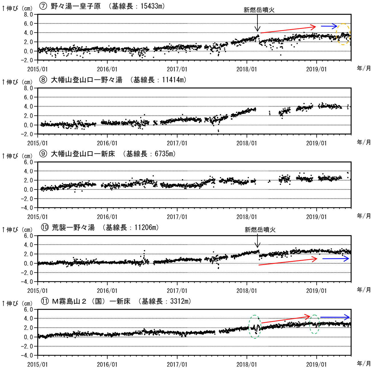
図 7-2 霧島山（新燃岳） GNSS 連続観測による基線長変化（2015 年 1 月～2019 年 6 月）
