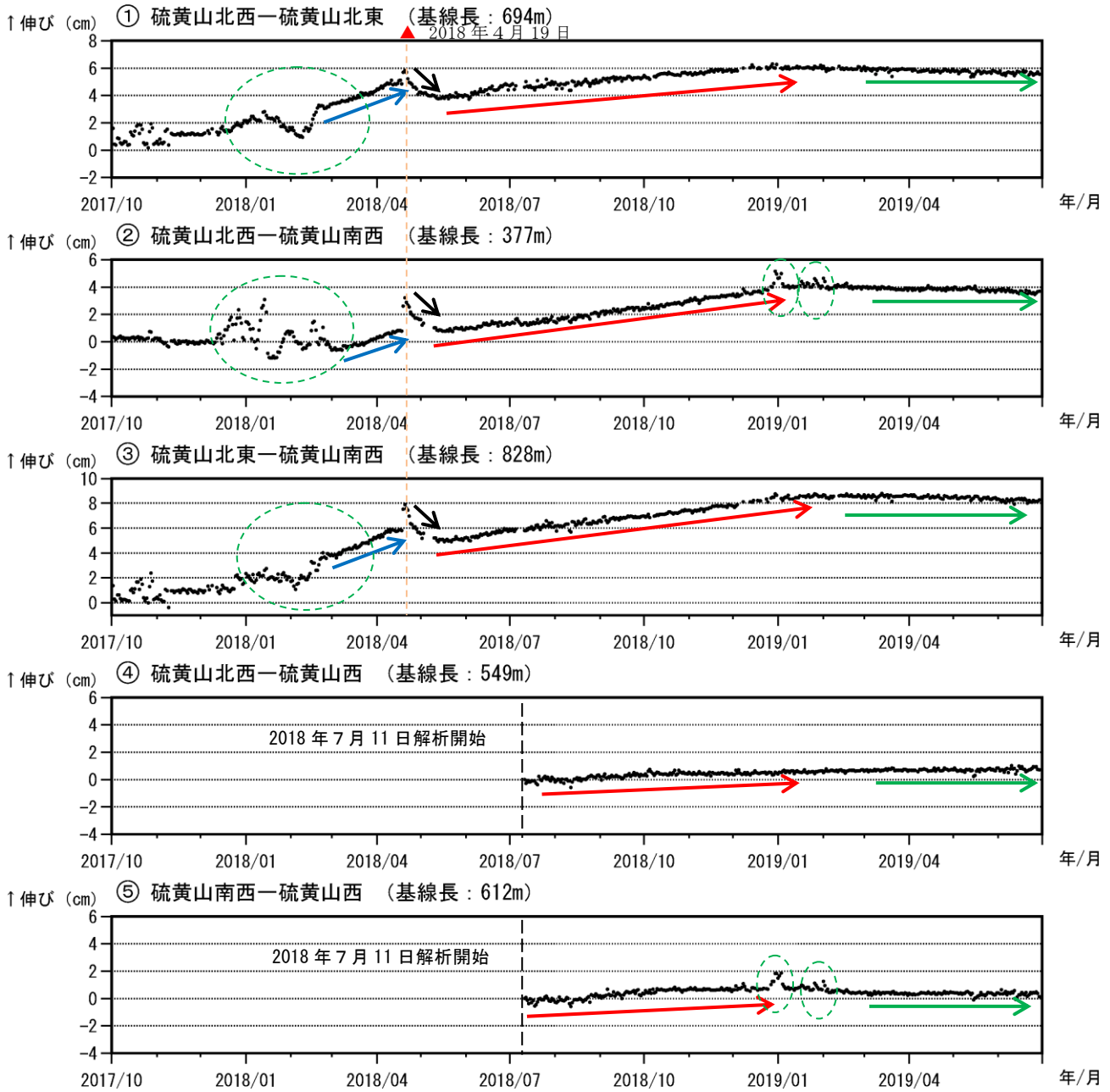
図7 霧島山（えびの高原（硫黄山）周辺） GNSS 連続観測による基線長変化 （2017年10月～2019年6月）
