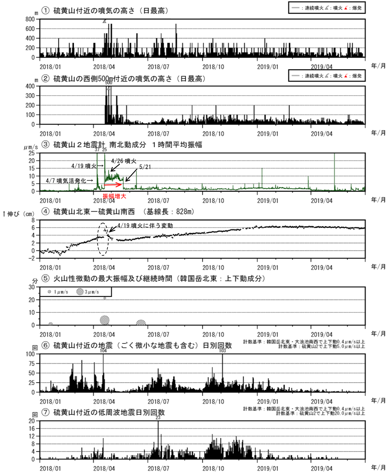
図5 霧島山（えびの高原（硫黄山）周辺） 火山活動経過図（2018年1月～2019年6月）
