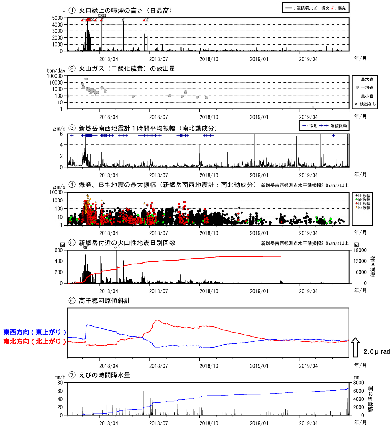
図5 霧島山（新燃岳） 火山活動経過図（2018年2月～2019年6月）
