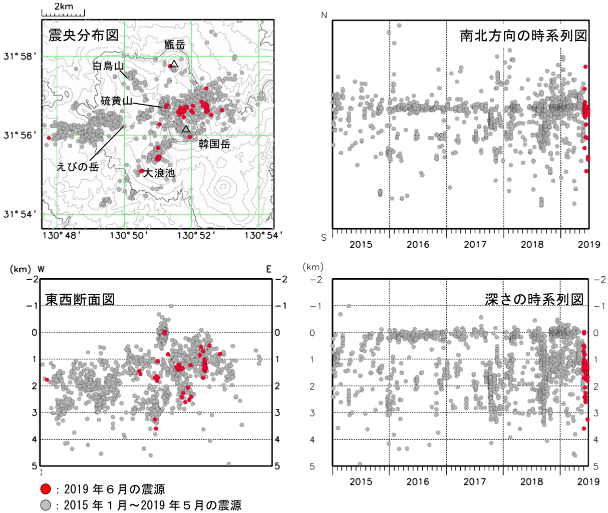
図4 霧島山（えびの高原（硫黄山）周辺） 震源分布図（2015年1月～2019年6月）
