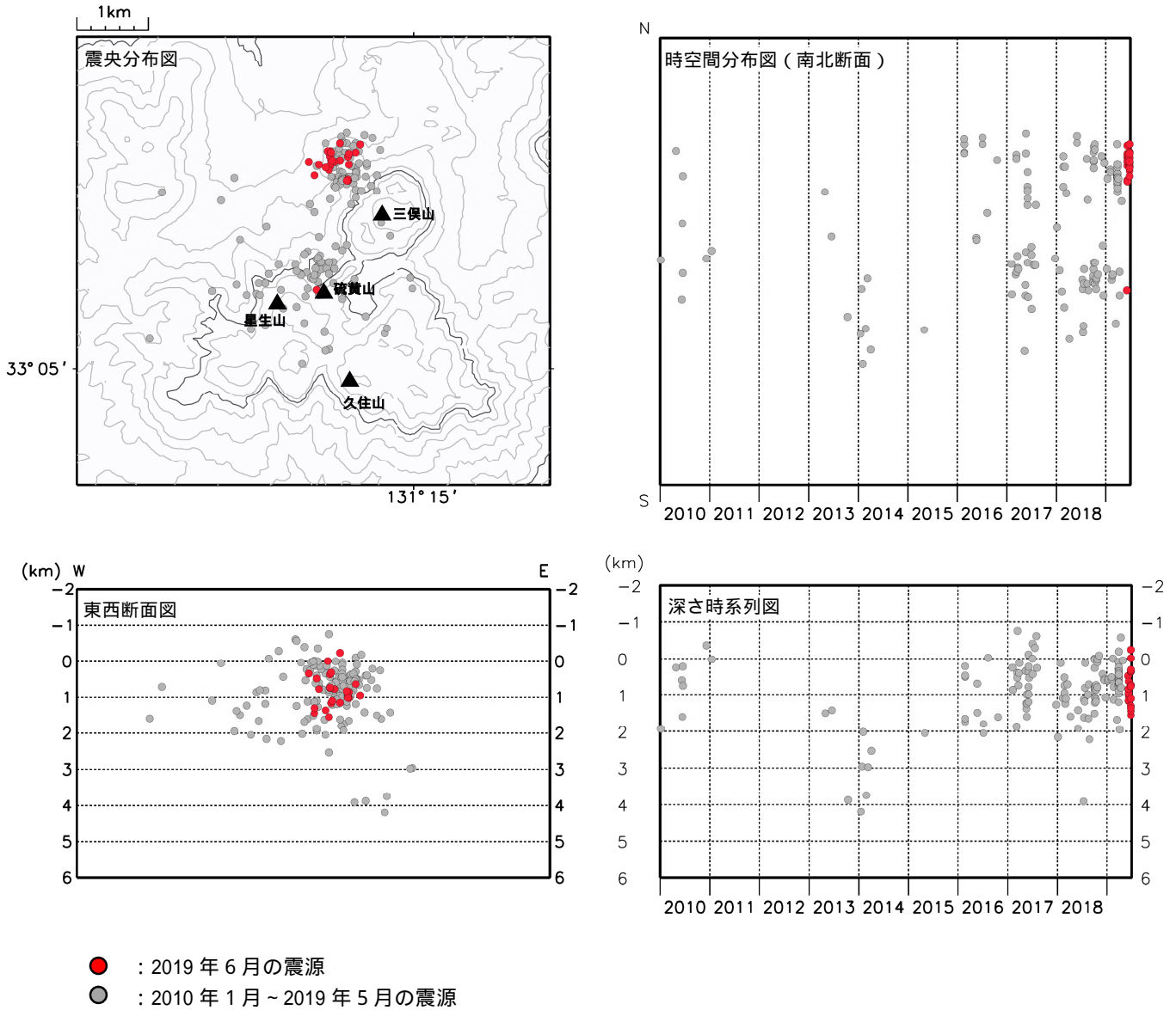
図 4-1 九重山 震源分布図（硫黄山付近の火山性地震）（2010年1月～2019年6月）
