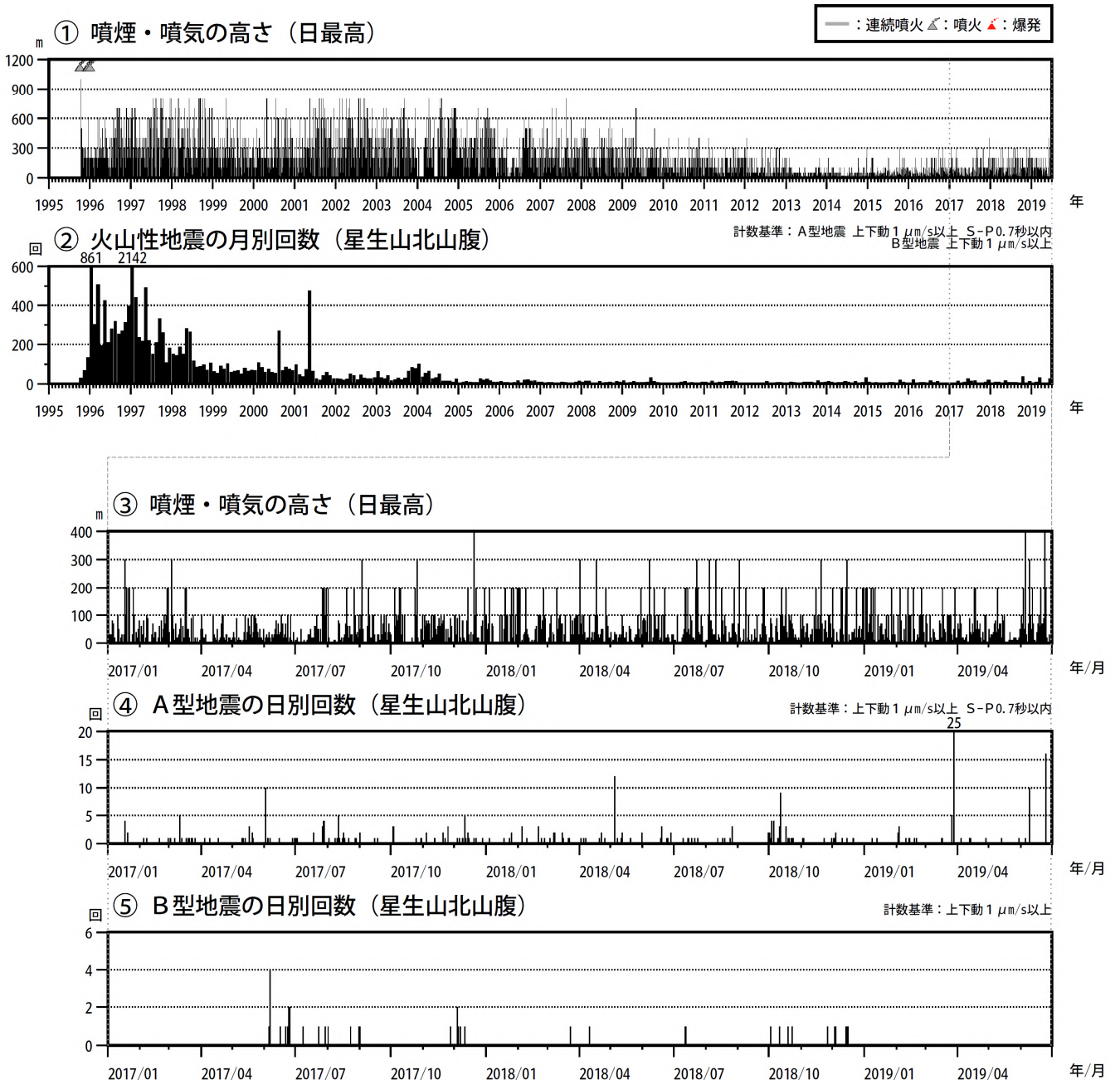
図3 九重山 火山活動経過図（1995年10月～2019年6月）
