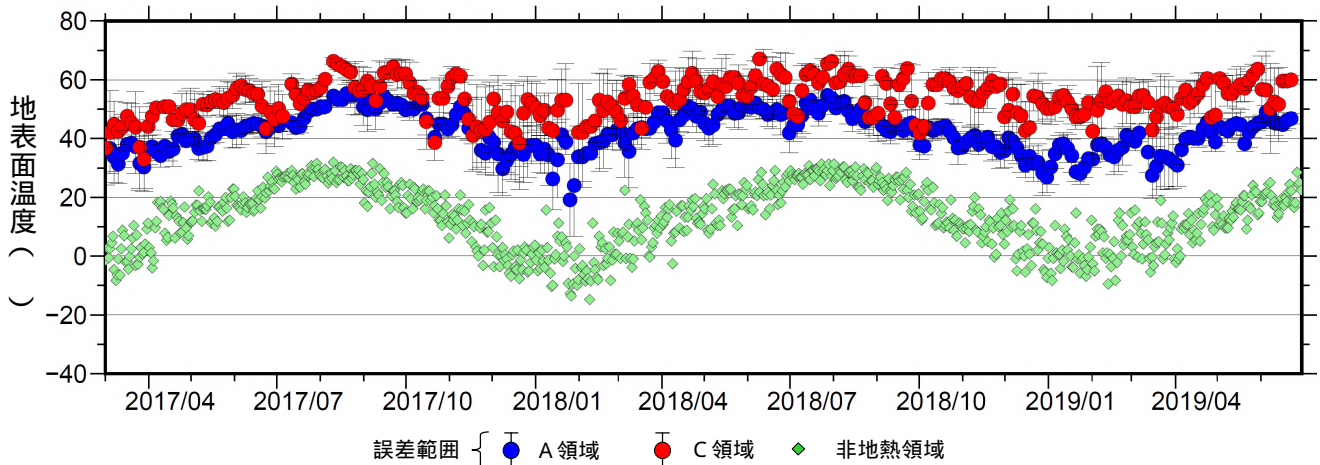
図2-2 九重山 星生山北尾根赤外熱映像装置による日別最高温度の7日間移動平均値 (2017年3月～2019年6月)
