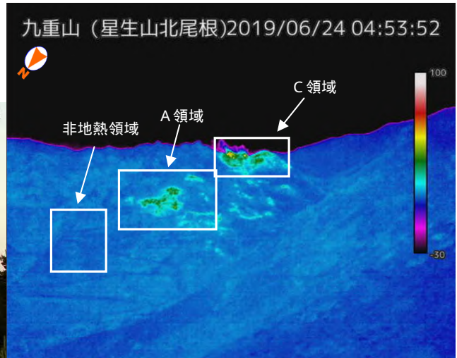
図2-1 九重山 地熱域の状況 (6月24日 星生山北尾根赤外熱映像装置による)
