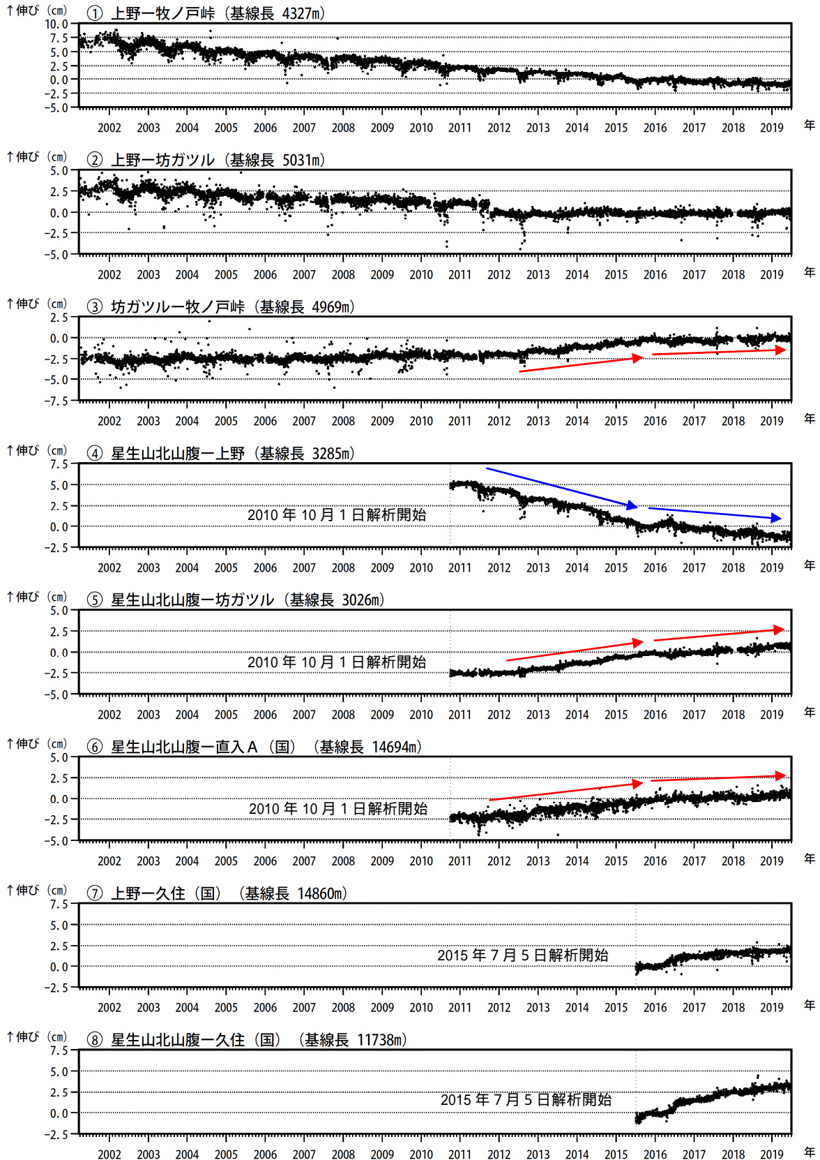
図8 九重山 GNSS連続観測による基線長変化（2001年3月～2019年6月）
