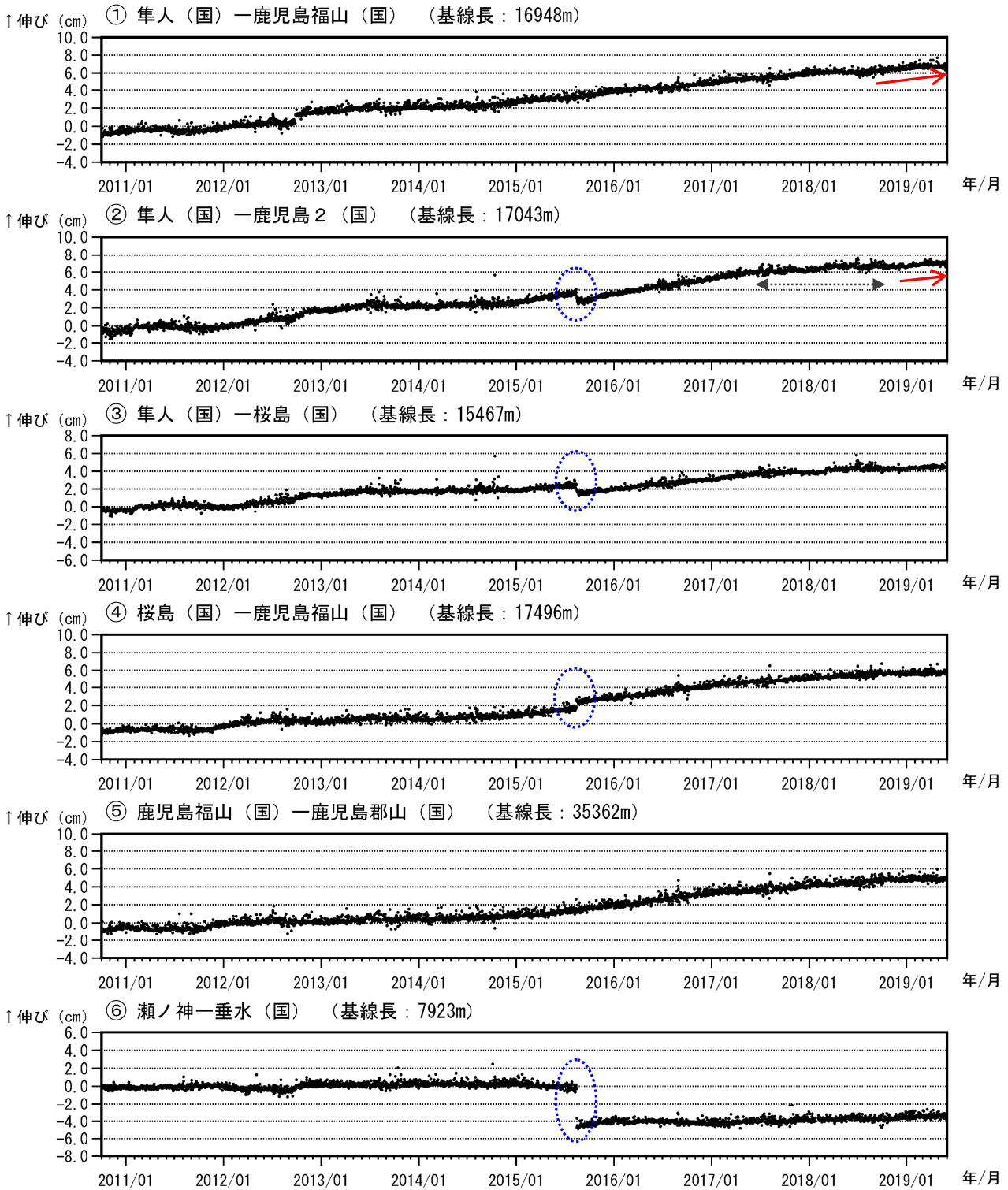
図 6-1 桜島 GNSS 連続観測による基線長変化（2010年10月～2019年5月）
