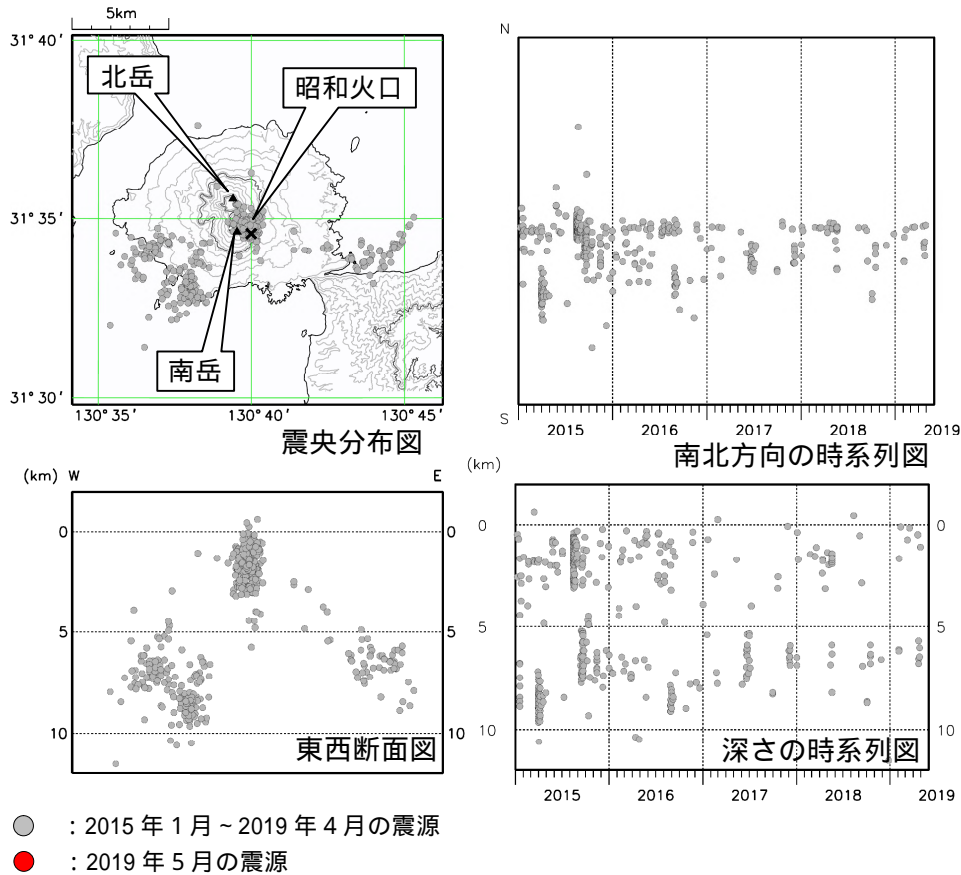
図4 桜島 震源分布図（2015年1月～2019年5月）
