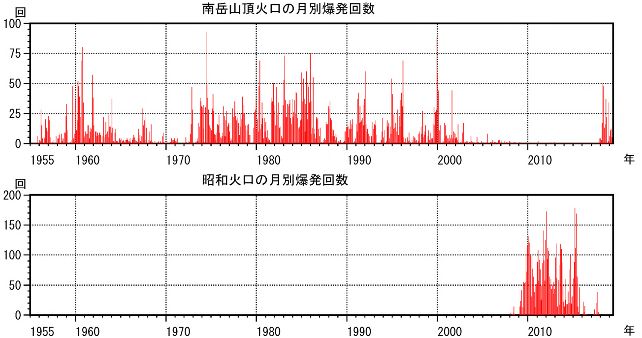
図 2-1 桜島 南岳山頂火口（上図）と昭和火口（下図）の月別爆発回数 （1955年1月～2019年5月）
