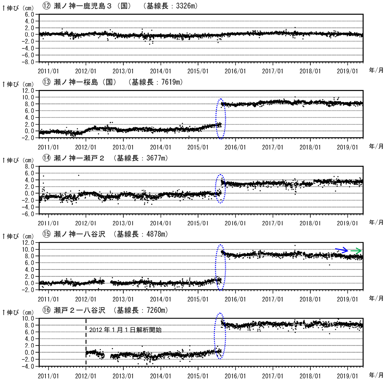
図 6-3 桜島 GNSS 連続観測による基線長変化 (2010 年 10 月 ~ 2019 年 5 月)
