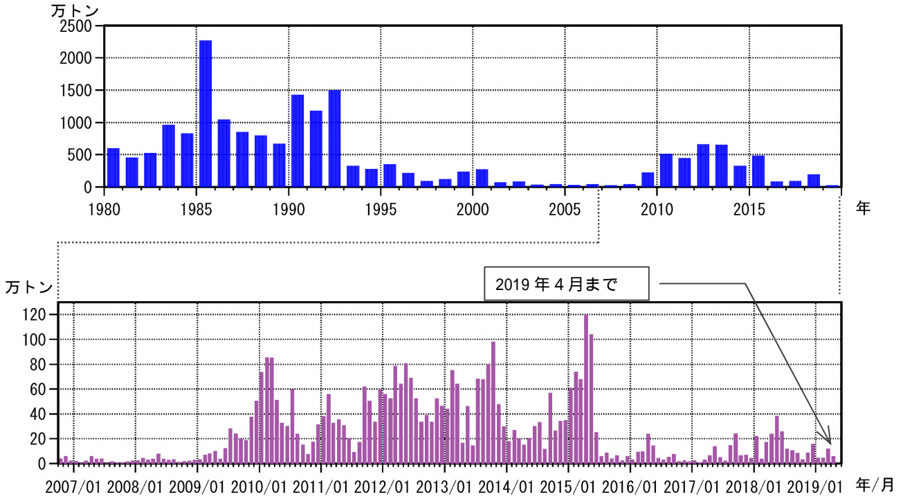
図8 桜島 鹿児島県が実施している降灰の観測データから推定した火山灰の総噴出量 （上段：1980年1月～2019年4月の年別値、下段：2006年10月～2019年4月の月別値）
