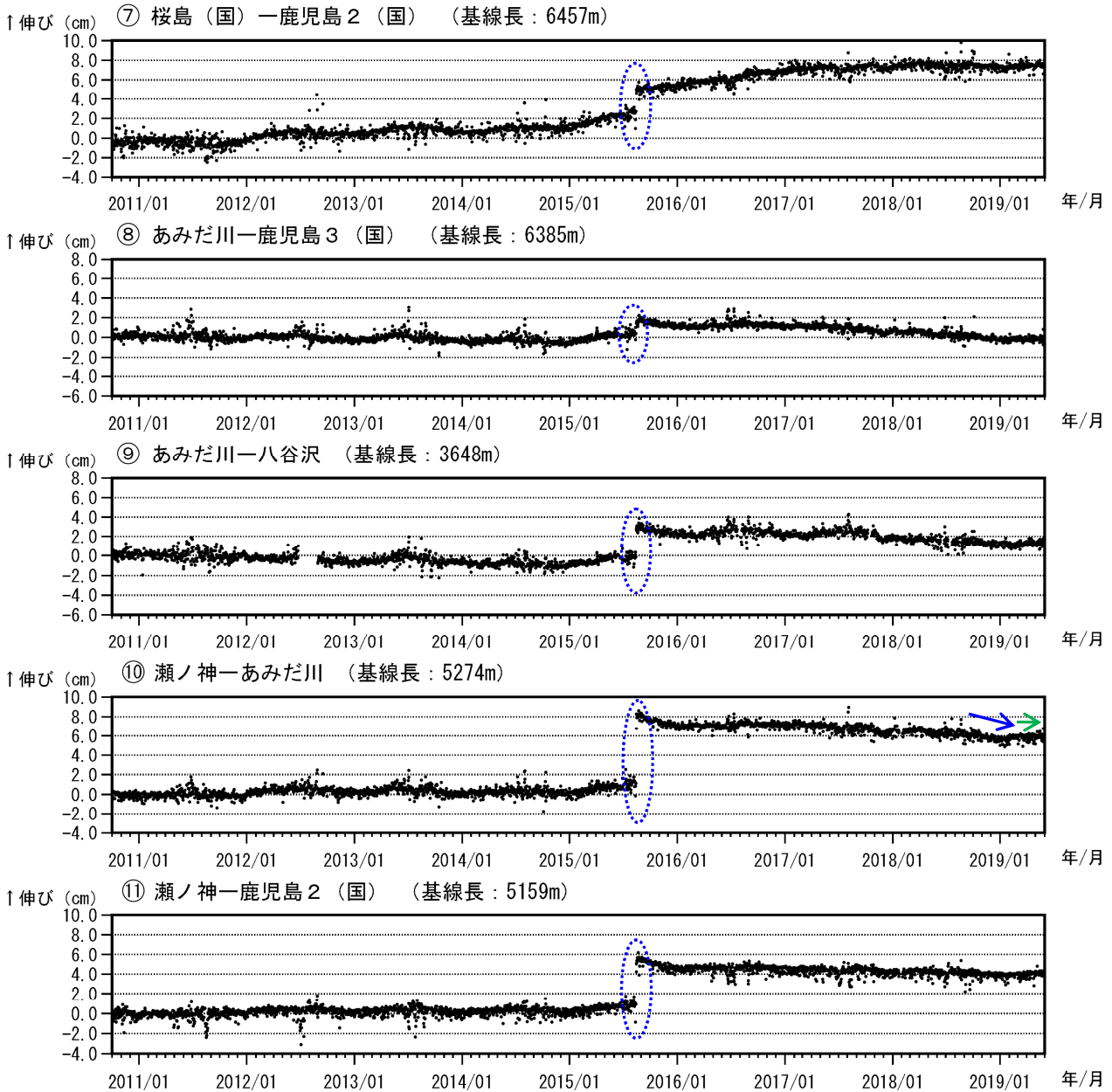
図 6-2 桜島 GNSS 連続観測による基線長変化（2010年10月～2019年5月）
