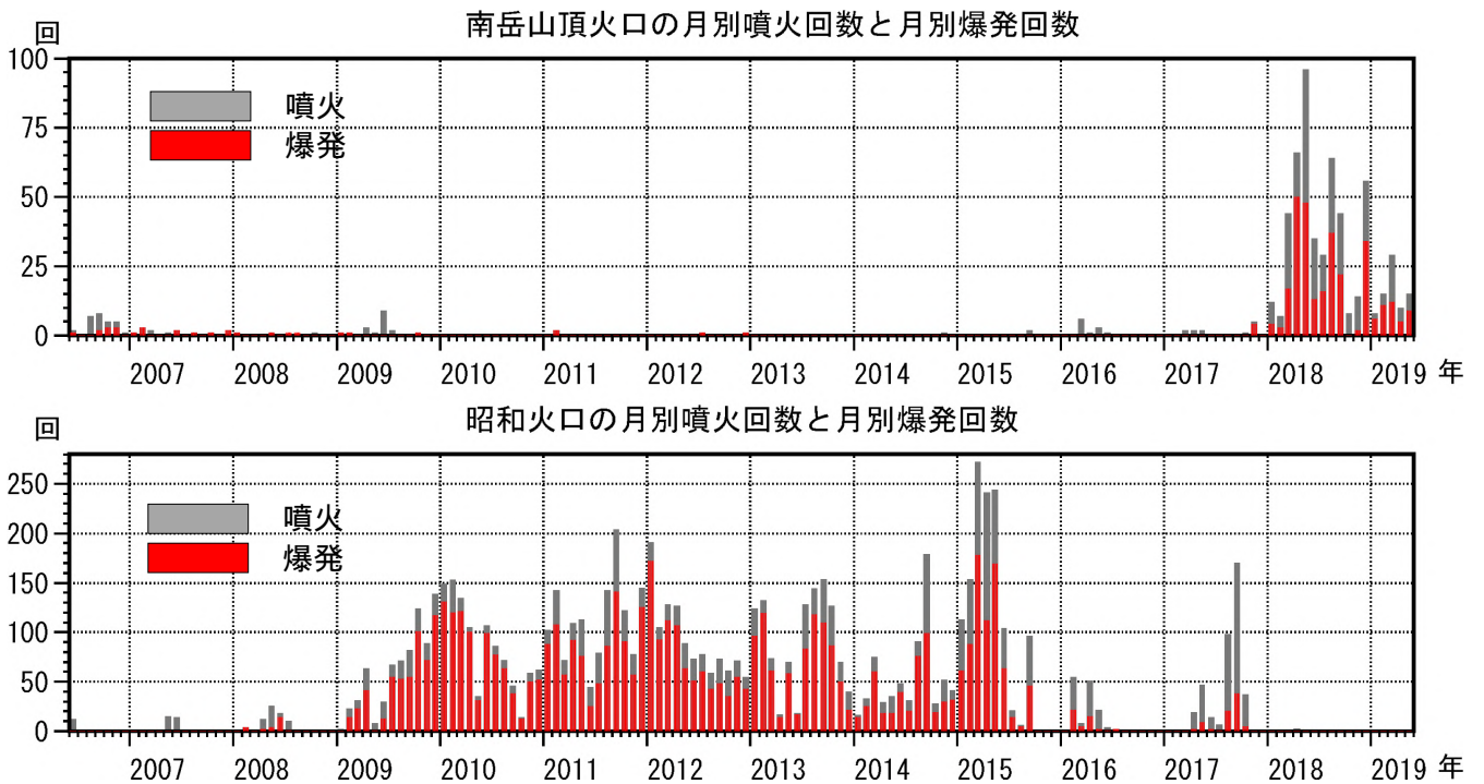
図 2-2 桜島 南岳山頂火口（上図）と昭和火口（下図）の月別噴火回数と月別爆発回数 （2006年6月～2019年5月）
