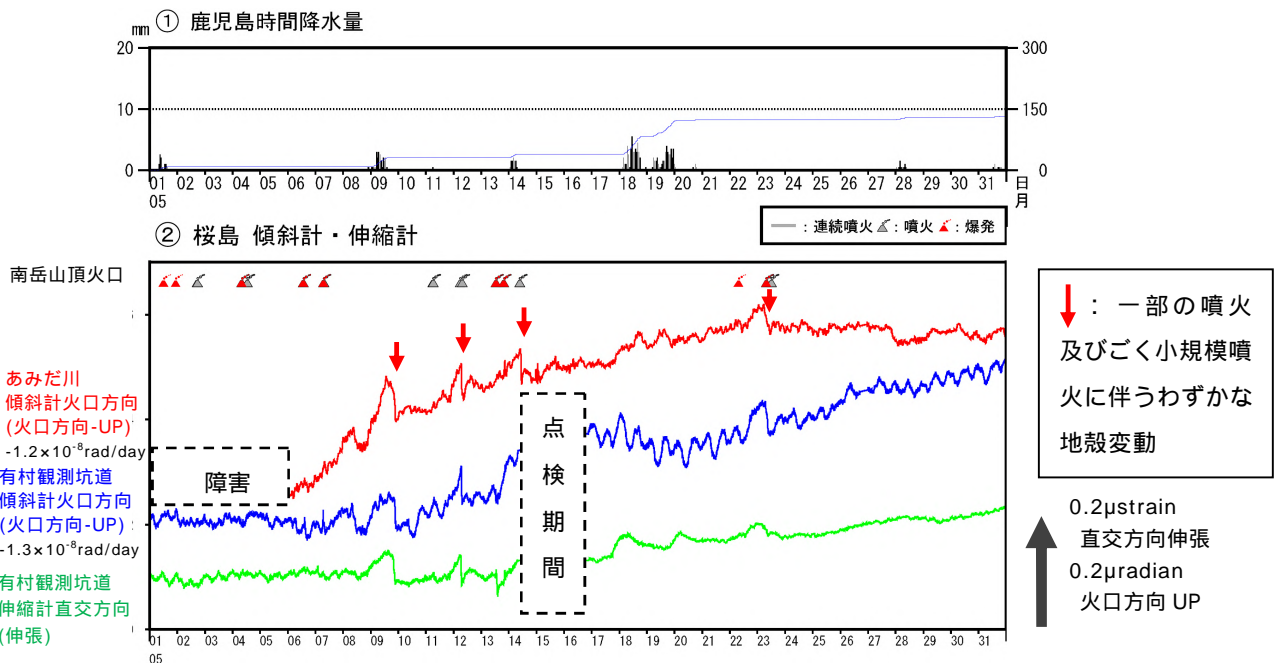
図5 桜島 傾斜計及び伸縮計による地殻変動の状況（2019年5月1日～5月31日）
