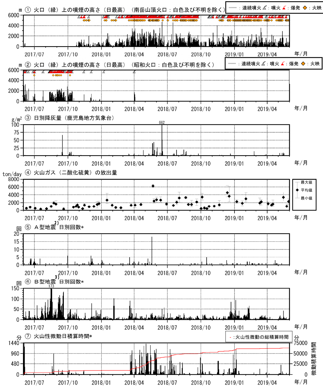
図3 桜島 最近2年間の活動経過図（2017年6月～2019年5月）
