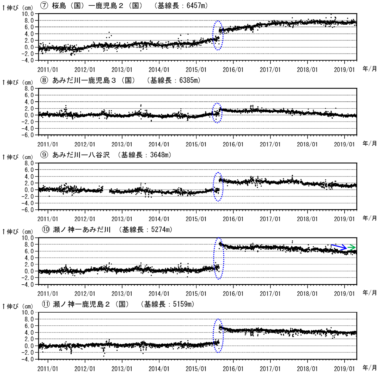
図 6-2 桜島 GNSS 連続観測による基線長変化（2010 年 10 月～2019 年 4 月）
