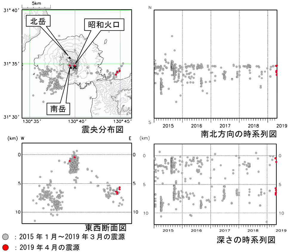
図 4 桜島 震源分布図（2015 年 1 月～2019 年 4 月）
