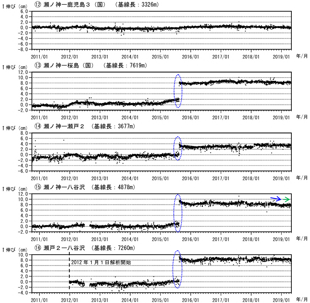
図 6-3 桜島 GNSS 連続観測による基線長変化（2010 年 10 月～2019 年 4 月）
