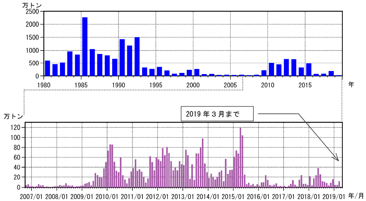
図 8 桜島 鹿児島県が実施している降灰の観測データから推定した火山灰の総噴出量 （上段：1980 年 1 月～2019 年 3 月の年別値、下段：2006 年 10 月～2019 年 3 月の月別値）
