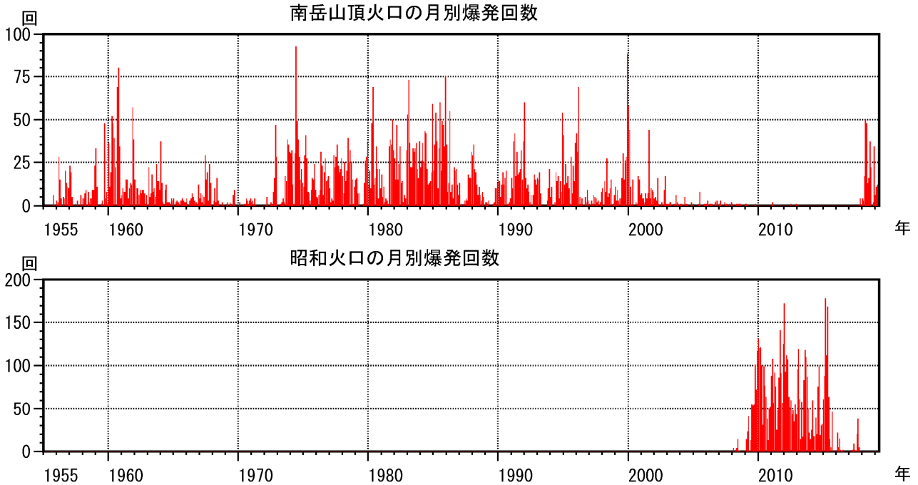
図 2-1 桜島 南岳山頂火口（上図）と昭和火口（下図）の月別爆発回数 （1955 年 1 月～2019 年 4 月）
