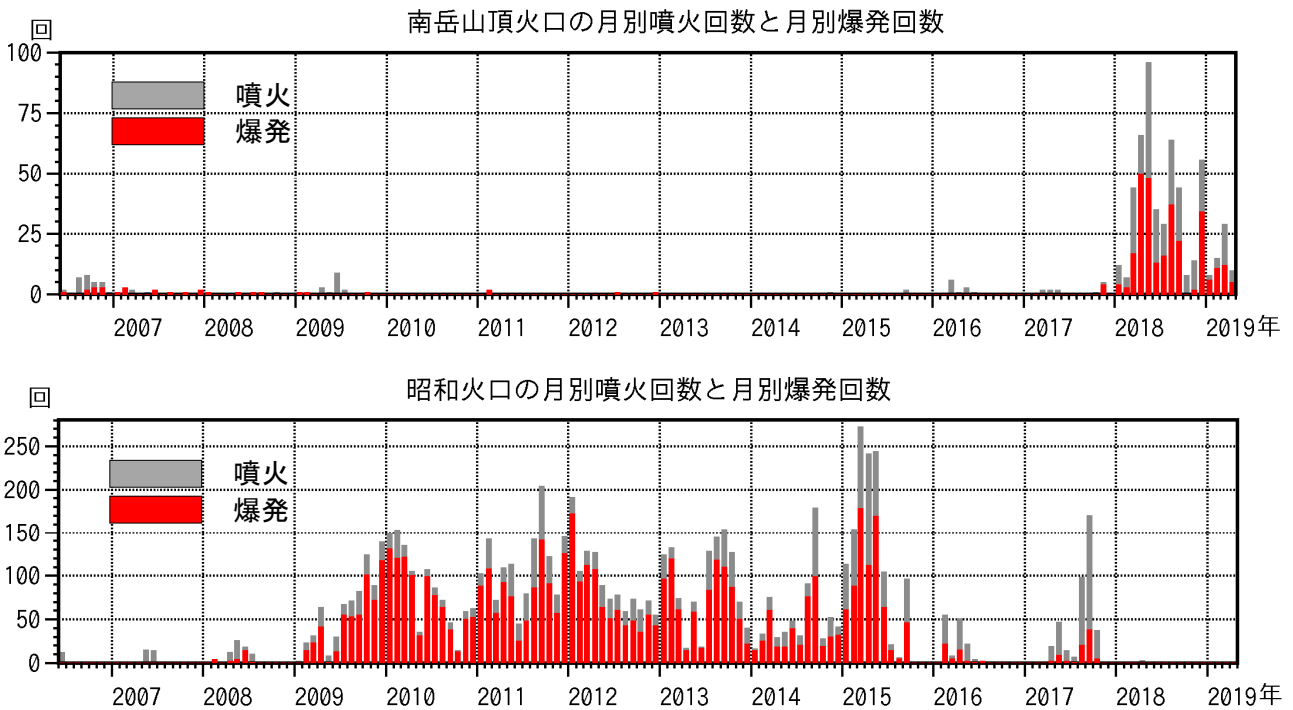
図 2-2 桜島 南岳山頂火口（上図）と昭和火口（下図）の月別噴火回数と月別爆発回数 （2006 年 6 月～2019 年 4 月）
