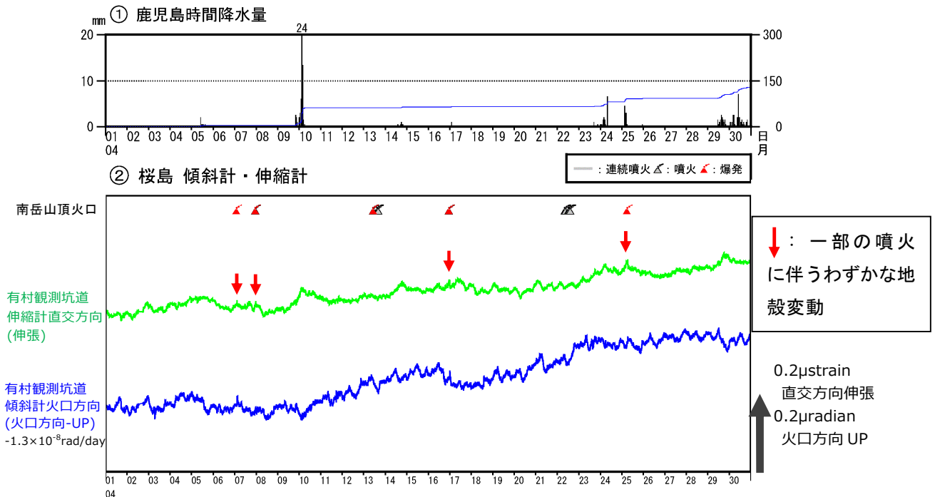
図 5 桜島 傾斜計及び伸縮計による地殻変動の状況（2019 年 4 月 1 日～4 月 30 日）
