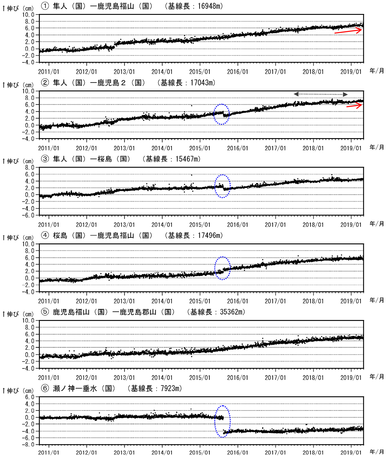
図 6-1 桜島 GNSS 連続観測による基線長変化 (2010 年 10 月～2019 年 4 月)
