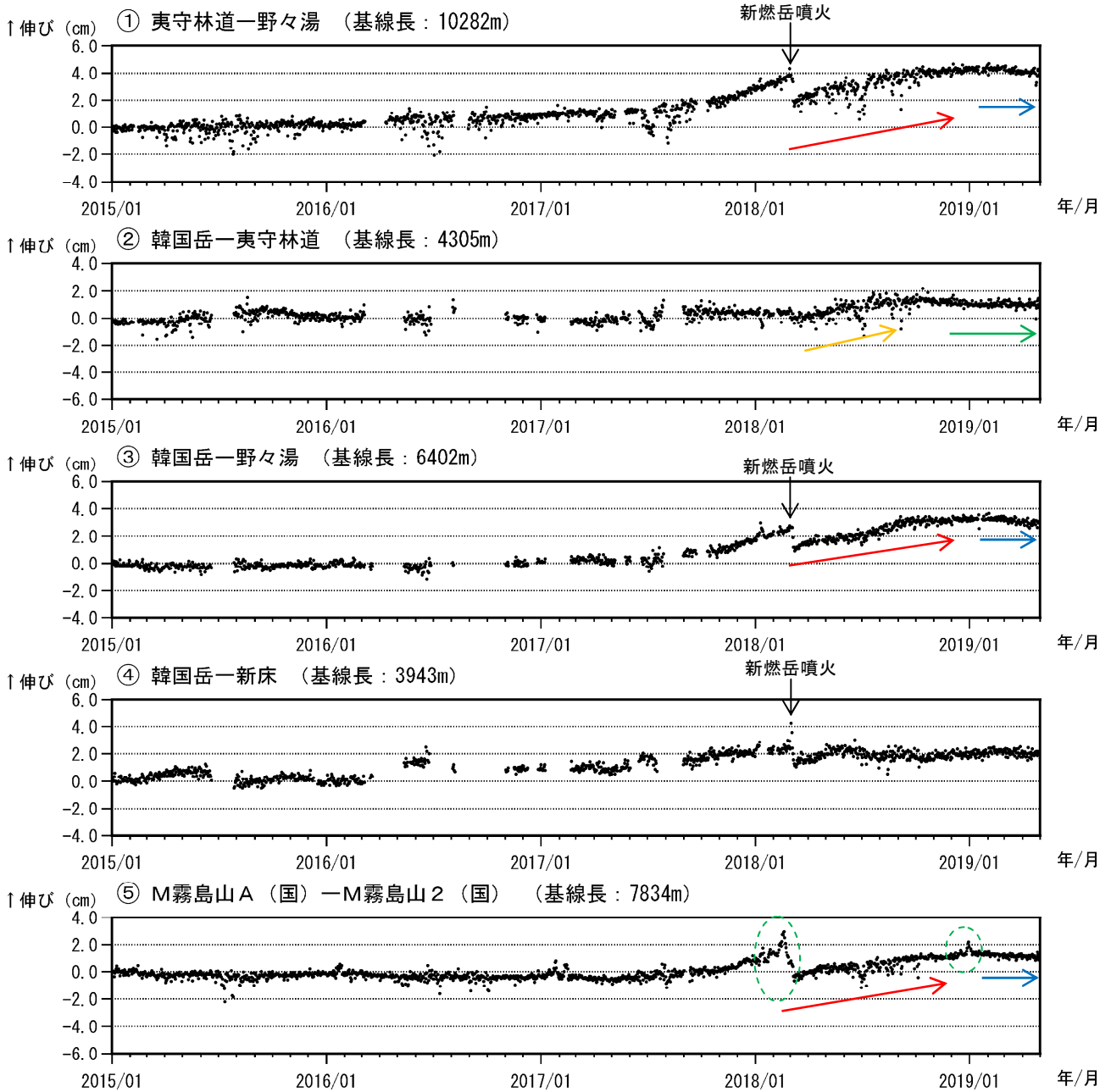
図 13-1 霧島山（えびの高原（硫黄山）周辺） GNSS 連続観測による基線長変化 (2015 年 1 月～2019 年 4 月)
