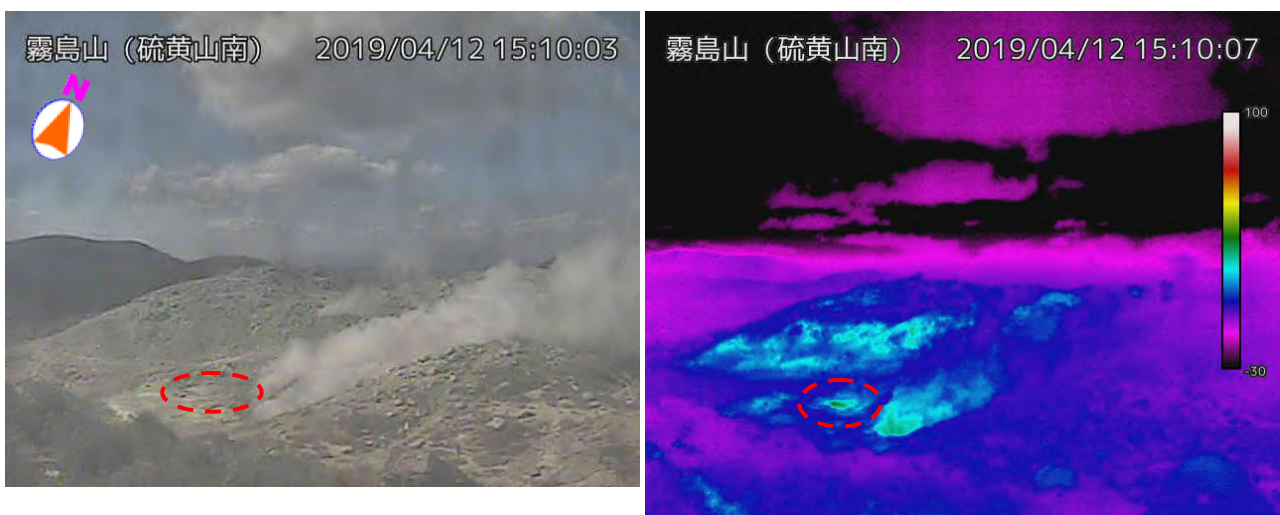
図 1-2 霧島山（えびの高原（硫黄山）周辺） 硫黄山南側の状況 （4月12日、硫黄山南監視カメラによる）
