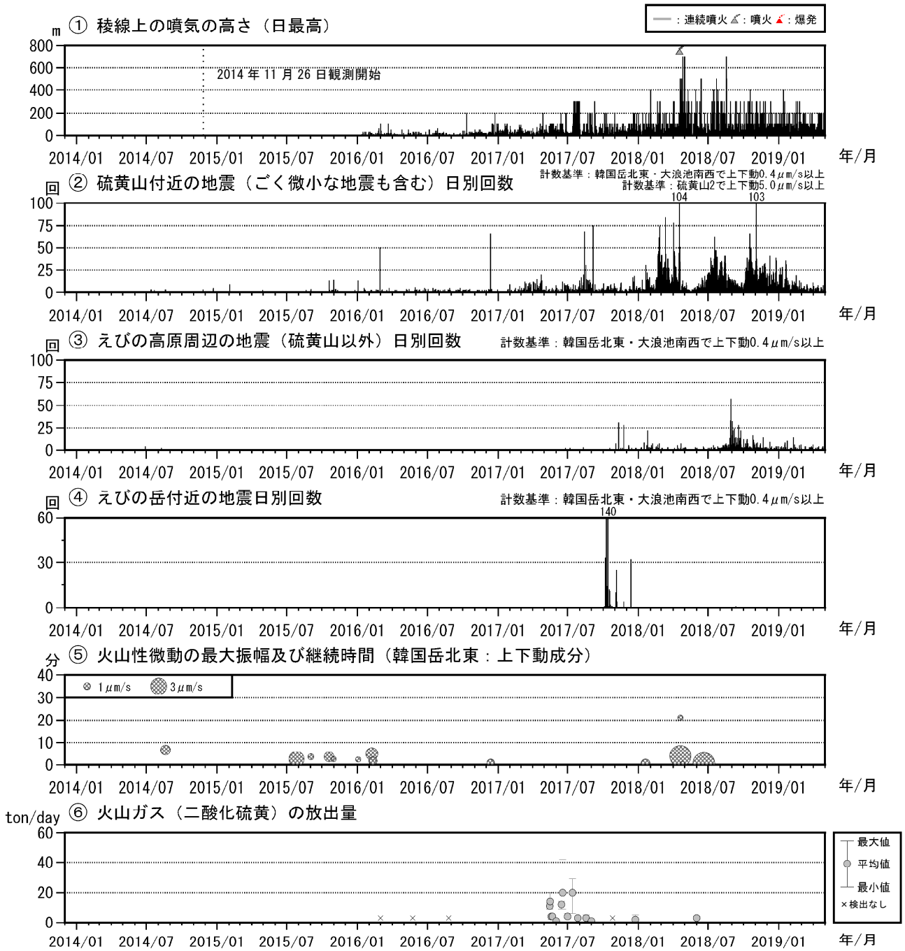
図 10 霧島山（えびの高原（硫黄山）周辺） 火山活動経過図（2013 年 12 月～2019 年 4 月）
