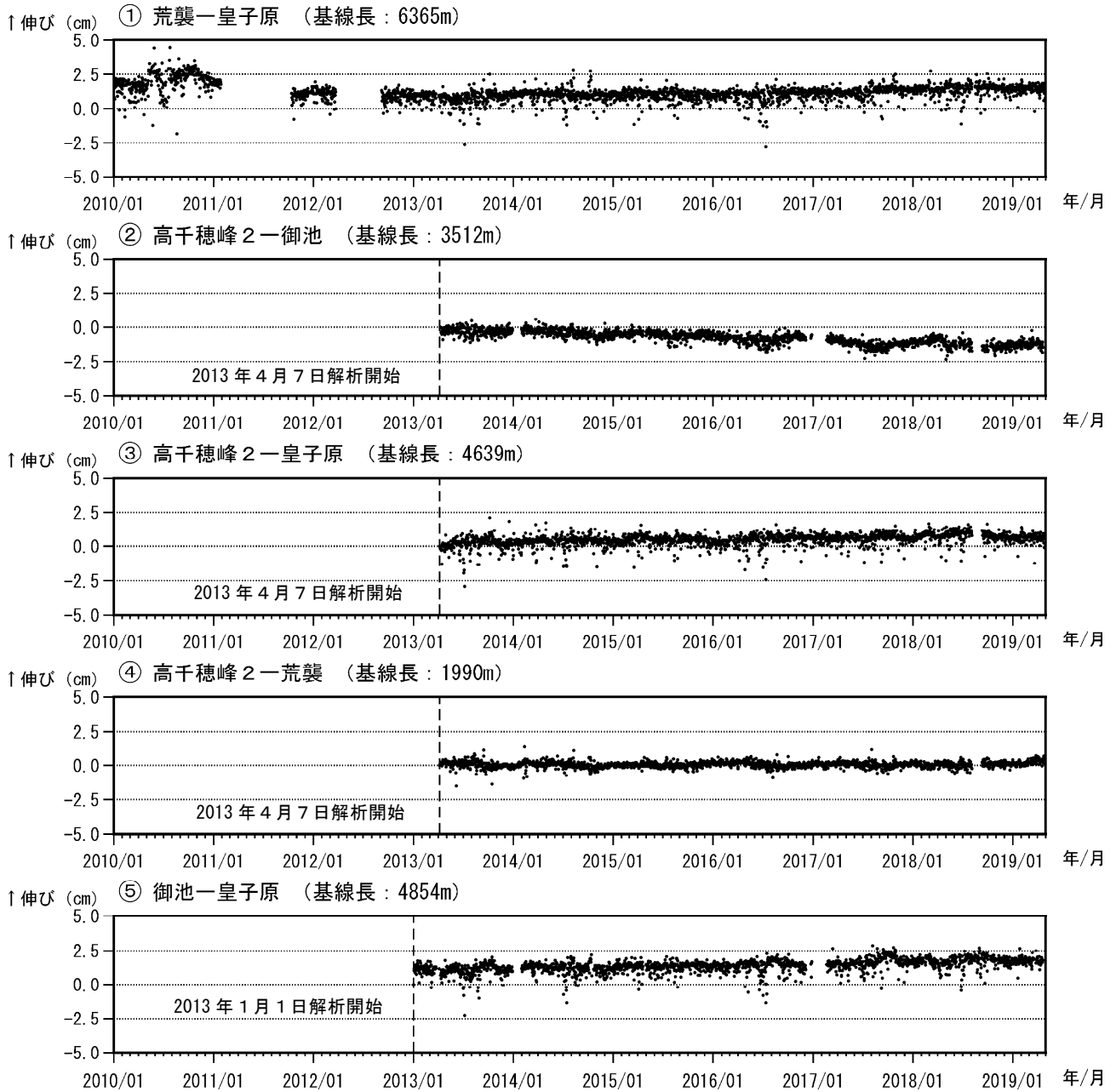
図4 霧島山（御鉢） GNSS 連続観測による基線長変化（2010年1月～2019年4月）
