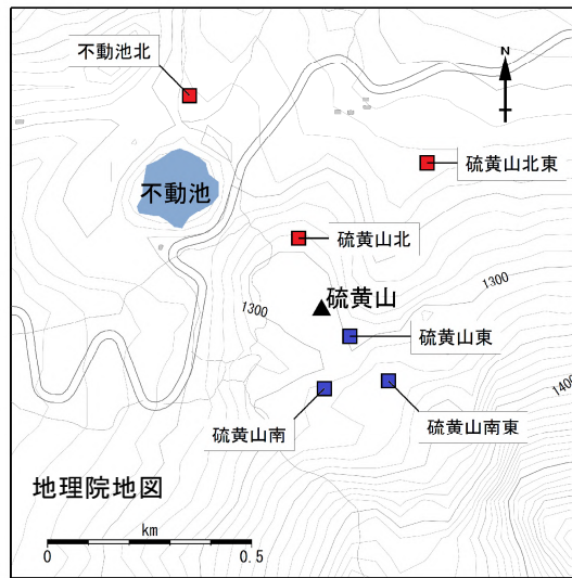
図 15 霧島山（えびの高原（硫黄山）周辺） 全磁力観測点配置図
