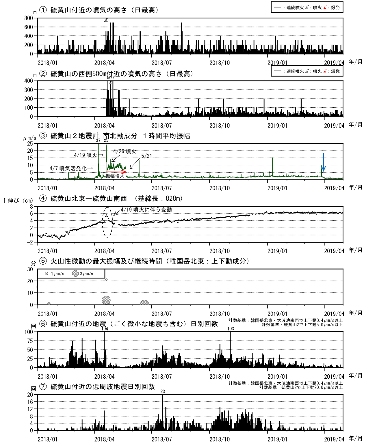
図9 霧島山（えびの高原（硫黄山）周辺）火山活動経過図（2018年1月～2019年4月）
