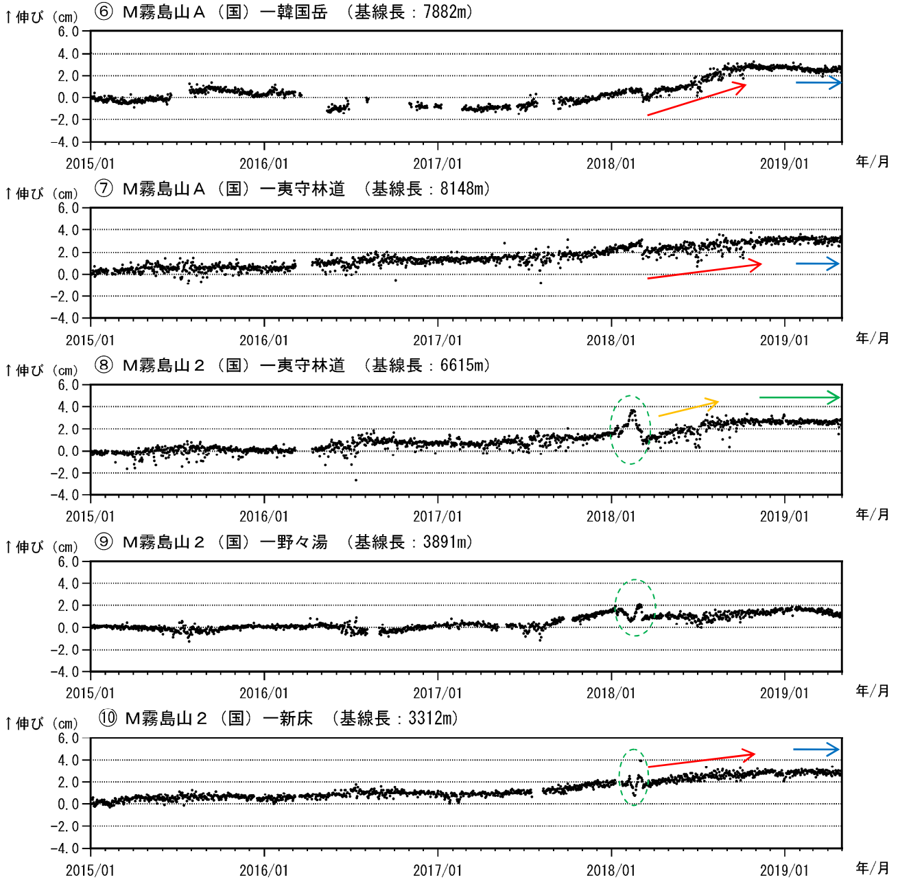
図 13-2 霧島山（えびの高原（硫黄山）周辺） GNSS 連続観測による基線長変化 (2015 年 1 月～2019 年 4 月)
