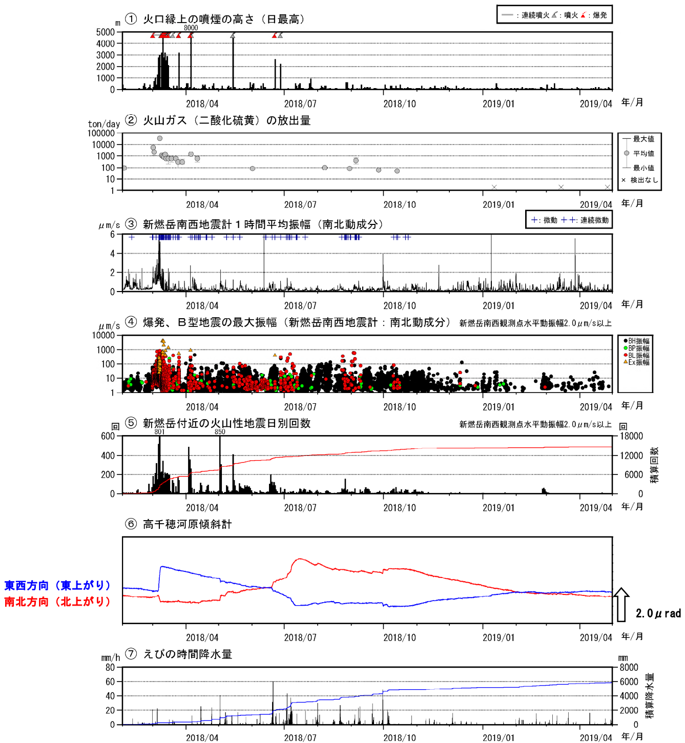
図5 霧島山（新燃岳） 火山活動経過図（2018年2月～2019年4月）
