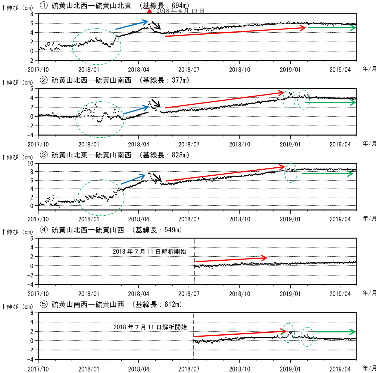
図 11 霧島山（えびの高原（硫黄山）周辺） GNSS 連続観測による基線長変化 （2017 年 10 月～2019 年 4 月）
