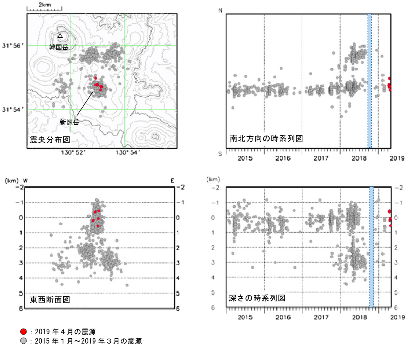
図 6 霧島山（新燃岳） 震源分布図（2015 年 1 月～2019 年 4 月）
