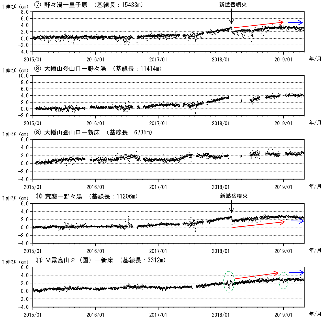
図 7-2 霧島山（新燃岳） GNSS 連続観測による基線長変化（2015 年 1 月～2019 年 4 月）
