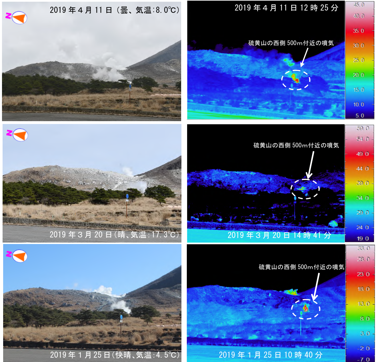
図4 霧島山（えびの高原（硫黄山）周辺） 硫黄山の状況（えびの高原（図7参照）から観測） ・硫黄山の南側の噴気地帯では、引き続き活発な噴気を確認しました。硫黄山の西側500m付近では引き続きやや活発な噴気活動がみられています。 ・硫黄山付近では引き続き地熱域を確認しましたが、これまでの観測と比べ特段の変化は認められませんでした。
