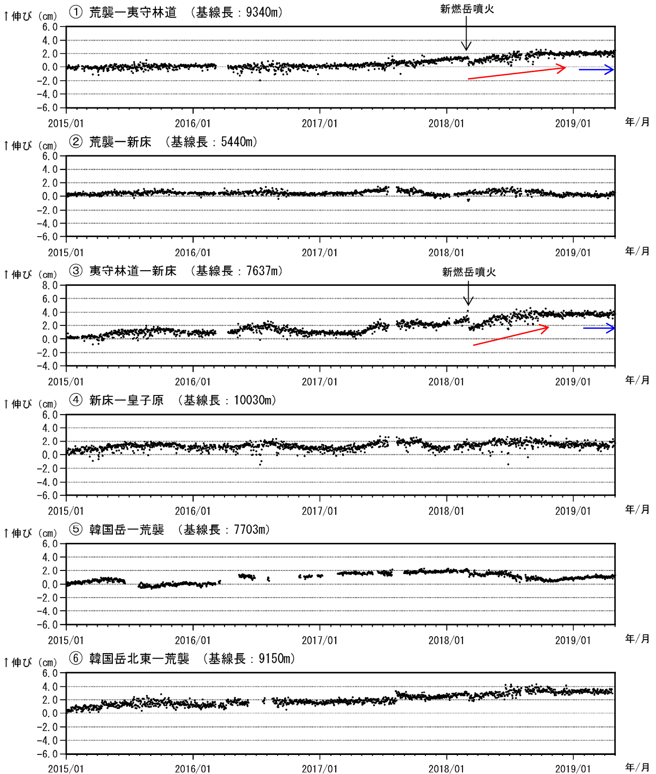
図 7-1 霧島山（新燃岳） GNSS 連続観測による基線長変化（2015 年 1 月～2019 年 4 月）
