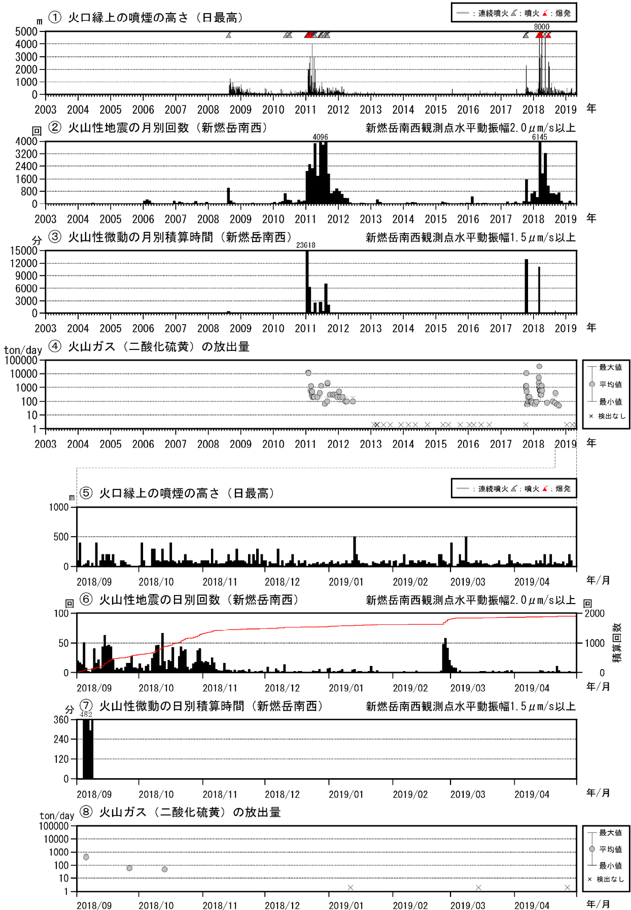
図 4 霧島山（新燃岳） 火山活動経過図（2003 年 1 月～2019 年 4 月）
