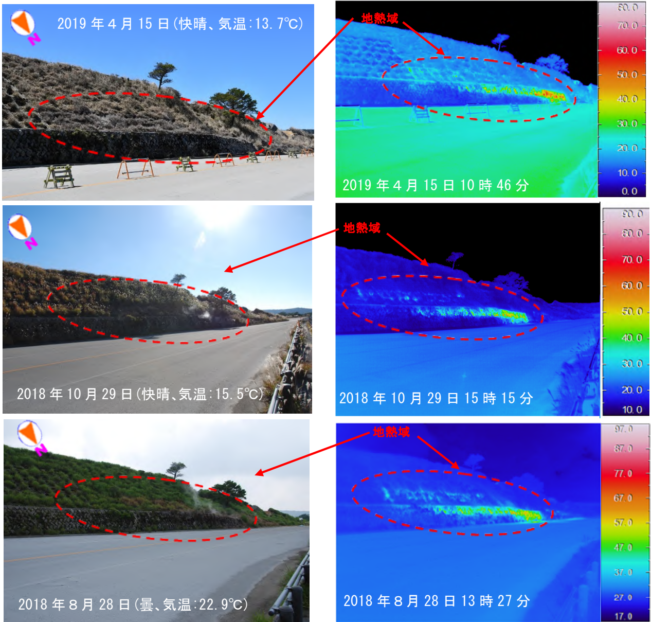
図6 霧島山（えびの高原（硫黄山）周辺） 硫黄山北西斜面周辺の状況 （えびの高原（図7参照）から観測） 硫黄山北西斜面で引き続き地熱域及び噴気を確認しました（赤破線）。
