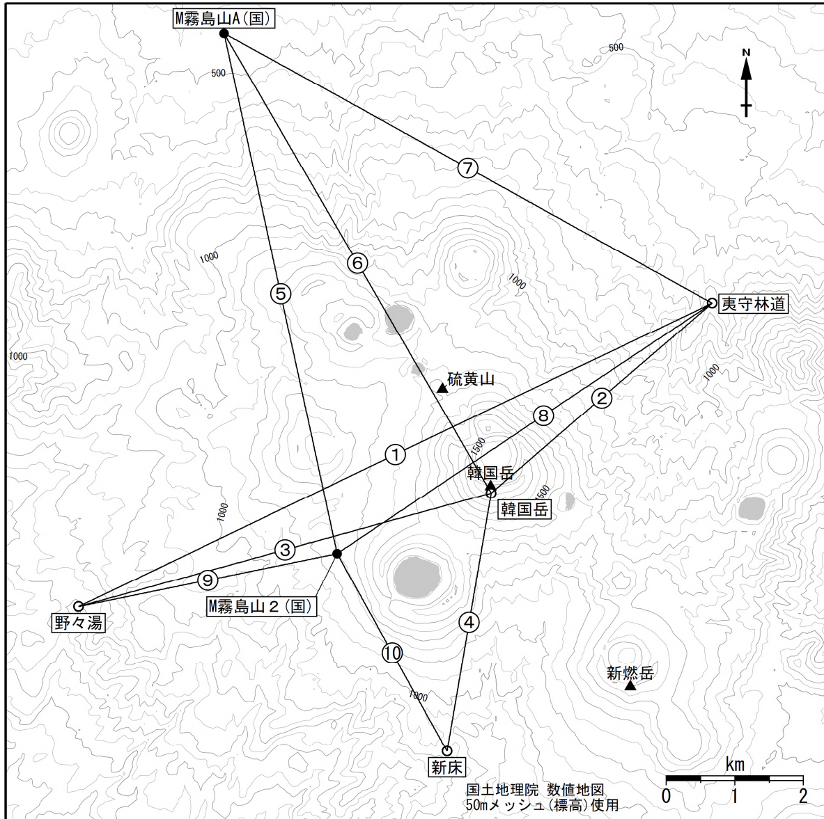
図 14 霧島山（えびの高原（硫黄山）周辺） 図 13 の GNSS 連続観測点と基線番号
