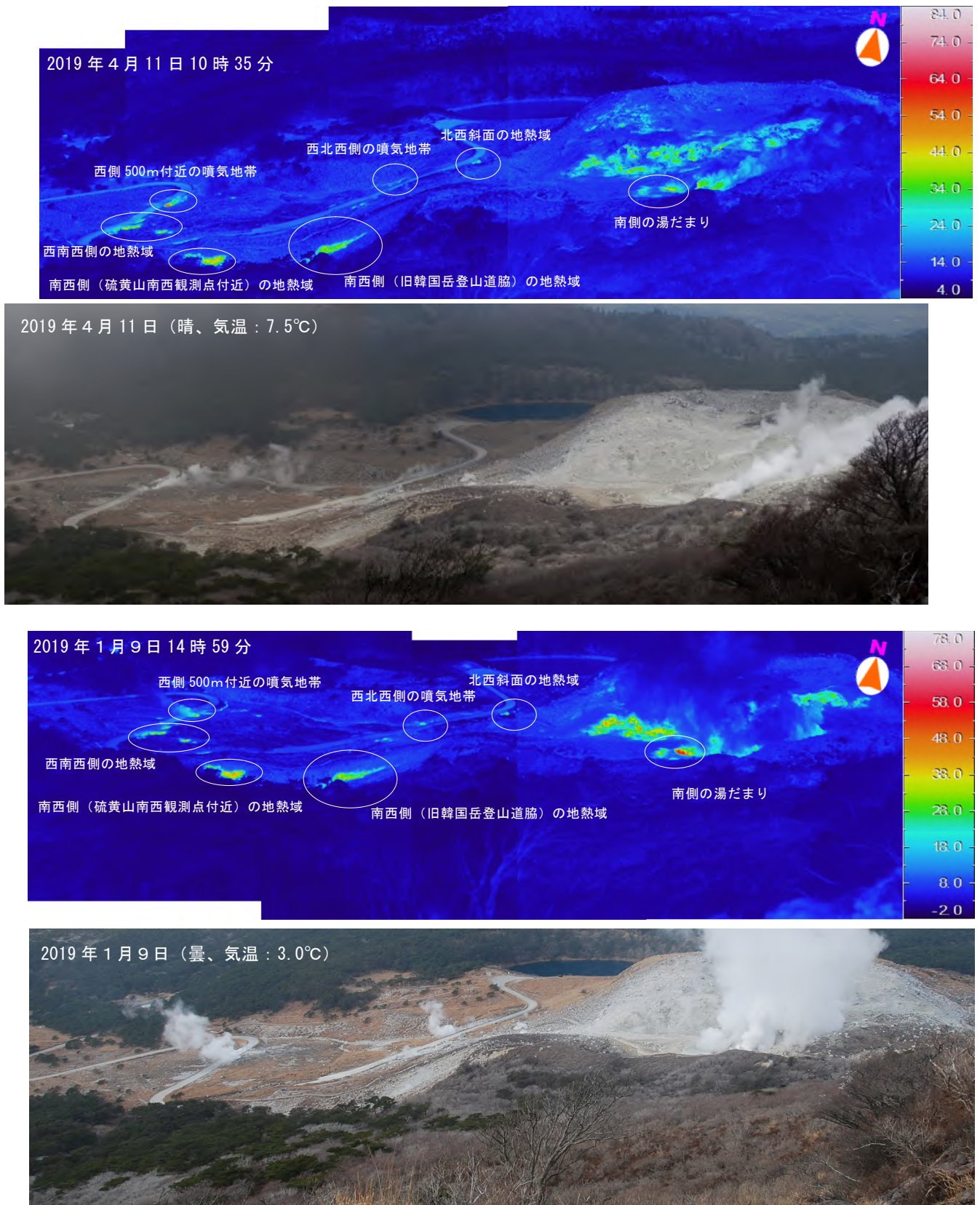
図 3 霧島山 (えびの高原 (硫黄山) 周辺) 硫黄山南側及び南西側斜面の状況
