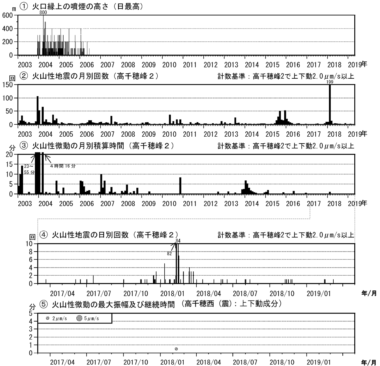
図2 霧島山（御鉢） 火山活動経過図（2003年1月～2019年4月）
