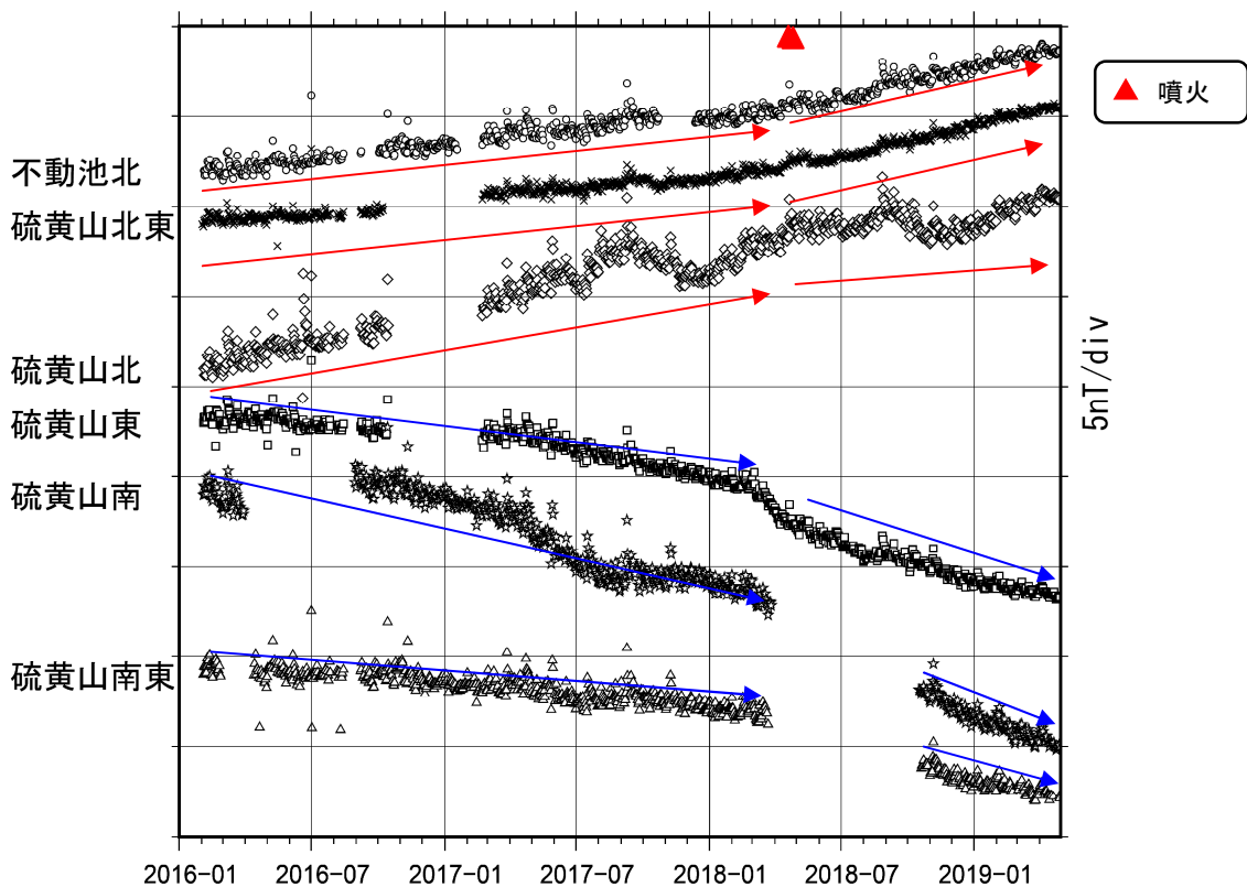
図 16 霧島山（えびの高原（硫黄山）周辺） 全磁力観測点で観測された全磁力変動 （2016 年 2 月～2019 年 4 月）
