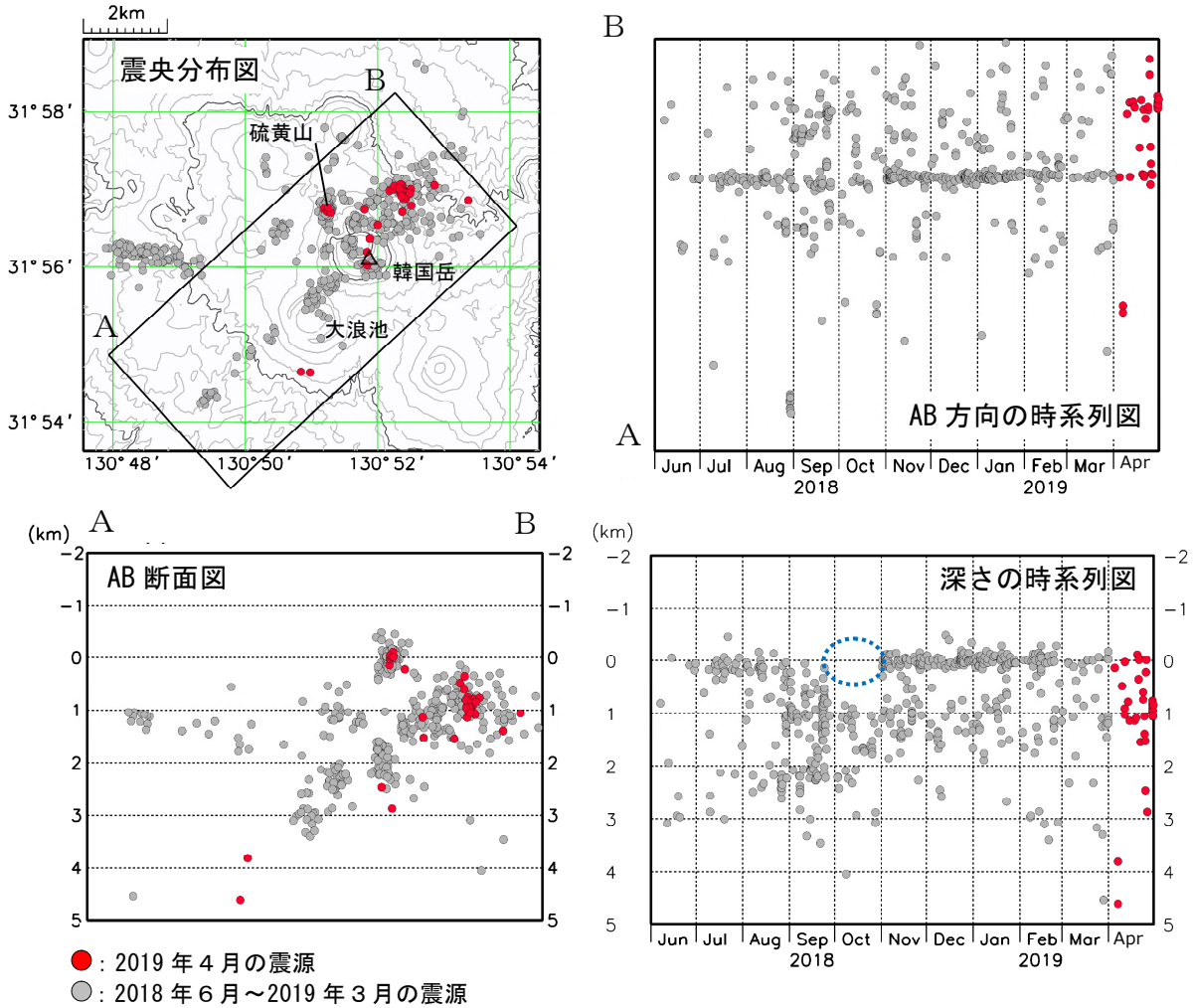
図 8-2 霧島山（えびの高原（硫黄山）周辺） 震源分布図（2018 年 6 月～2019 年 4 月）
