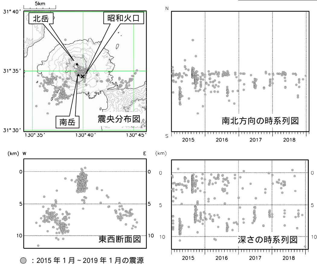
図7 桜島 震源分布図（2015年1月～2019年1月）
