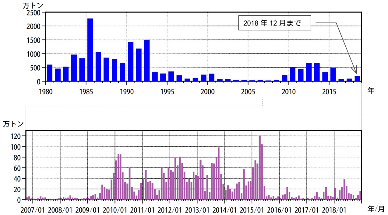
図11 桜島 鹿児島県が実施している降灰の観測データから推定した火山灰の総噴出量 (上段：1980年1月～2018年12月の年別値、下段：2006年10月～2018年12月の月別値)
