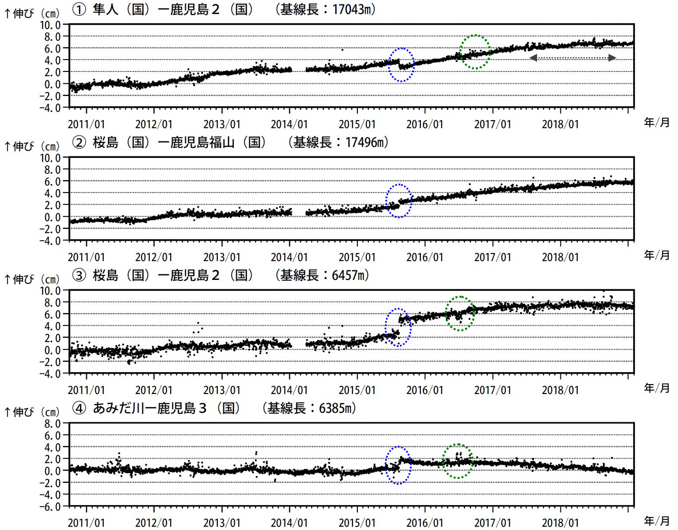
図 9-1 桜島 GNSS 連続観測による基線長変化 (2010 年 10 月 ~ 2019 年 1 月)
