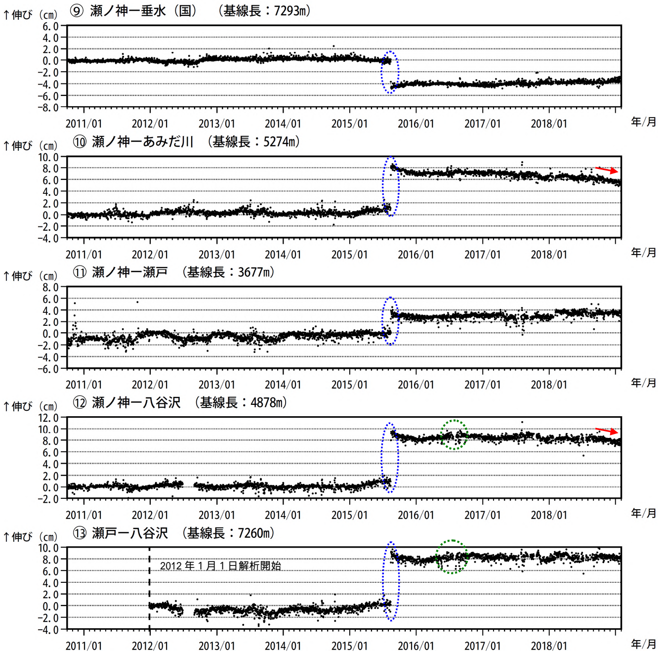
図 9-3 桜島 GNSS 連続観測による基線長変化 (2010 年 10 月 ~ 2019 年 1 月)
