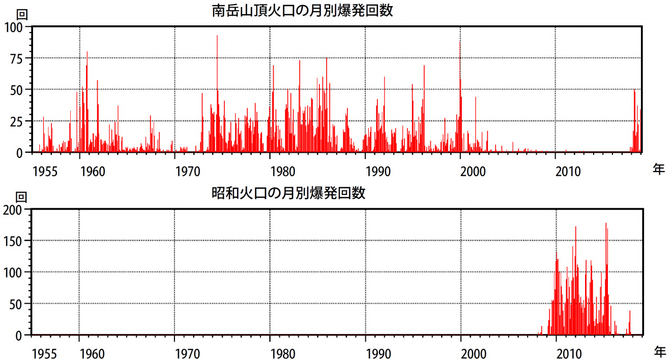
図 5-1 桜島 南岳山頂火口（上図）と昭和火口（下図）の月別爆発回数 （1955 年 1 月～2019 年 1 月）
