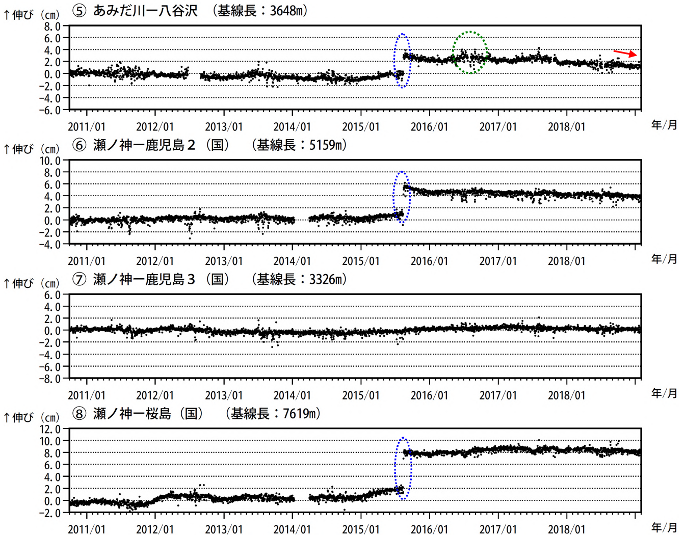
図 9-2 桜島 GNSS 連続観測による基線長変化 (2010 年 10 月 ~ 2019 年 1 月)
