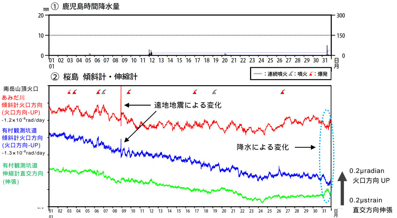
図8 桜島 傾斜計及び伸縮計による地殻変動の状況（2019年1月1日～1月31日）
