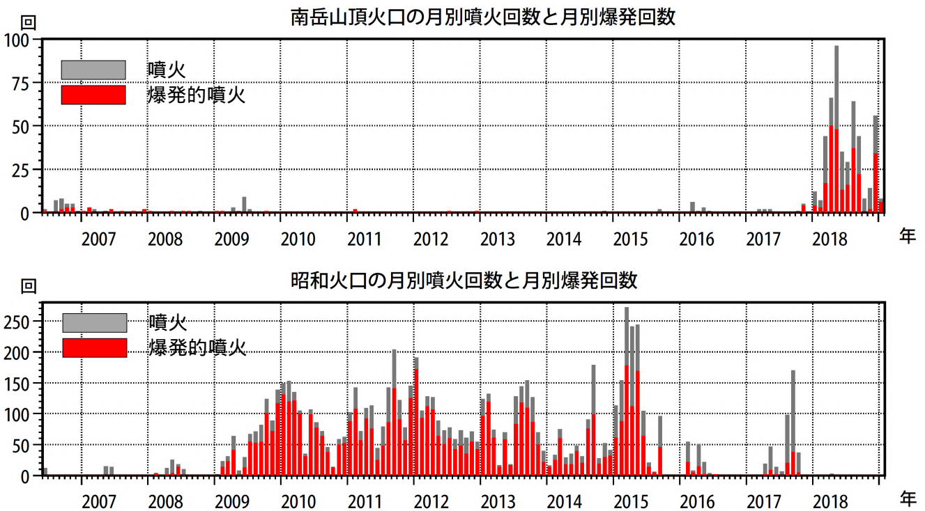
図 5-2 桜島 南岳山頂火口（上図）と昭和火口（下図）の月別噴火回数と月別爆発回数 （2006 年 6 月～2019 年 1 月）
