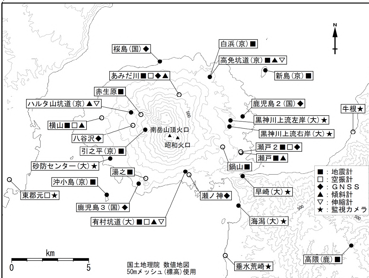
図12 桜島 観測点配置図
