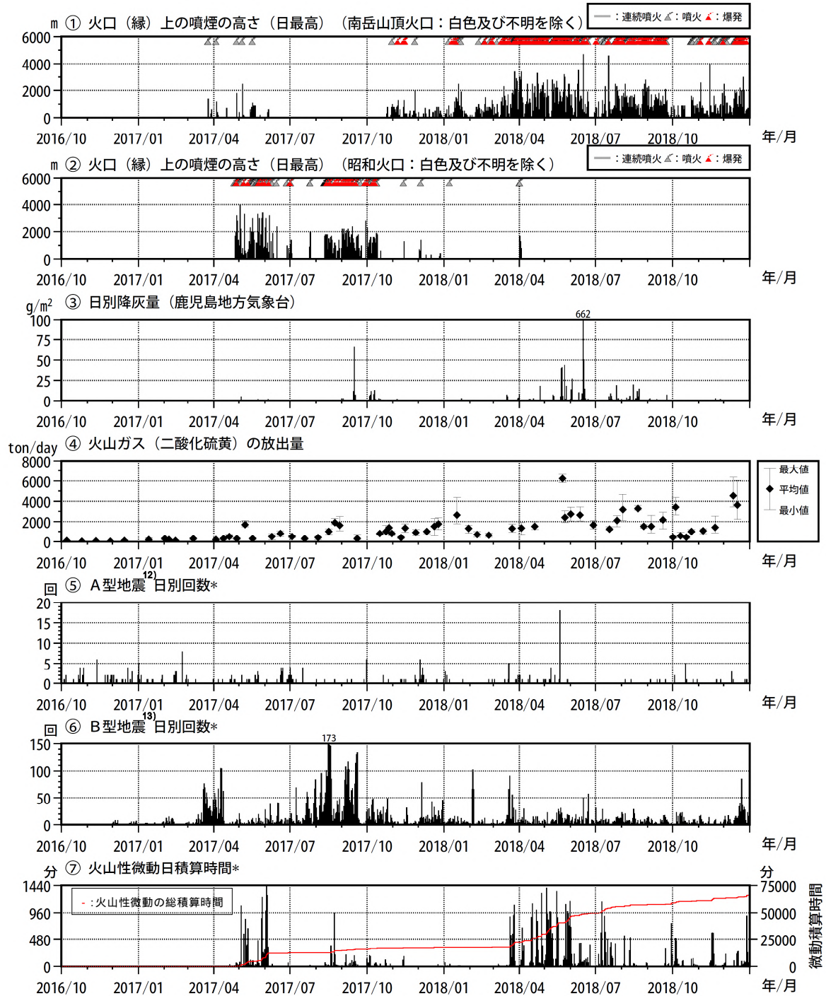
図3 桜島 最近2年間の活動経過図（2016年10月～2018年12月）
