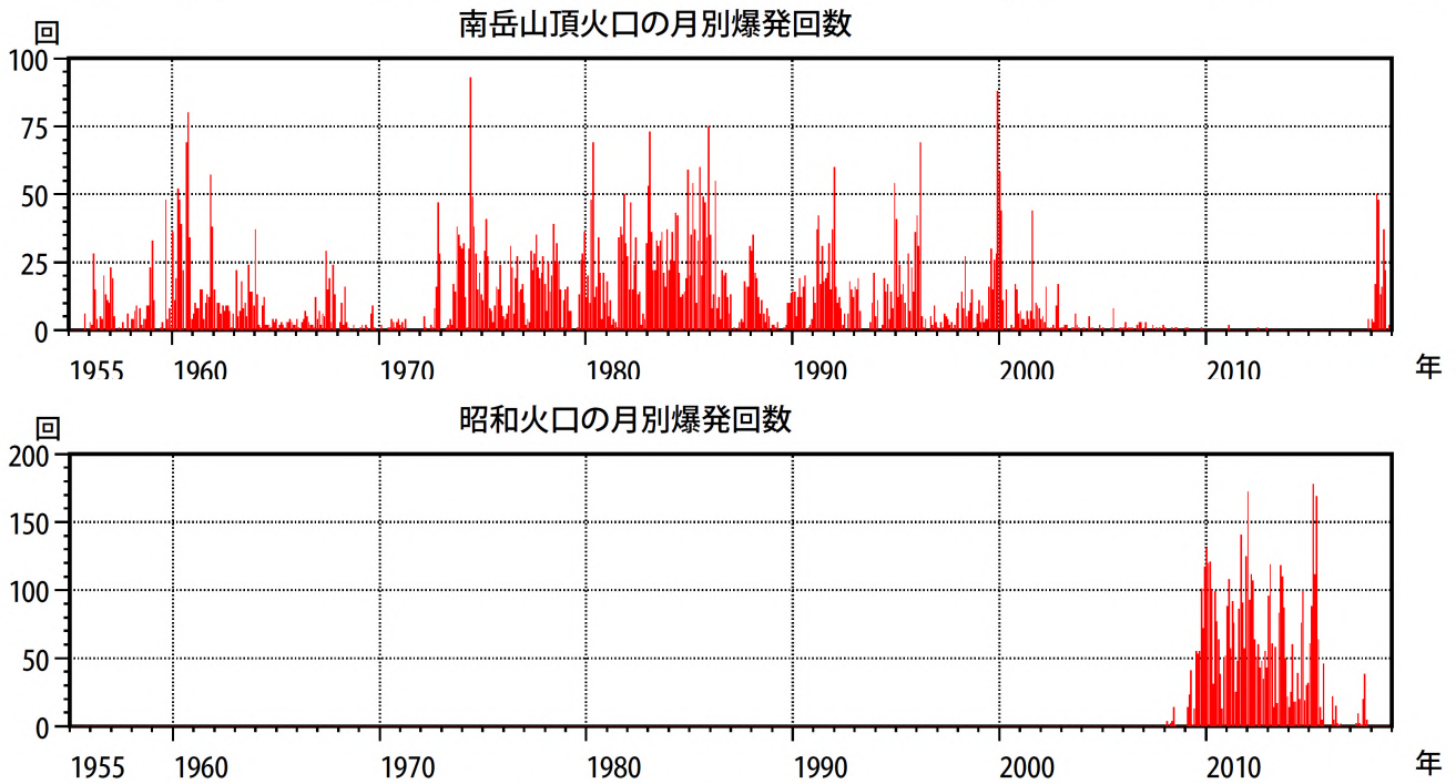
図 2-1 桜島 南岳山頂火口（上図）と昭和火口（下図）の月別爆発回数 （1955 年 1 月～2018 年 12 月）
