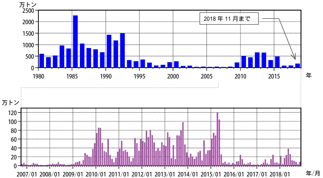
図 8 桜島 鹿児島県が実施している降灰の観測データから推定した火山灰の総噴出量 （上段：1980 年 1 月～2018 年 11 月の年別値、下段：2006 年 10 月～2018 年 11 月の月別値）
