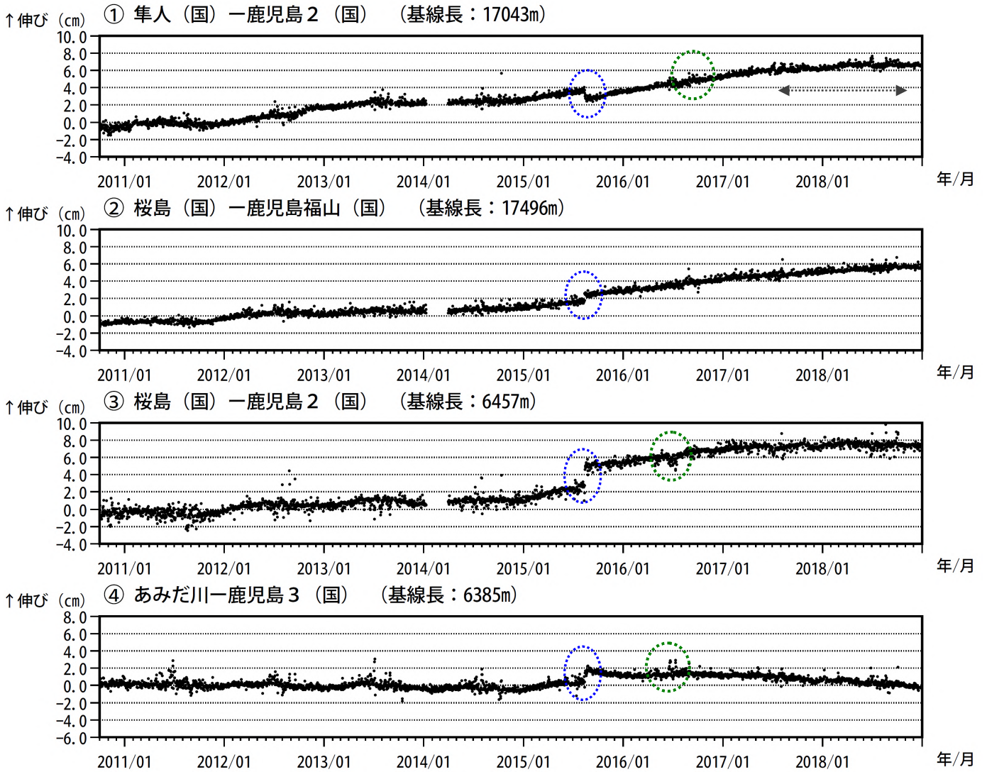
図 6-1 桜島 GNSS 連続観測による基線長変化（2010 年 10 月～2018 年 12 月）
