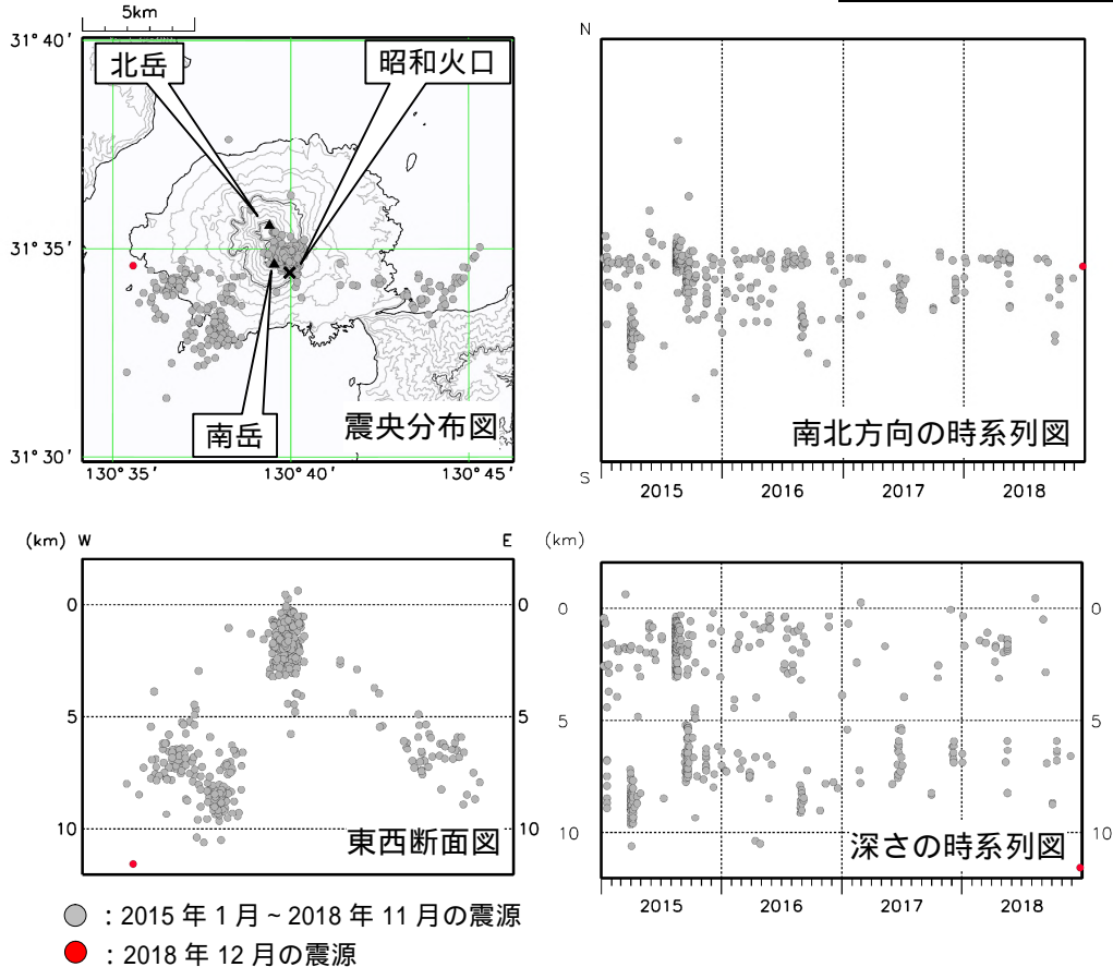
図4 桜島 震源分布図(2015年1月~2018年12月)
