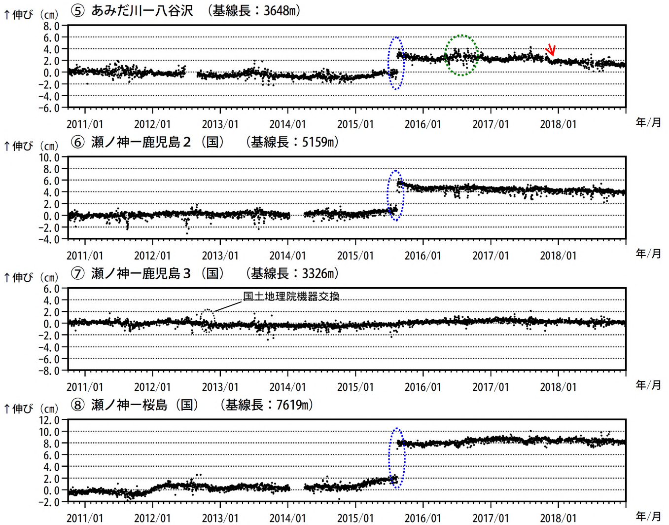
図 6-2 桜島 GNSS 連続観測による基線長変化 (2010 年 10 月 ~ 2018 年 12 月)
