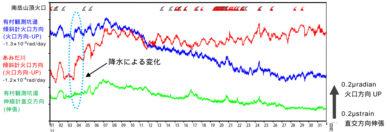
図5 桜島 傾斜計及び伸縮計による地殻変動の状況(2018年12月1日~12月31日)
