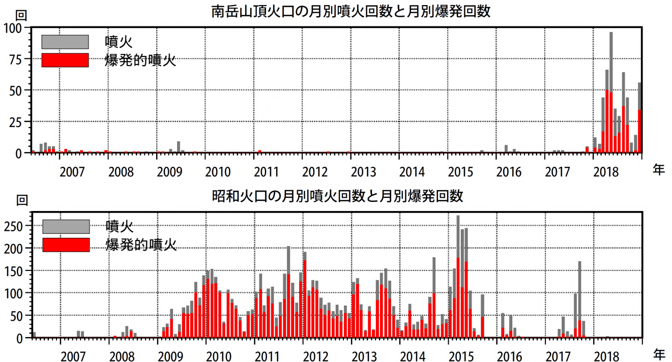
図 2-2 桜島 南岳山頂火口（上図）と昭和火口（下図）の月別噴火回数と月別爆発回数 （2006 年 6 月～2018 年 12 月）
