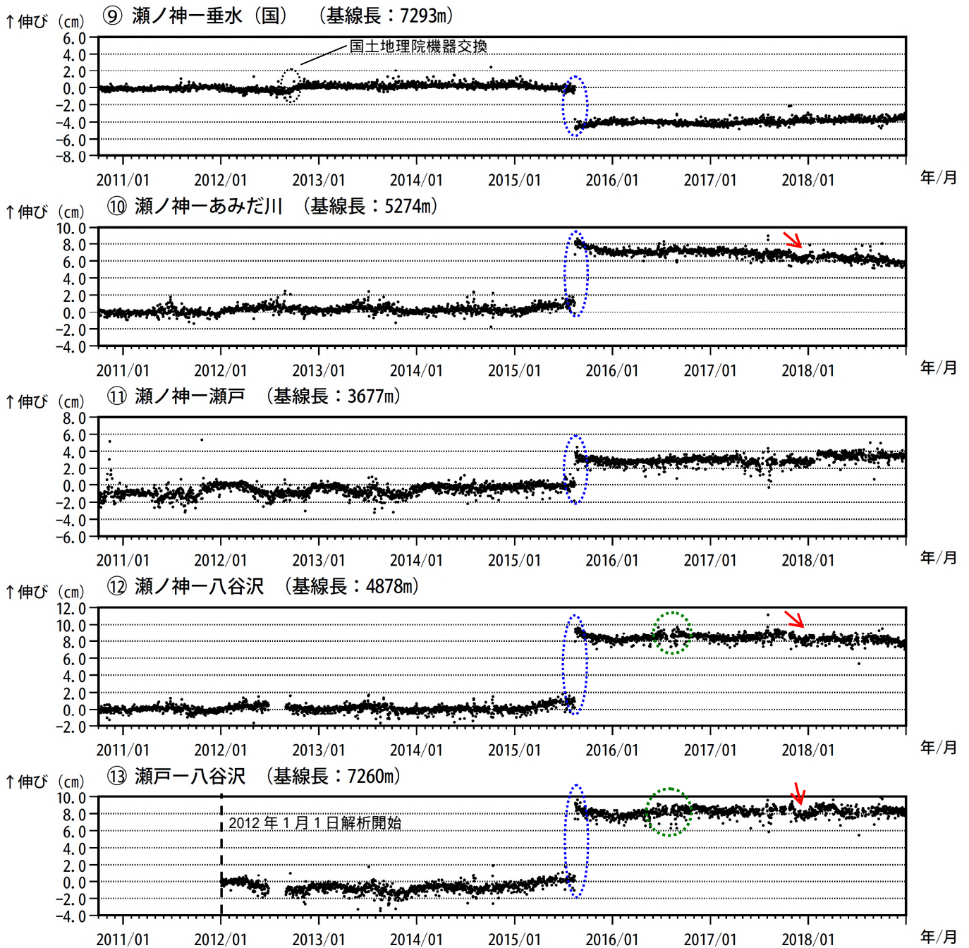
図 6-3 桜島 GNSS 連続観測による基線長変化（2010 年 10 月～2018 年 12 月）
