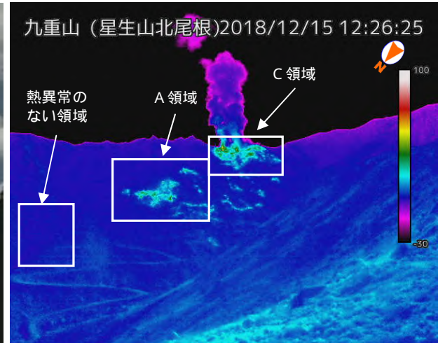
図2-1 九重山 熱異常域の状況 (12月15日、星生山北尾根赤外熱映像装置による)
