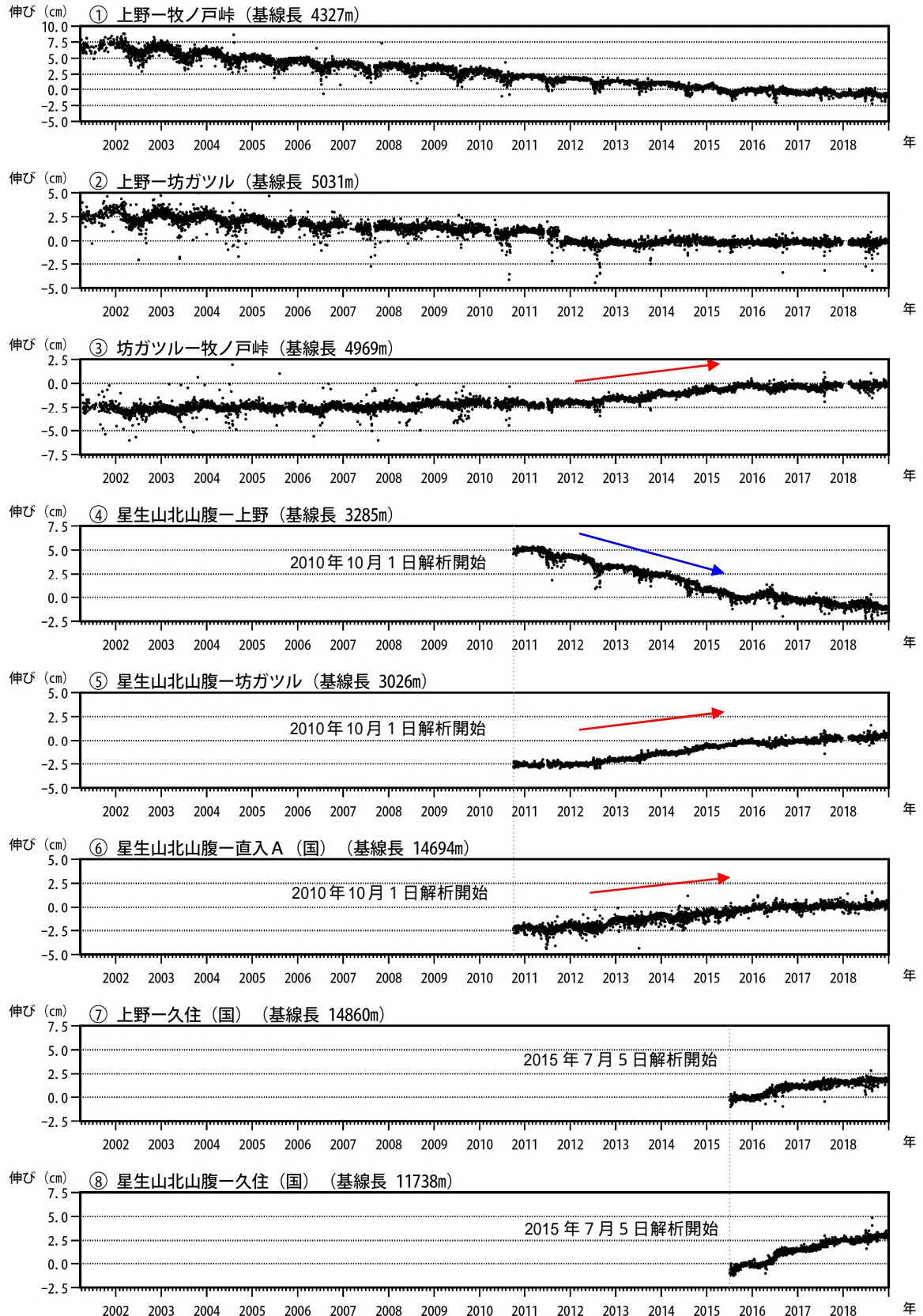
図 8 九重山 GNSS 連続観測による基線長変化（2001 年 3 月～2018 年 12 月）
