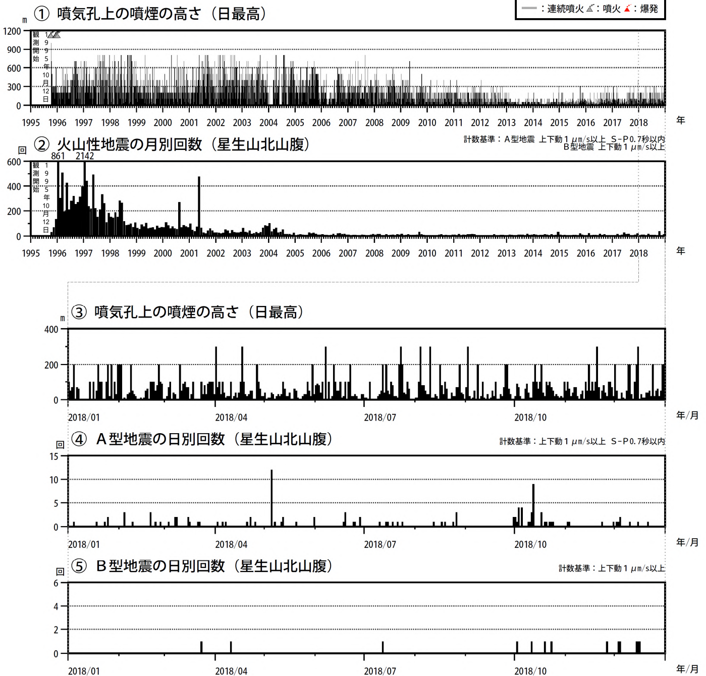
図3 九重山 火山活動経過図（1995年10月～2018年12月）
