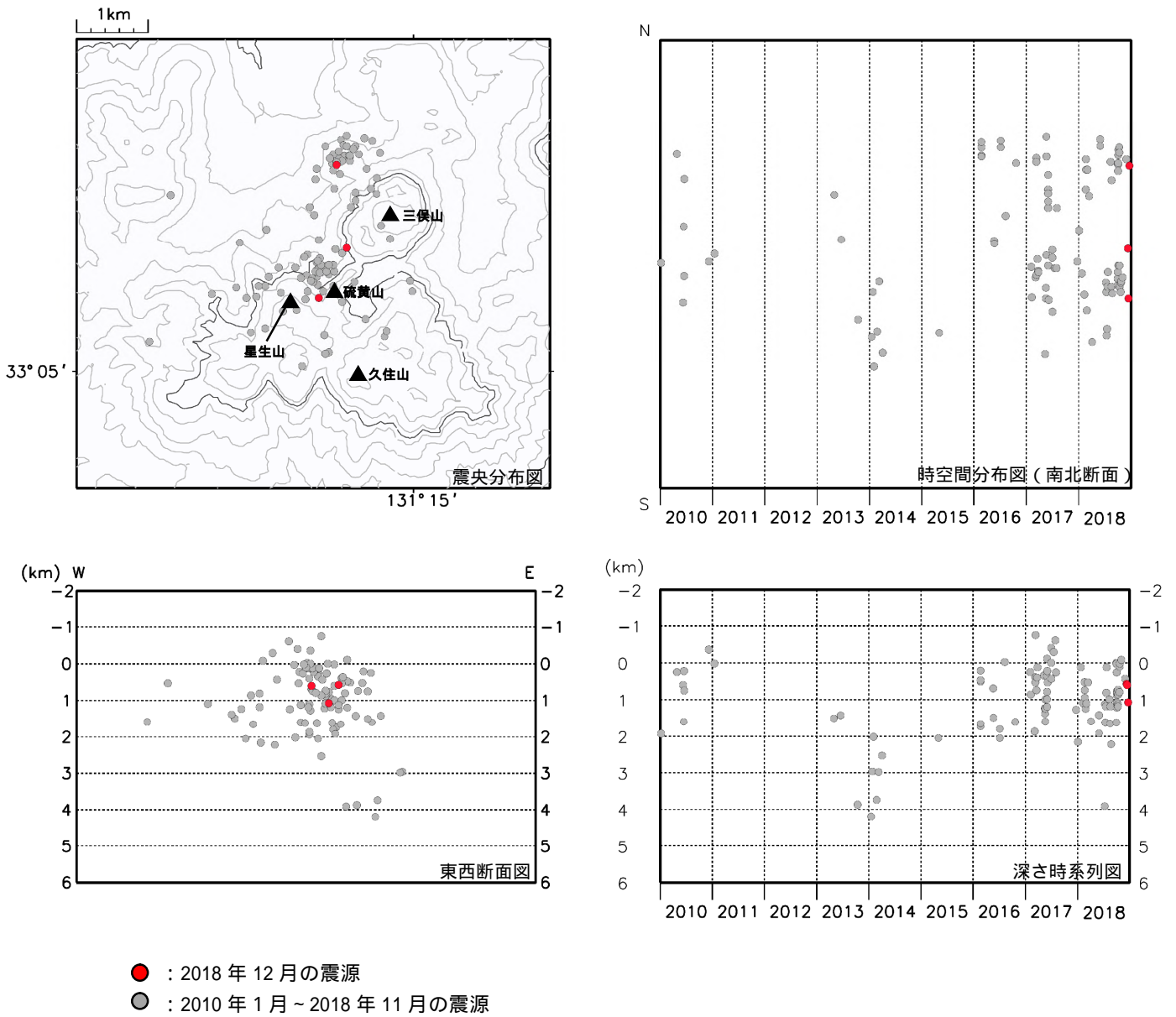
図 4-1 九重山 震源分布図（硫黄山付近の火山性地震）（2010 年 1 月 ~ 2018 年 12 月）
