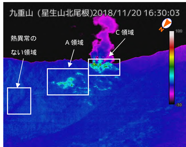
図 2-1 九重山 熱異常域の状況 (11月20日、星生山北尾根赤外熱映像装置による)
