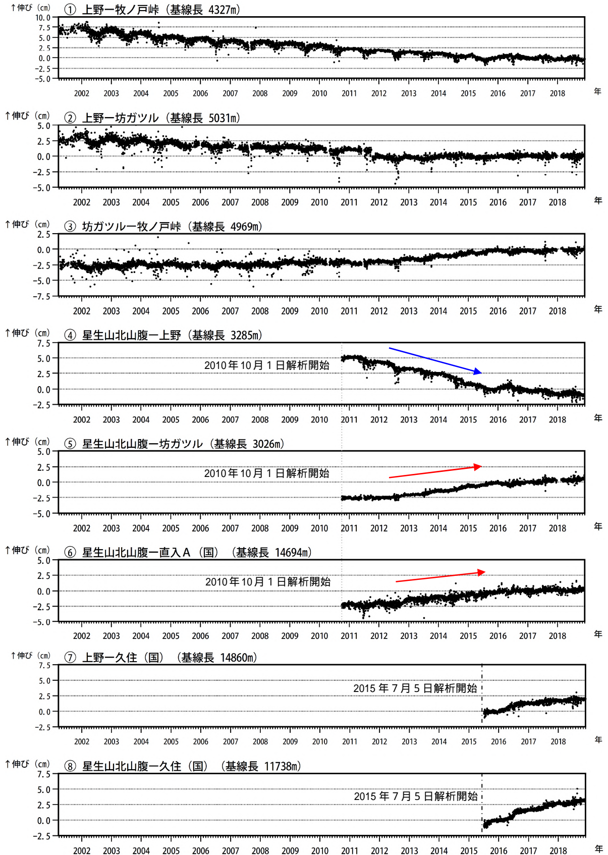
図 8 九重山 GNSS 連続観測による基線長変化（2001 年 3 月～2018 年 11 月）
