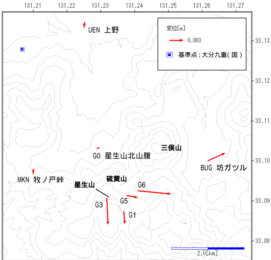
図10 九重山 GNSS 繰り返し観測による水平変位ベクトル(2017年11月~2018年9月)
