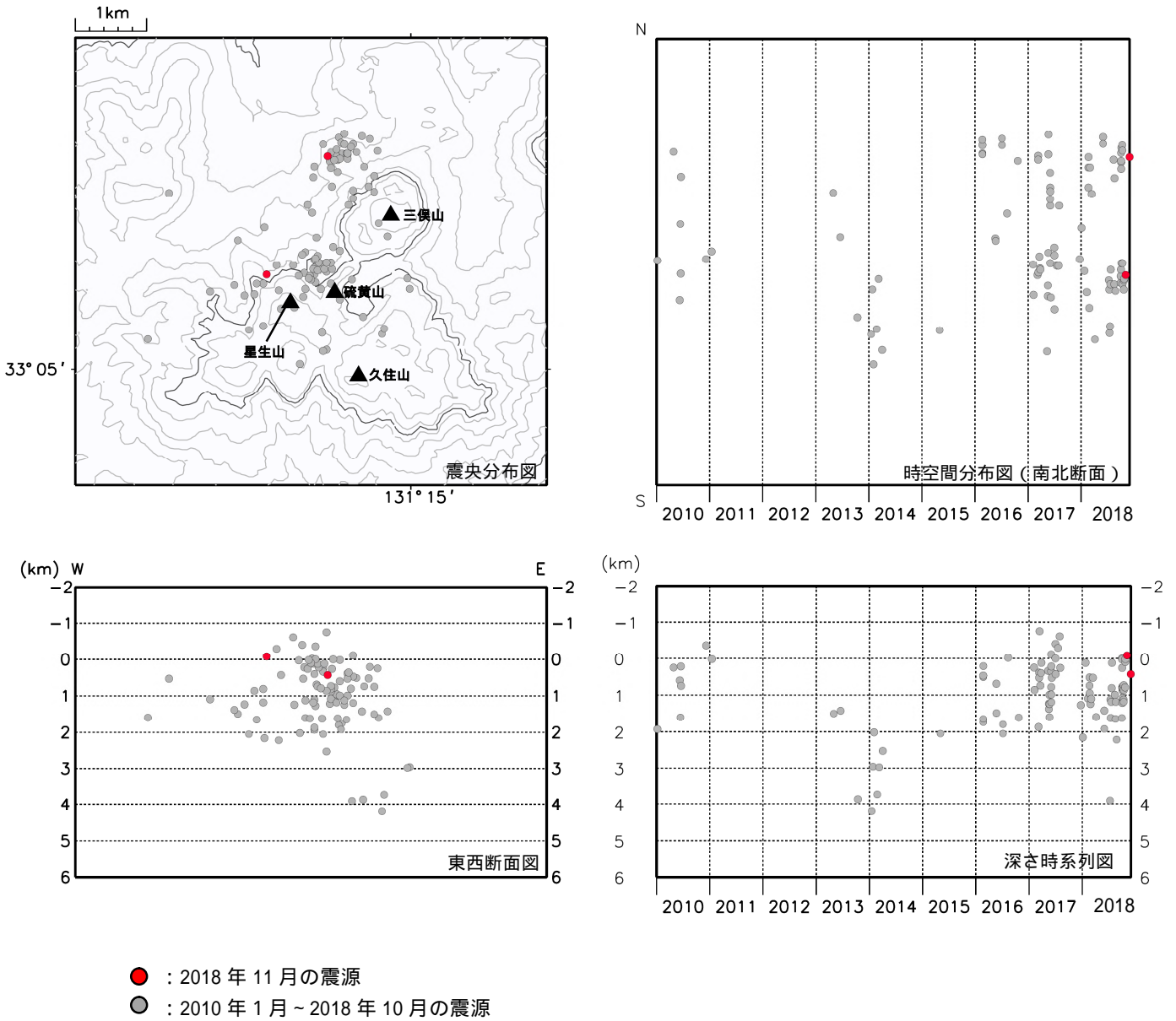
図 4-1 九重山 震源分布図（硫黄山付近の火山性地震）（2010 年 1 月 ~ 2018 年 11 月）
