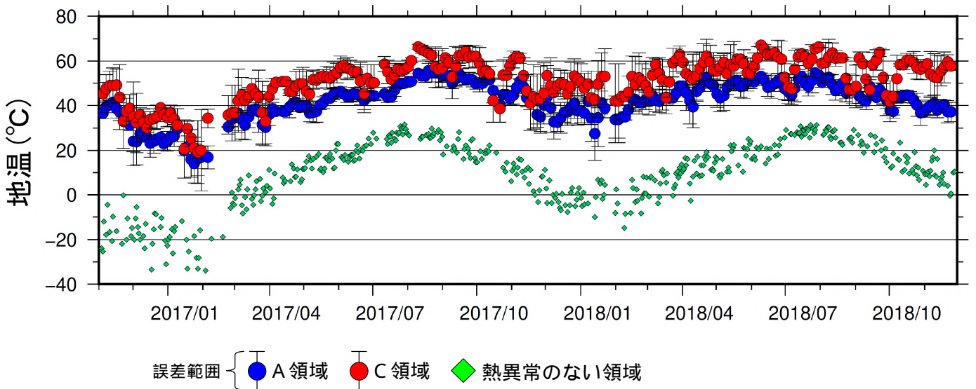
図 2-2 九重山 星生山北尾根赤外熱映像装置による日別最高温度の7日間移動平均値と分散 (2016年11月～2018年11月)
