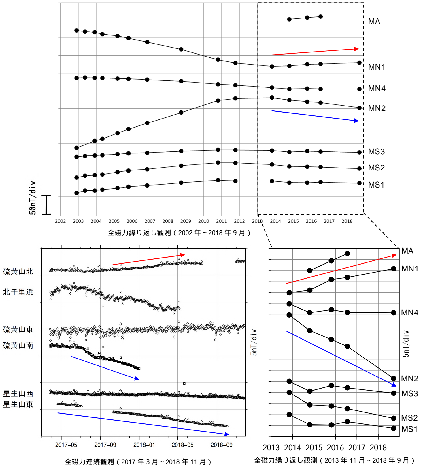
図5 九重山 全磁力観測による値の変化
