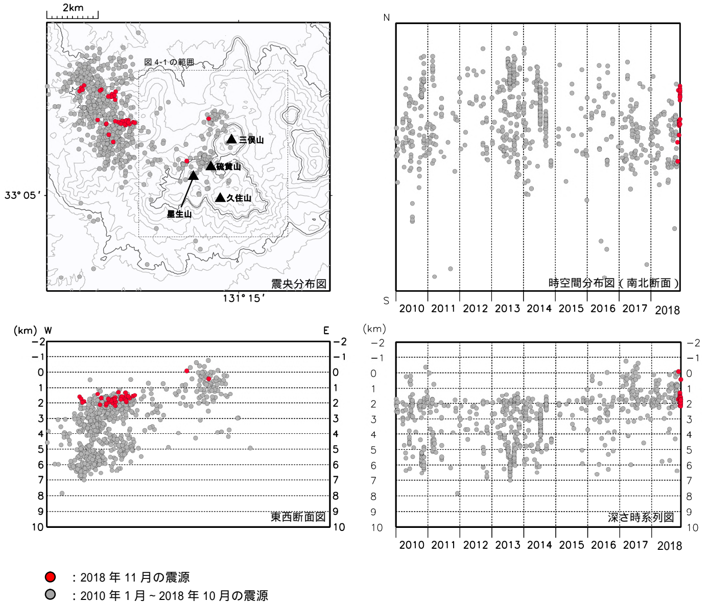
図 4-2 九重山 震源分布図（広域）（2010 年 1 月～2018 年 11 月）
