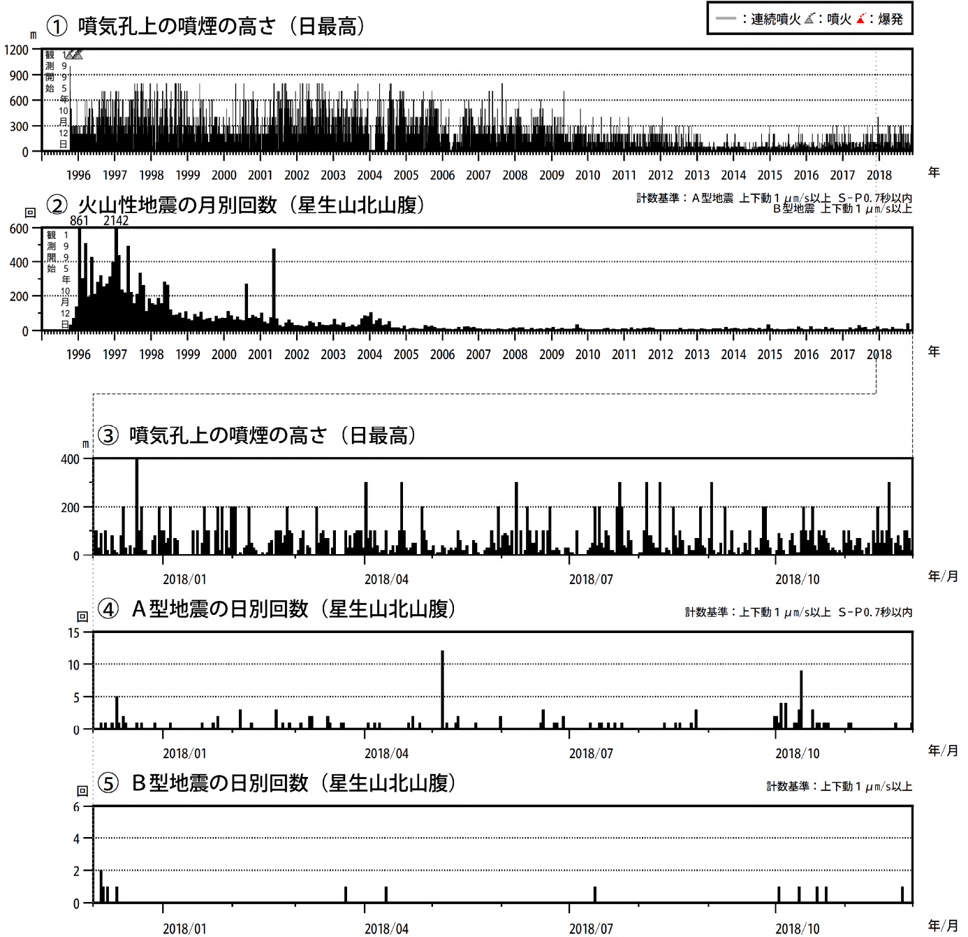
図3 九重山 火山活動経過図（1995年10月～2018年11月）
