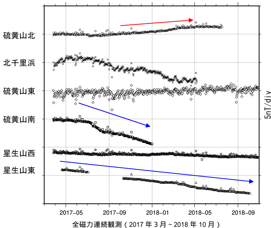
図5 九重山 全磁力観測による値の変化
