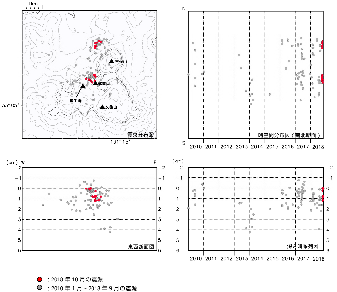
図4-1 九重山 震源分布図(硫黄山付近の火山性地震)(2010年1月~2018年10月)
