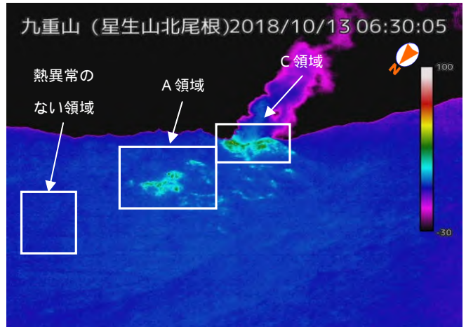
図2-1 九重山 熱異常域の状況 (10月13日、星生山北尾根赤外熱映像装置による)
