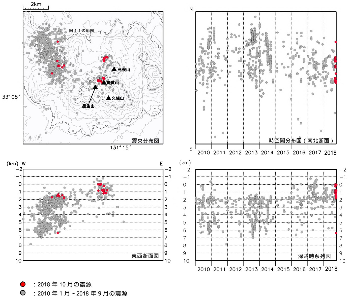
図 4-2 九重山 震源分布図（広域）（2010 年 1 月～2018 年 10 月）
