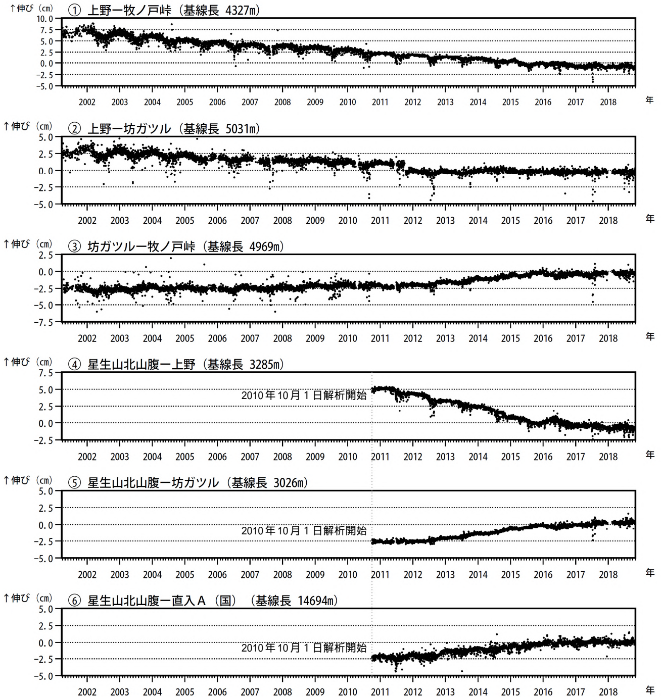
図 8-1 九重山 GNSS 連続観測による基線長変化（2001 年 3 月～2018 年 10 月）
