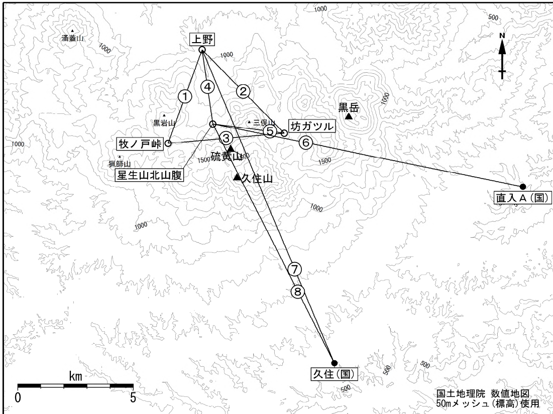
図 9 九重山 GNSS 連続観測点と基線番号
