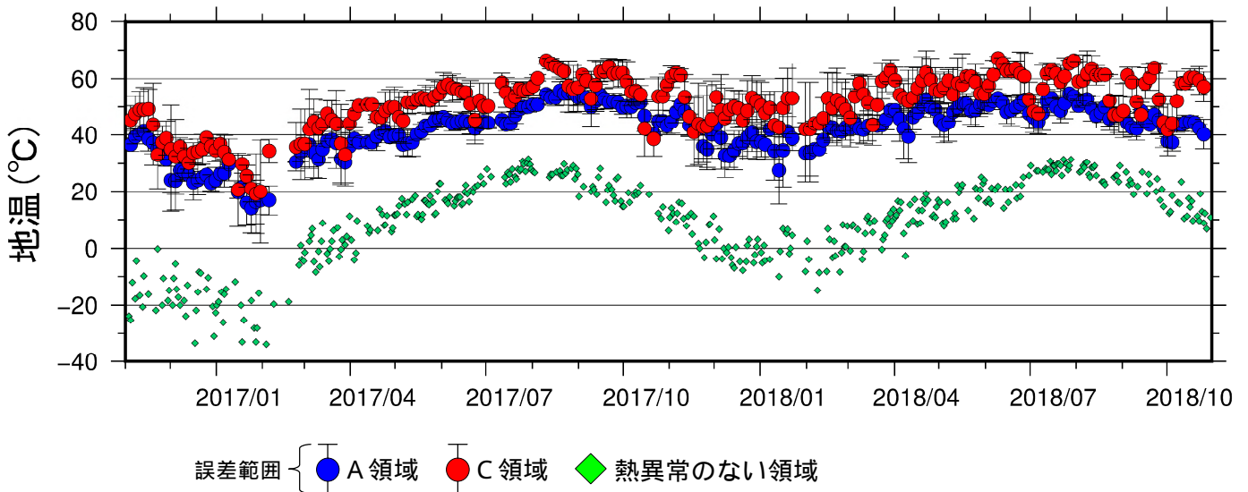
図2-2 九重山 星生山北尾根赤外熱映像装置による日別最高温度の7日間移動平均値と分散 (2016年11月～2018年10月)
