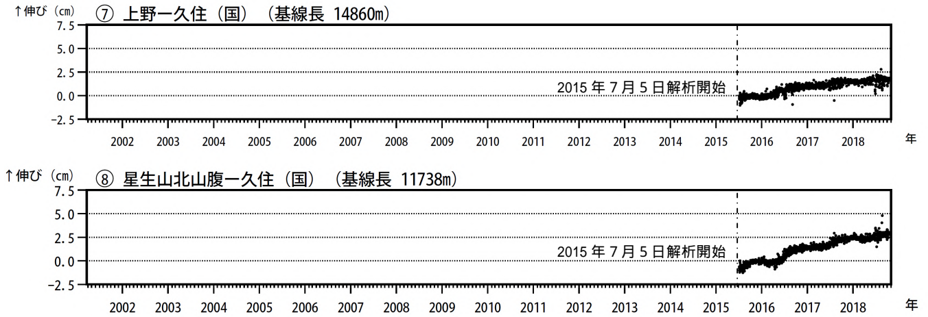
図 8-2 九重山 GNSS 連続観測による基線長変化（2001 年 3 月～2018 年 10 月）
