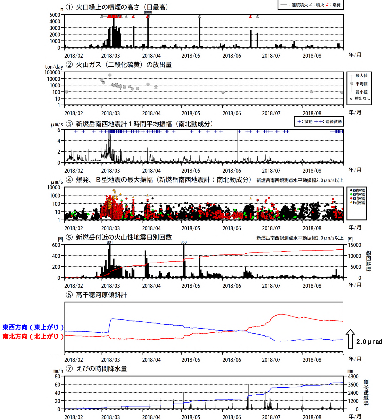
図 5 霧島山（新燃岳） 火山活動経過図（2018 年 2 月～2018 年 8 月）
