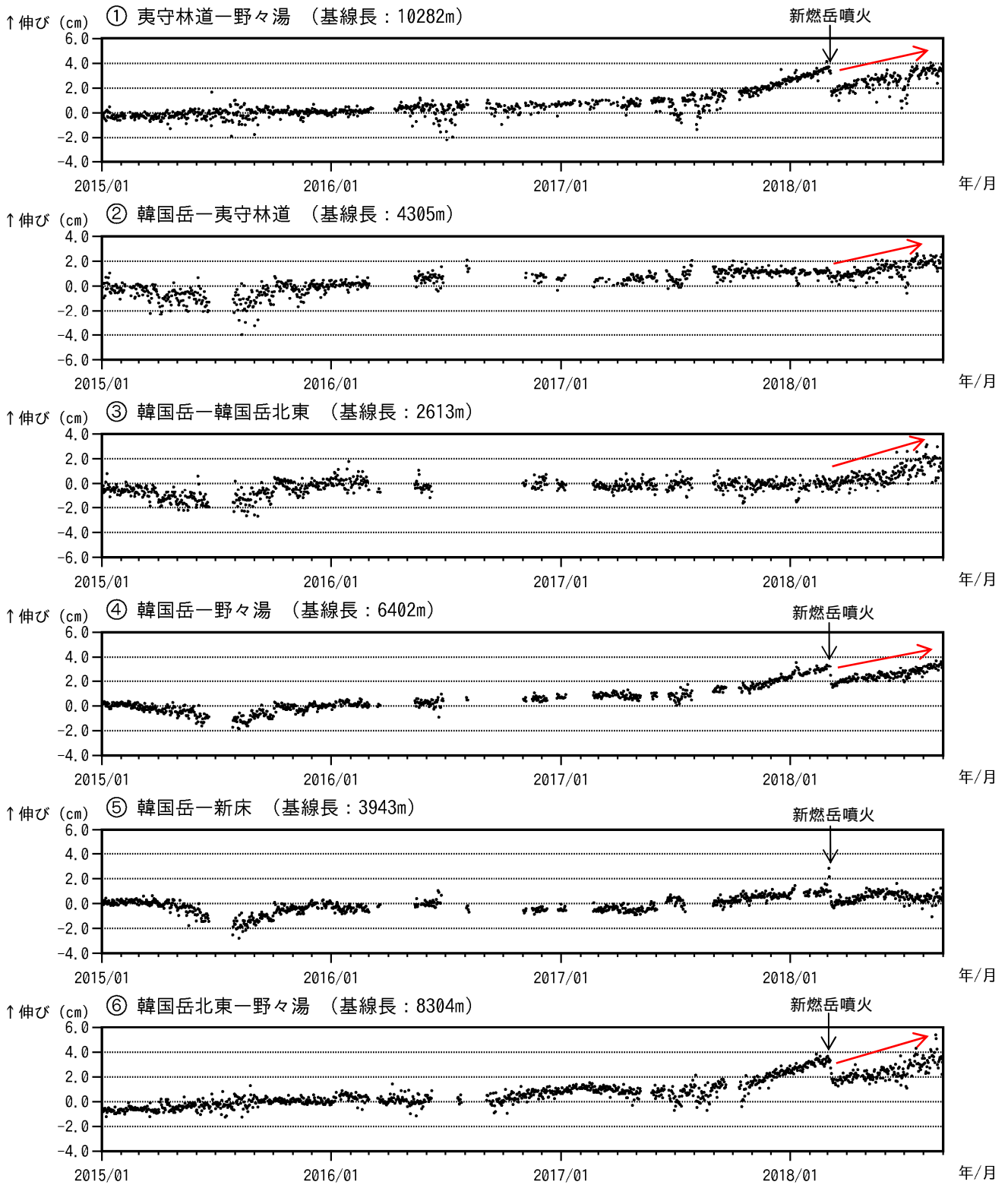
図 13-1 霧島山(えびの高原(硫黄山)周辺) GNSS 連続観測による基線長変化 (2015年1月~2018年8月)
