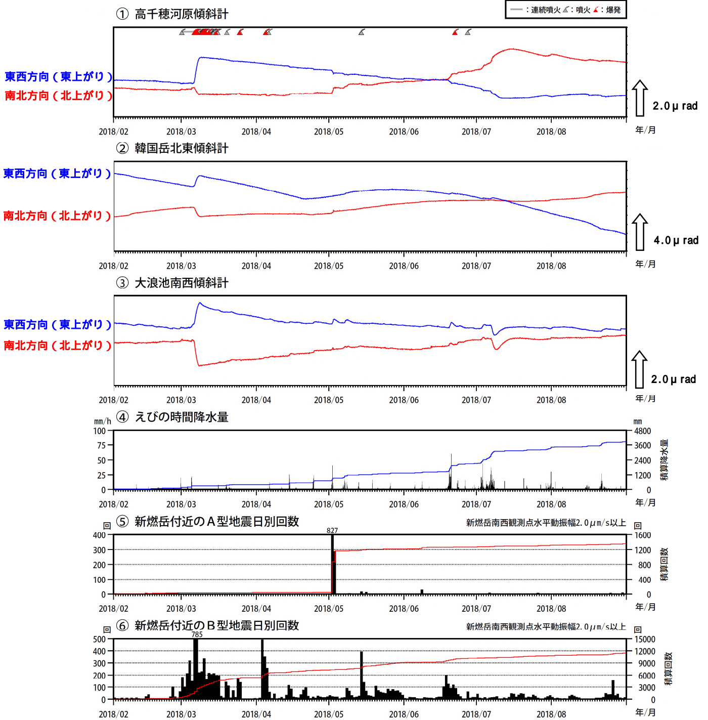
図 6 霧島山（新燃岳） 傾斜変動と火山性地震の日別回数（2018 年 2 月～ 8 月）
