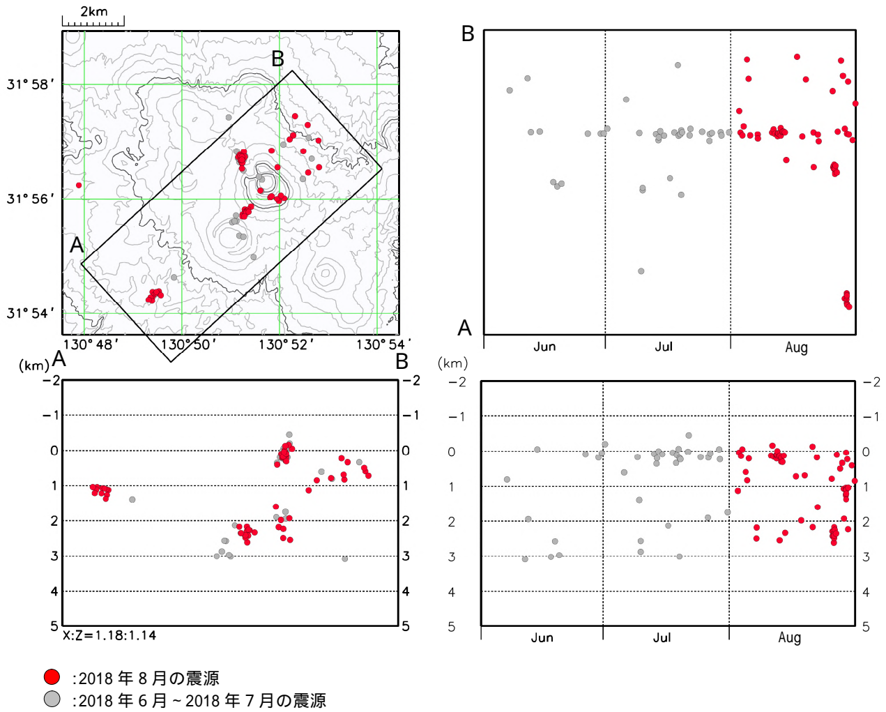
図7-2 霧島山(えびの高原(硫黄山)周辺) 震源分布図(2018年6月~2018年8月)
