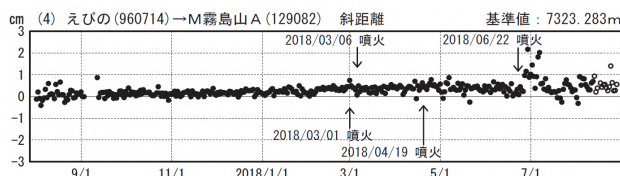
図11 霧島山 国土地理院による地殻変動観測結果(2017年8月1日~2018年8月27日)
