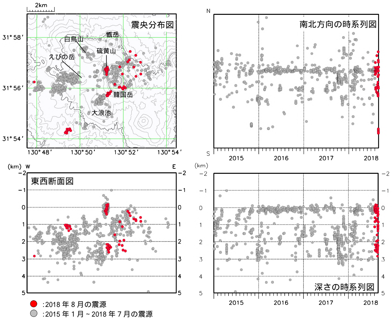
図 7-1 霧島山（えびの高原（硫黄山）周辺） 震源分布図（2015年1月～2018年8月）
