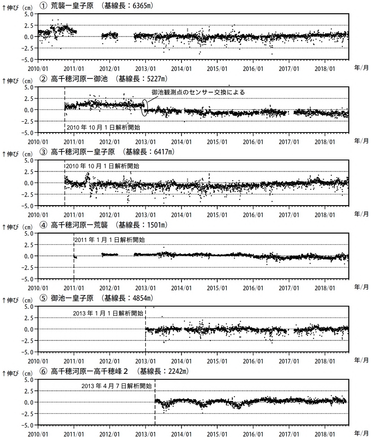
図3 霧島山(御鉢) GNSS連続観測による基線長変化(2010年1月~2018年8月)
