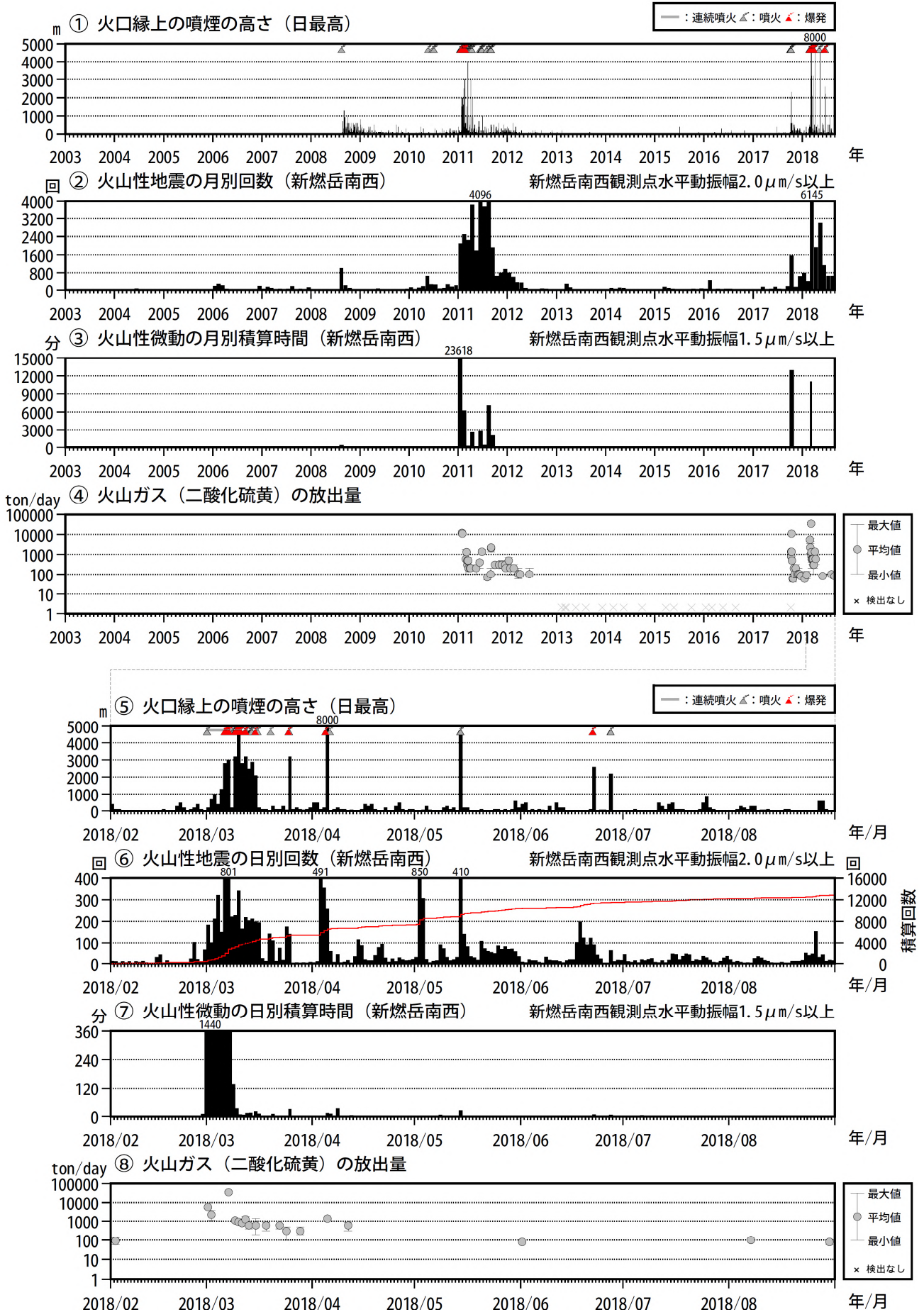
図 4 霧島山（新燃岳） 火山活動経過図（2003 年 1 月～2018 年 8 月）
