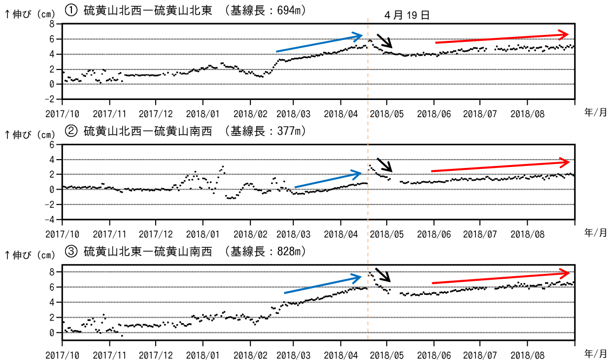
図 11 霧島山（えびの高原（硫黄山）周辺） GNSS 連続観測による基線長変化 （2017 年 10 月～2018 年 8 月）
