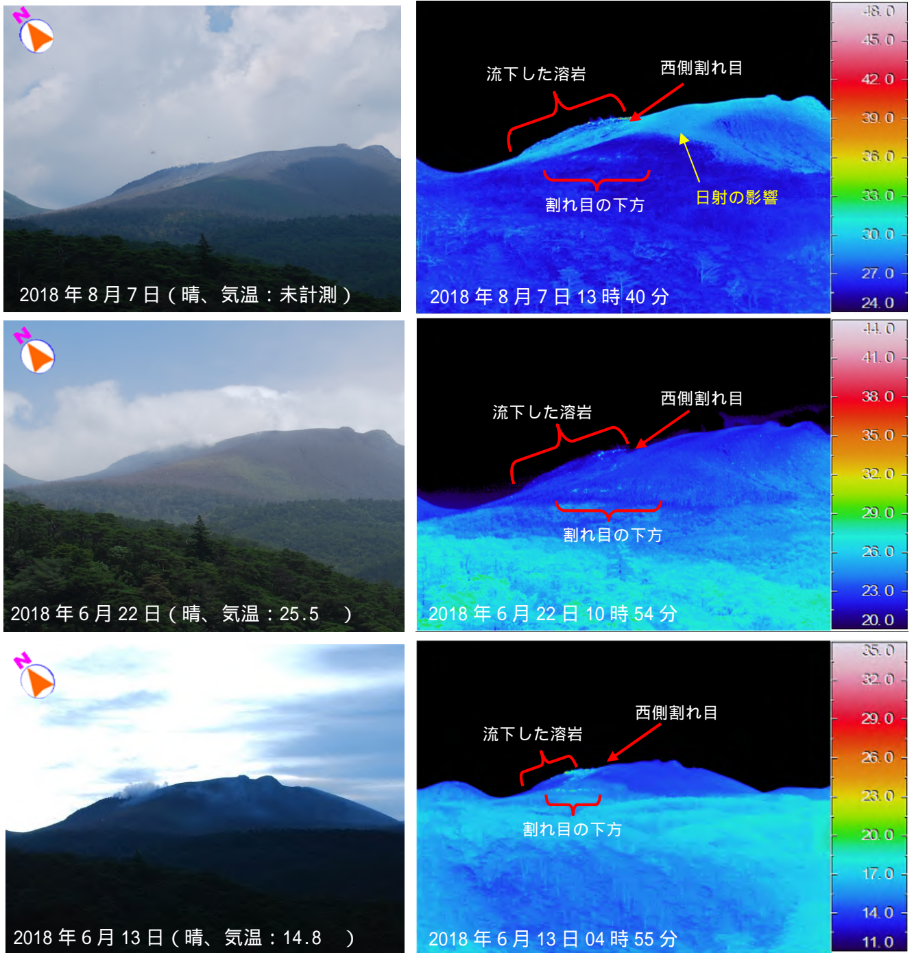
図3 霧島山（新燃岳）の状況（新湯温泉定点からの観測）
