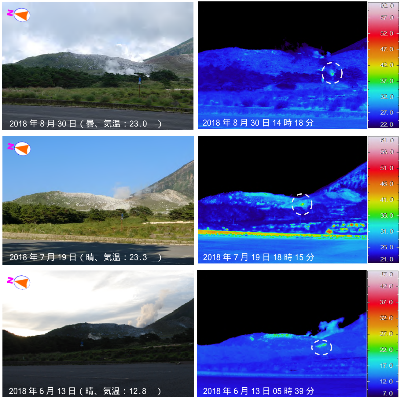
図5 霧島山(えびの高原(硫黄山)周辺) 硫黄山の状況(えびの高原から観測)
