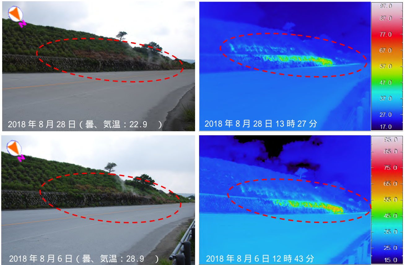
図3 霧島山(えびの高原(硫黄山)周辺) 硫黄山北西斜面の状況(えびの高原から観測)
