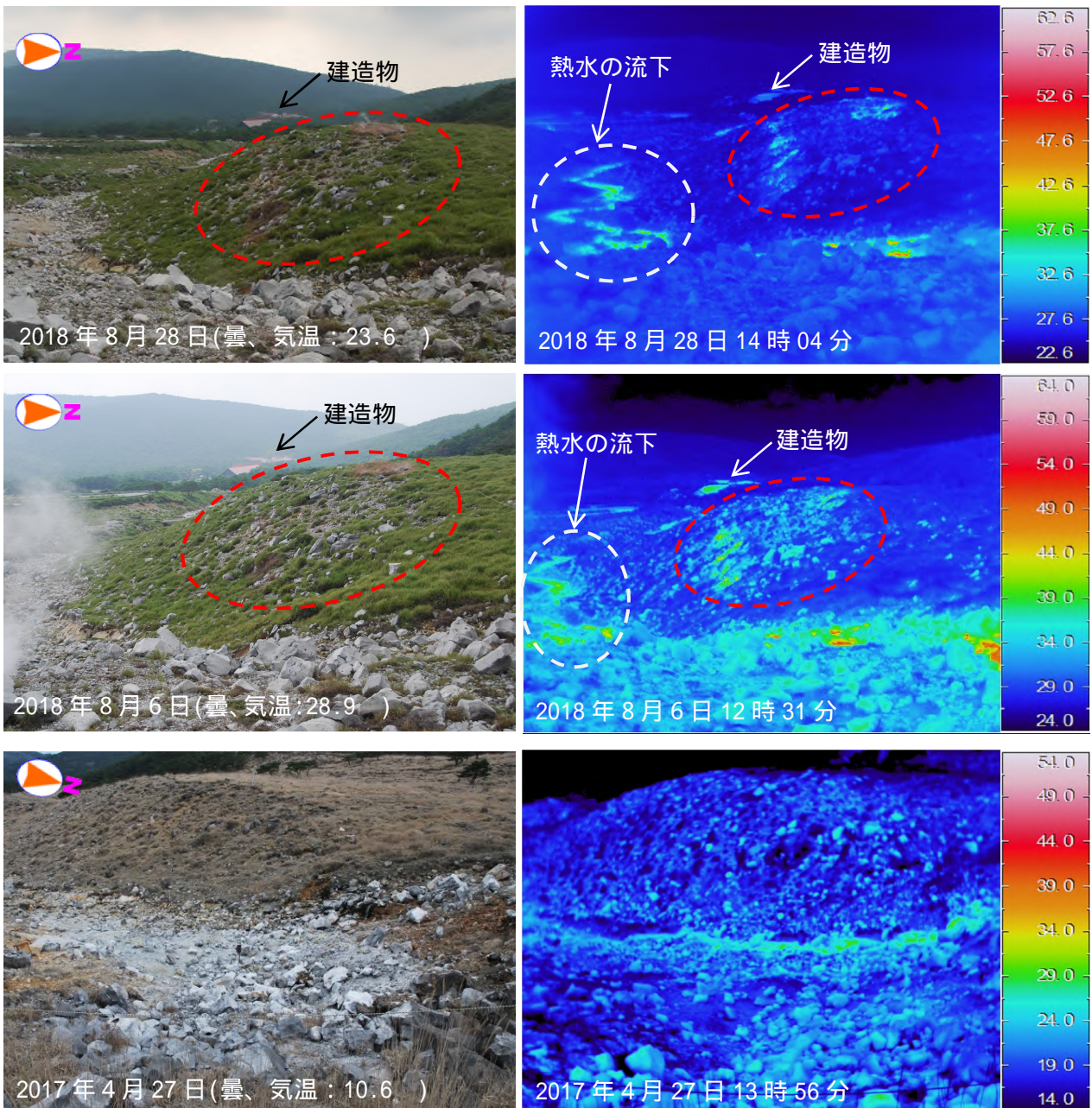
図4 霧島山(えびの高原(硫黄山)周辺) 硫黄山の西側の状況(えびの高原から観測)
