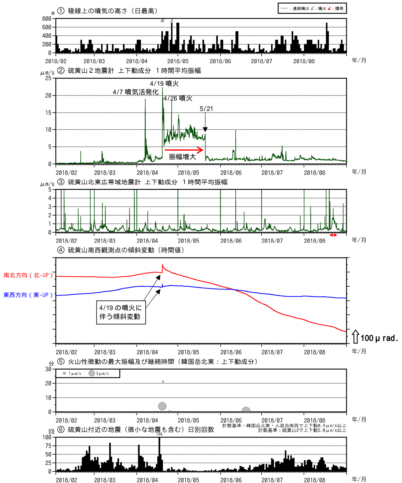
図8 霧島山(えびの高原(硫黄山)周辺) 火山活動経過図(2018年2月~8月)
