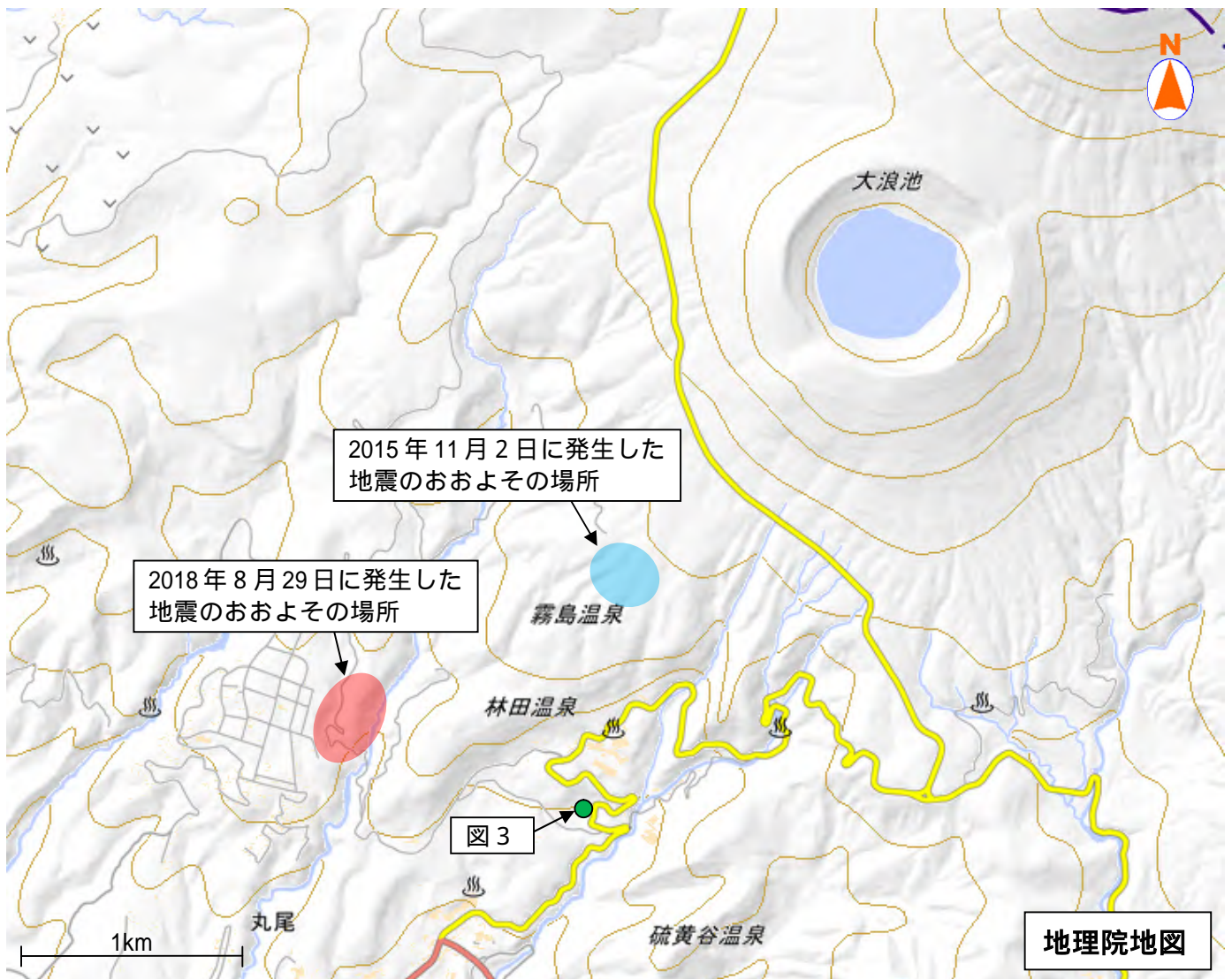
図4 霧島山 30日に実施した現地調査の地点(図中の緑丸)
