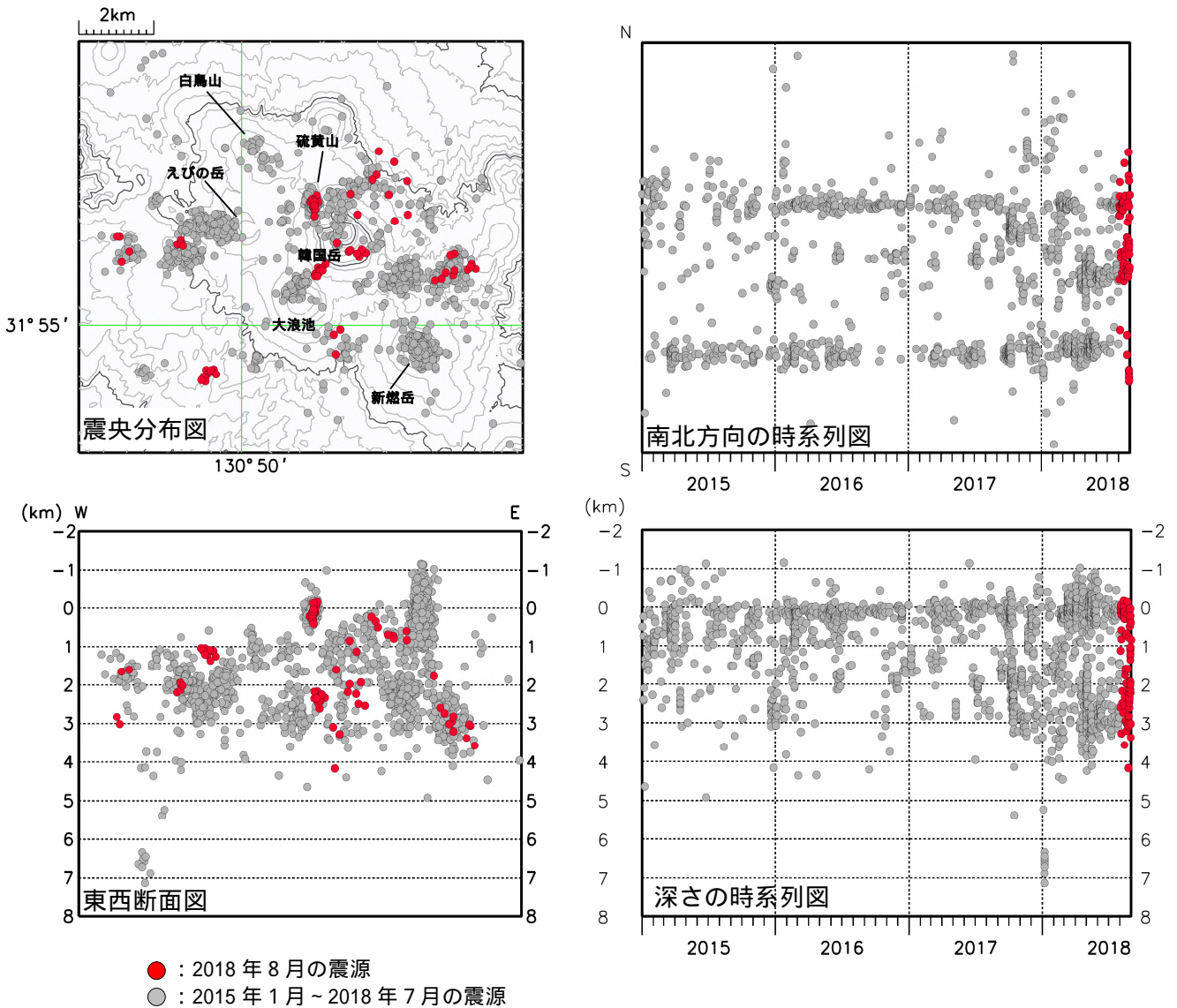
図8 霧島山 新燃岳から硫黄山周辺の火山性地震の震源分布図(2015年1月～2018年8月)
