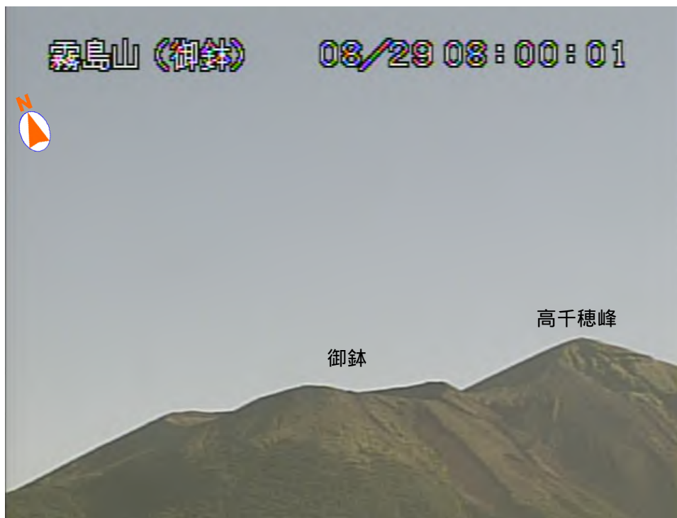
図 1 霧島山（御鉢） 御鉢の状況（8 月 29 日、猪子石監視カメラによる）
