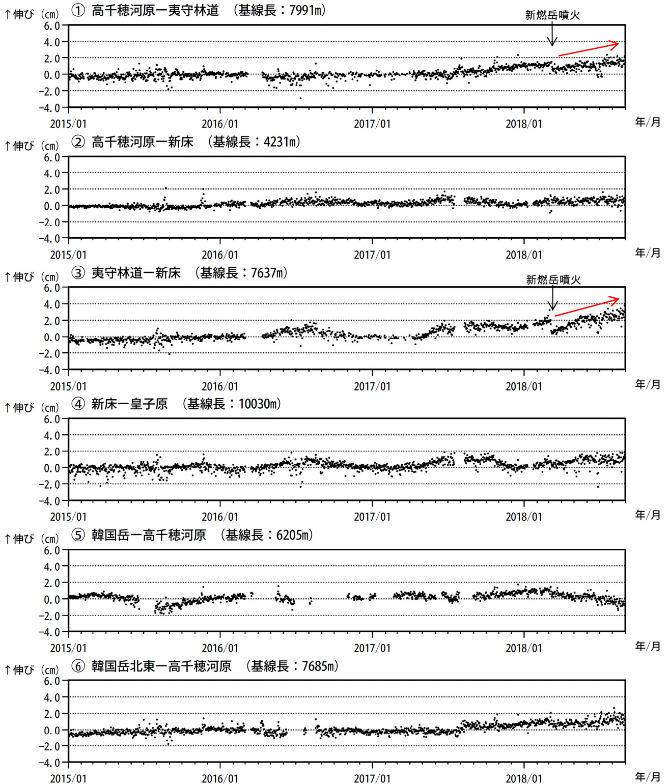
図9-1 霧島山(新燃岳) GNSS連続観測による基線長変化(2015年1月~2018年8月)
