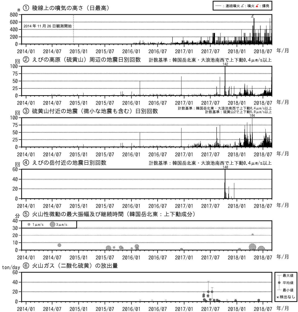
図 10 霧島山（えびの高原（硫黄山）周辺） 火山活動経過図（2013 年 12 月～2018 年 8 月）
