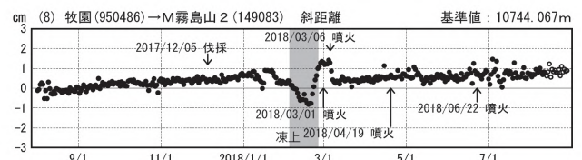
図11 霧島山 国土地理院による地殻変動観測結果(2017年8月1日~2018年8月27日)
