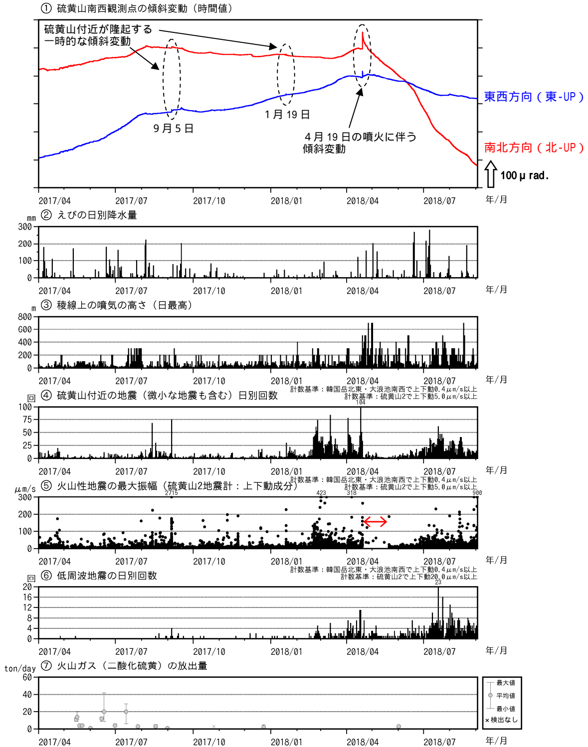
図9 霧島山（えびの高原（硫黄山）周辺） 硫黄山南西傾斜計の傾斜変動と硫黄山付近の火山活動経過図（2017年4月～2018年8月）
