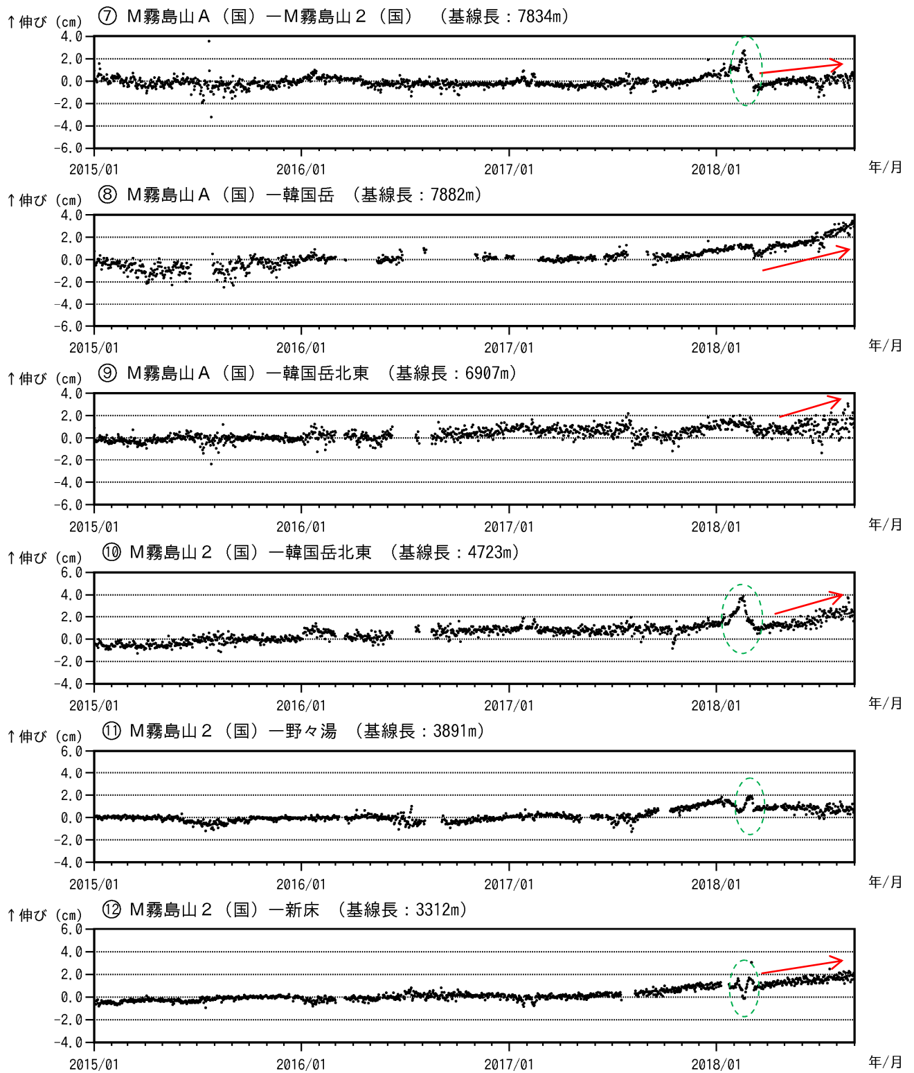
図 13-2 霧島山(えびの高原(硫黄山)周辺) GNSS連続観測による基線長変化 (2015年1月~2018年8月)
