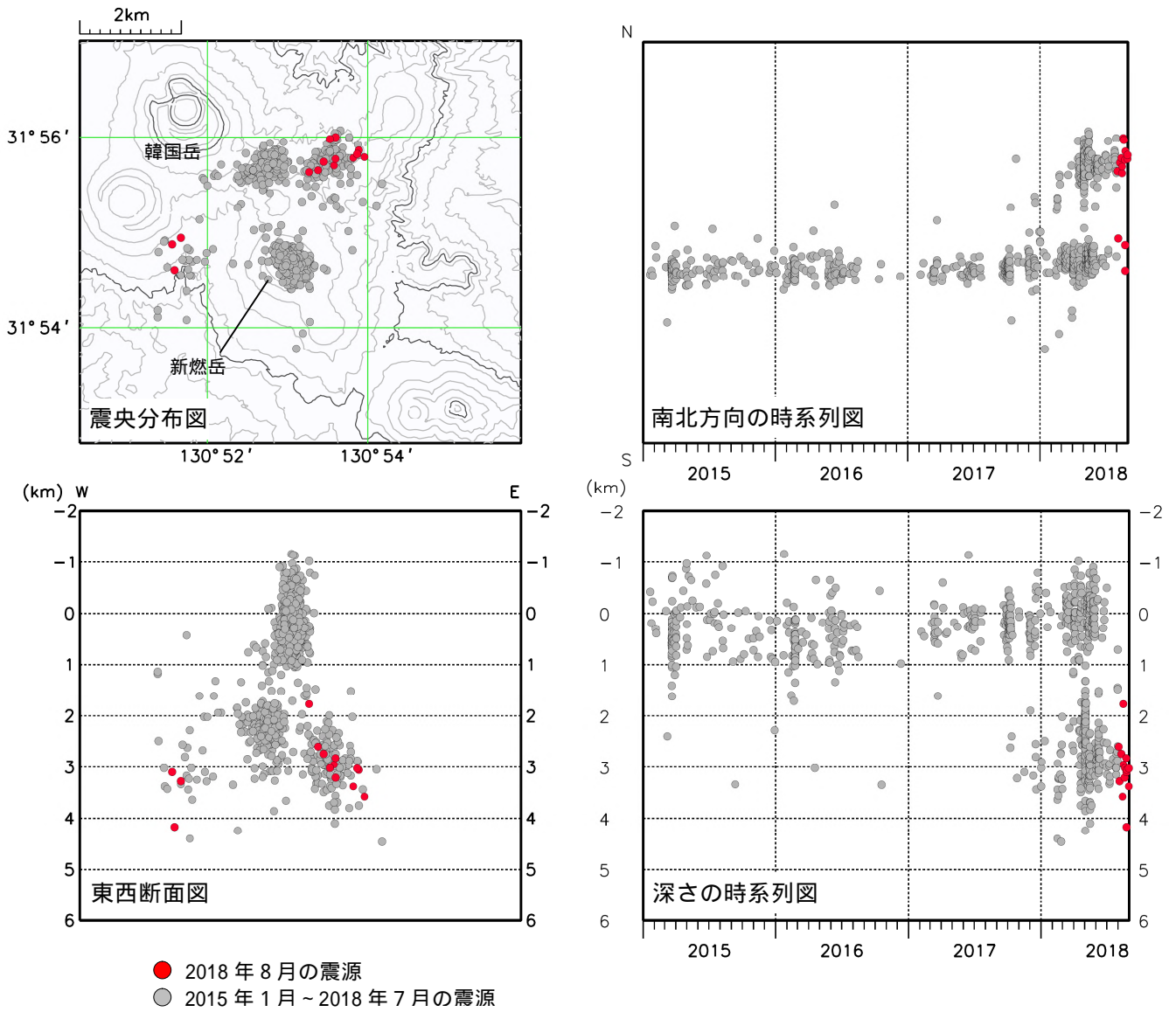
図7 霧島山（新燃岳） 震源分布図（2015年1月～2018年8月）
