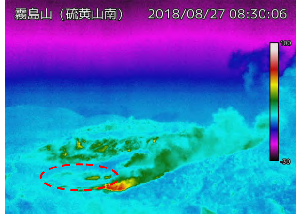
図 1-2 霧島山（えびの高原（硫黄山）周辺） 硫黄山南側の状況 （8月7日及び27日、硫黄山南監視カメラによる）
