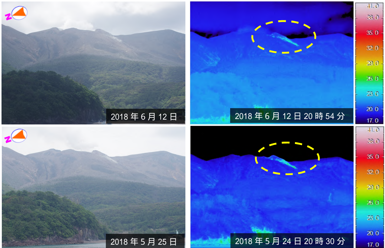
図2 口永良部島 本村から撮影した新岳火口及び新岳火口西側割れ目付近の可視画像と地表面温度分布前月(5月24日)と比較して、噴気及び熱異常域(黄破線)に特段の変化は認められませんでした。
