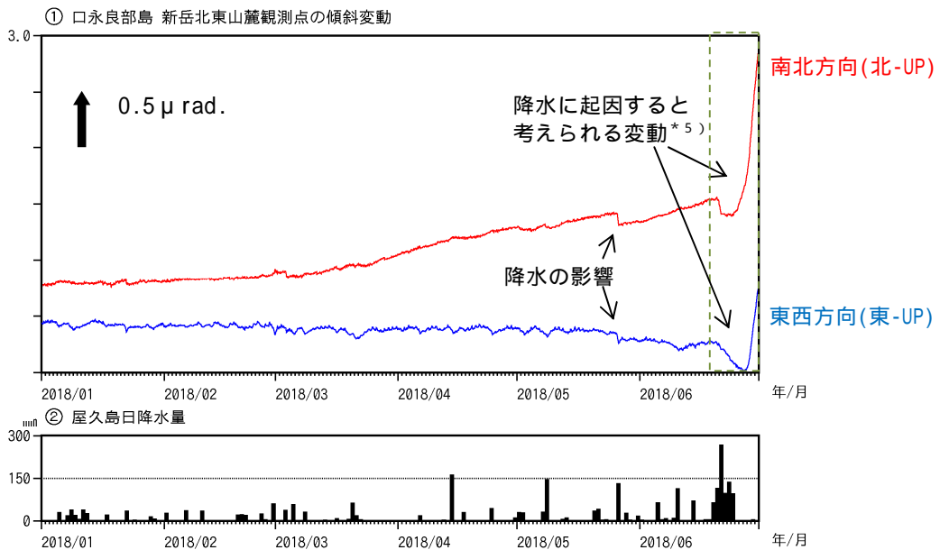
図7 口永良部島 新岳北東山麓観測点の傾斜変動(2018年1月~6月)
