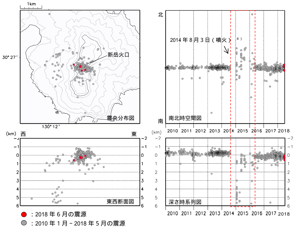
図6 口永良部島 震源分布図(2010年1月~2018年6月)
