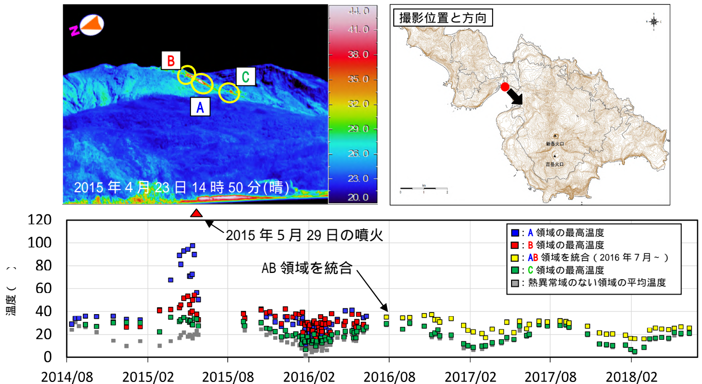
図3 口永良部島 新岳西斜面の熱異常域の温度時系列(2014年8月~2018年6月)
