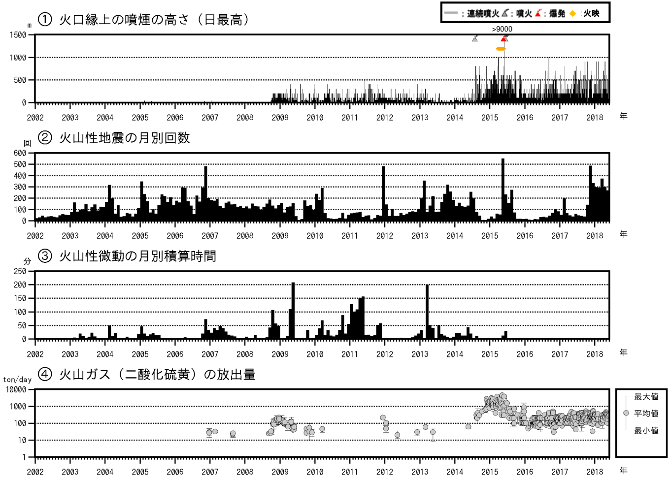
図4 口永良部島 火山活動経過図(2002年1月~2018年6月)
