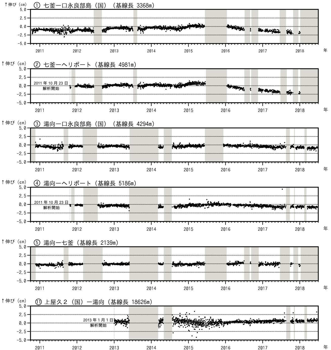
図8 口永良部島 GNSS連続観測による基線長変化(2010年10月~2018年6月)
