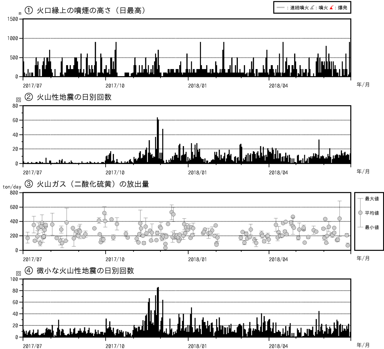
図5 口永良部島 最近の火山活動経過図(2017年7月~2018年6月)
