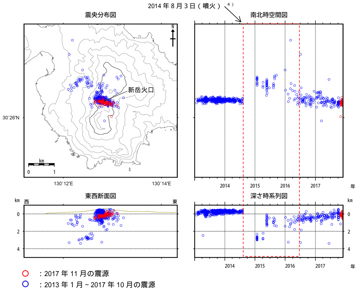
図 6 口永良部島 震源分布図（2013 年 1 月～2017 年 11 月）
