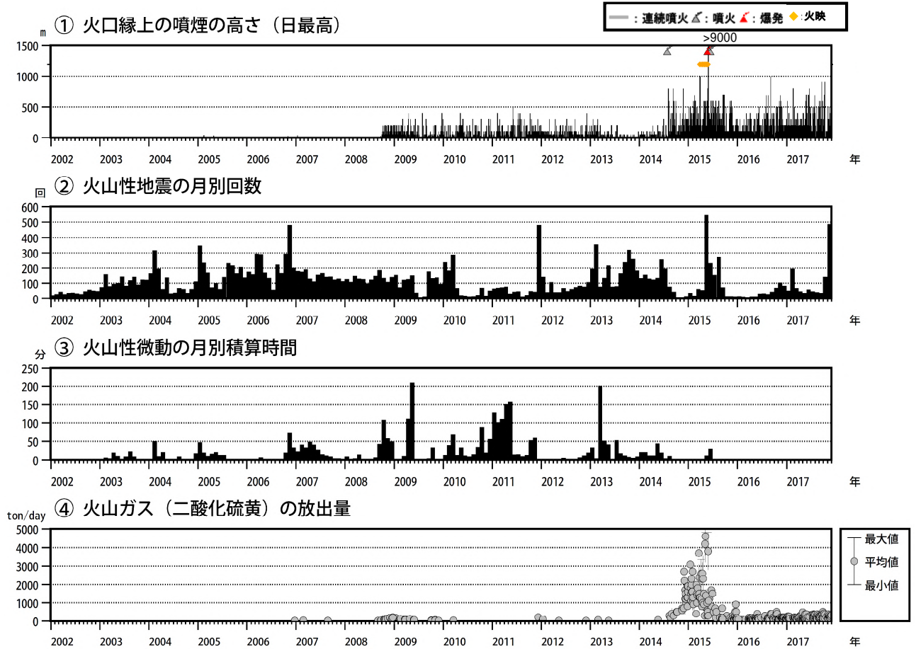
図 4 口永良部島 火山活動経過図（2002 年 1 月～2017 年 11 月）
