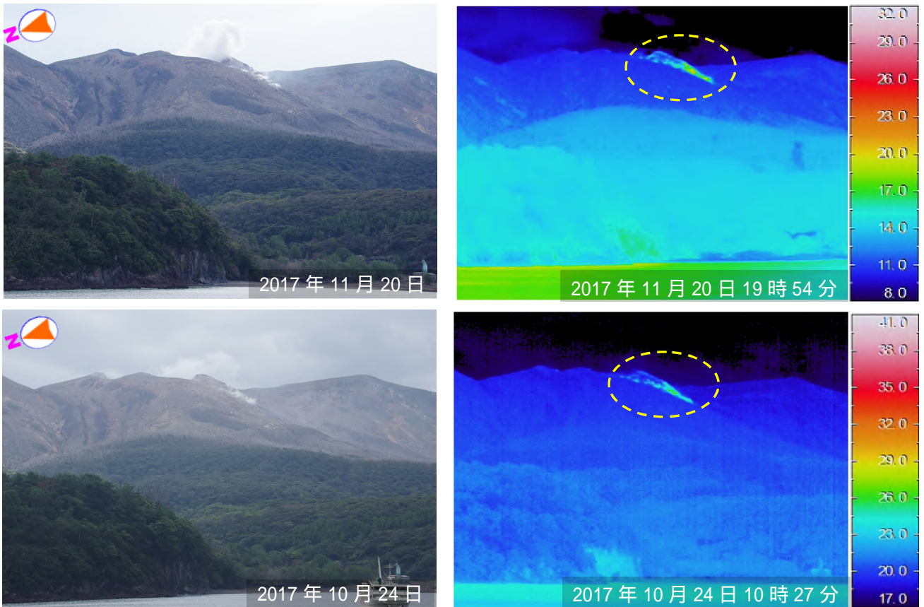
図 2 口永良部島 本村から撮影した新岳火口及び新岳火口西側割れ目付近の可視画像と地表面温度分布 前月（10月24日）と比較して、噴気及び熱異常域（黄色破線）に特段の変化は認められませんでした。
