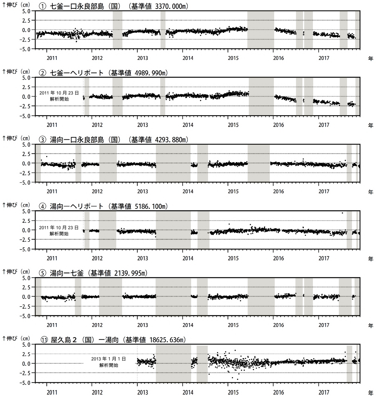
図 8 口永良部島 GNSS 連続観測による基線長変化 (2010 年 10 月 ~ 2017 年 11 月)
