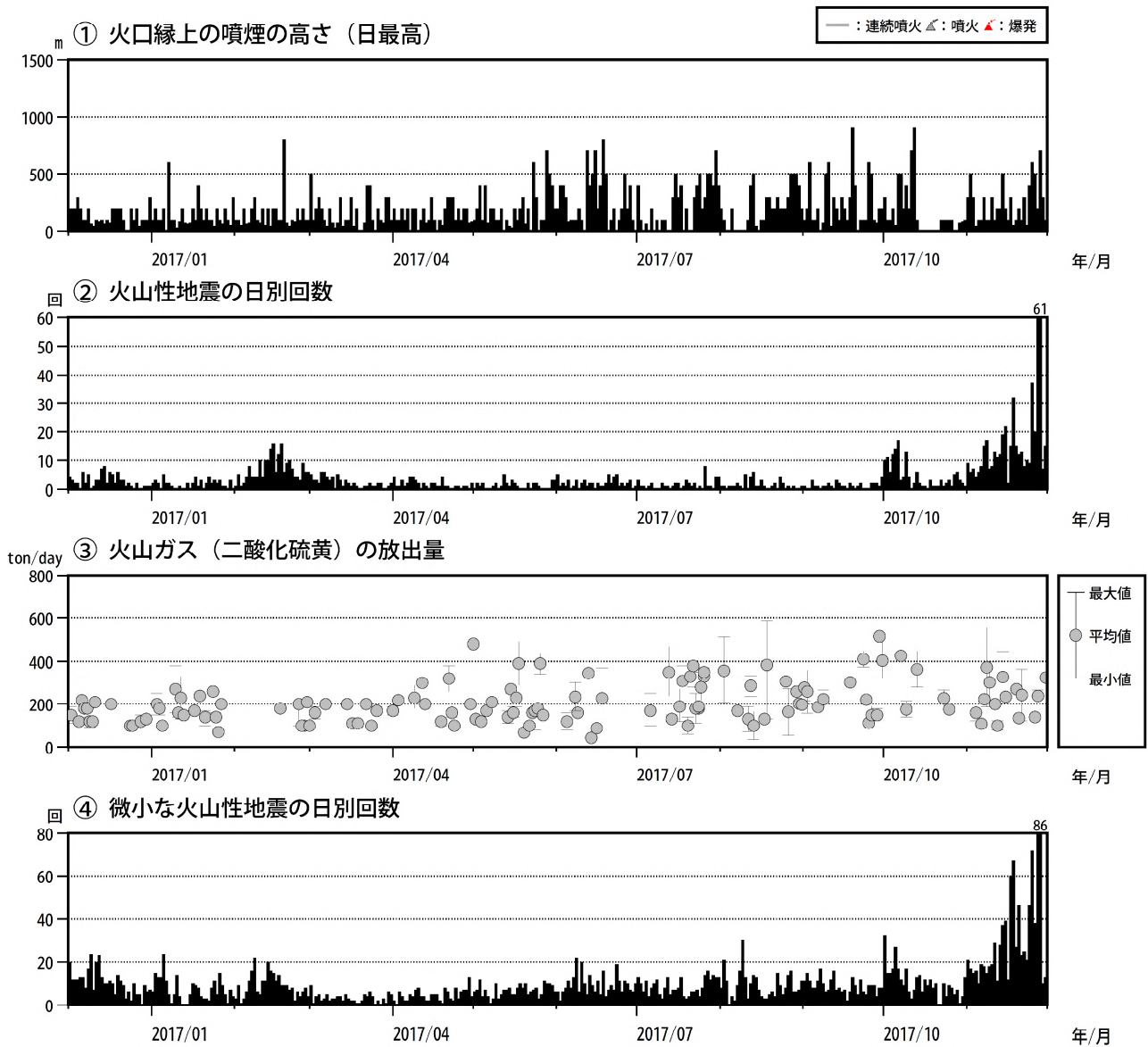
図 5 口永良部島 最近の火山活動経過図（2016 年 12 月～2017 年 11 月）
