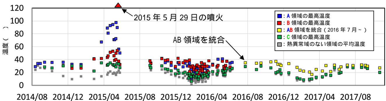
図 3 口永良部島 新岳西斜面の熱異常域の温度時系列（2014年8月～2017年11月）
