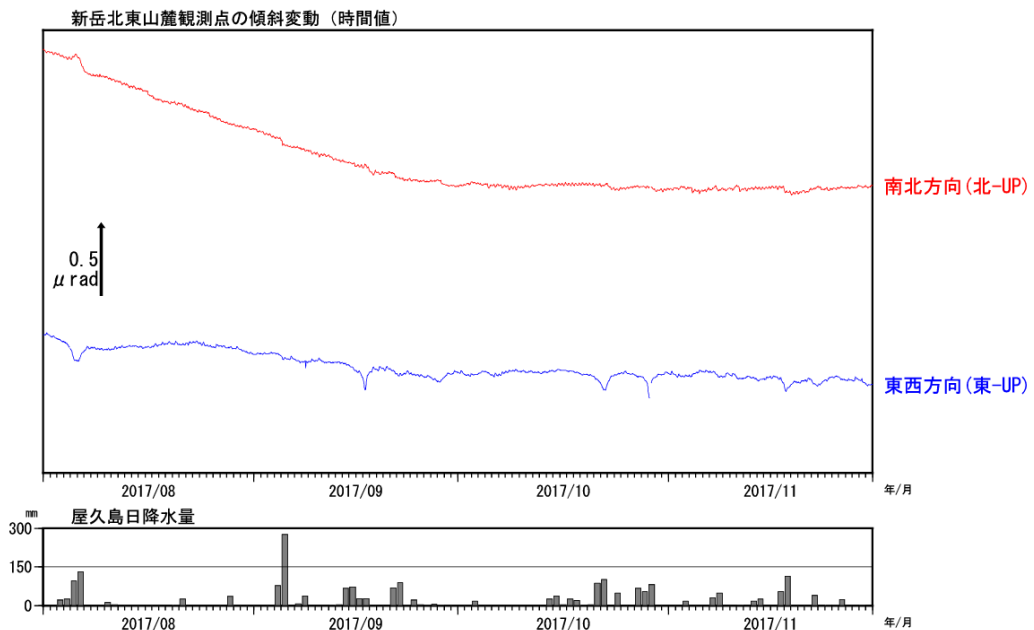
図 7 口永良部島 新岳北東山麓観測点の傾斜変動（2017 年 8 月～2017 年 11 月）
