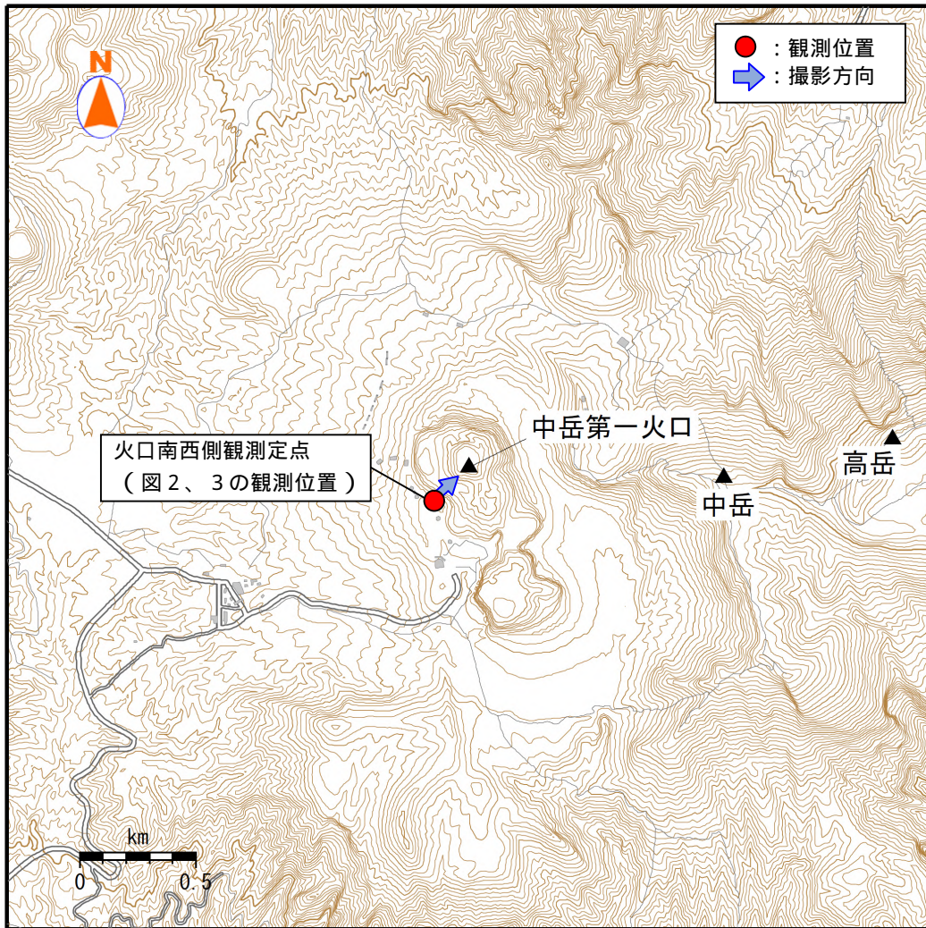
図 4 阿蘇山 中岳第一火口の現地調査観測点
