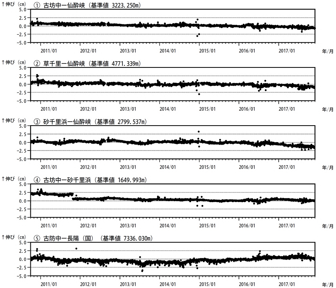
図 9-1 阿蘇山 GNSS連続観測による長期の基線長変化（2010 年 10 月～2017 年 11 月）
