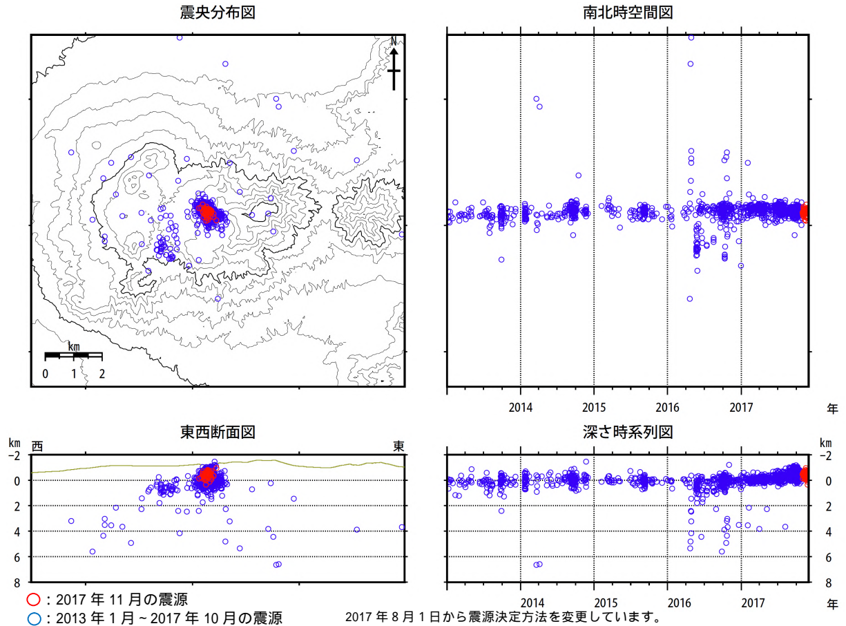
図 7 阿蘇山 火山性地震の震源分布（2013 年 1 月～2017 年 11 月）
