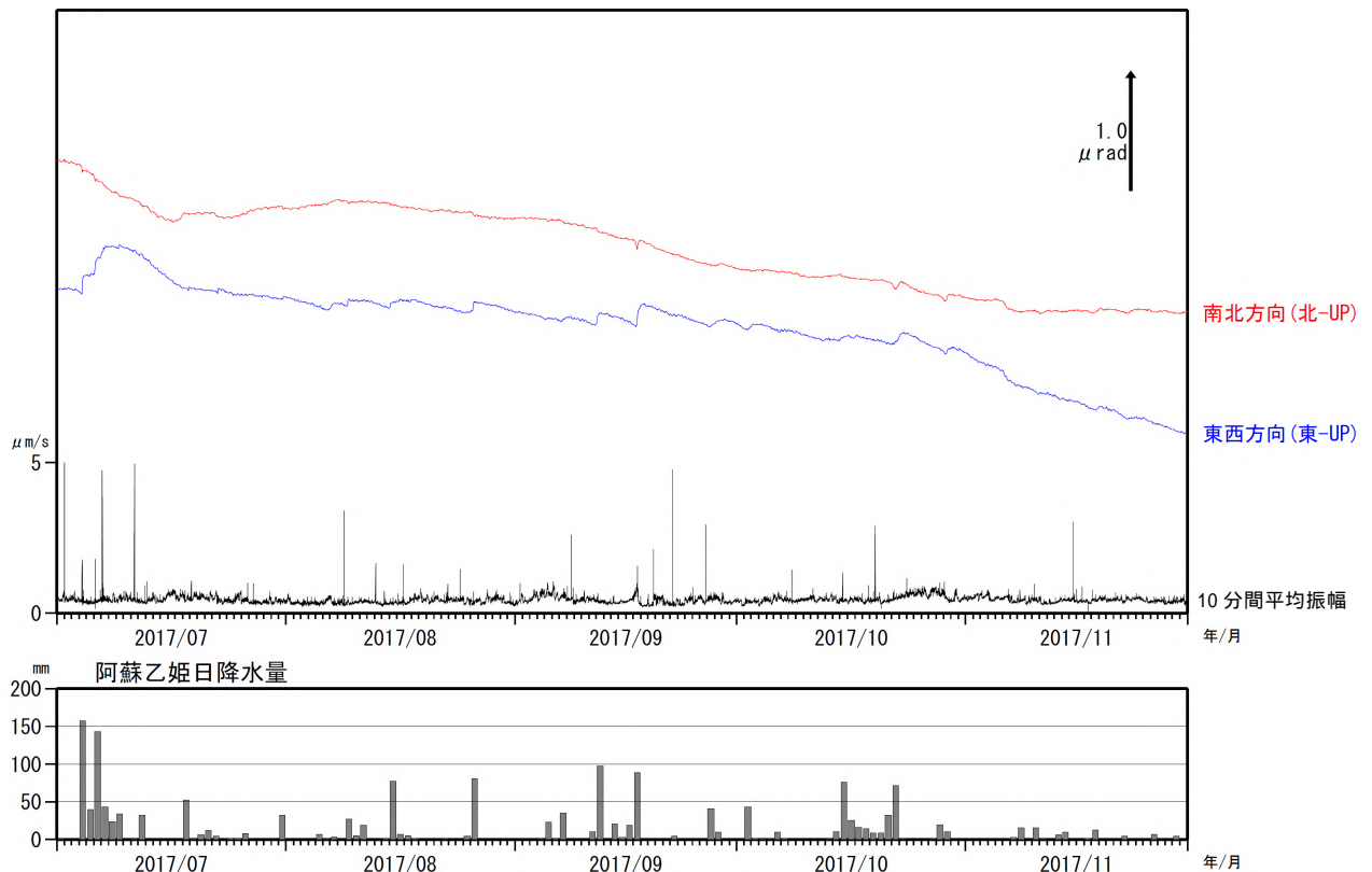
図 8 阿蘇山 古坊中観測点の傾斜変動と中岳西山腹観測点南北動の 10 分間平均振幅（2017 年 7 月～11 月）
