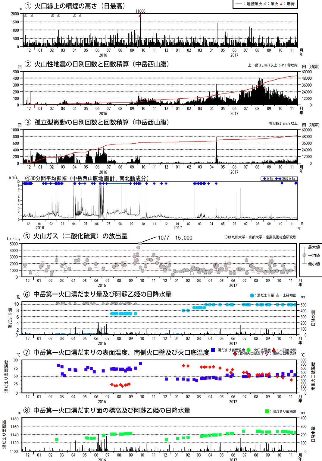
図6 阿蘇山 火山活動経過図（2015年12月～2017年11月）
