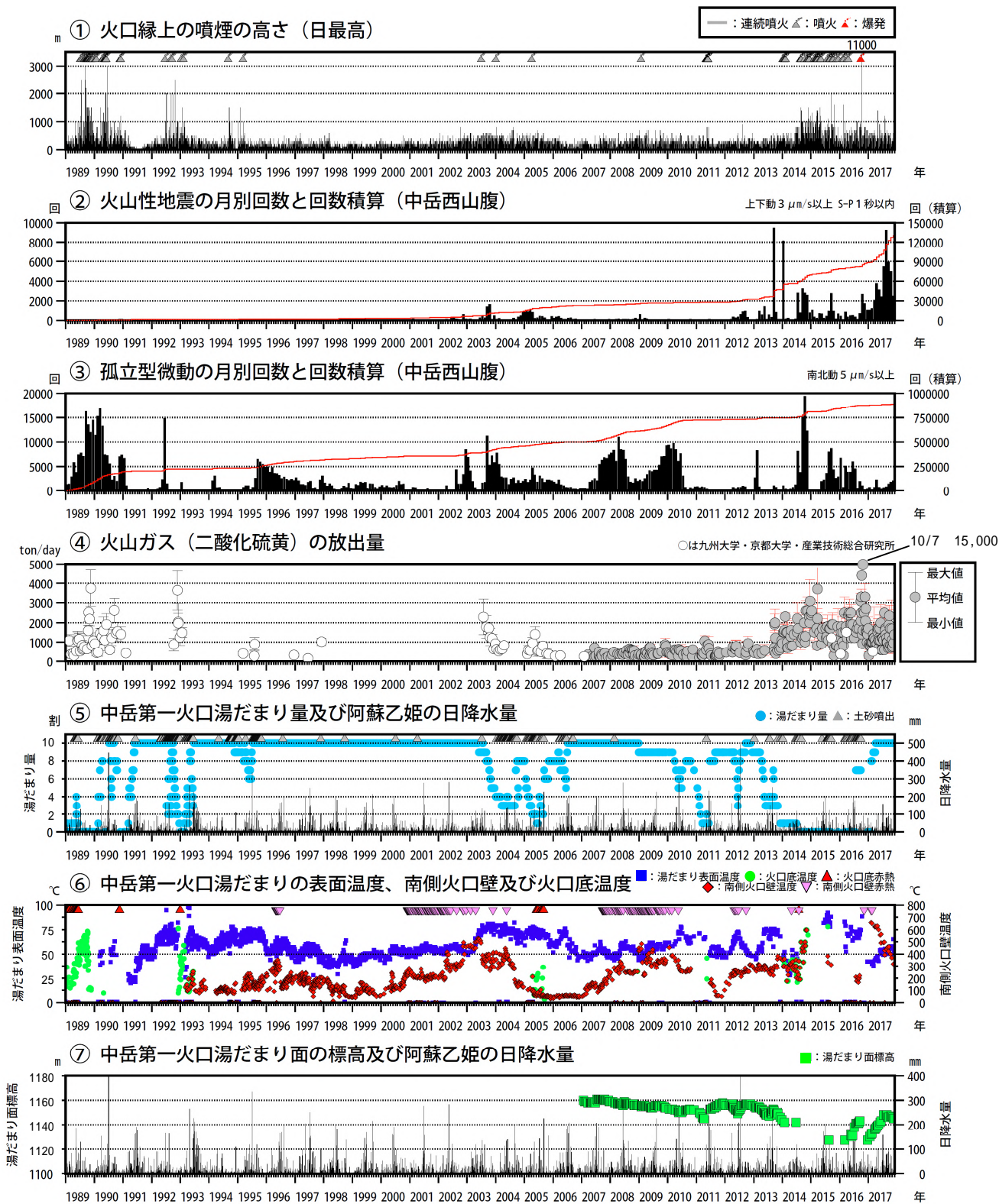
図 5 阿蘇山 火山活動経過図（1989 年 1 月～2017 年 11 月）
