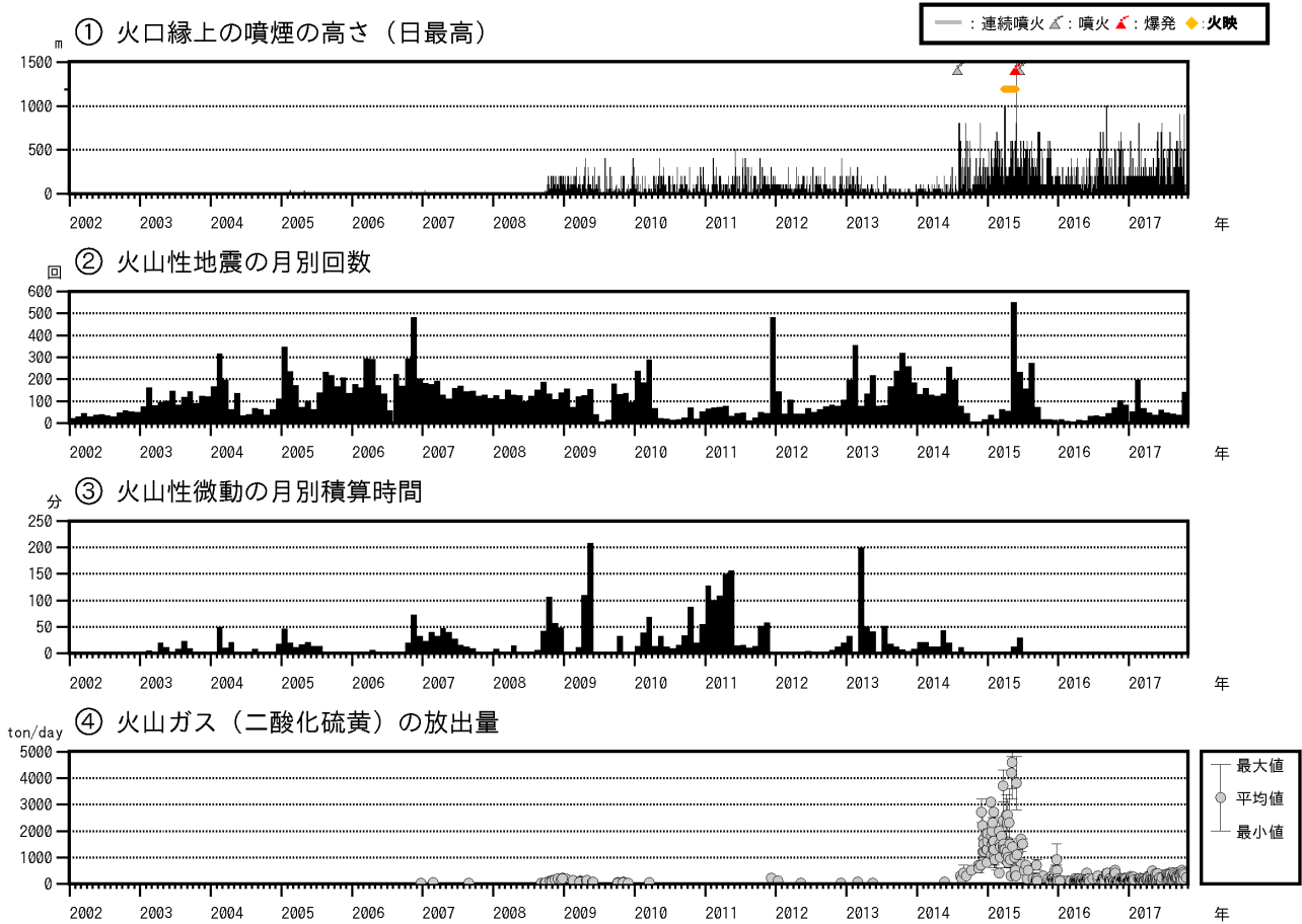
図 4 口永良部島 火山活動経過図（2002 年 1 月～2017 年 10 月）
