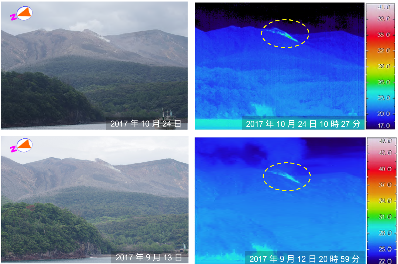
図 2 口永良部島 本村から撮影した新岳火口及び新岳火口西側割れ目付近の可視画像と地表面温度分布 前月（9 月 12、13 日）と比較して、噴気及び熱異常域（黄色破線）に特段の変化は認められませんでした。
