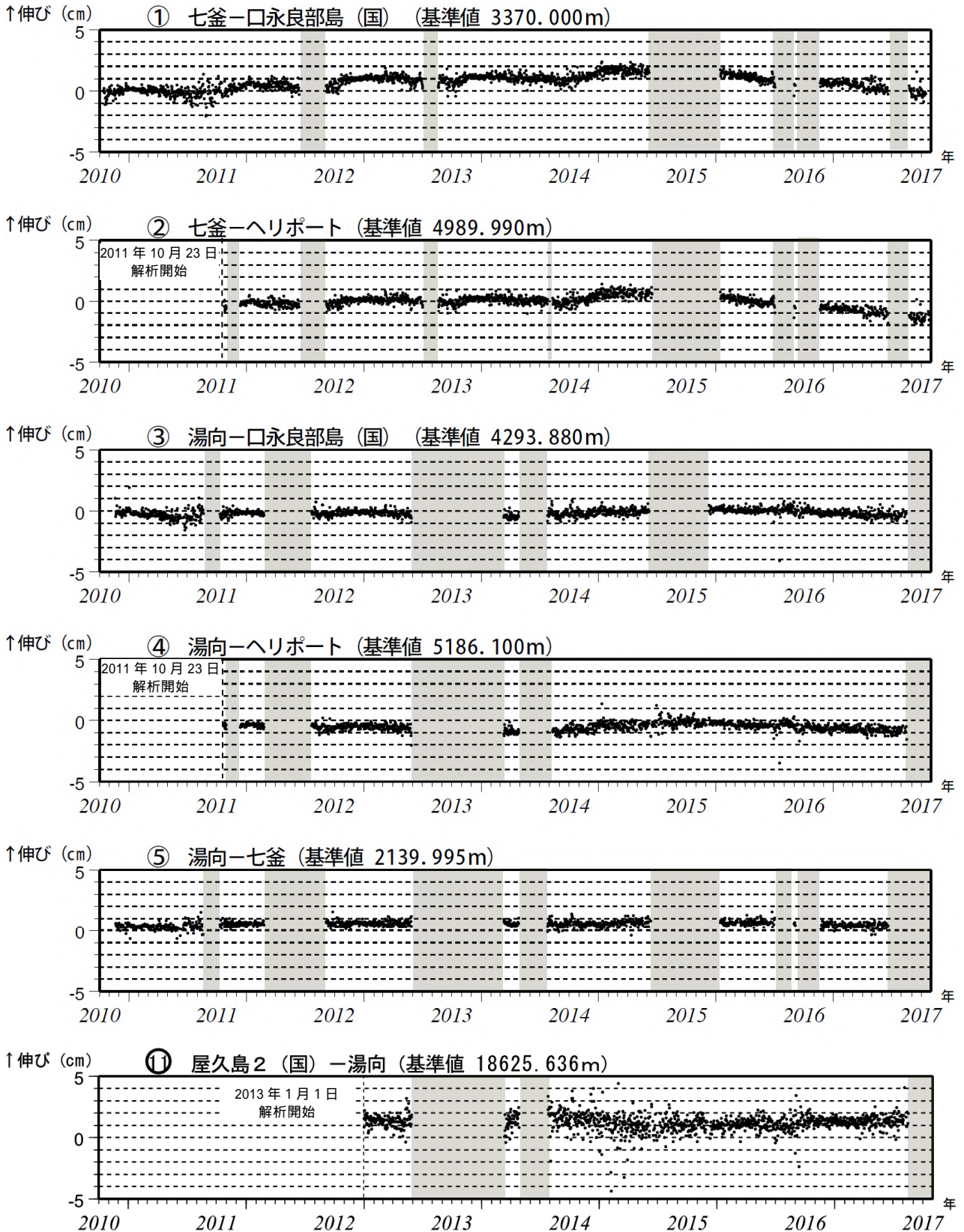
図 7 口永良部島 GNSS 連続観測による基線長変化（2010 年 10 月～2017 年 10 月）
