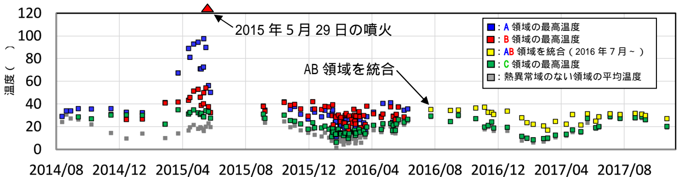
図 3 口永良部島 新岳西斜面の熱異常域の温度時系列（2014 年 8 月～2017 年 10 月）
