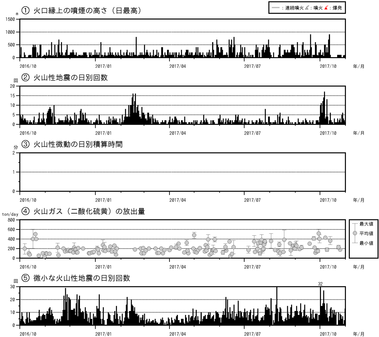
図 5 口永良部島 最近の火山活動経過図（2016 年 10 月～2017 年 10 月）
