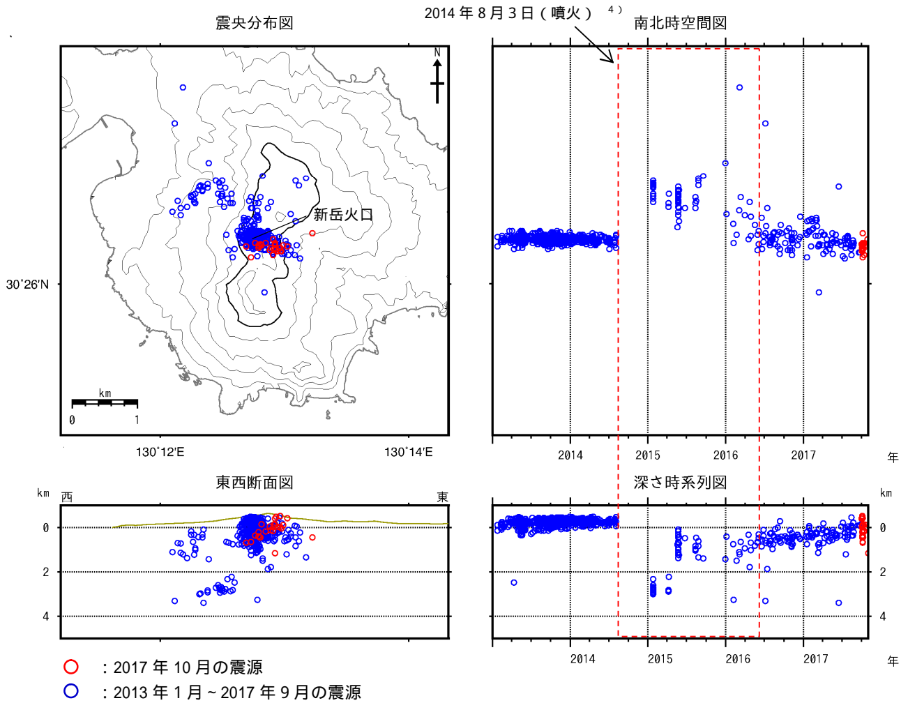
図6 口永良部島 震源分布図（2013年1月～2017年10月）
