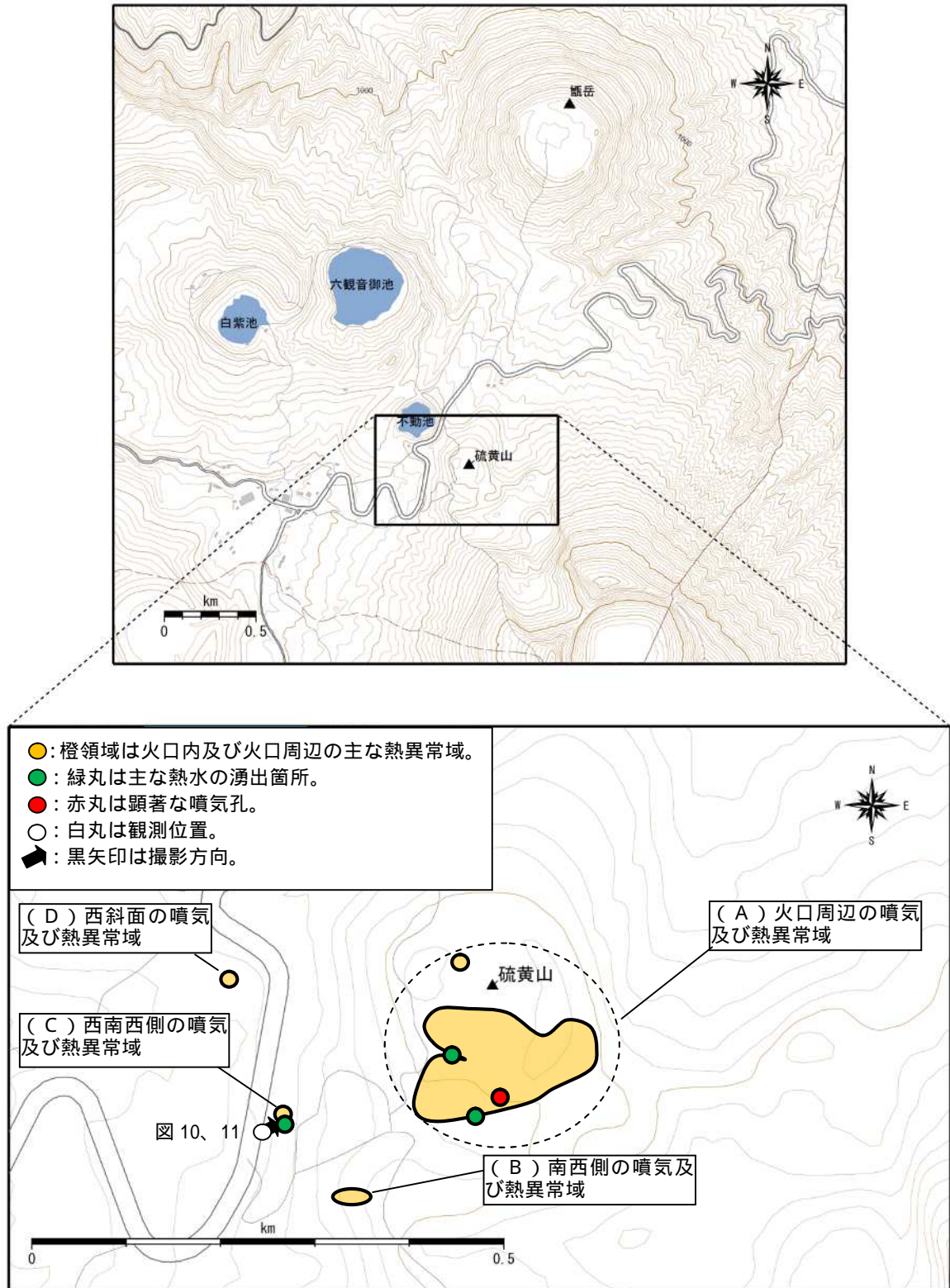
図 12 霧島山（えびの高原(硫黄山)周辺） 主な噴気位置と現地調査観測点位置 噴気及び熱異常域（A）～（D）は、えびの高原監視カメラの画像（図 1）の A～D に対応しています。
