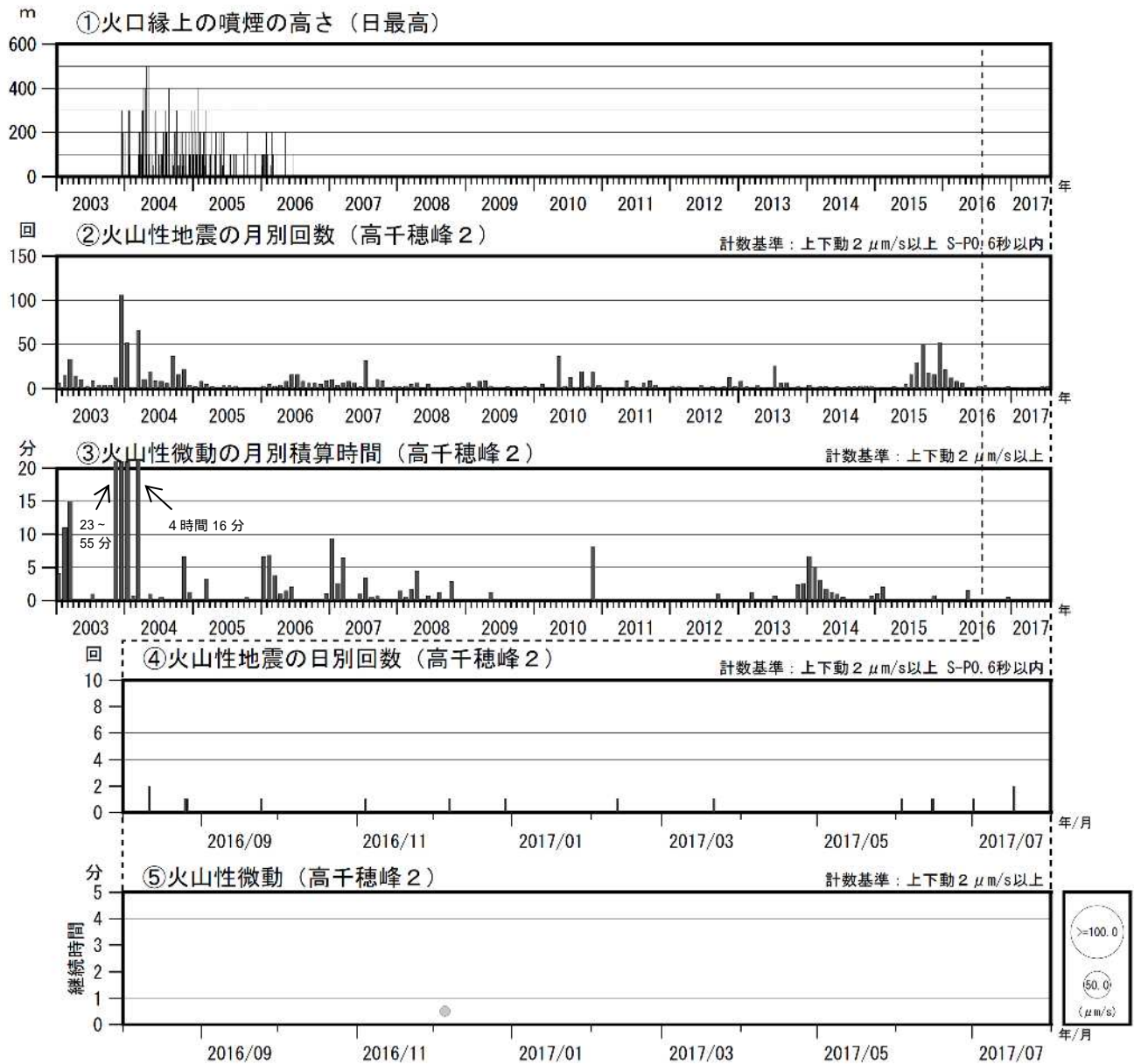
図2 霧島山（御鉢） 火山活動経過図（2003年1月～2017年7月）
