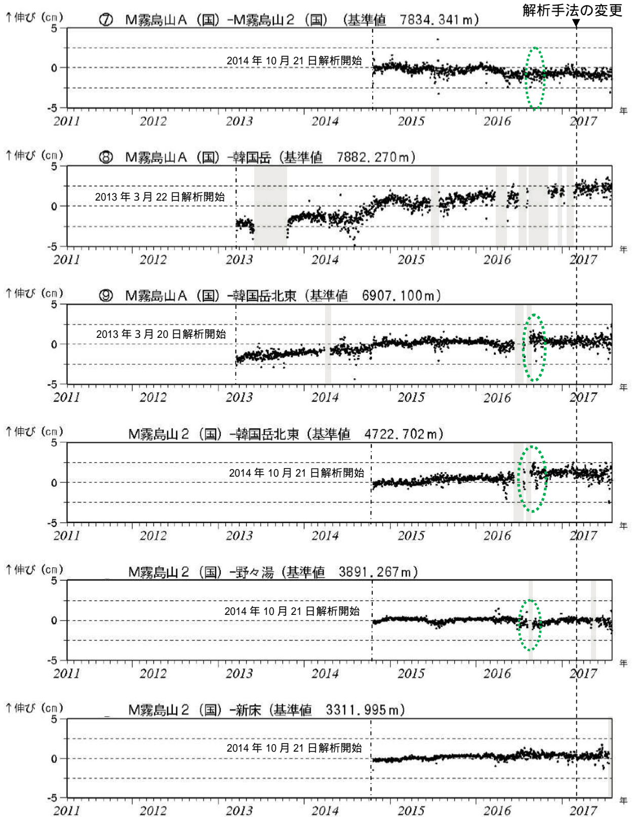
図 6-2 霧島山（えびの高原（硫黄山）周辺） GNSS 連続観測による基線長変化 （2011 年 4 月～2017 年 7 月）
