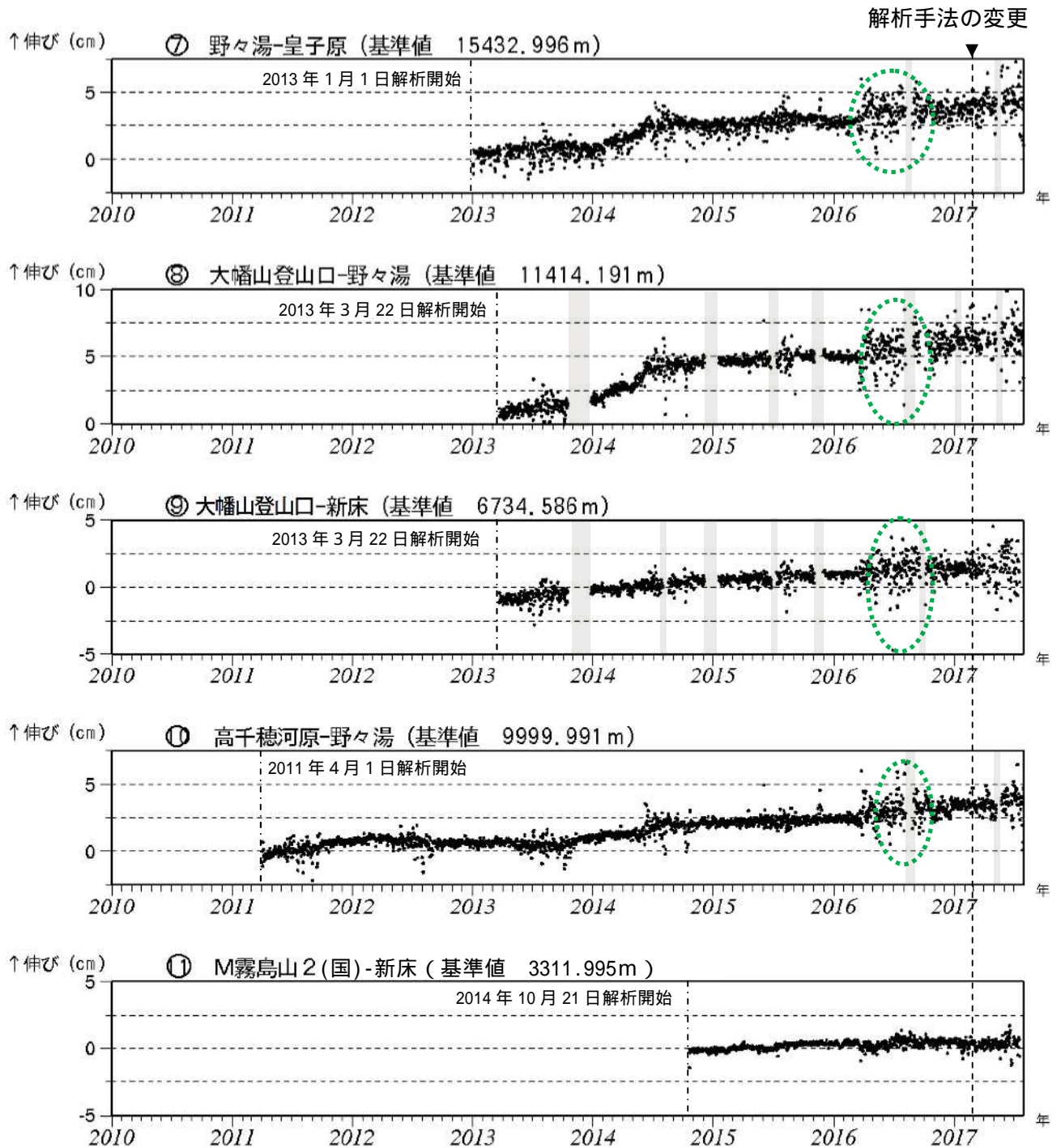
図 5-2 霧島山（新燃岳） GNSS 連続観測による基線長変化（2010 年 1 月～2017 年 7 月）
