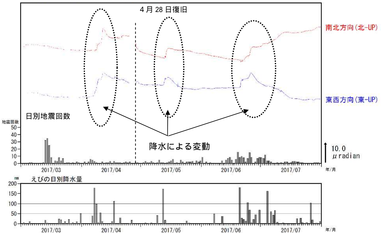
図3 霧島山(新燃岳) 新燃岳北東観測点の傾斜変動と火山性地震の日別回数 (2017年3月~2017年7月)
