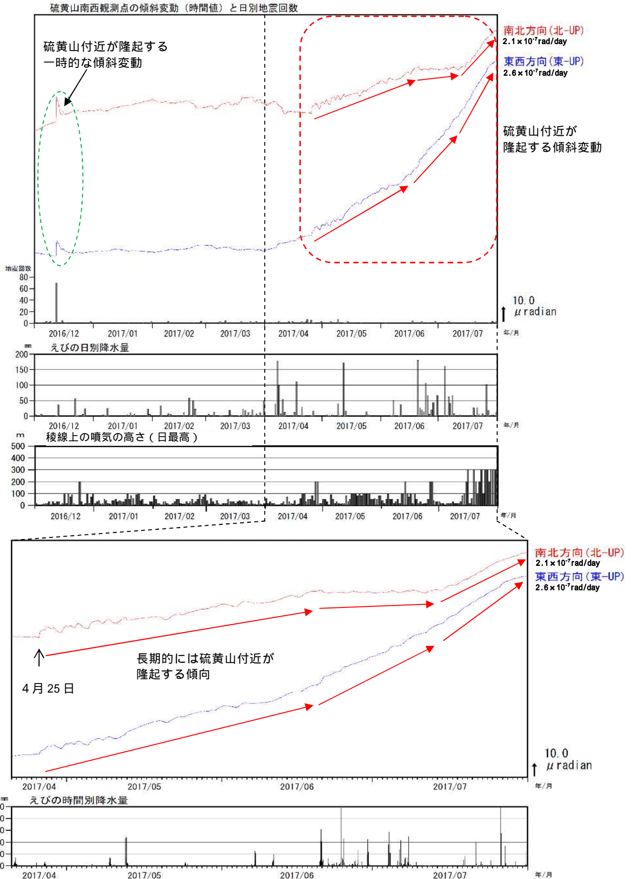
図5 霧島山（えびの高原（硫黄山）周辺）硫黄山南西傾斜計の傾斜変動と火山性地震の日別回数（2016年12月～2017年7月）
