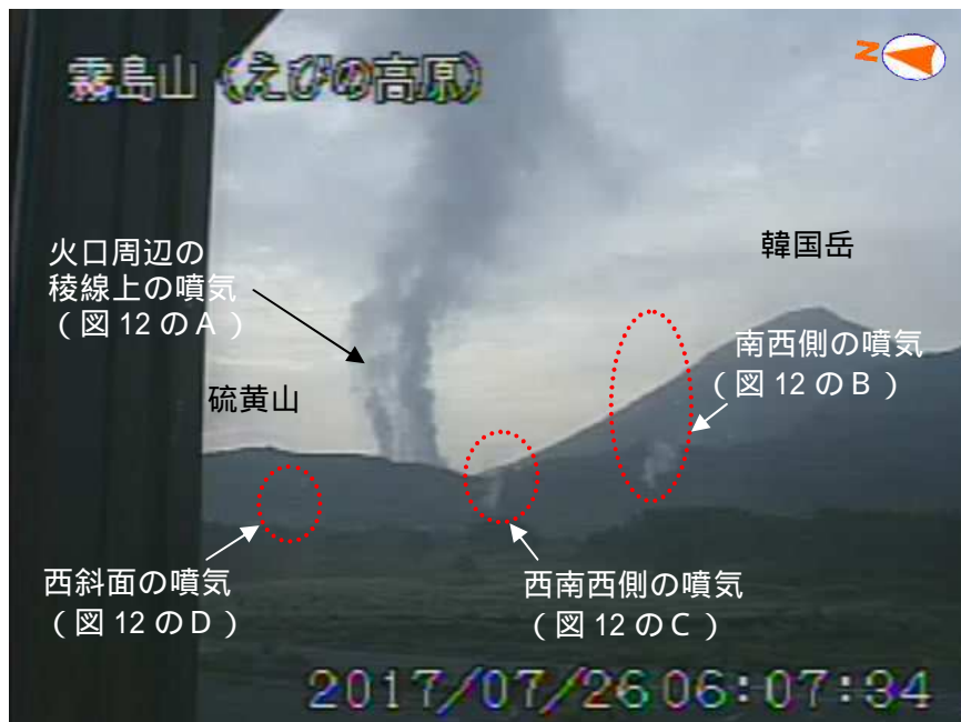
図 1 霧島山（えびの高原（硫黄山）周辺） 硫黄山付近の状況 （7 月 26 日 えびの高原監視カメラによる）
