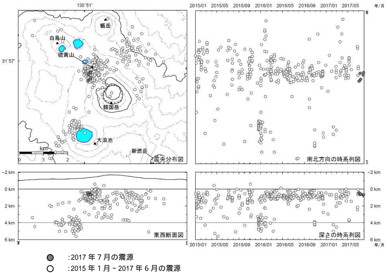
図 3 霧島山（えびの高原（硫黄山）周辺） 震源分布図（2015 年 1 月～2017 年 7 月）
