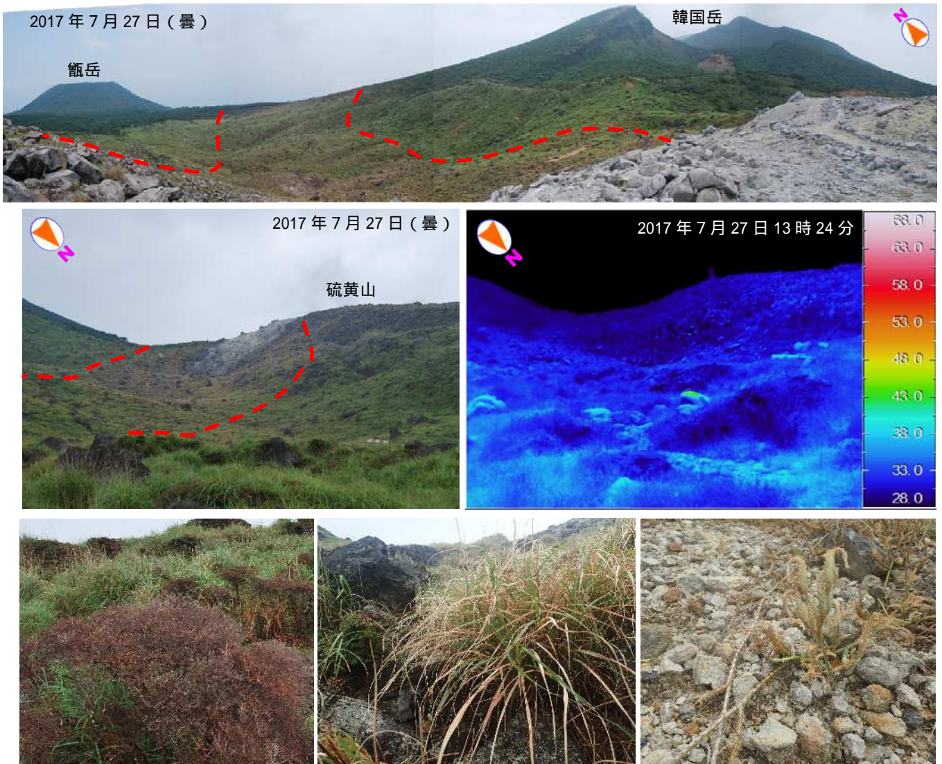
図 8 霧島山(えびの高原(硫黄山)周辺) 硫黄山火口の北東側に分布する変色域の状況(7月27日) 上段: 硫黄山の稜線から撮影 中段: 硫黄山北東側の可視及び熱画像 下段: 植物の枯死や葉の変色の状況 ・硫黄山火口の北東側(赤破線の内側)で植物が枯死(変色)していることを確認しました。 ・硫黄山の北東斜面には熱異常域は認められませんでした。
