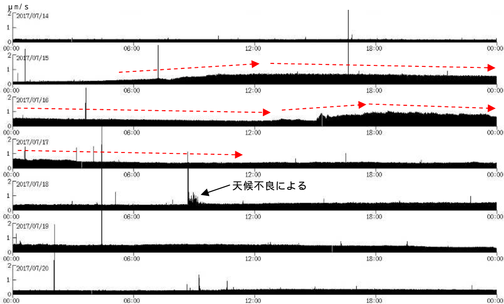
図 4 霧島山（えびの高原（硫黄山）周辺） 火口近傍に設置した地震計の 1 分間平均振幅の推移（霧島硫黄山 2 観測点上下動：2017 年 7 月 14 日～7 月 20 日）
