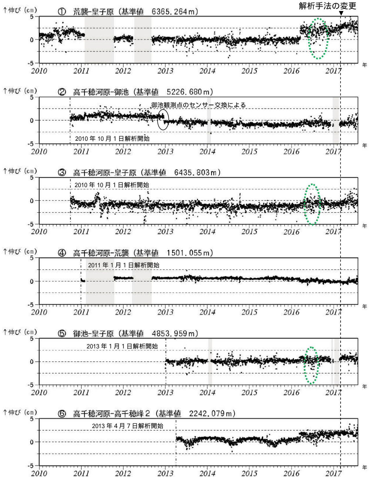
図3 霧島山（御鉢） GNSS 連続観測による基線長変化（2010年1月～2017年7月）
