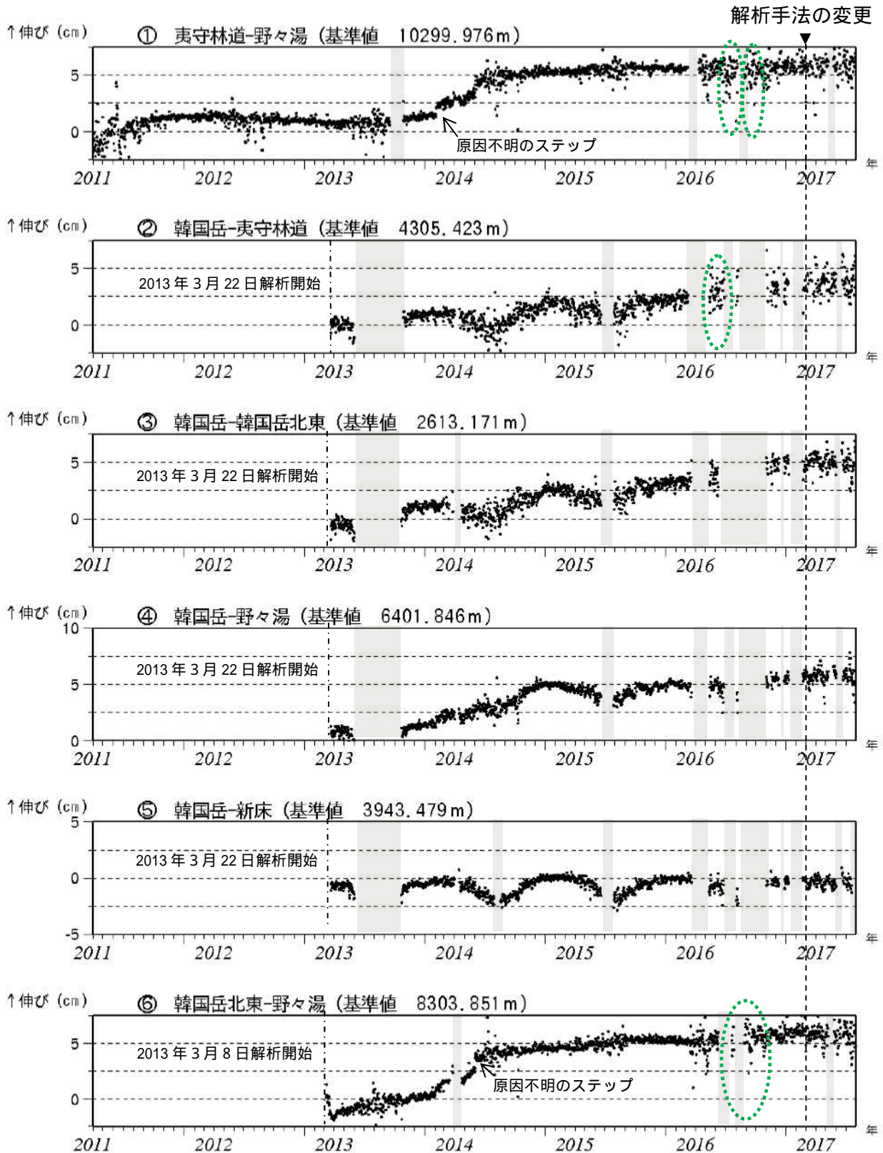
図 6-1 霧島山(えびの高原(硫黄山)周辺) GNSS 連続観測による基線長変化 (2011年4月~2017年7月)
