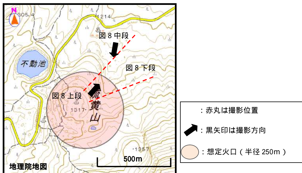
図 9 霧島山(えびの高原(硫黄山)周辺) 図 8 の撮影位置と変色域の分布領域 硫黄山火口の北東方向(赤破線の内側)で植物の枯死や草木が変色していることを確認しました。
