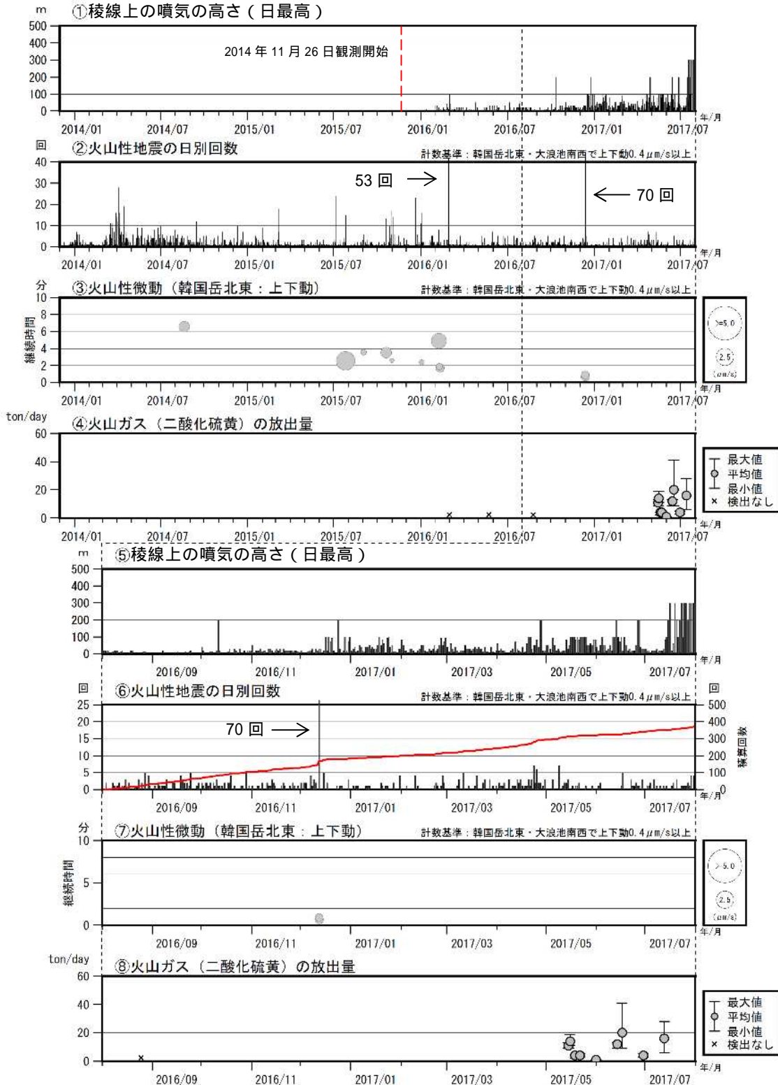
図2 霧島山（えびの高原（硫黄山）周辺）火山活動経過図（2013年12月～2017年7月）
