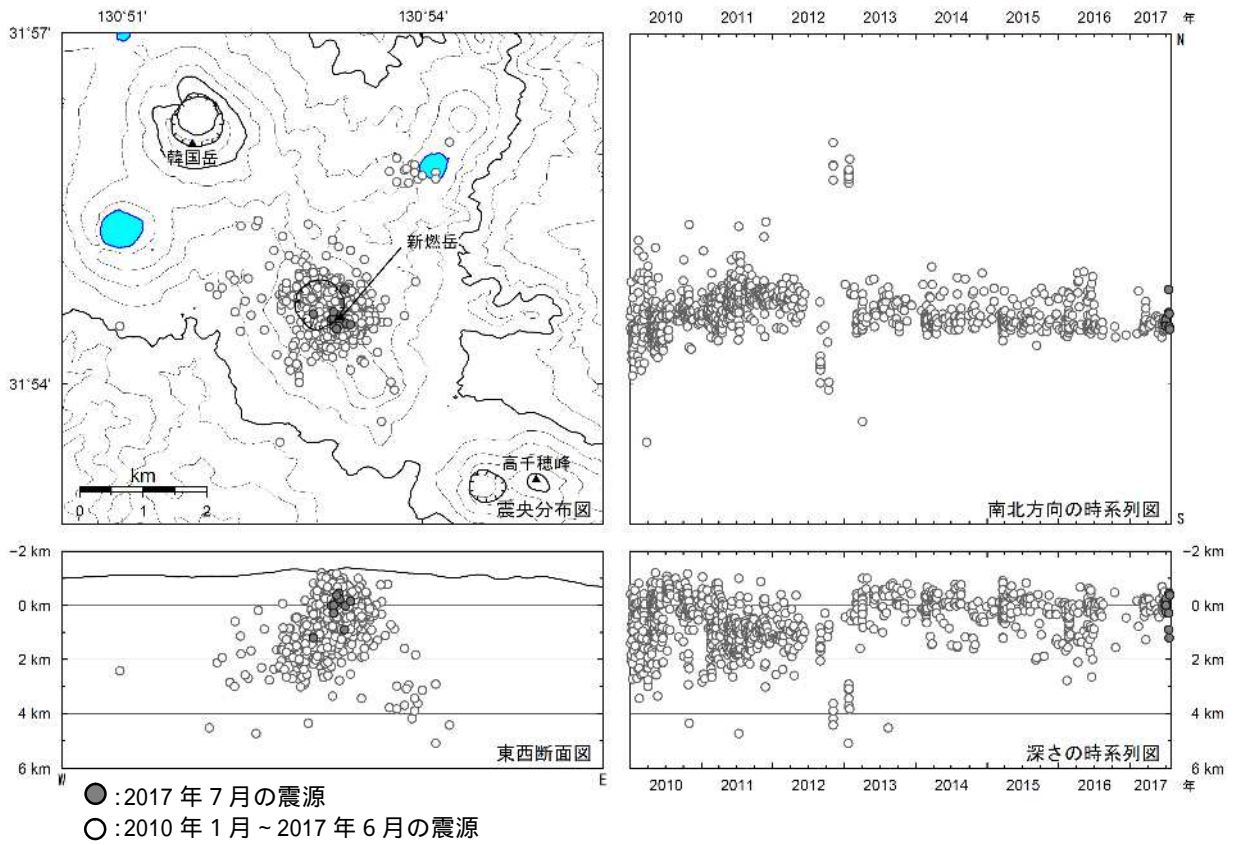
図2 霧島山(新燃岳) 震源分布図(2010年1月~2017年7月)
