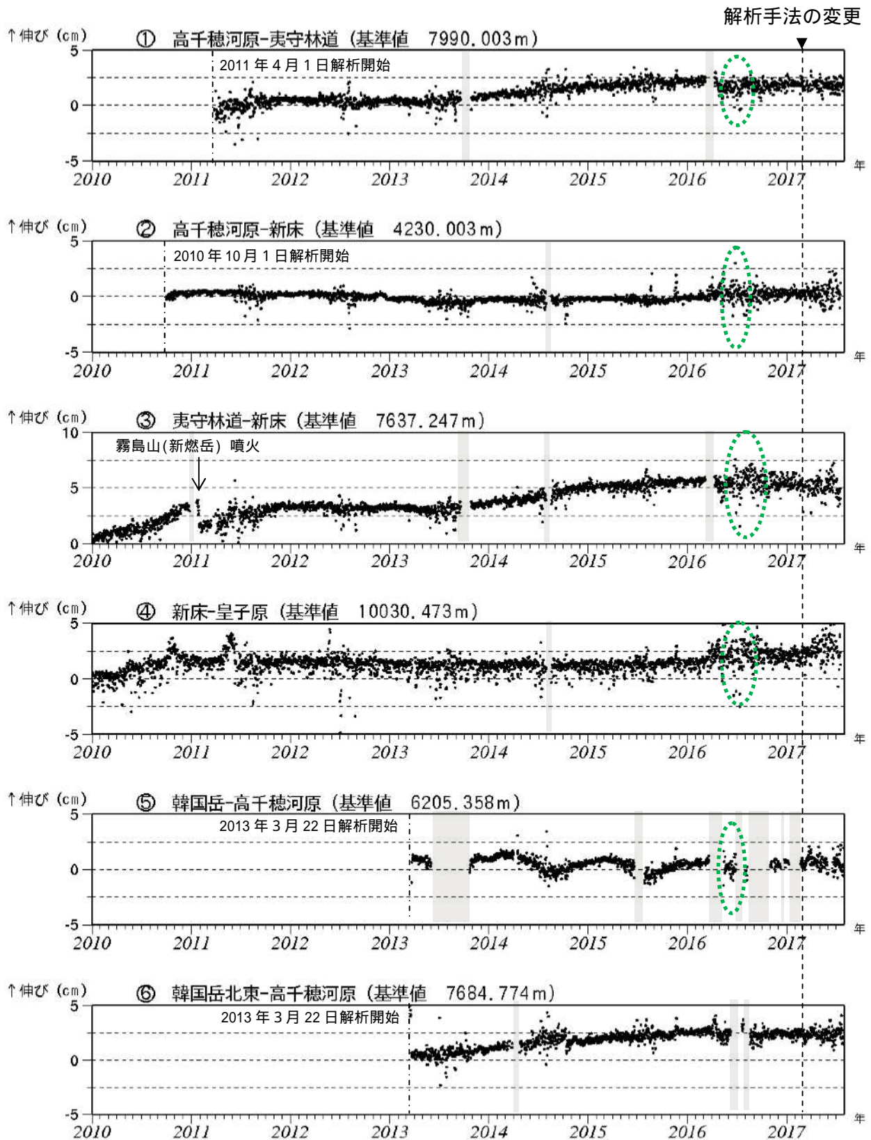
図 5-1 霧島山（新燃岳） GNSS 連続観測による基線長変化（2010 年 1 月～2017 年 7 月）
