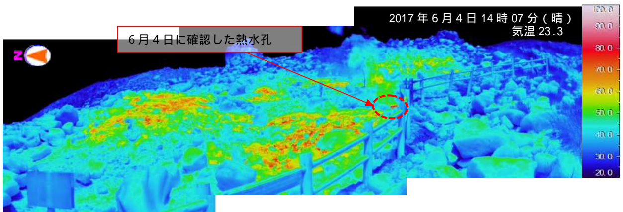
図 10 霧島山(えびの高原(硫黄山)周辺) 硫黄山西南西側(図 12 のC及びその周辺)の状況 (韓国岳登山口から観測)
