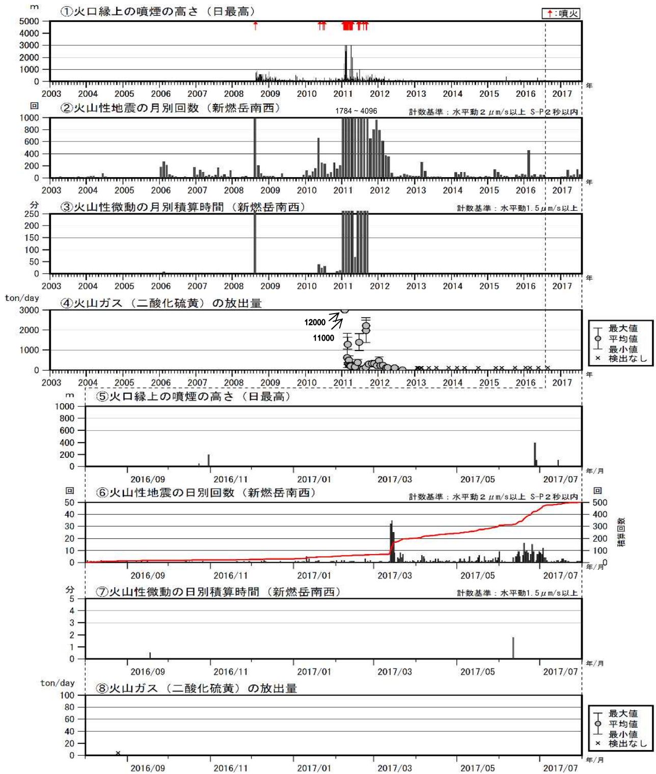
図4 霧島山（新燃岳） 火山活動経過図（2003年1月～2017年7月）
