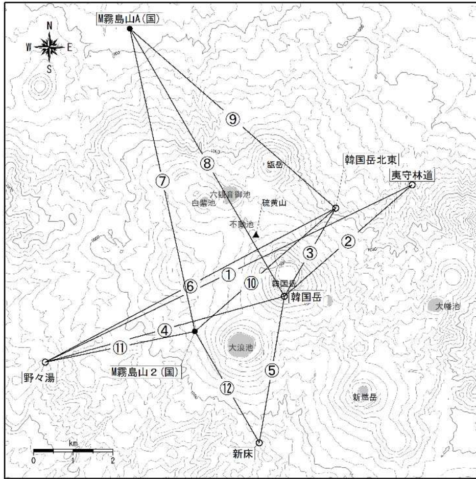
図7 霧島山（えびの高原（硫黄山）周辺） GNSS 連続観測点と基線番号
