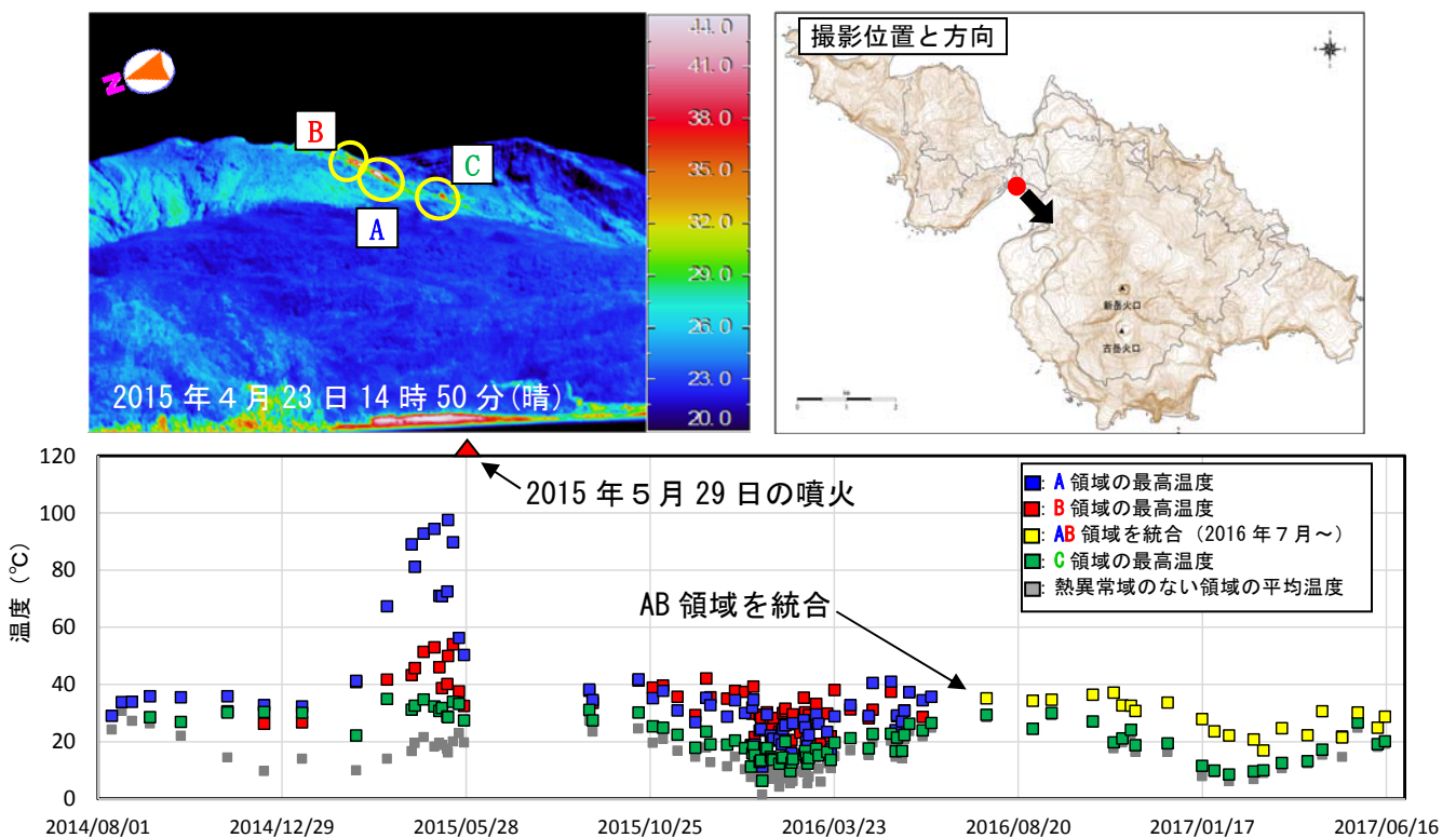
図3 口永良部島 新岳西斜面の熱異常域の温度時系列（2014年8月～2017年6月） ＜6月の状況＞
