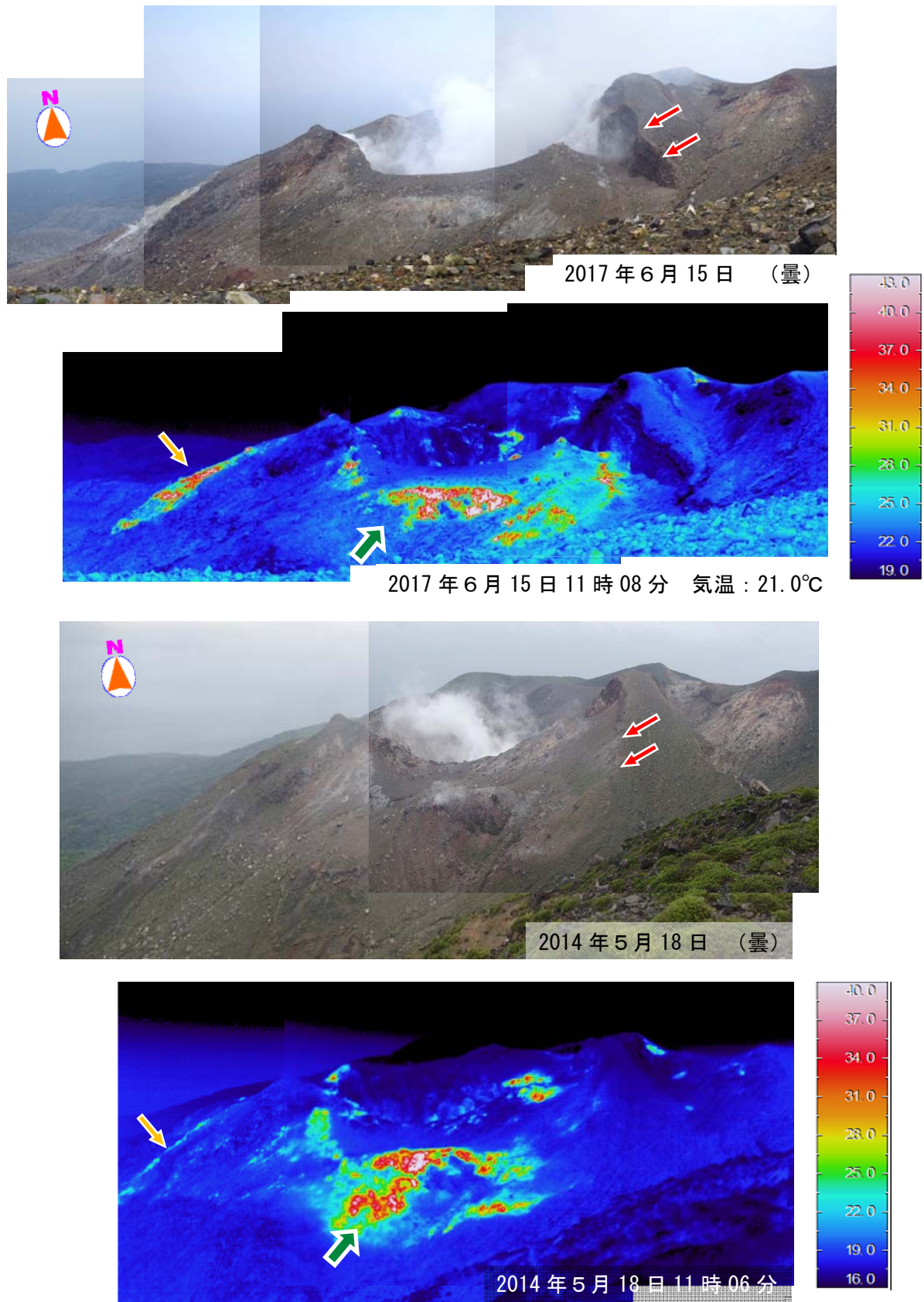
図4 口永良部島 新岳火口南西側の可視画像および赤外熱映像装置による地表面温度分布 ・火口の南東側（図中の赤矢印）には2014年8月3日噴火で出現した割れ目が確認できます。 ・地表面温度分布は、前回（2015年5月18日）と比べて、火口外壁南側の熱異常域の一部が縮小していました（図中の緑矢印）。 ・火口西側割れ目の熱異常（図中の黄矢印）は、2014年8月の噴火前の2014年5月18日よりも温度が高く拡大していました。
