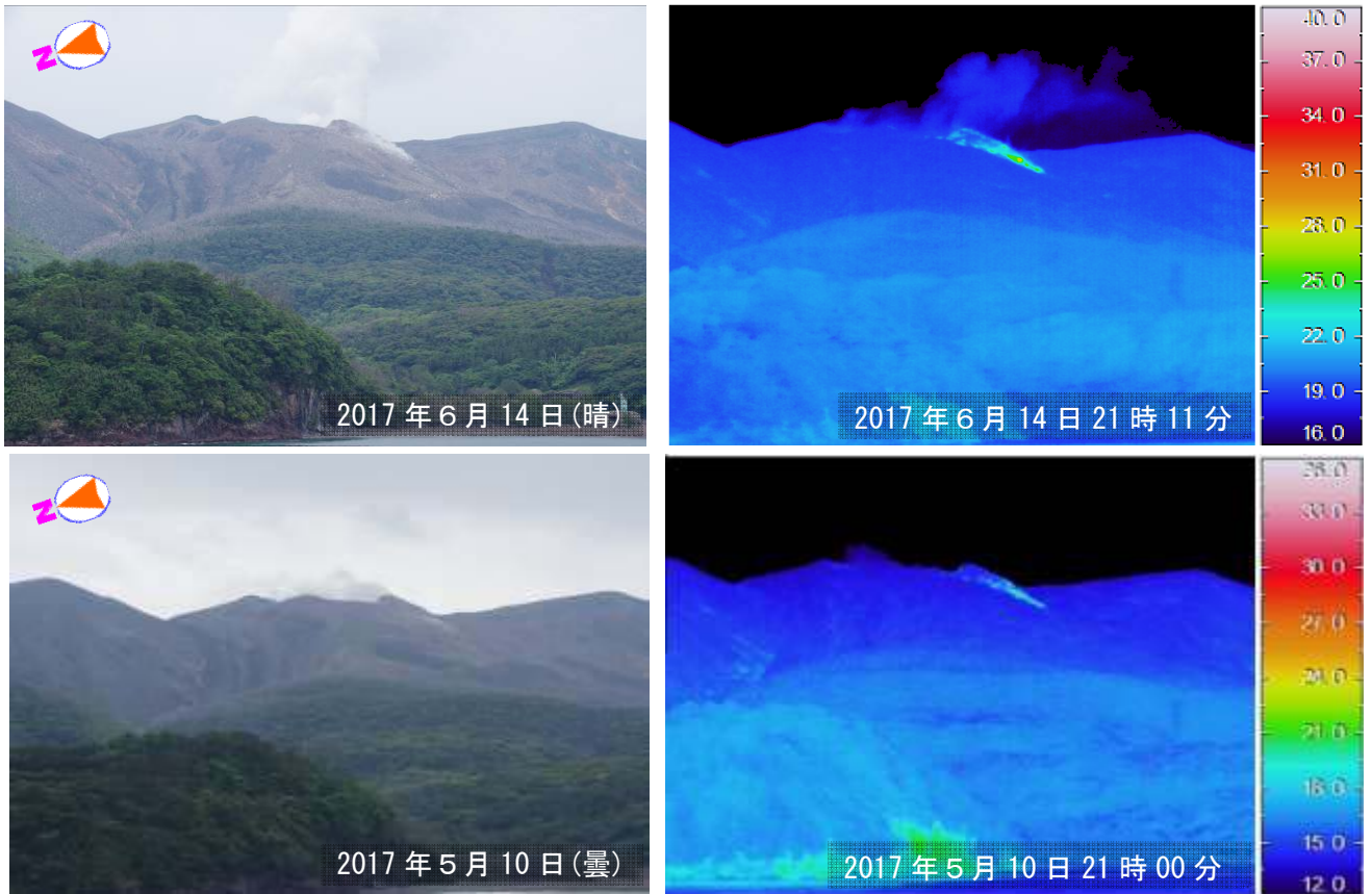
図2 口永良部島 本村から撮影した可視画像と地表面温度分布 前月（5月10日）と比較して、噴気及び熱異常域に特段の変化は認められませんでした。
