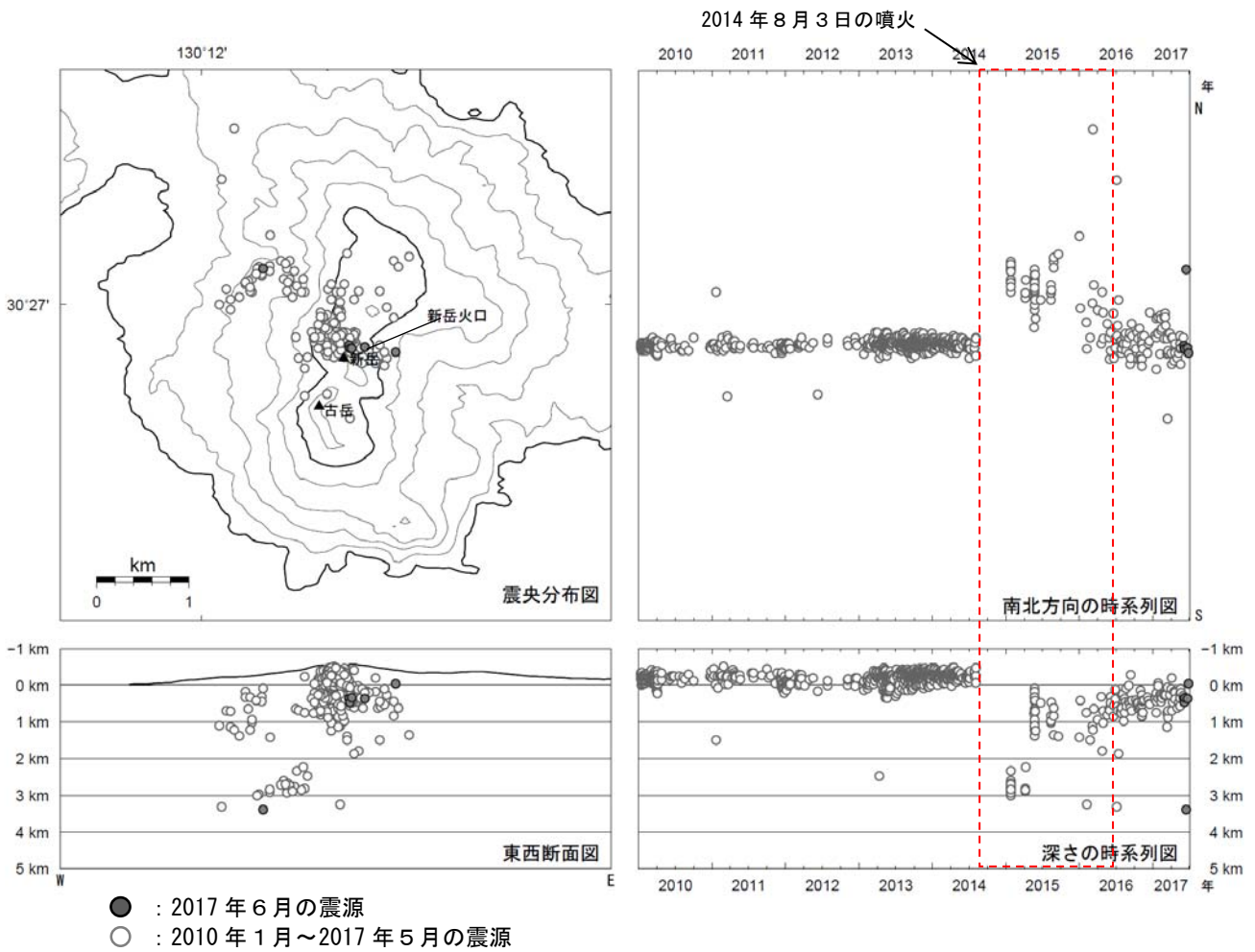
図9 口永良部島 震源分布図（2010年1月～2017年6月）
