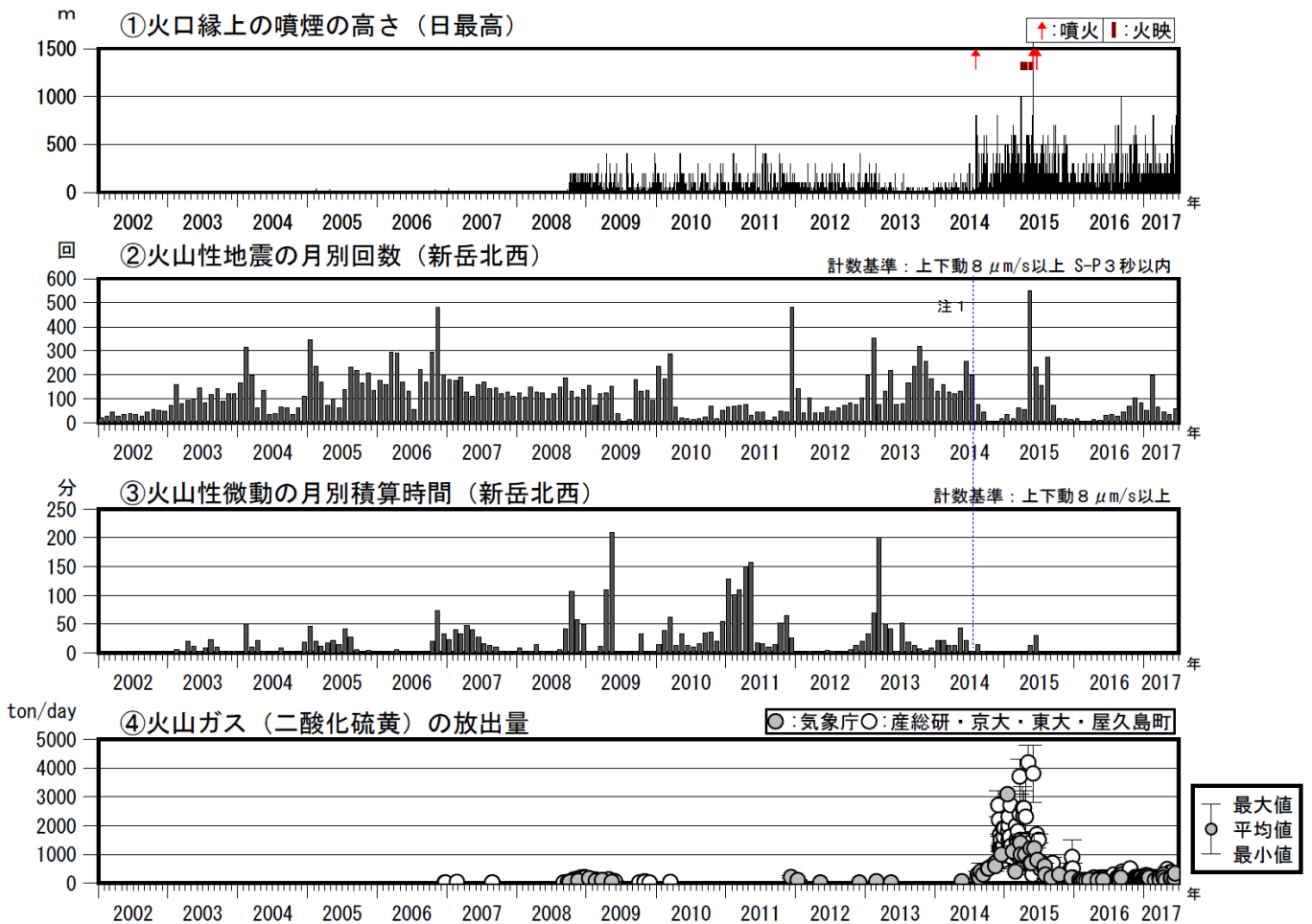
図7 口永良部島 火山活動経過図（2002年1月～2017年6月）
