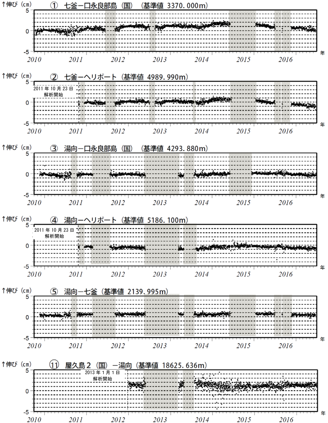
図 10 口永良部島 GNSS 連続観測による基線長変化 (2010 年 10 月～2017 年 6 月)
