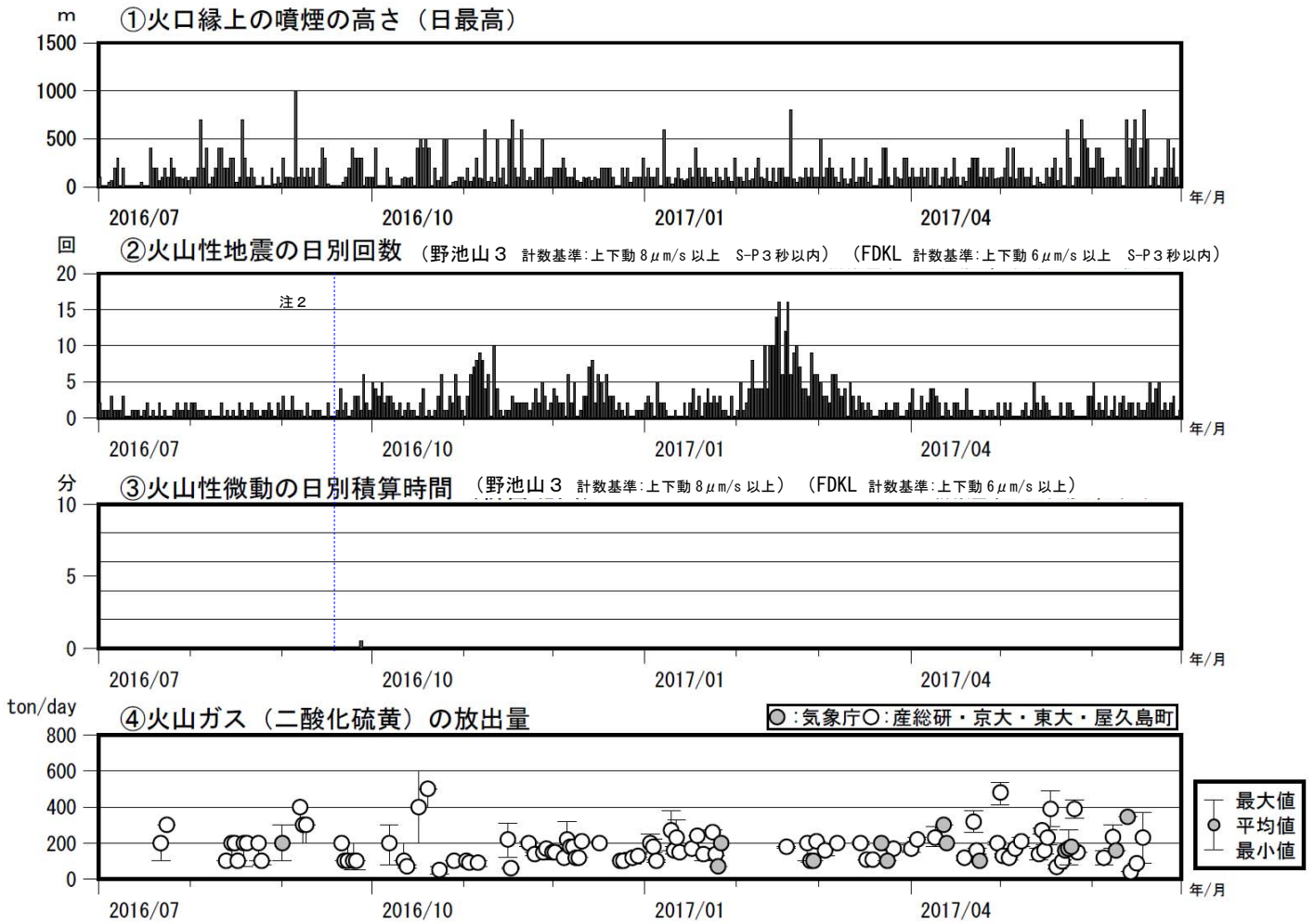
図8 口永良部島 最近の火山活動経過図（2016年7月～2017年6月）
