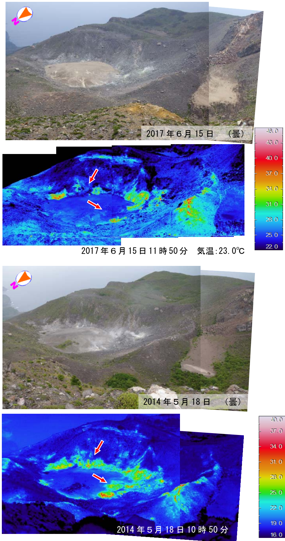
図5 口永良部島 古岳火口の可視画像および赤外熱映像装置による地表面温度分布
