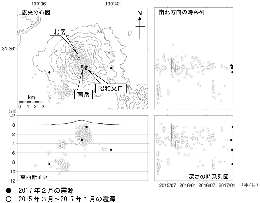
図 9 桜島 火山性地震の震源分布図（2015 年 3 月～2017 年 2 月）
