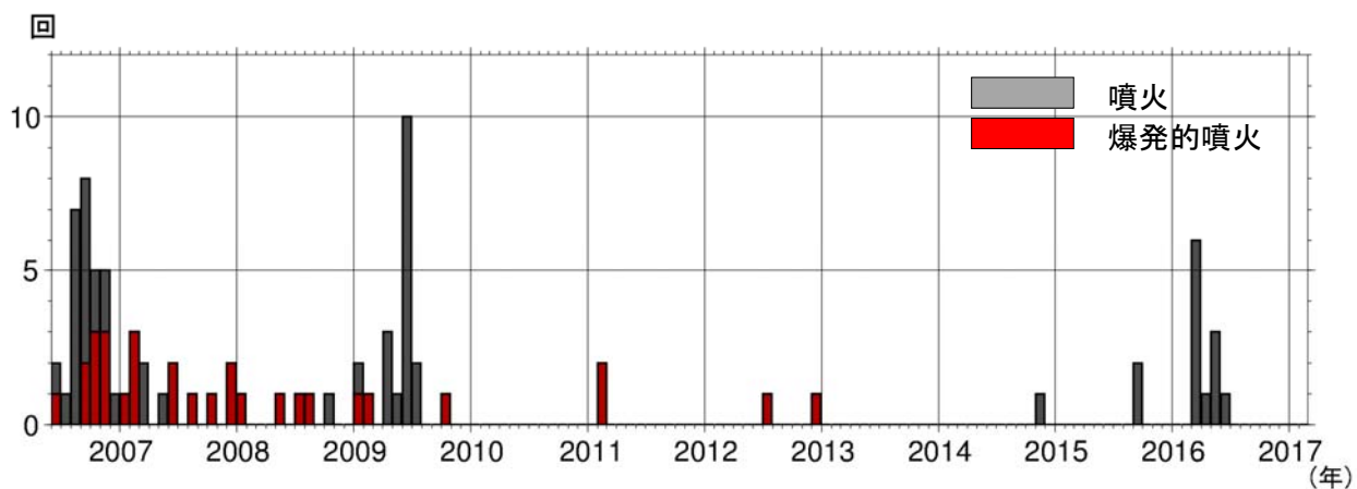
図2 桜島 昭和火口（上図）と南岳山頂火口（下図）の月別噴火回数（灰色）と月別爆発回数（赤色）（2006年1月～2017年2月）
