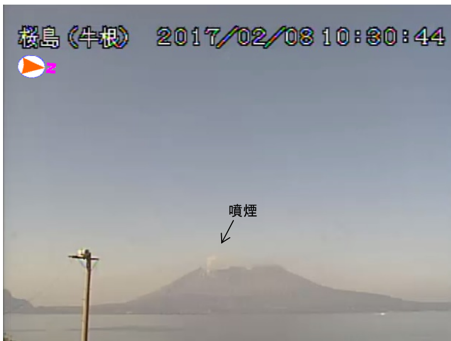
図1 桜島 噴煙の状況（2月8日10時30分 牛根監視カメラによる） ・桜島では、ごく小規模な噴火も含め、噴火は観測されていません。 ・白色の噴煙が最高で火口縁上 300m（南岳山頂火口）まで上がりました。
