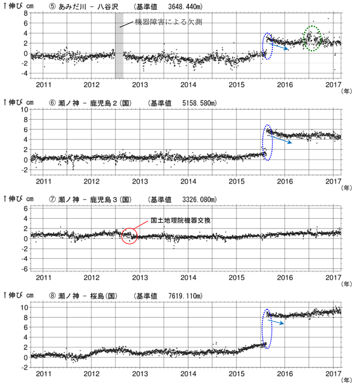
図 11-2 桜島 GNSS 連続観測による基線長変化 (2010 年 10 月～2017 年 2 月)
