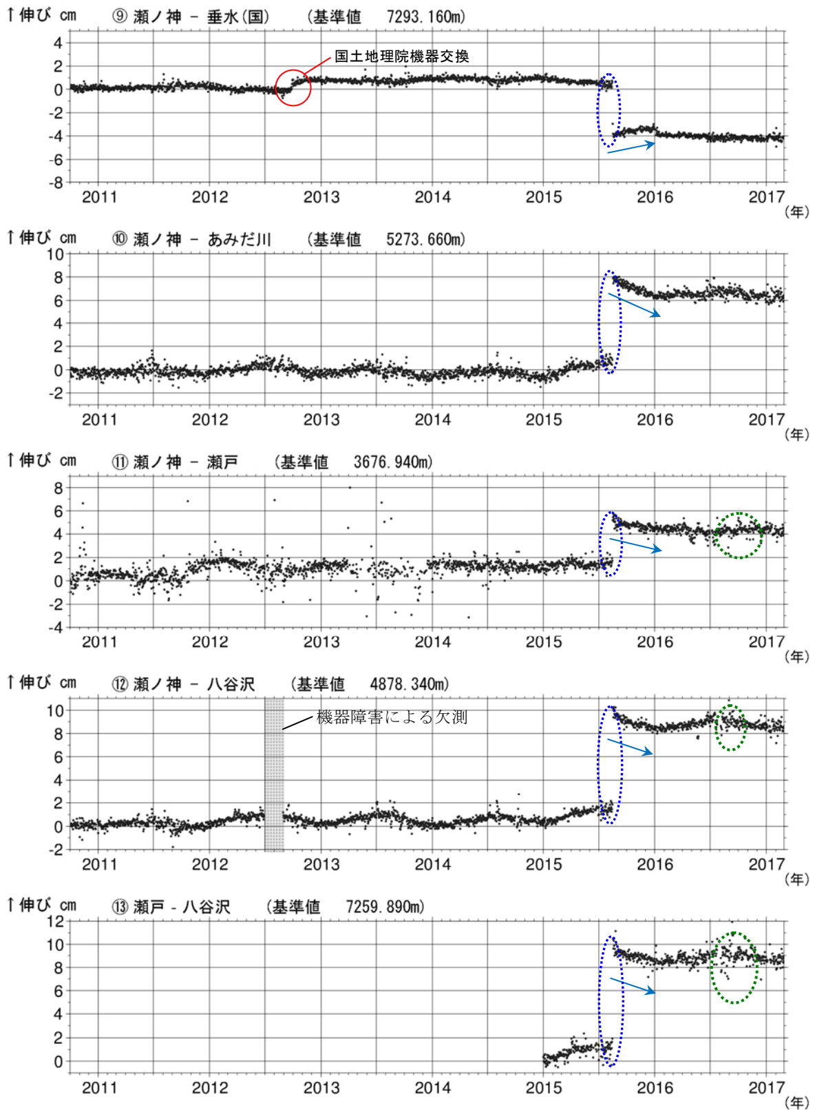
図 11-3 桜島 GNSS 連続観測による基線長変化（2010 年 10 月～2017 年 2 月）
