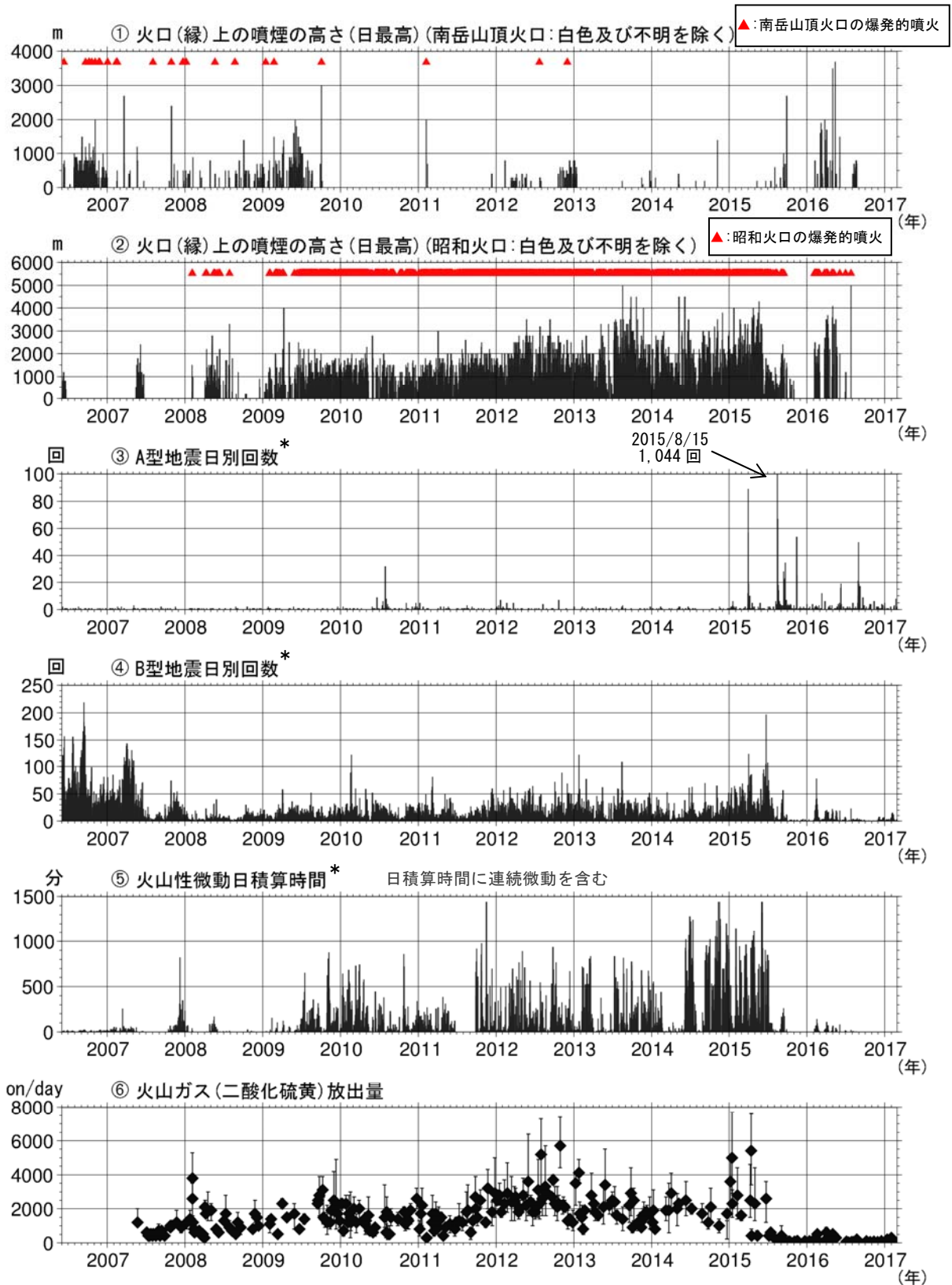
図8 桜島 昭和火口噴火活動再開(2006年6月)以降の活動経過図(2006年6月~2017年2月)
