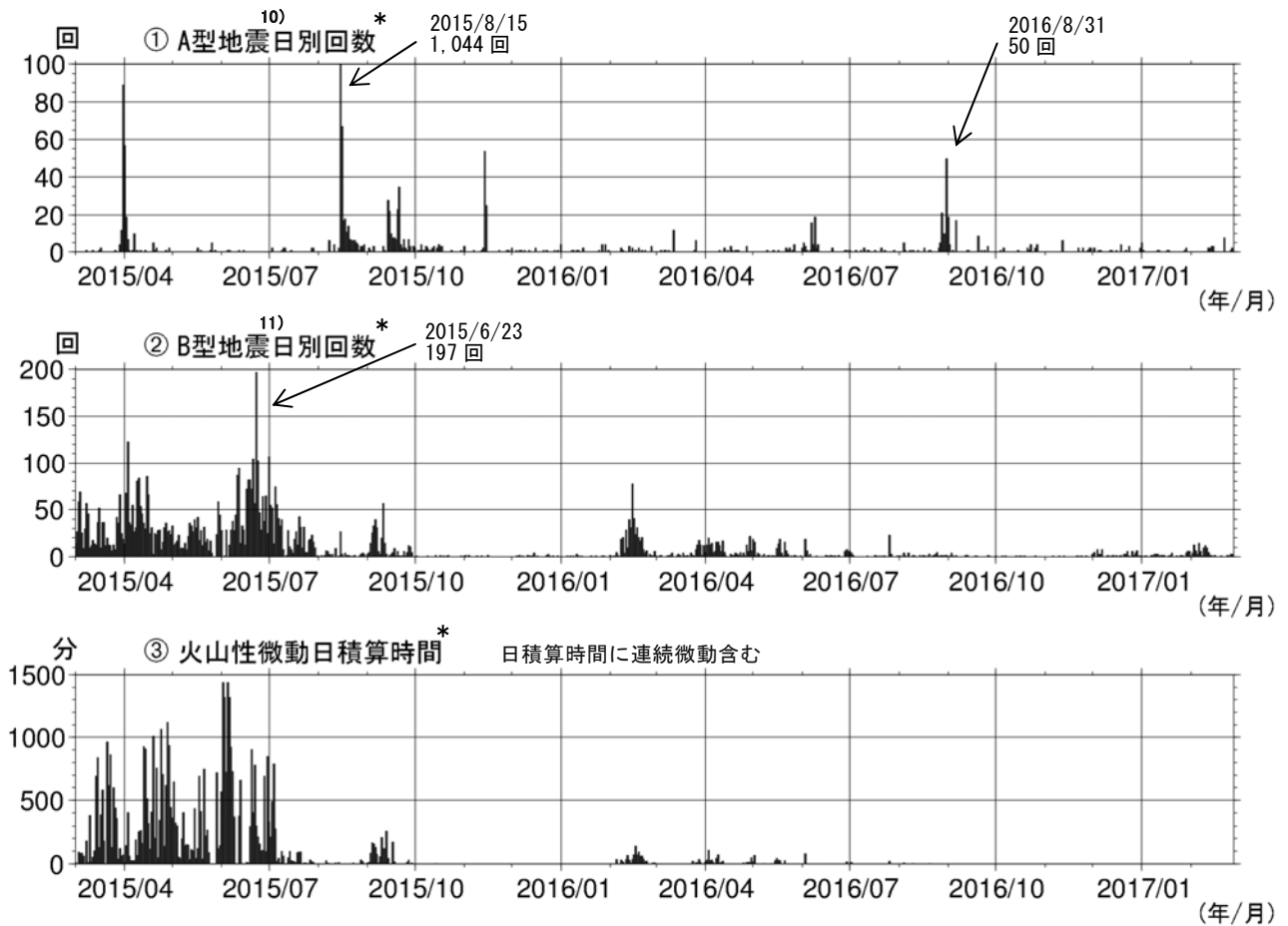
図6 桜島 最近2年間の活動経過図（2015年3月～2017年2月）
