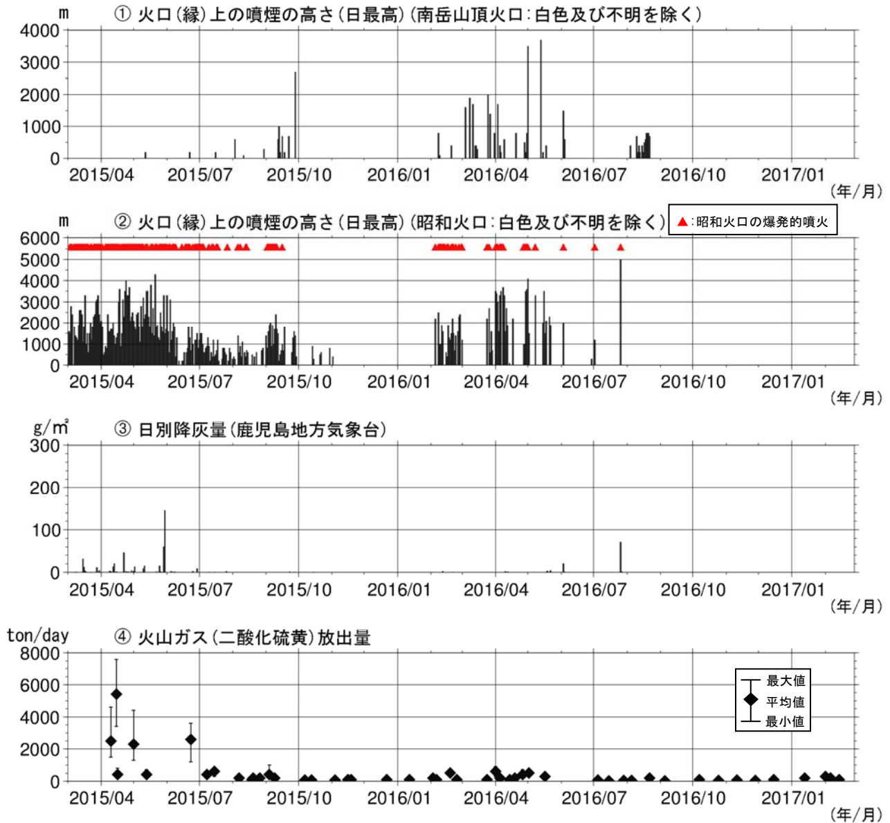
図7 桜島 最近2年間の活動経過図（2015年3月～2017年2月）
