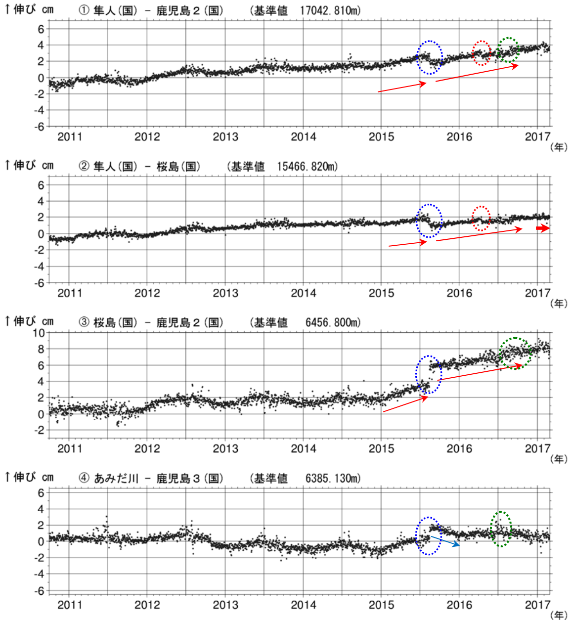
図 11-1 桜島 GNSS 連続観測による基線長変化（2010 年 10 月～2017 年 2 月）
