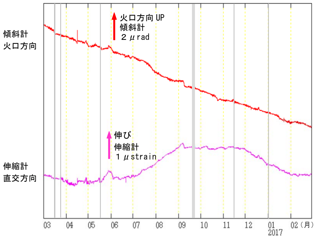
図 10 桜島 有村観測坑道の傾斜計及び伸縮計の変化（2016 年 3 月 1 日～2017 年 2 月 28 日）
