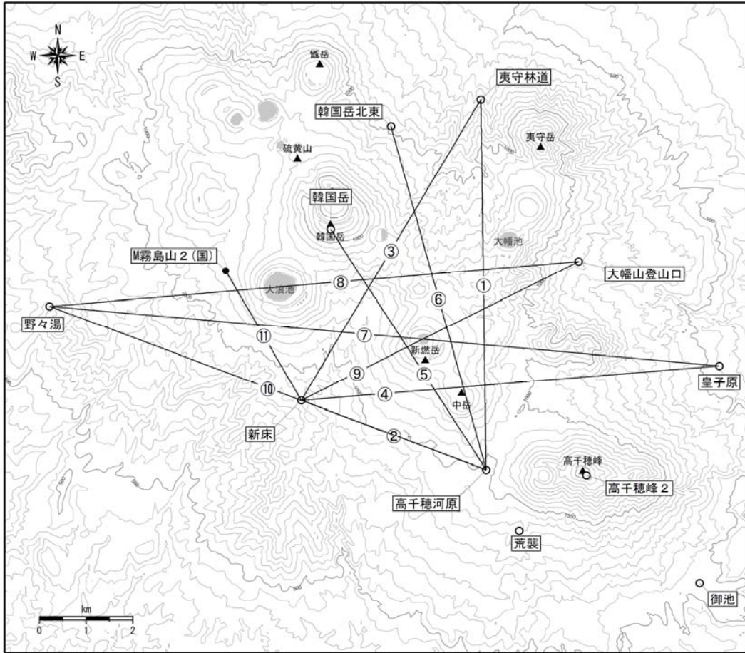
図 16 霧島山（新燃岳） GNSS 連続観測点と基線番号
