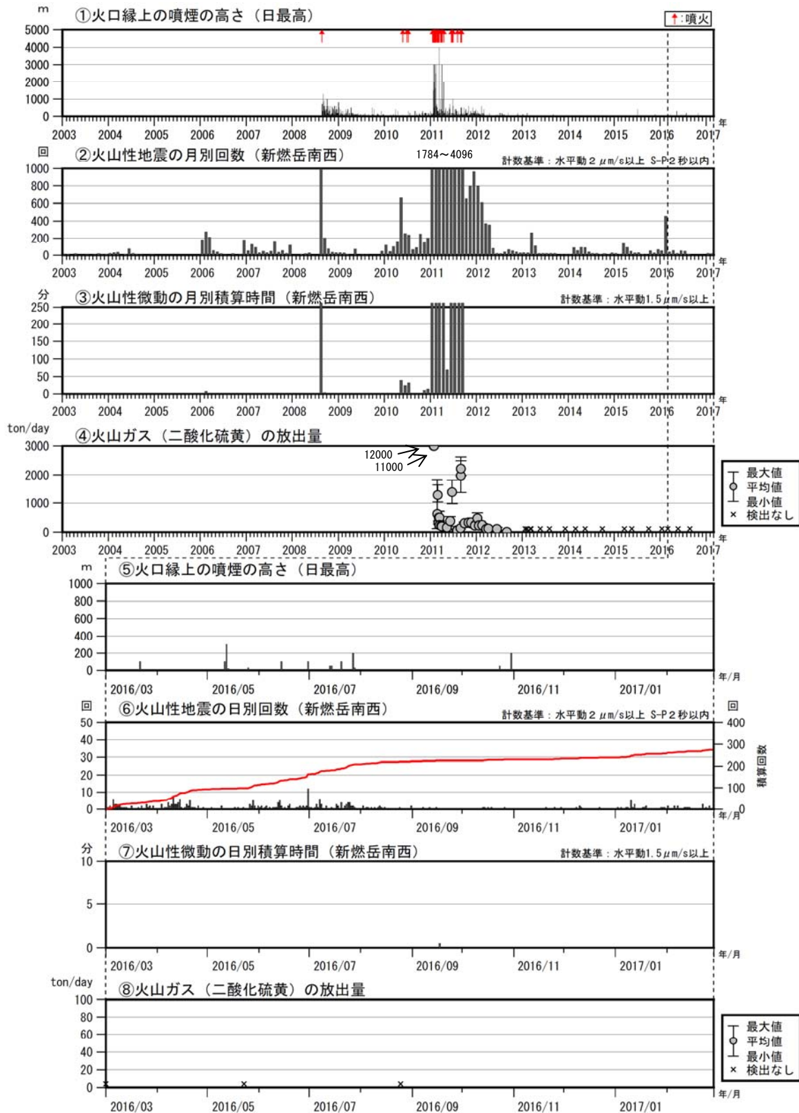
図 12 霧島山（新燃岳） 火山活動経過図（2003 年 1 月～2017 年 2 月）
