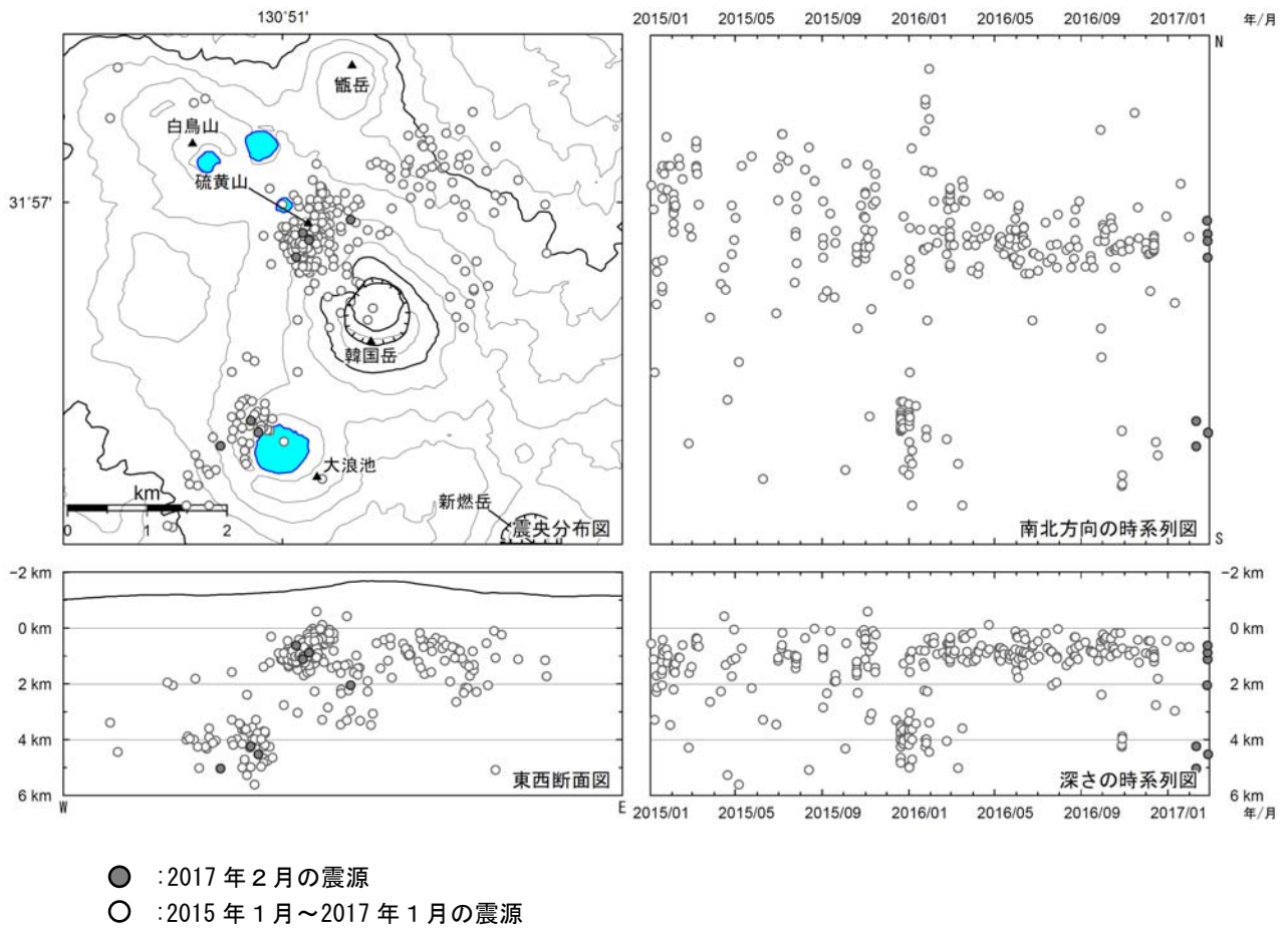
図3 霧島山（えびの高原（硫黄山）周辺） 震源分布図（2015年1月～2017年2月）
