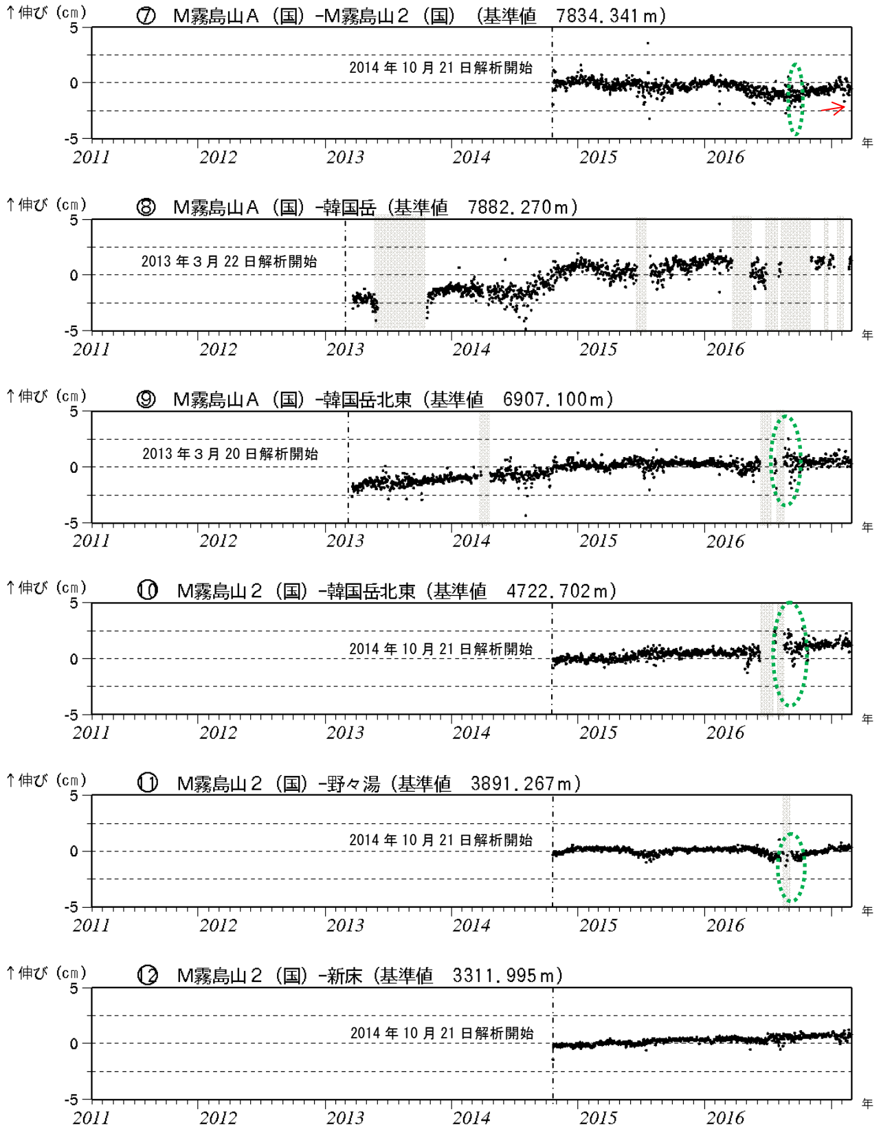
図 4-2 霧島山（えびの高原（硫黄山）周辺） GNSS 連続観測による基線長変化 （2011 年 4 月～2017 年 2 月）
