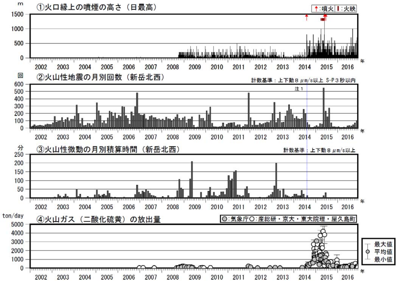
図3 口永良部島 火山活動経過図（2002年1月～2016年11月）
