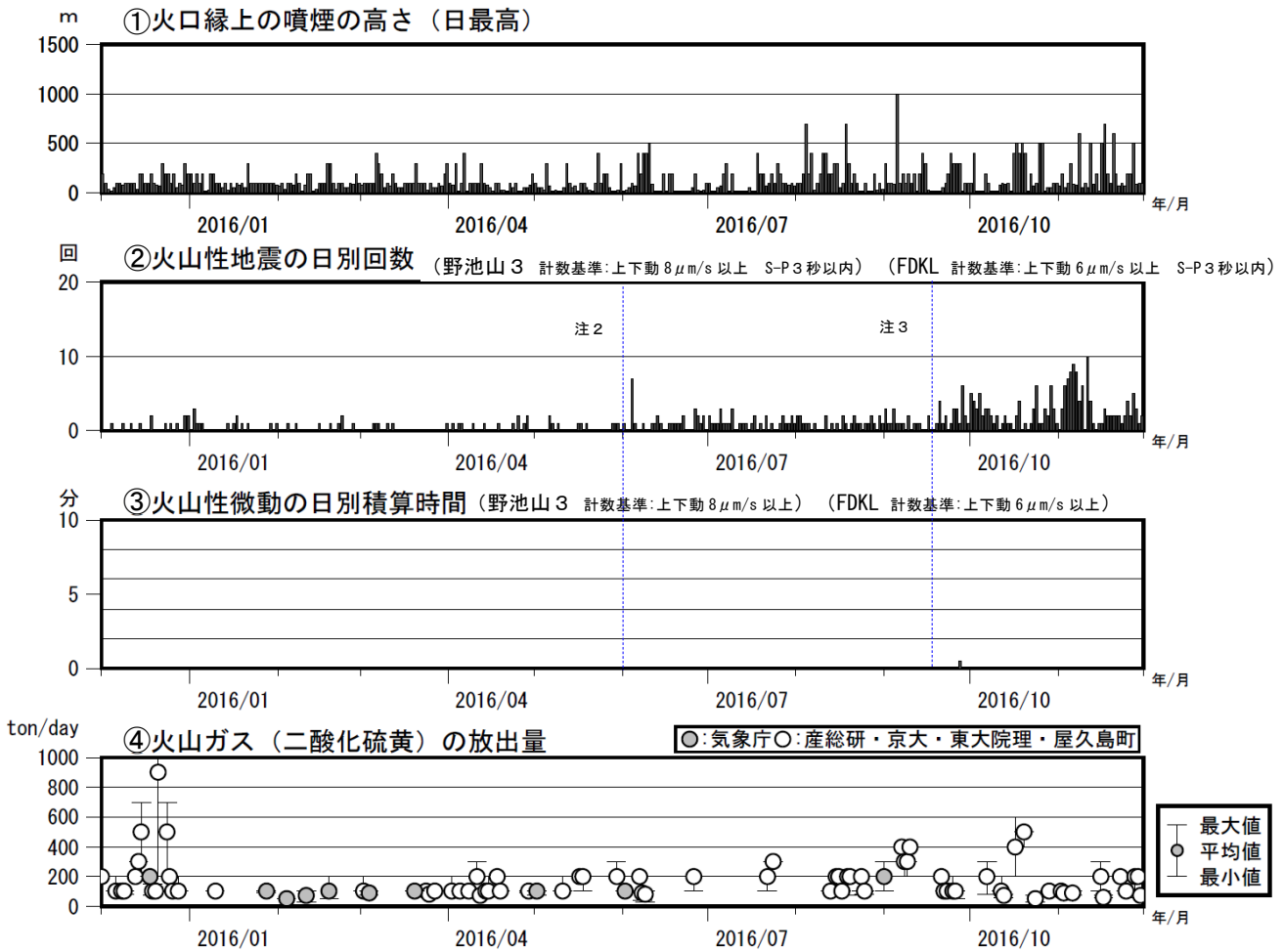
図4 口永良部島 最近の火山活動経過図（2015年12月～2016年11月）
