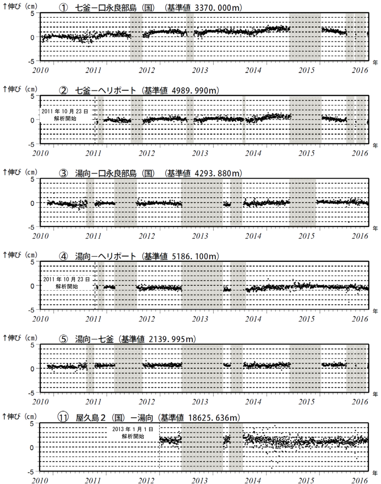
図6 口永良部島 GNSS 連続観測による基線長変化（2010年10月～2016年11月）
