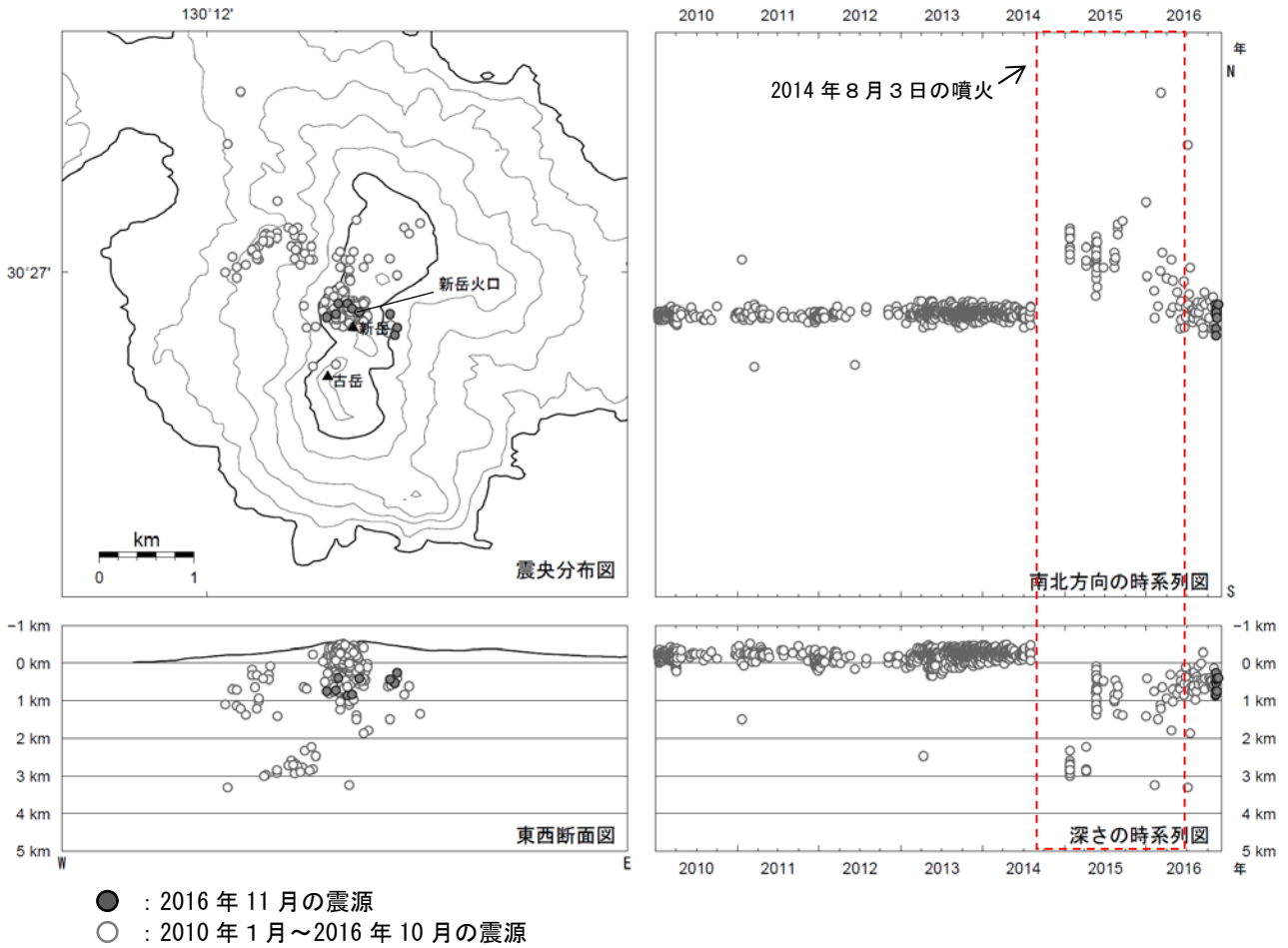
図5 口永良部島 震源分布図（2010年1月～2016年11月）
