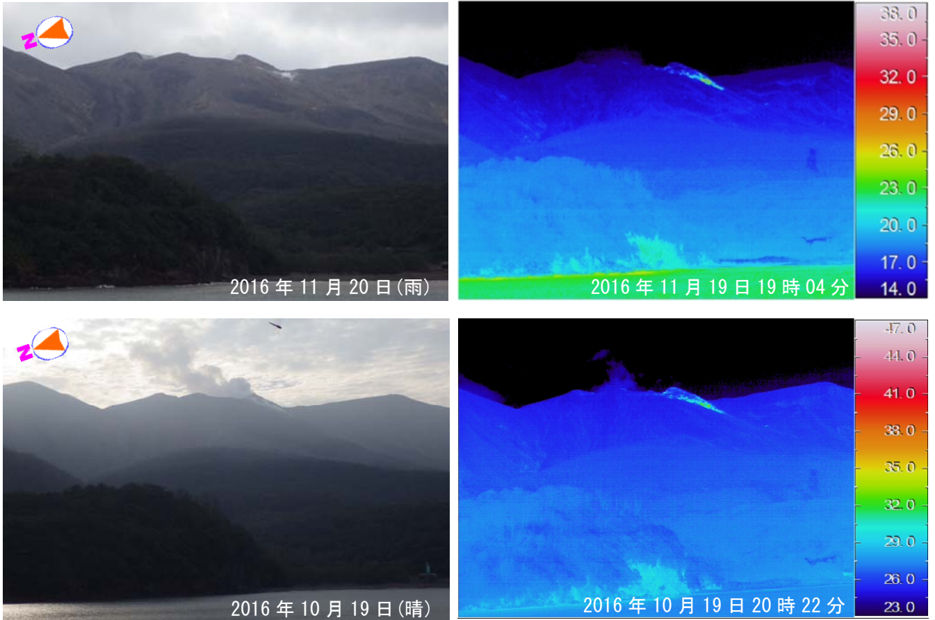
本村から撮影した可視画像と地表面温度分布
