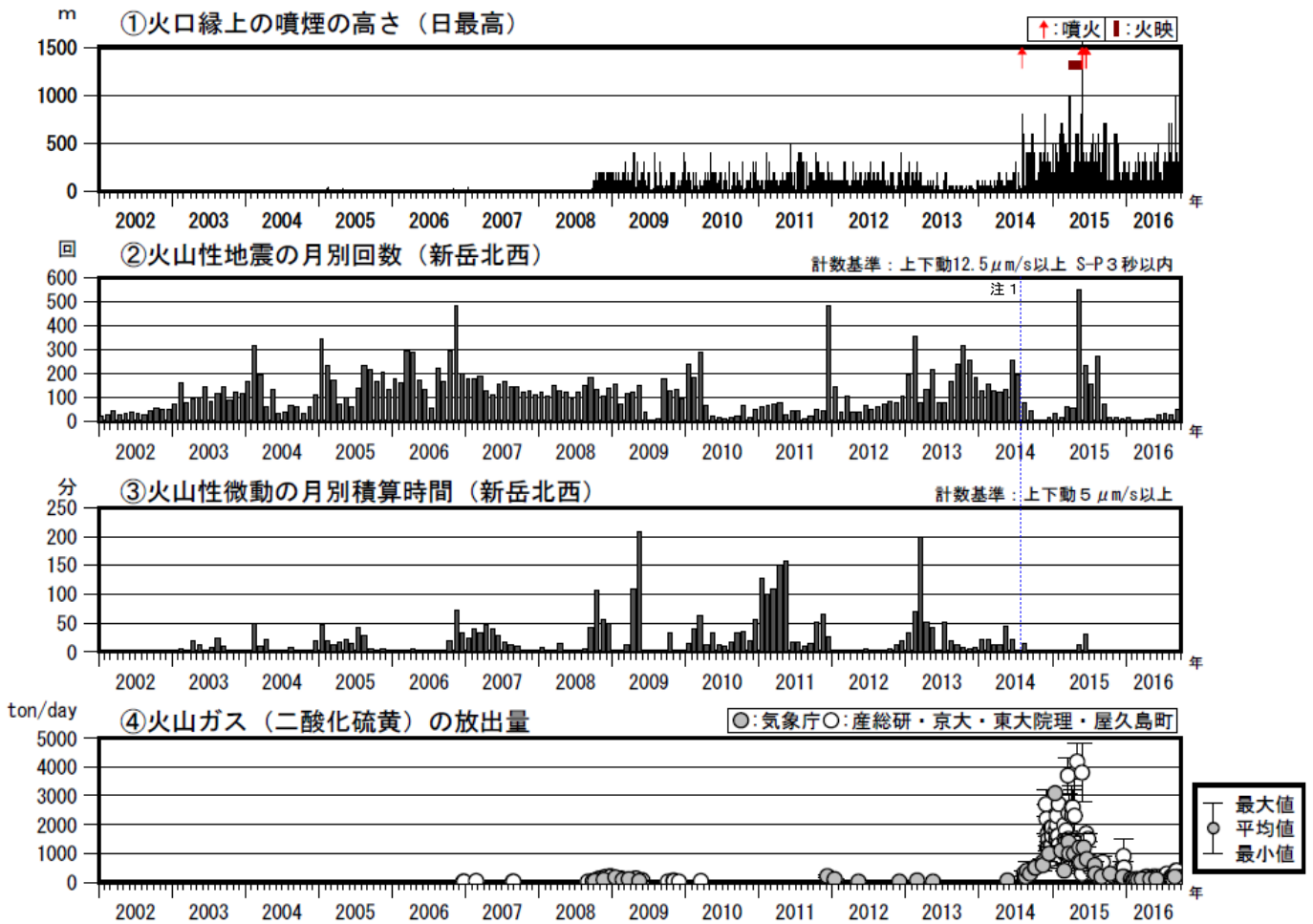
図3 口永良部島 火山活動経過図（2002年1月～2016年9月）
