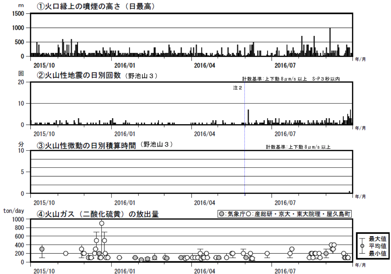
図4 口永良部島 最近の火山活動経過図（2015年10月～2016年9月）
