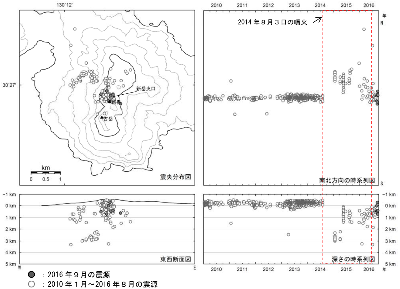
図 5 口永良部島 震源分布図（2010 年 1 月～2016 年 9 月）
