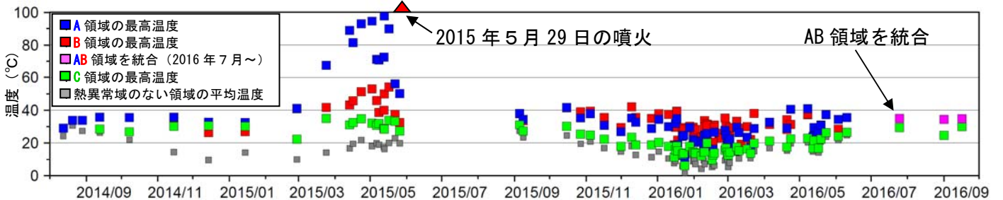
図2 口永良部島 新岳西斜面の地表面温度分布と熱異常域の温度時系列 （2014年8月～2016年9月：本村から新岳の北西側を撮影）
