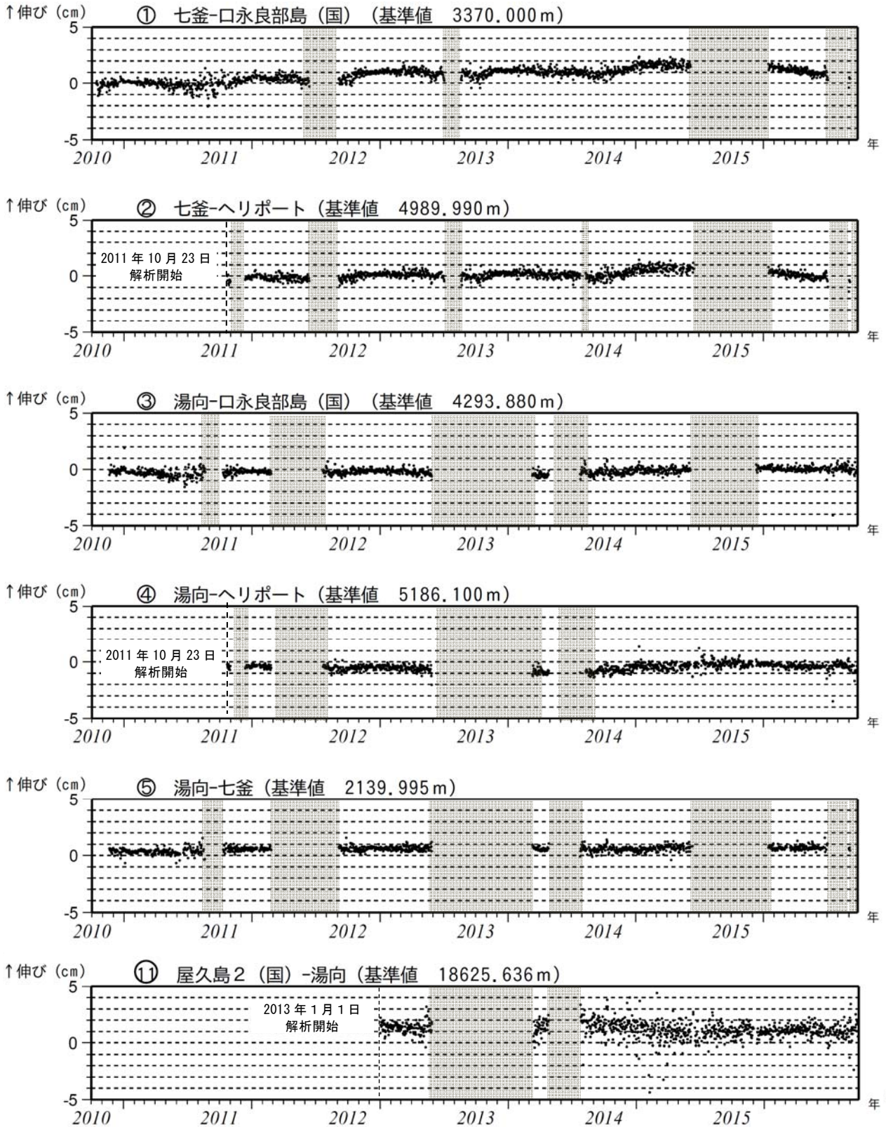
図6 口永良部島 GNSS 連続観測による基線長変化（2010年10月～2016年9月）
