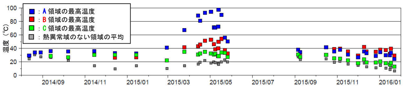
図2 口永良部島 新岳西斜面の地表面温度分布と熱異常域の温度時系列 （本村から新岳の北西側を撮影、2014年8月～2016年1月）
