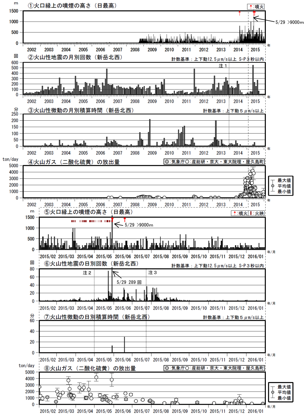
図3 口永良部島 火山活動経過図（2002年1月～2016年1月）
