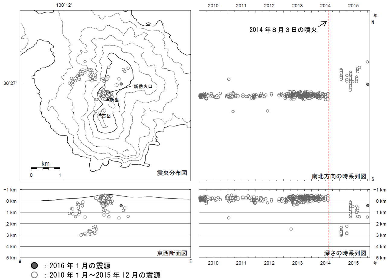
図 4 口永良部島 震源分布図（2010 年 1 月～2016 年 1 月）
