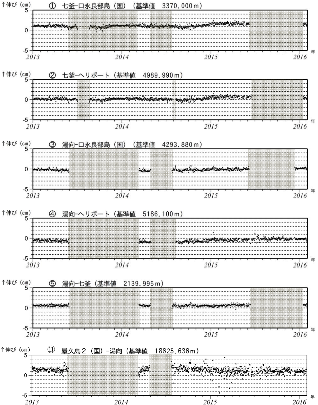
図5 口永良部島 GNSS 連続観測による基線長変化（2013 年 1 月～2016 年 1 月）
