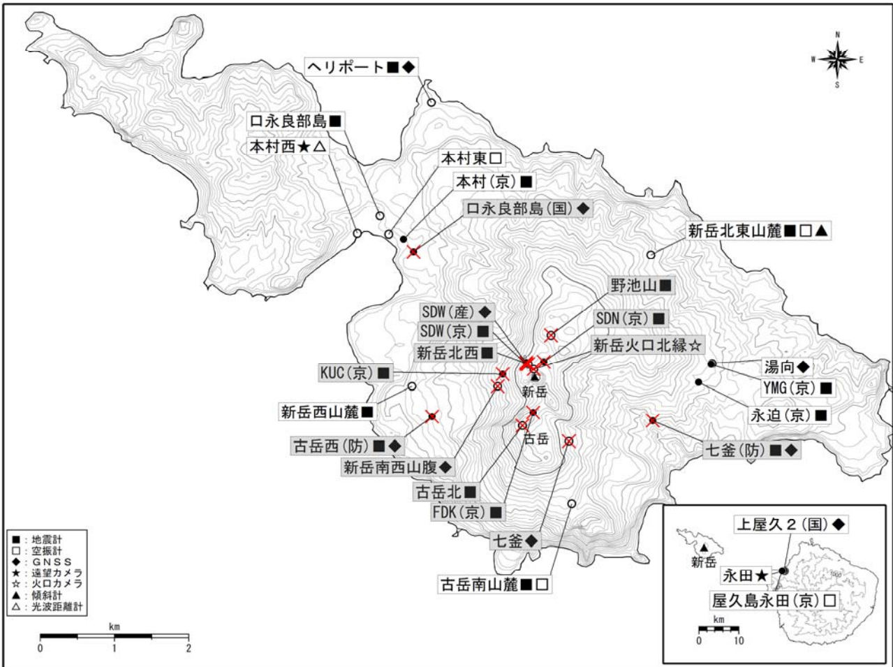
図 11 口永良部島 観測点配置図
