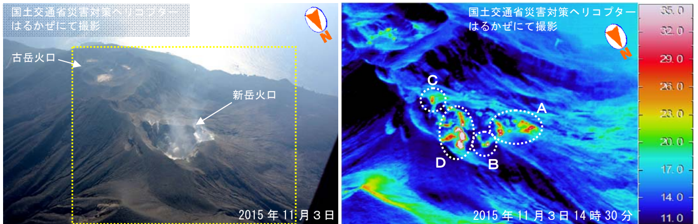
図4 口永良部島 新岳及び古岳の火口内とその周辺の状況（2015年11月3日撮影） （黄色破線は右の熱画像の範囲を示しています）
