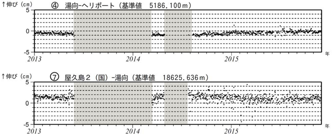
図 8 口永良部島 GNSS 連続観測による基線長変化（2013 年 1 月～2015 年 11 月）
