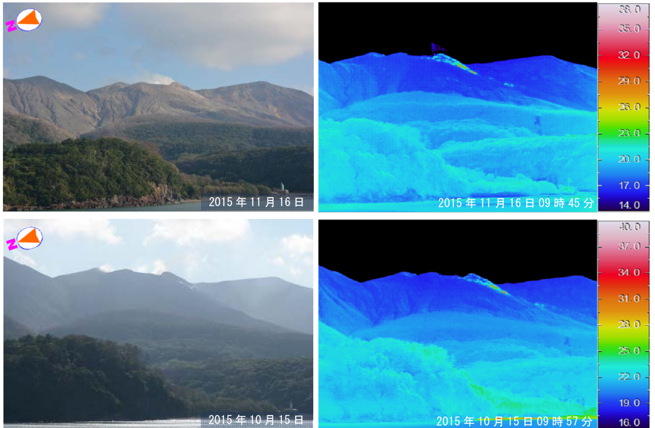
本村から撮影した可視画像と地表面温度分布（上図：2015年11月16日、下図：2015年10月15日）
