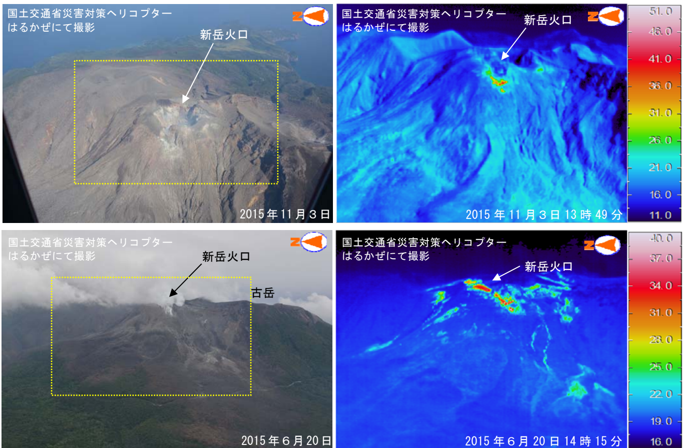
図 3 口永良部島 新岳火口及び西側斜面の状況（上：2015 年 11 月 3 日、下：2015 年 6 月 20 日撮影） （黄色破線は右の熱画像の範囲を示しています）
