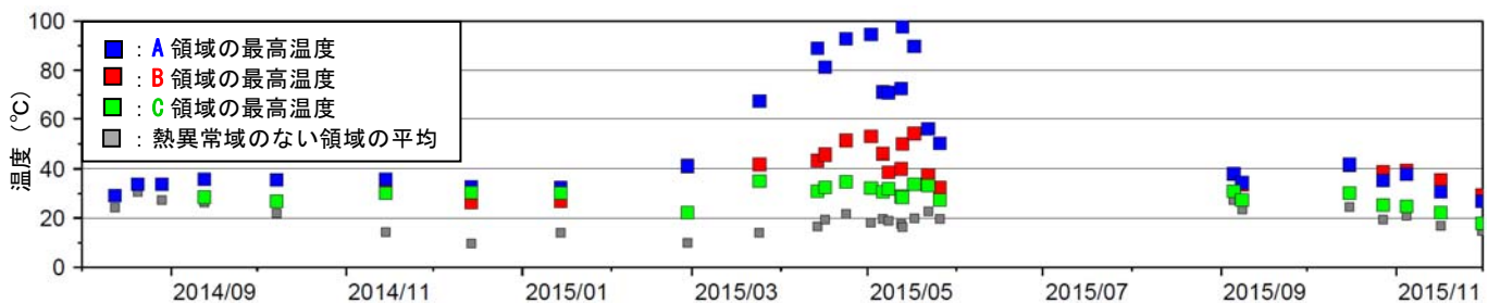
図6 口永良部島 新岳西斜面の地表面温度分布と熱異常域の温度時系列 （本村から新岳の北西側を撮影）
