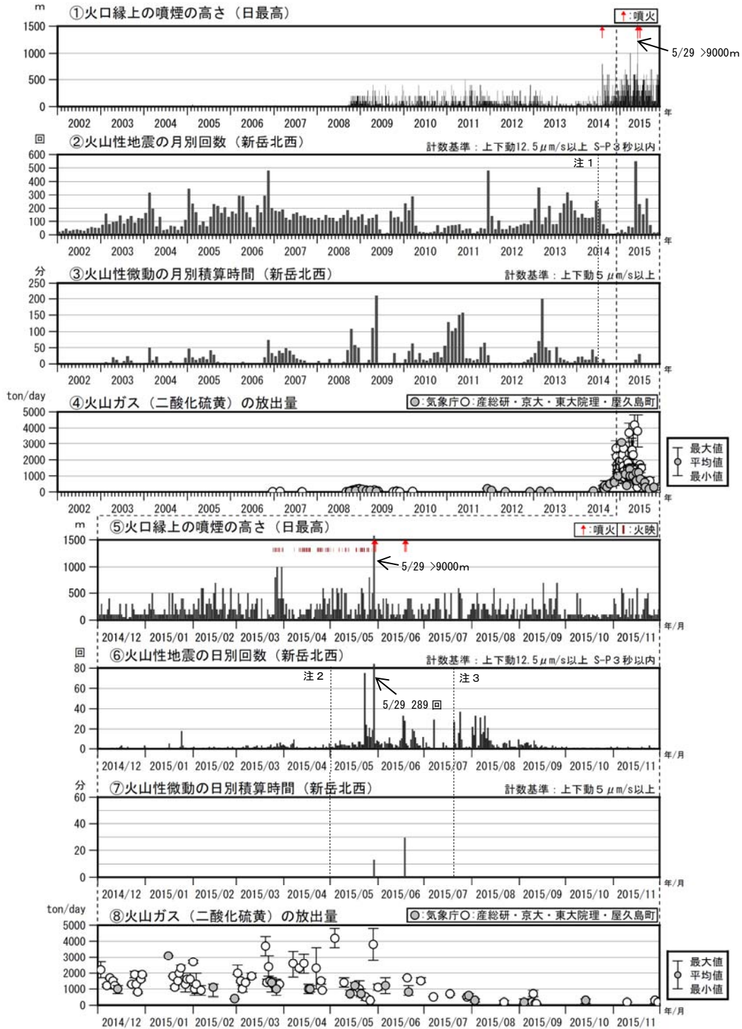
図 7 口永良部島 火山活動経過図（2002 年 1 月～2015 年 11 月）
