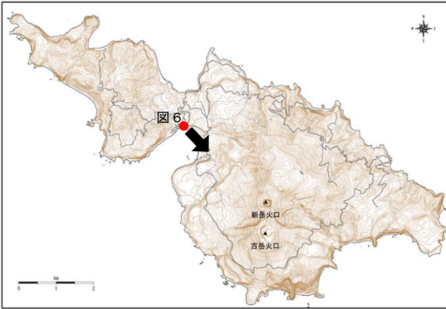
図 10 口永良部島 図 6 の撮影位置図
