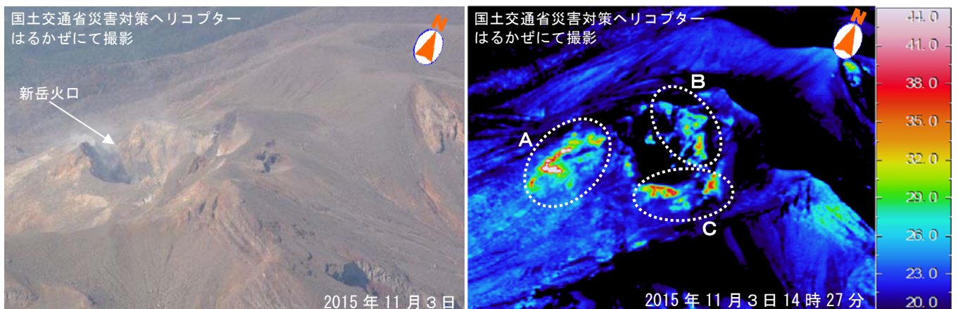
図5 口永良部島 新岳火口内とその周辺の状況（2015年11月3日撮影）
