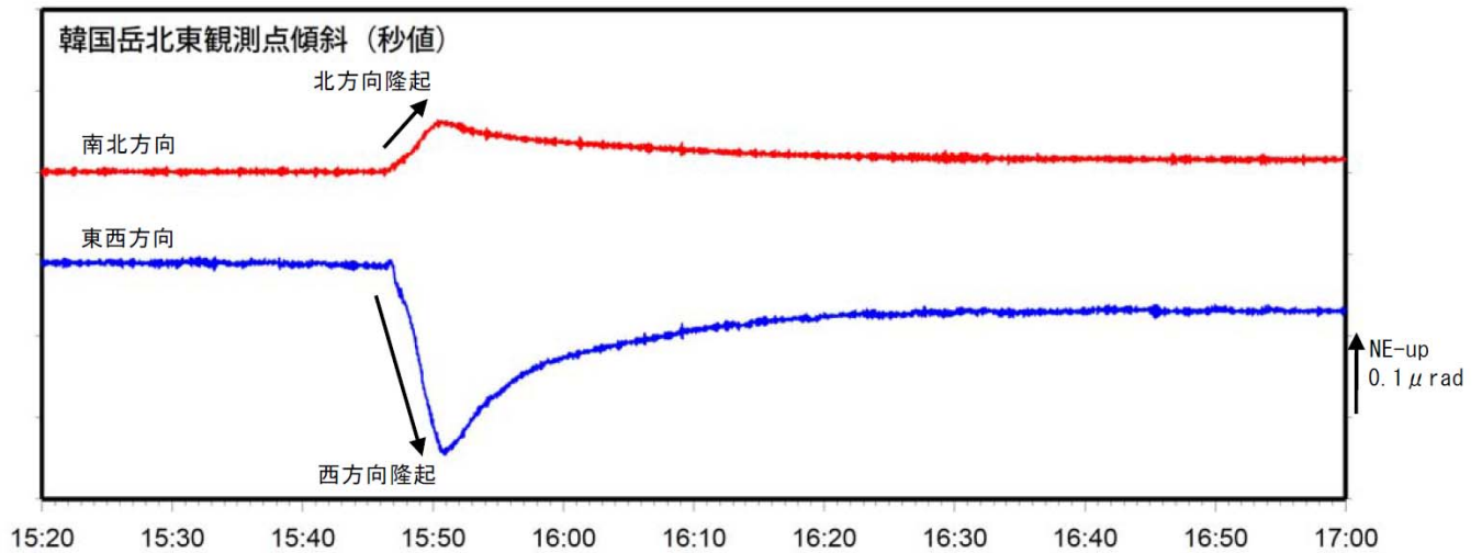
図 15-2 霧島山（えびの高原（硫黄山）周辺） 火山性微動に伴う傾斜変動 （10月19日15時20分～17時00分：韓国岳北東観測点、秒値） 火山性微動の発生に伴い、硫黄山の北西方向がわずかに隆起するような変動を観測しました。
