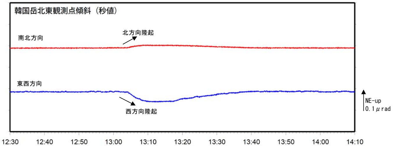
図 16-2 霧島山（えびの高原（硫黄山）周辺） 火山性微動に伴う傾斜変動 （10 月 31 日 12 時 30 分～14 時 10 分：韓国岳北東観測点、秒値） 火山性微動の発生に伴い、硫黄山の北西方向がわずかに隆起するような変動を観測しました。
