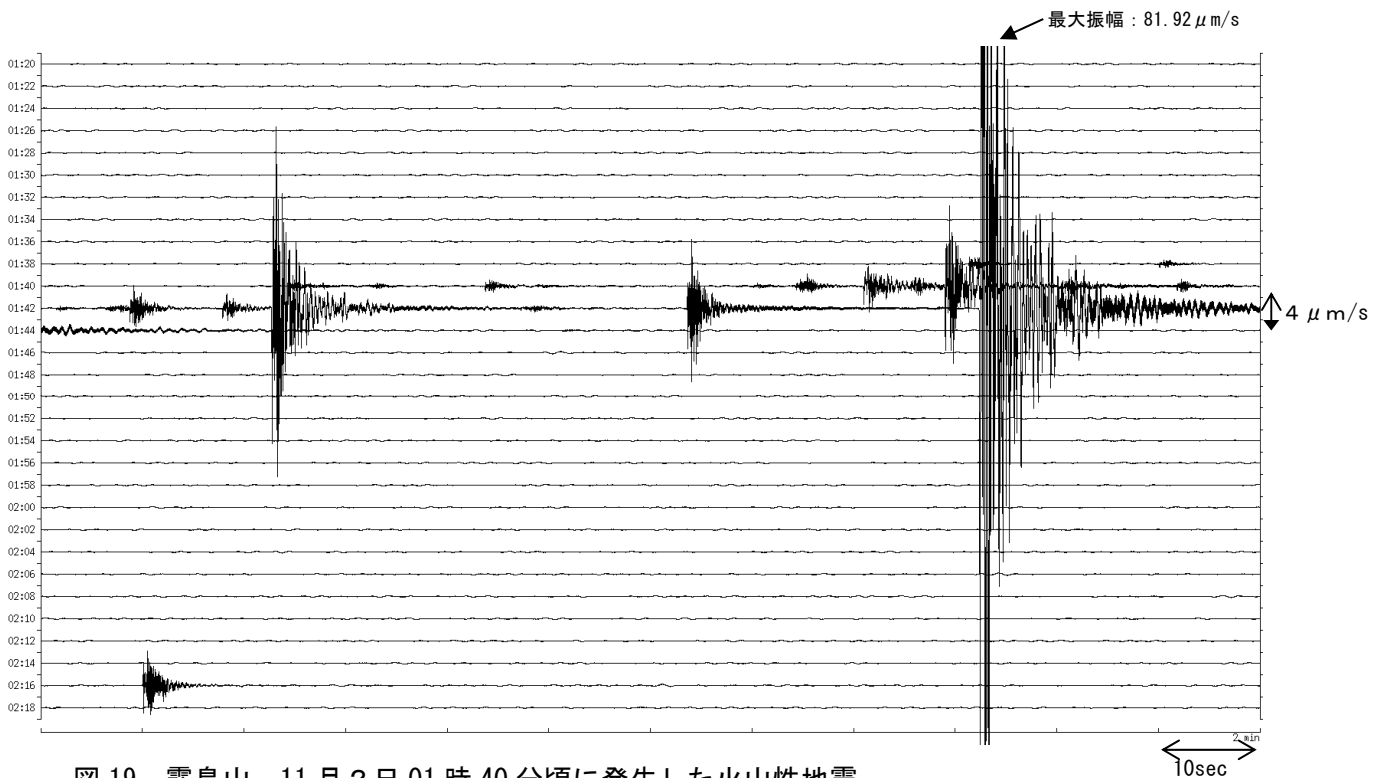
図 19 霧島山 11月2日01時40分頃に発生した火山性地震
