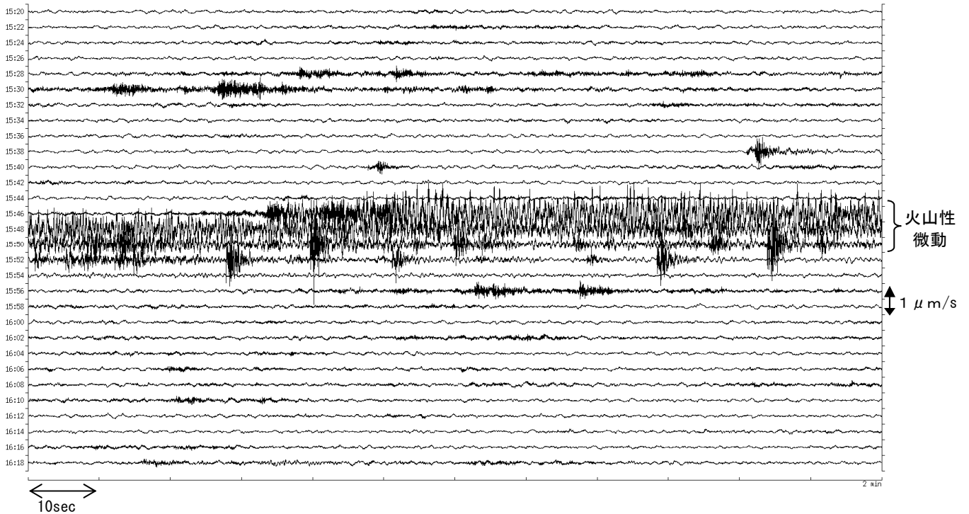
図 15-1 霧島山（えびの高原（硫黄山）周辺） 10月19日15時46分に発生した火山性微動 （10月19日15時30分～16時30分：韓国岳北東観測点） 火山性微動の継続時間は約3分30秒でした。
