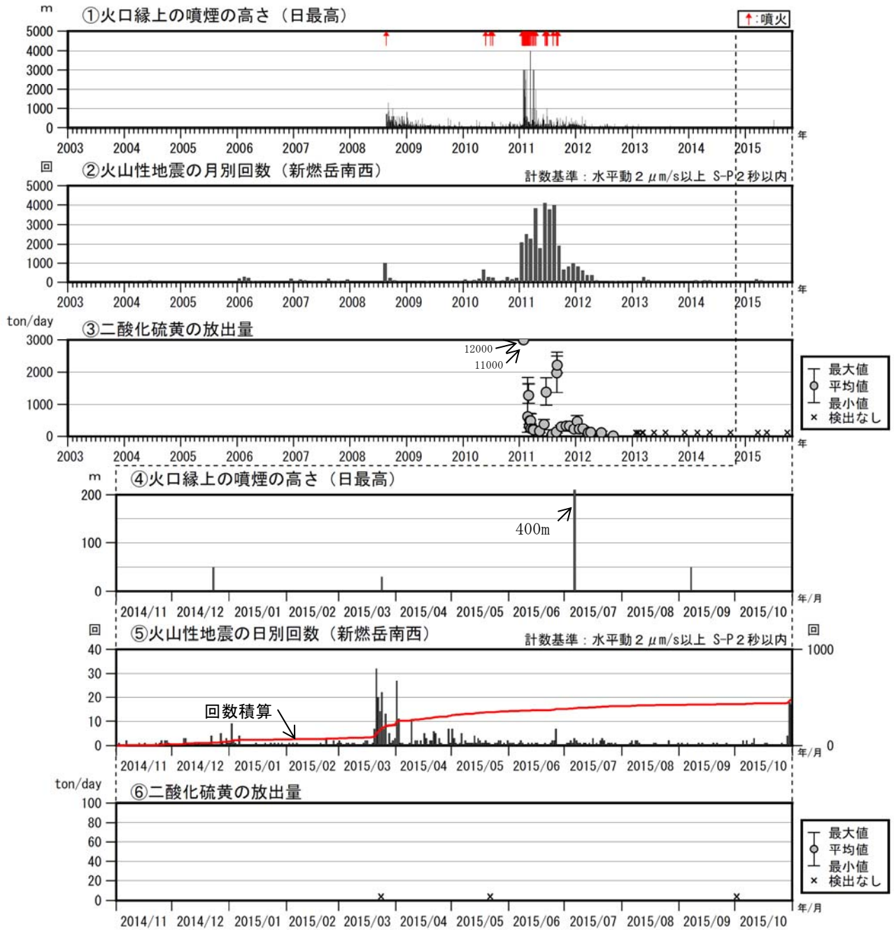
図3 霧島山（新燃岳） 火山活動経過図（2003年1月～2015年10月）
