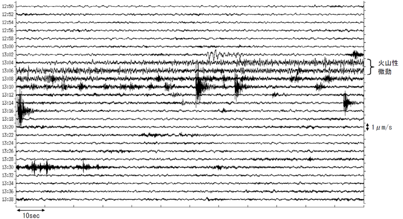
図 16-1 霧島山（えびの高原（硫黄山）周辺） 10 月 31 日 13 時 04 分頃に発生した火山性微動 （10 月 31 日 12 時 50 分～13 時 40 分：韓国岳北東観測点） 火山性微動の継続時間は約 2 分 30 秒でした。
