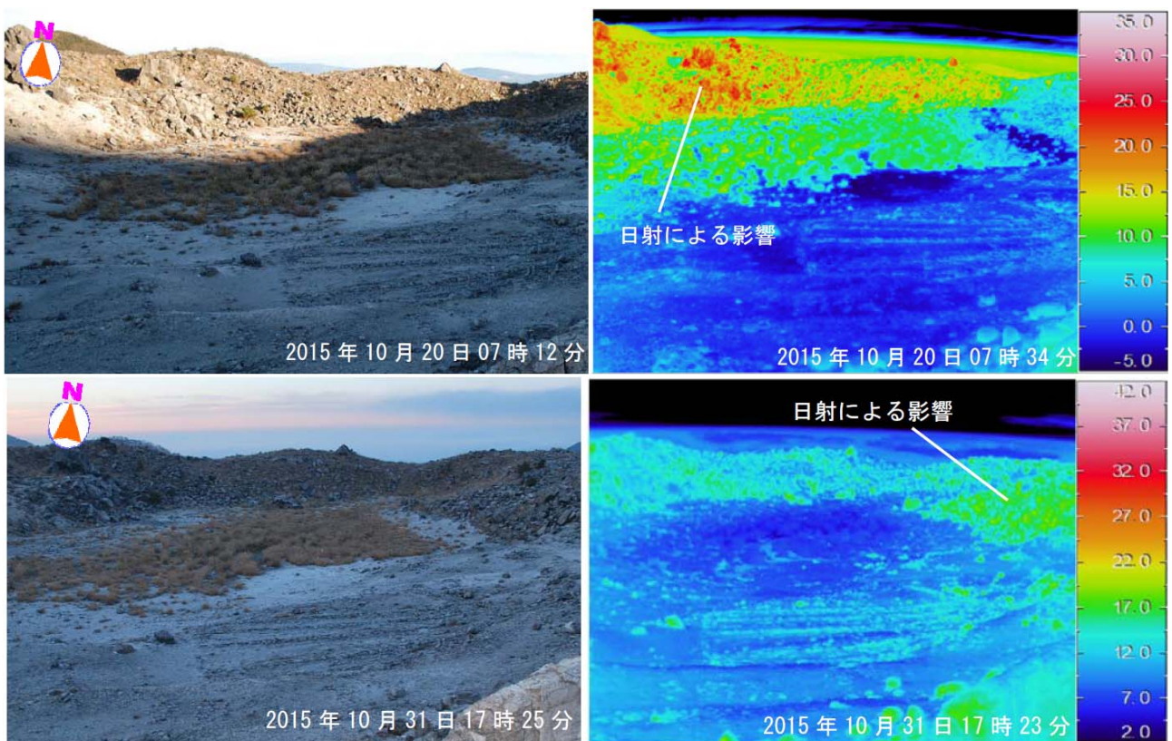
図 17-2 霧島山（えびの高原（硫黄山）周辺） 硫黄山火口内の状況（左：可視、右：地表面温度分布） 硫黄山周辺では噴気や熱異常域は認められませんでした。
