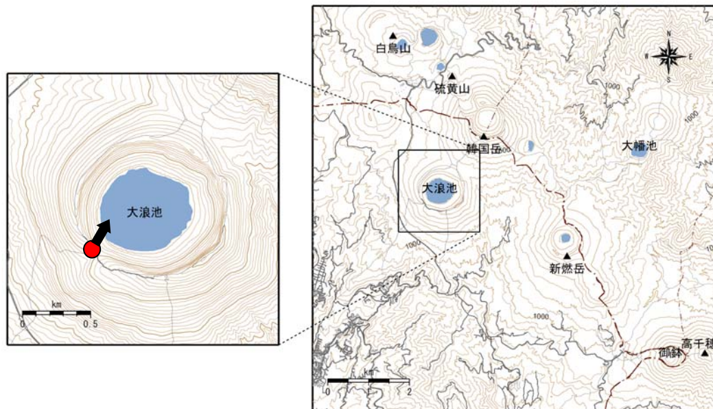
図 22 霧島山 図 21 の撮影位置
