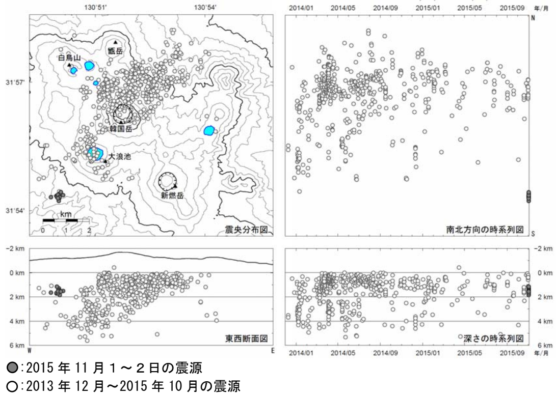
図 20 霧島山 11 月 2 日の震源分布図（2013 年 12 月 ~ 2015 年 11 月 2 日）
