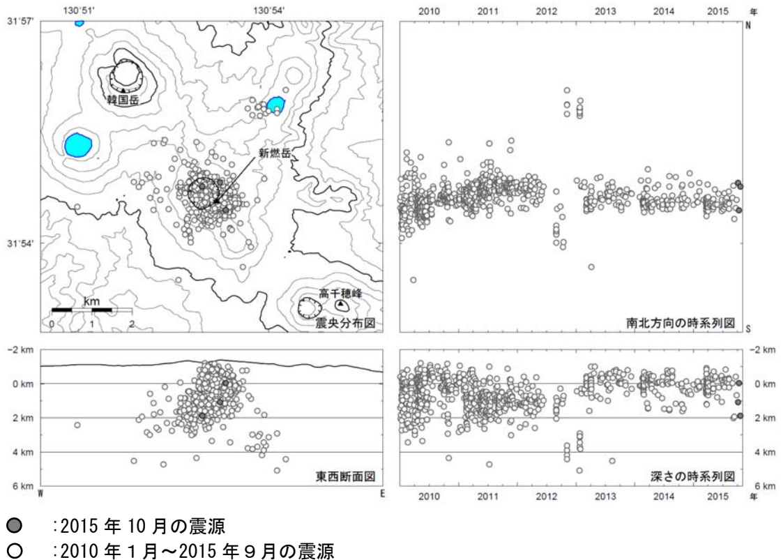
図2 霧島山（新燃岳） 震源分布図（2010年1月～2015年10月）
