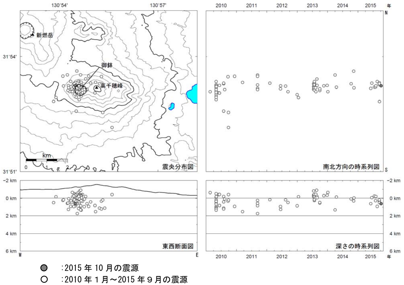
図 11 霧島山（御鉢） 震源分布図（2010 年 1 月～2015 年 10 月）
