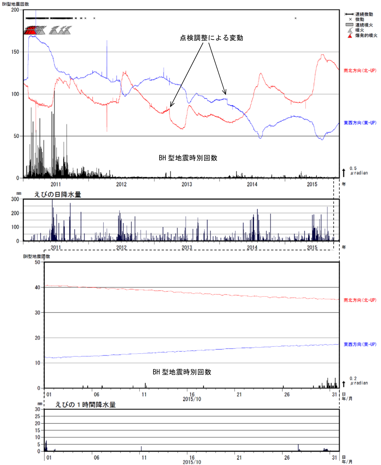
図4 霧島山（新燃岳） BH型地震の時間別回数と高千穂河原傾斜計の傾斜変動（2011年1月～2015年10月）
