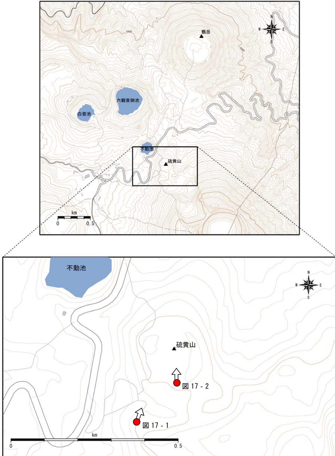
図 18 霧島山（えびの高原（硫黄山）周辺） 図 17 の撮影位置 （●は撮影位置、矢印は撮影方向を示す）
