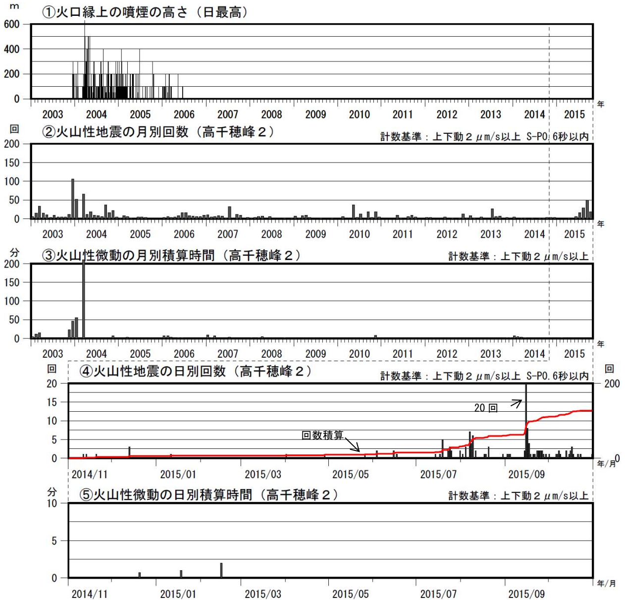
図 10 霧島山（御鉢） 火山活動経過図（2003 年 1 月～2015 年 10 月）
