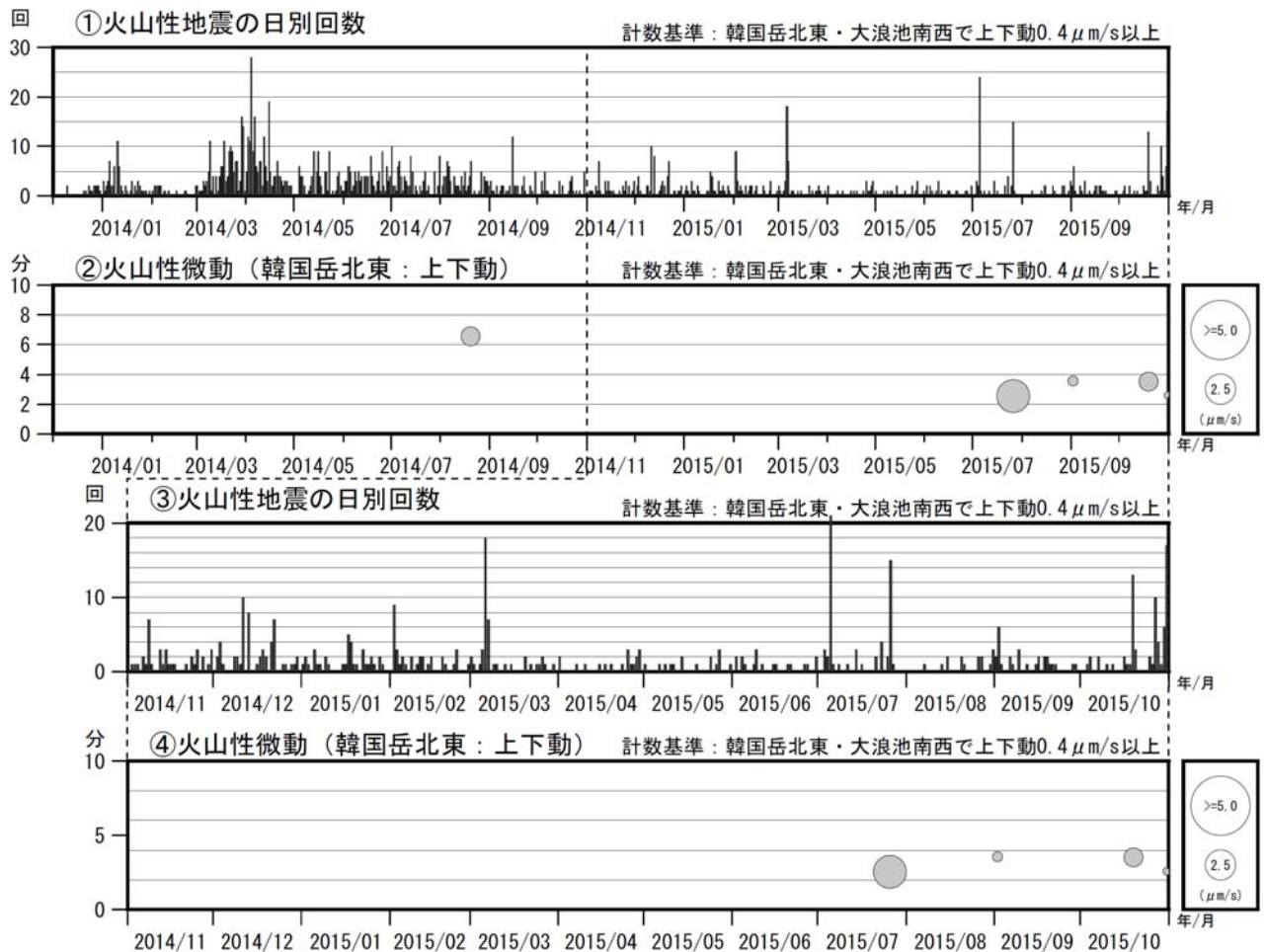
図 13 霧島山（えびの高原（硫黄山）周辺） 火山活動経過図（2013年12月～2015年10月）
