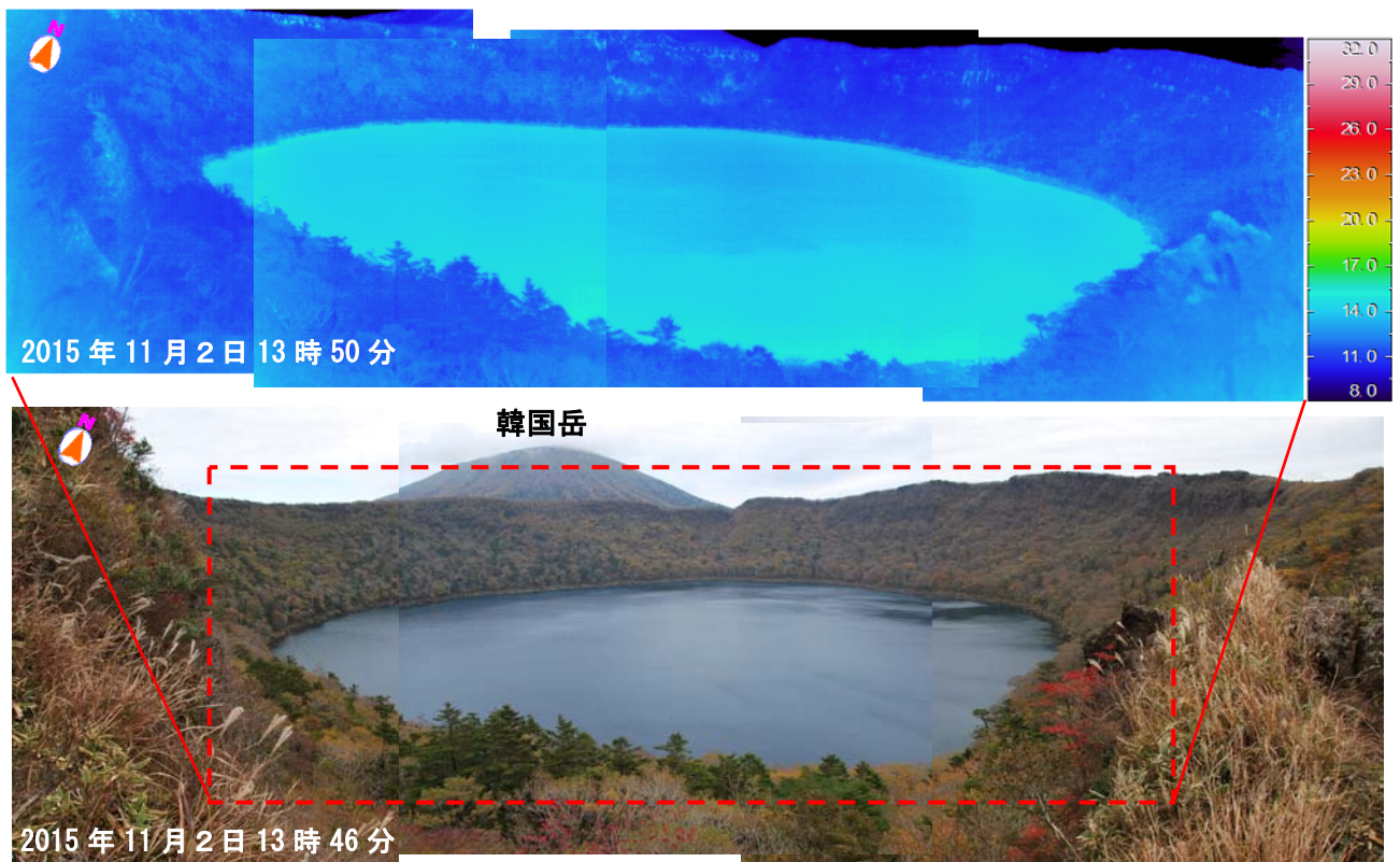
図 21 霧島山 南西側から見た大浪池の状況（2015 年 11 月 2 日） （上：地表面温度分布、下：可視画像）
