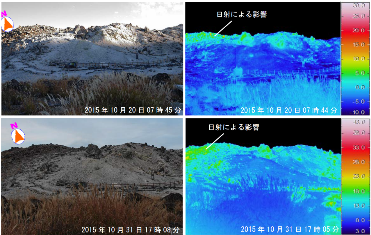
図 17-1 霧島山（えびの高原（硫黄山）周辺） 硫黄山南西側の状況（左：可視、右：地表面温度分布） 硫黄山周辺では噴気や熱異常域は認められませんでした。
