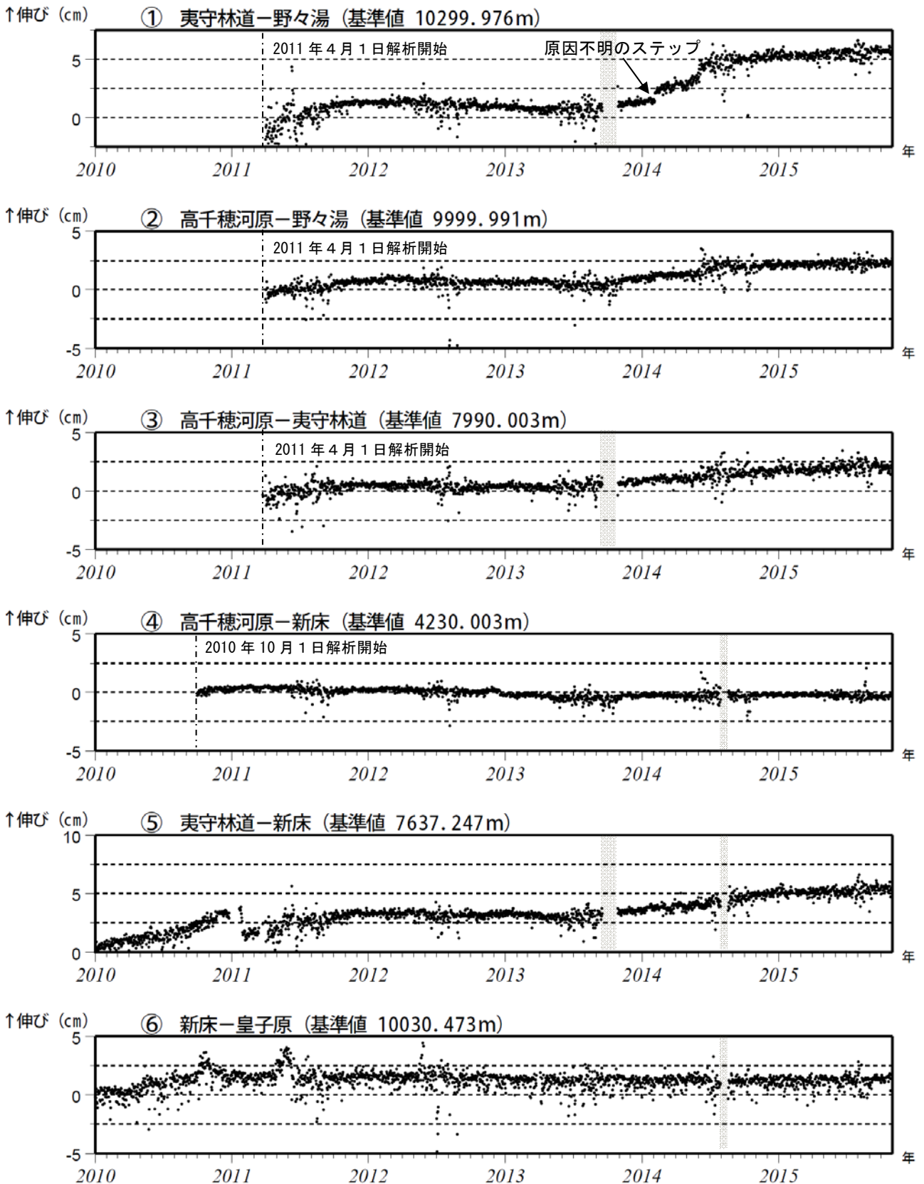
図 6-1 霧島山 GNSS 連続観測による基線長変化 (2010 年 1 月～2015 年 10 月)
