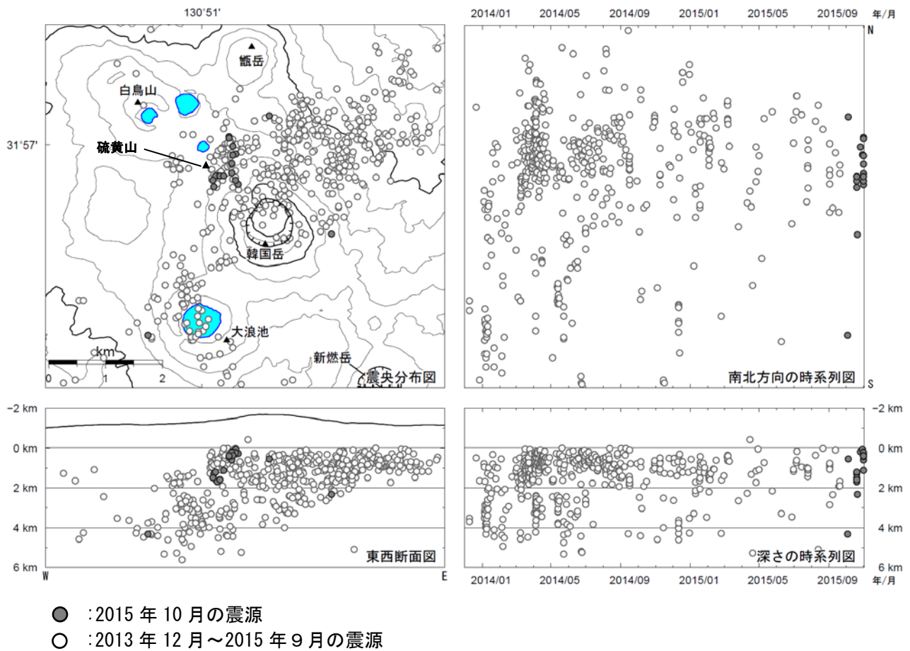
図 14 霧島山（えびの高原（硫黄山）周辺） 震源分布図（2013 年 12 月～2015 年 10 月）
