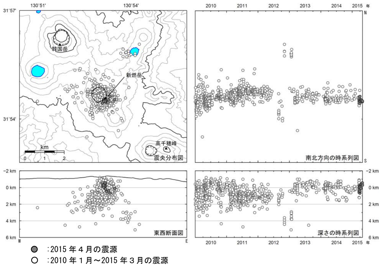
図 2 霧島山（新燃岳） 震源分布図（2010年1月～2015年4月）
