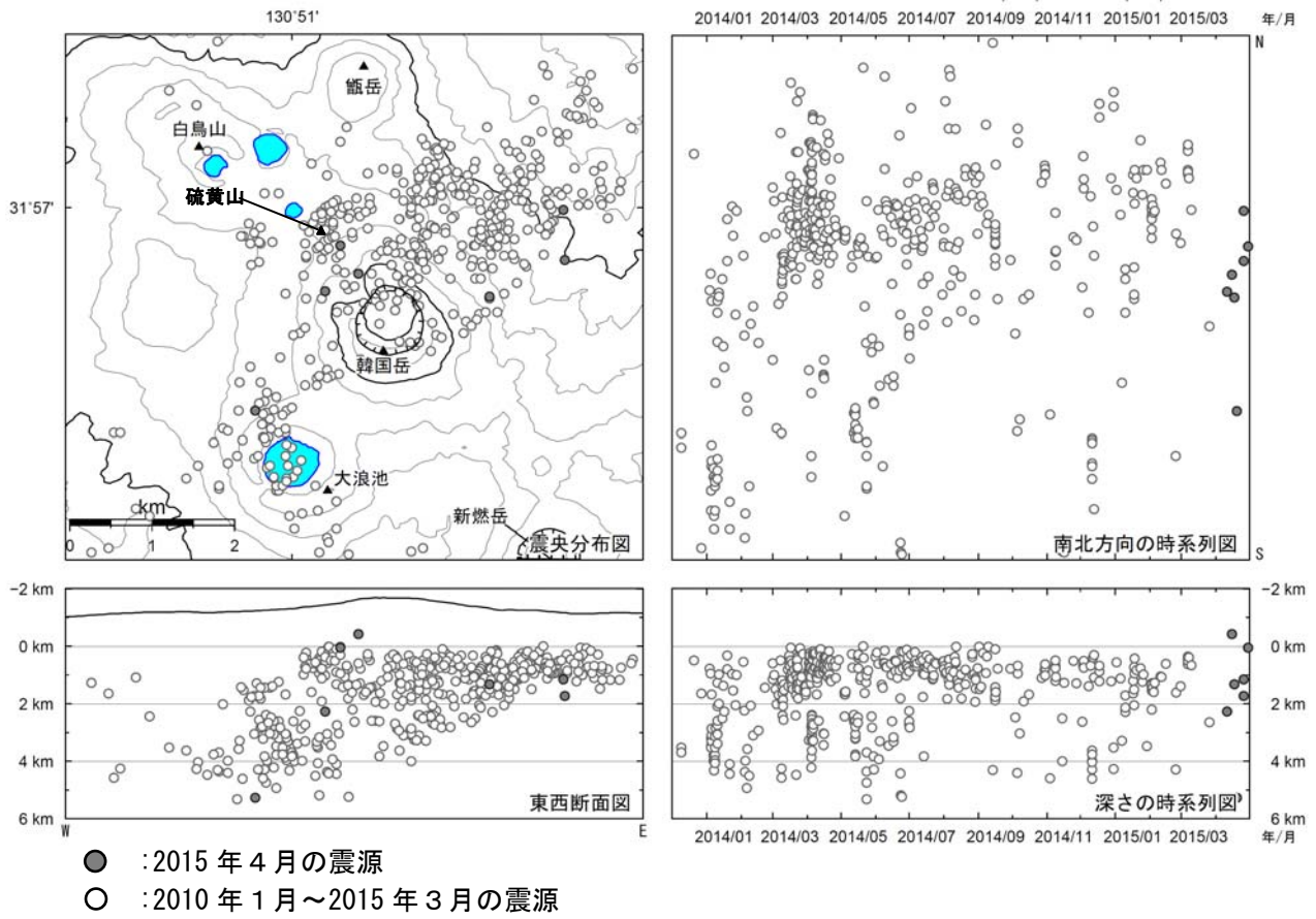
図 13 霧島山（えびの高原（硫黄山）周辺） 震源分布図（2013 年 12 月～2015 年 4 月）
