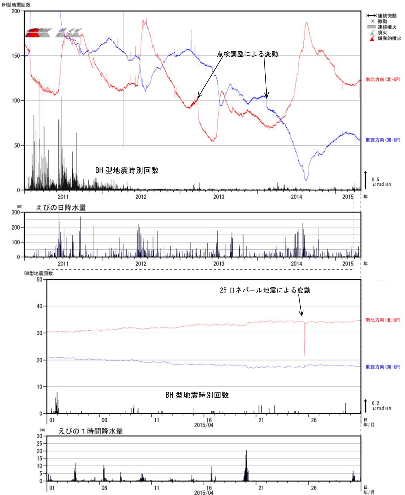
図4 霧島山（新燃岳） BH型地震の時間別回数と高千穂河原傾斜計の傾斜変動（2011年1月～2015年4月）
