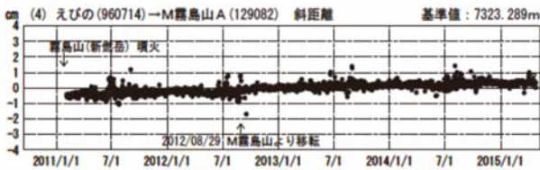
図5 霧島山（新燃岳） 国土地理院による広域的な地殻変動観測結果* (2010年10月1日～2015年4月26日)
