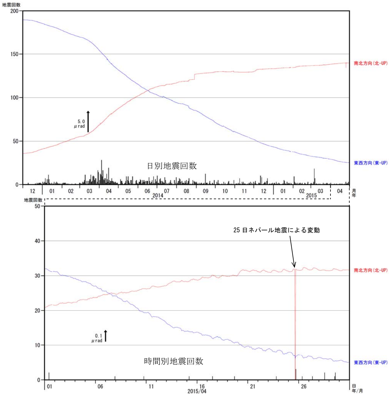
図 14 霧島山（えびの高原（硫黄山）周辺） 地震回数と韓国岳北東傾斜計の傾斜変動（時間値） （2013 年 12 月～2015 年 4 月）
