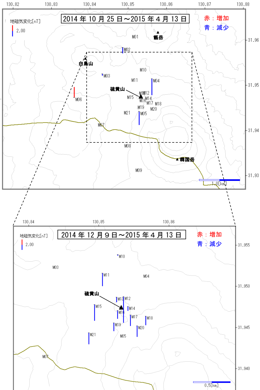
図 18 霧島山（えびの高原（硫黄山周辺）繰り返し観測による全磁力の変化 (上段：えびの高原周辺 2014 年 10 月 25 日～2015 年 4 月 13 日、 下段：硫黄山周辺 2014 年 12 月 9 日～2015 年 4 月 13 日)
