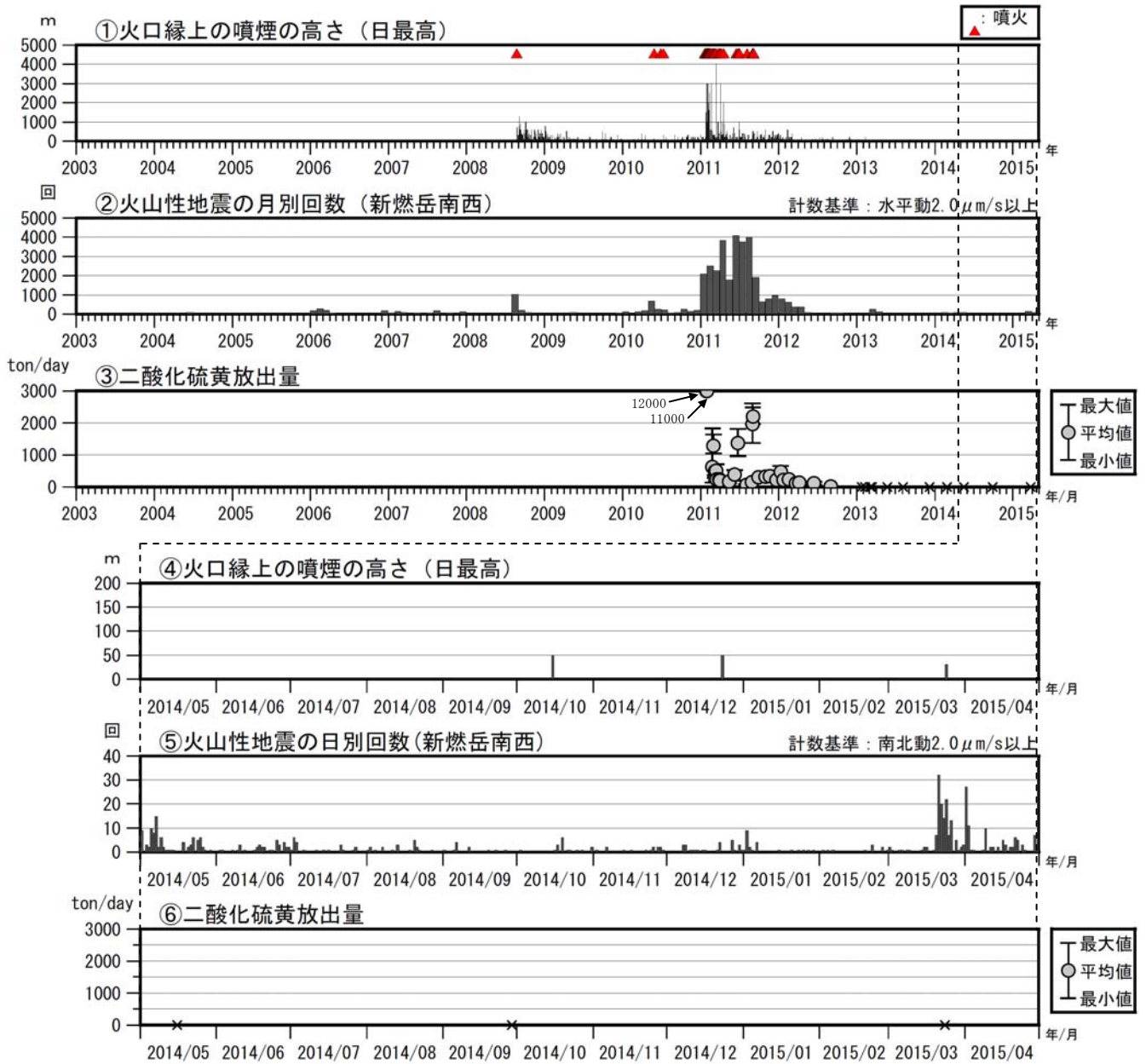
図3 霧島山（新燃岳） 火山活動経過図（2003年1月～2015年4月）
