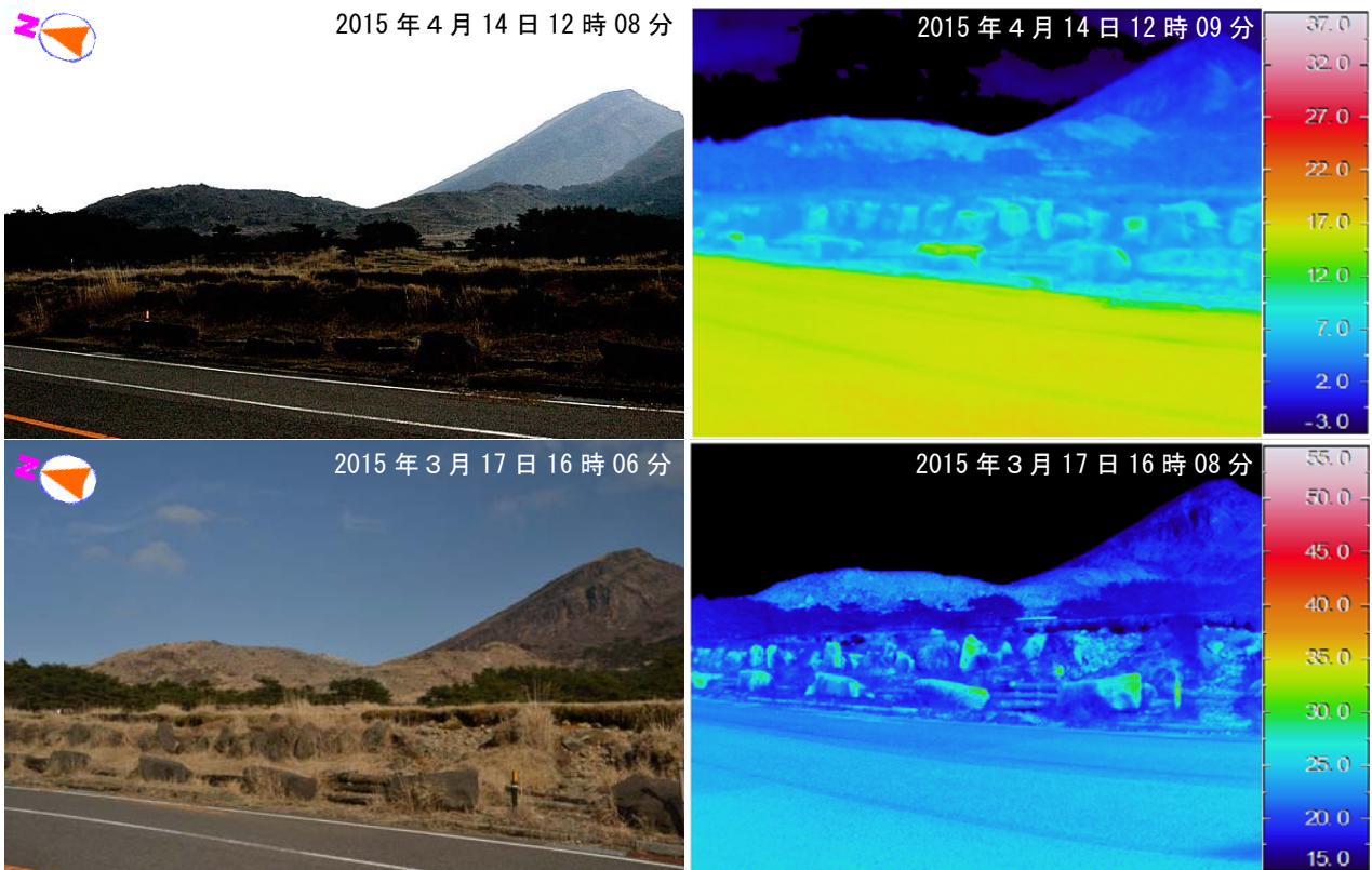
図 15-1 霧島山（えびの高原（硫黄山）周辺） えびのエコミュージアムセンター駐車場からの可視画像および赤外熱映像装置による地表面温度分布 噴気および熱異常域は認められませんでした。
