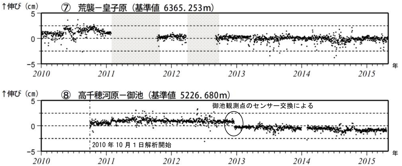
図 6-2 霧島山 GNSS 連続観測による基線長変化（2010 年 1 月～2015 年 4 月）
