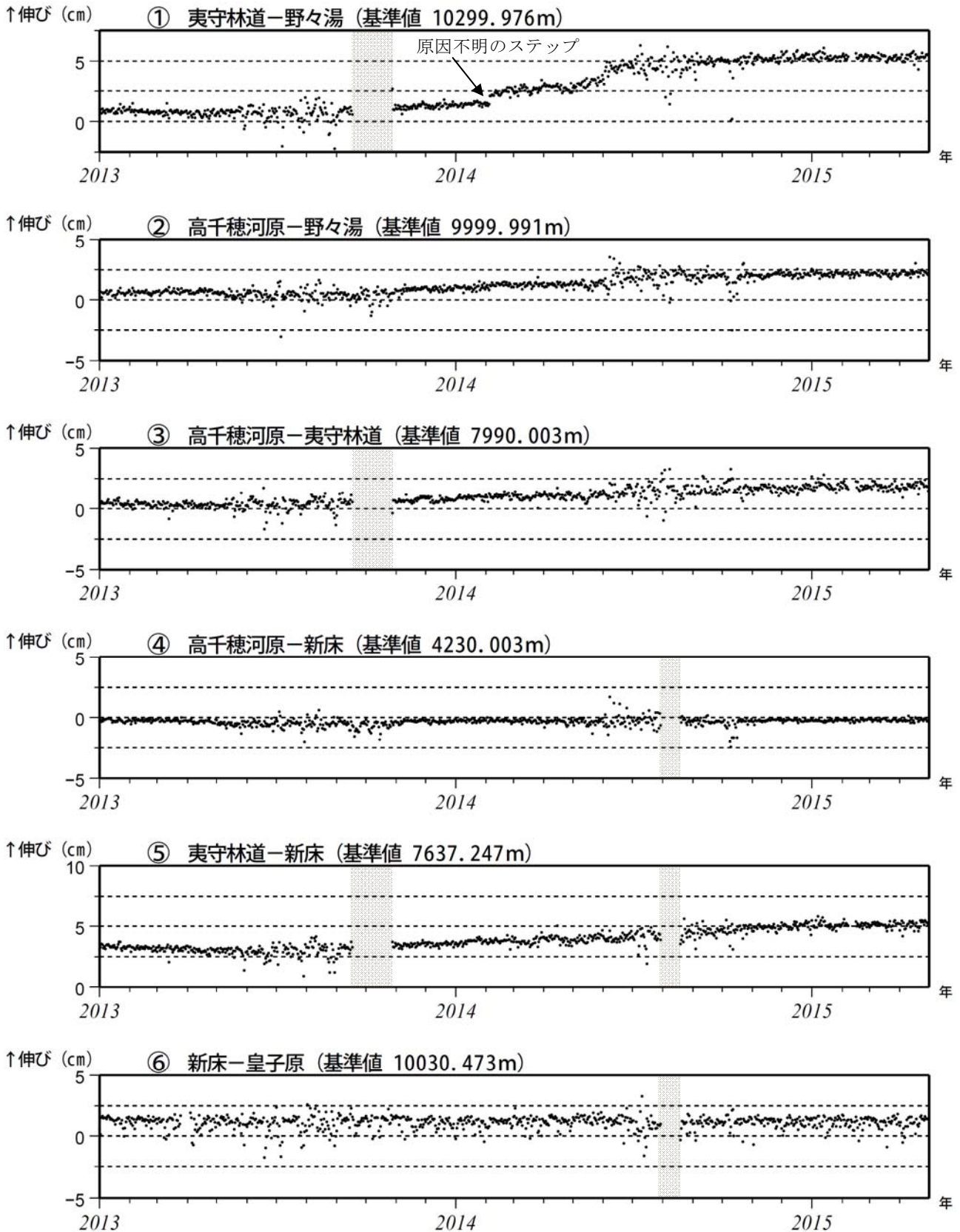
図 6-1 霧島山 GNSS 連続観測による基線長変化 (2010 年 1 月～2015 年 4 月)
