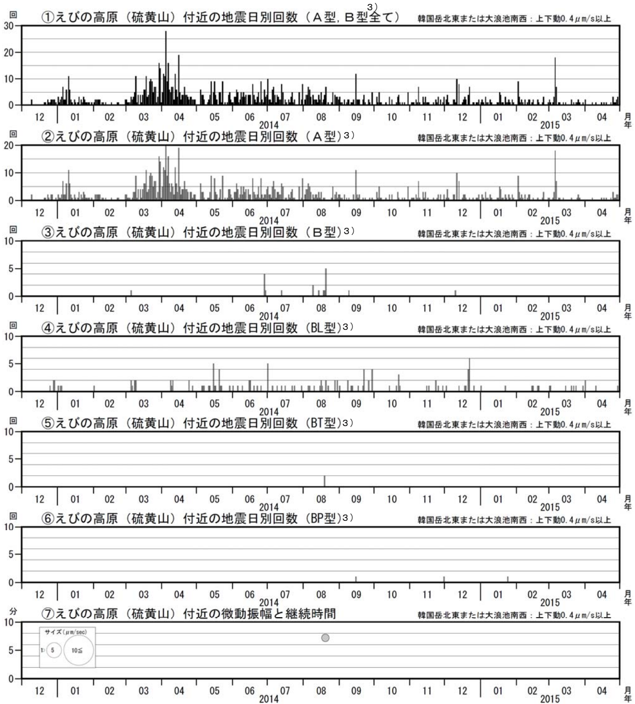
図 12 霧島山（えびの高原（硫黄山）周辺） 火山活動経過図（2013 年 12 月～2015 年 4 月）
