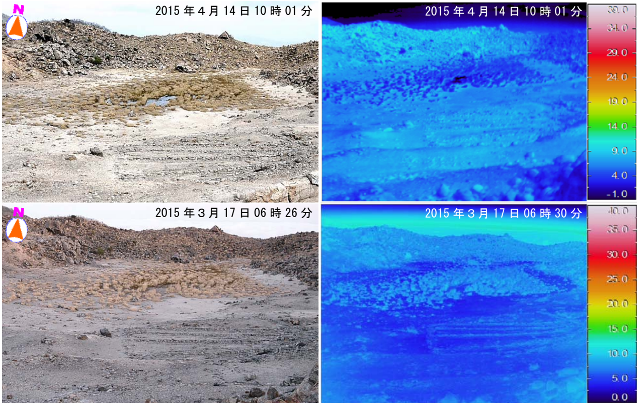
図 15-3 霧島山（えびの高原（硫黄山）周辺） 硫黄山火口南側からの可視画像および赤外熱映像装置による地表面温度分布 噴気および熱異常域は認められませんでした。
