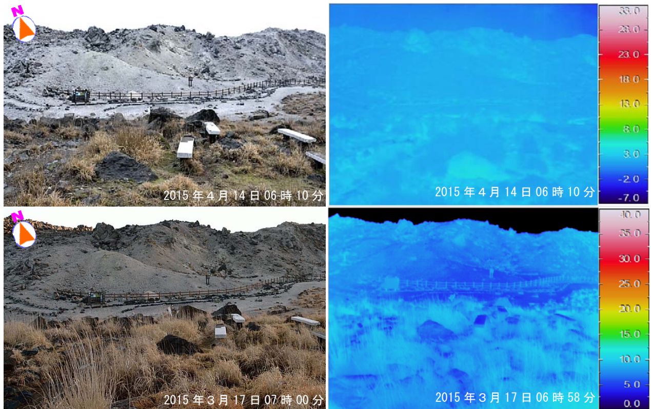
図 15-2 霧島山（えびの高原（硫黄山）周辺） 韓国岳登山道入り口のベンチからの可視画像および赤外熱映像装置による地表面温度分布 噴気および熱異常域は認められませんでした。
