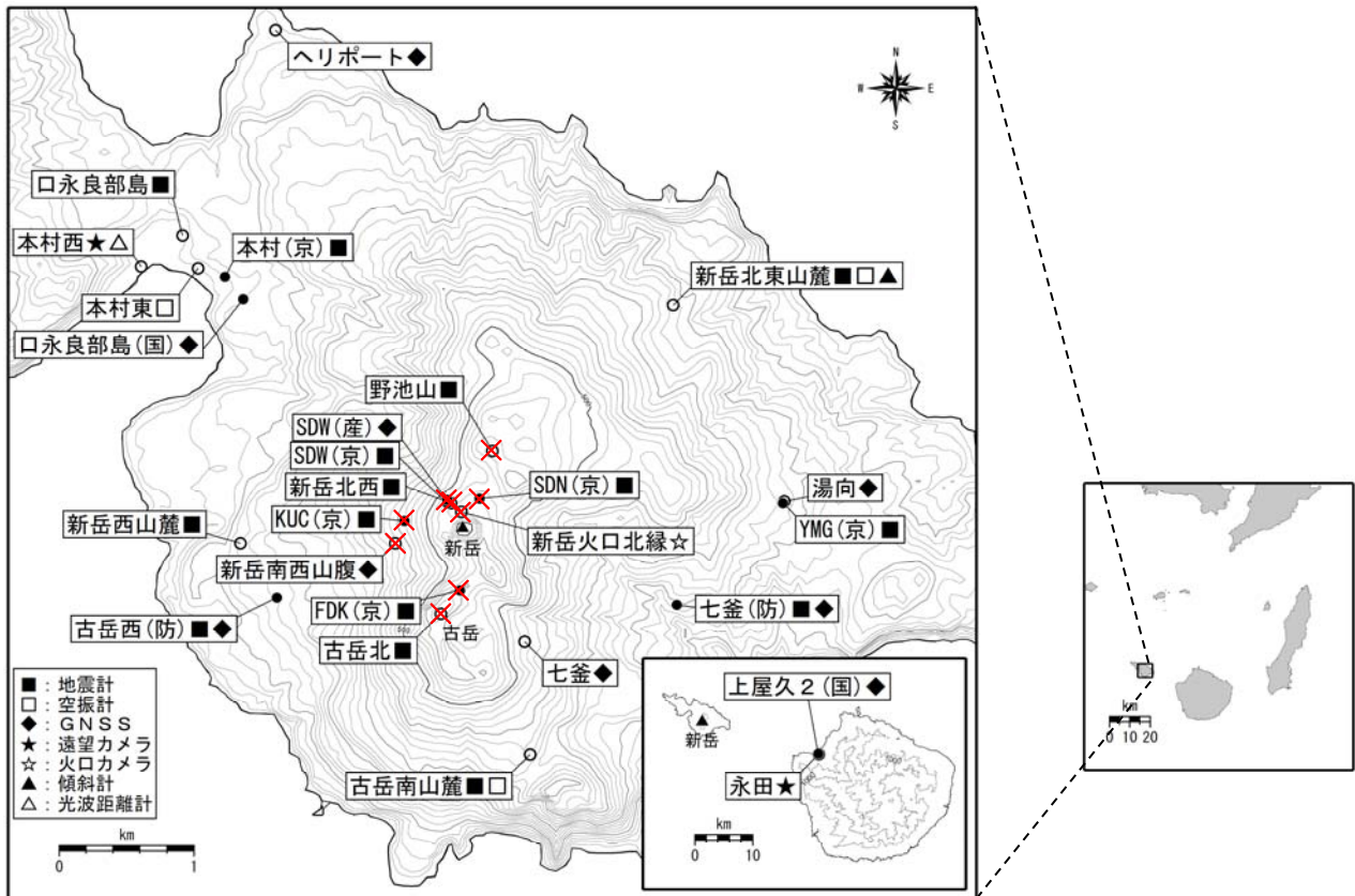
図 5 口永良部島 観測点配置図
