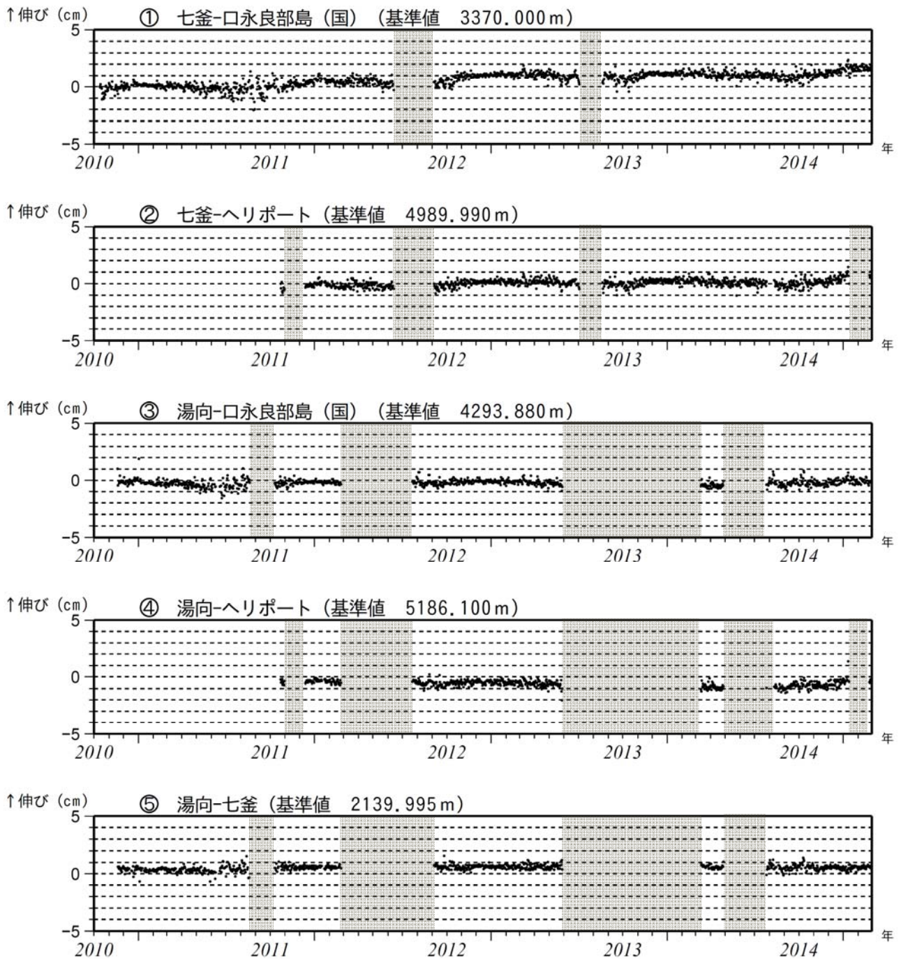
図3 口永良部島 GNSS 連続観測による基線長変化 (2010 年 10 月~2015 年 2 月) GNSS 連続観測では、2014 年 12 月頃から一部の基線にわずかな伸びの傾向が認められます。 これらの基線は図4の①~⑤に対応しています。灰色部分は観測点障害のため欠測を表しています。 (国) : 国土地理院、(防) : 防災科学技術研究所
