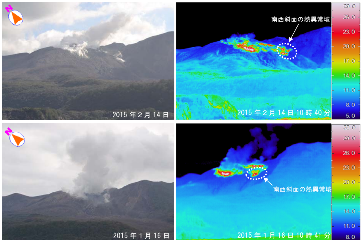
図 6-2 口永良部島 赤外熱映像装置による新岳火口付近の地表面温度分布（西南西側海上より撮影）
