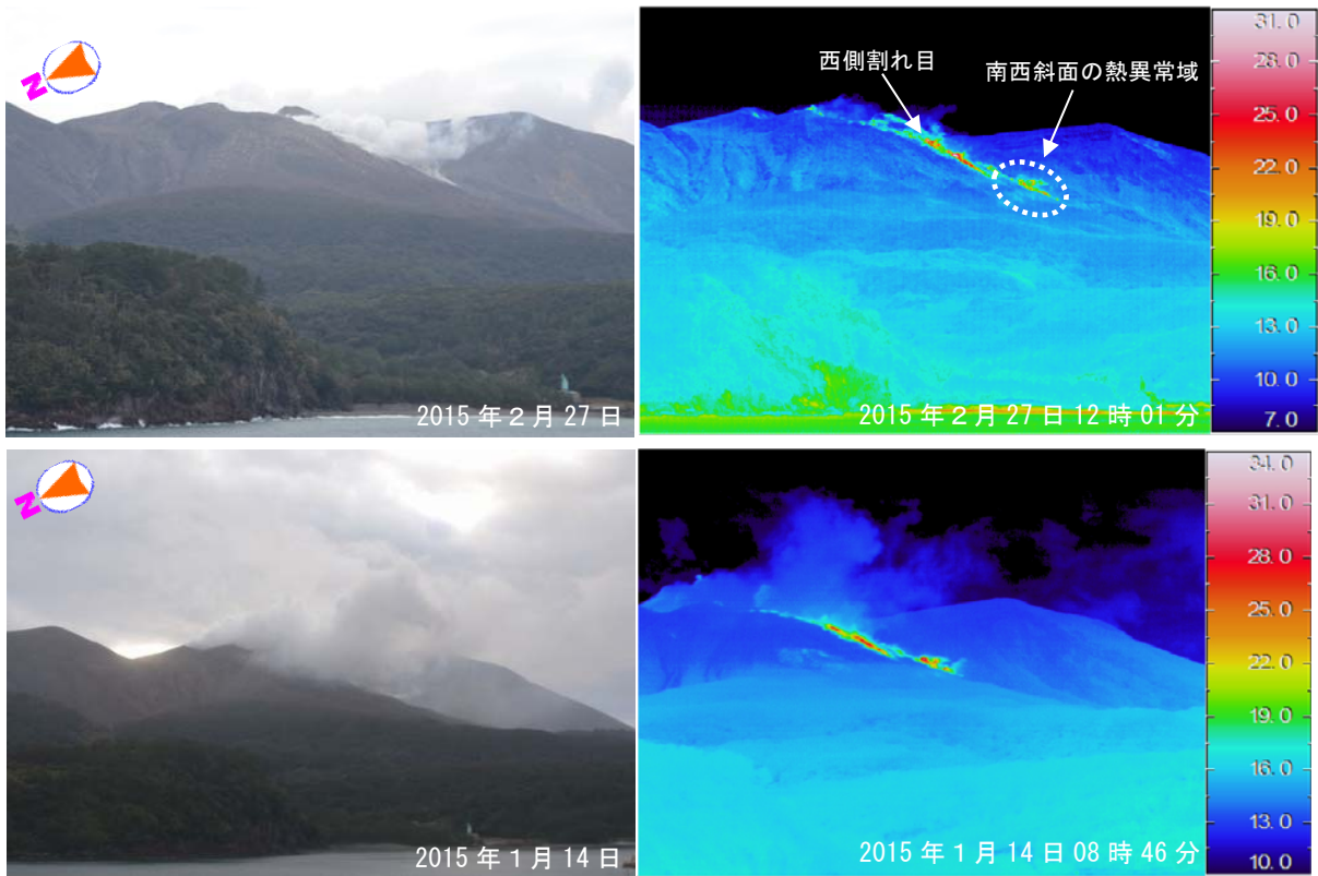
図 6-1 口永良部島 赤外熱映像装置による新岳火口付近の地表面温度分布（本村より撮影）
