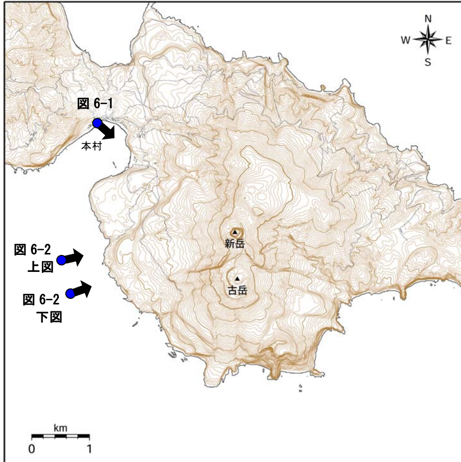
図 7 口永良部島 図 6 の撮影位置
