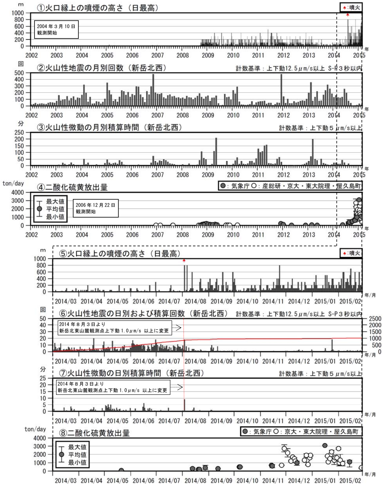
図2 口永良部島 火山活動経過図（2002年1月～2015年2月）
