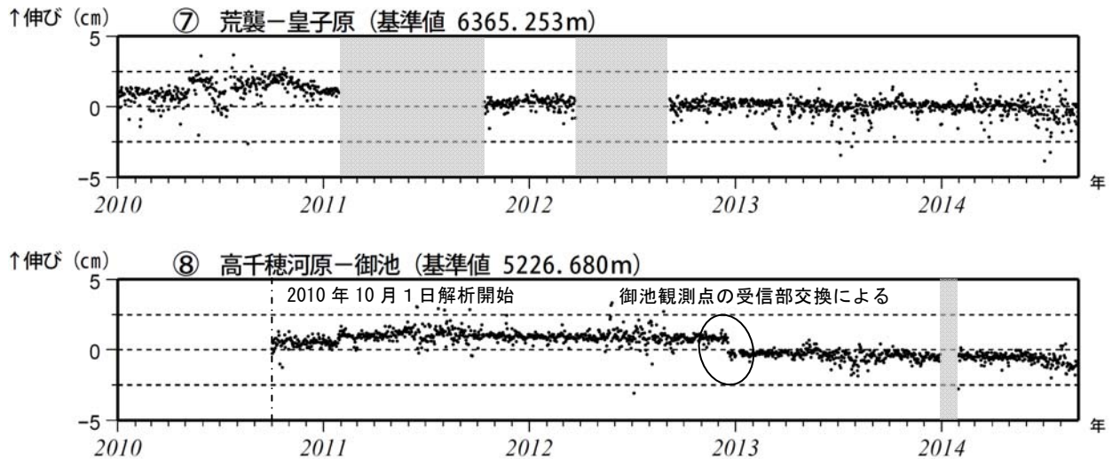
図 6-2 霧島山 GNSS 連続観測による基線長変化（2010 年 1 月～2014 年 8 月）
