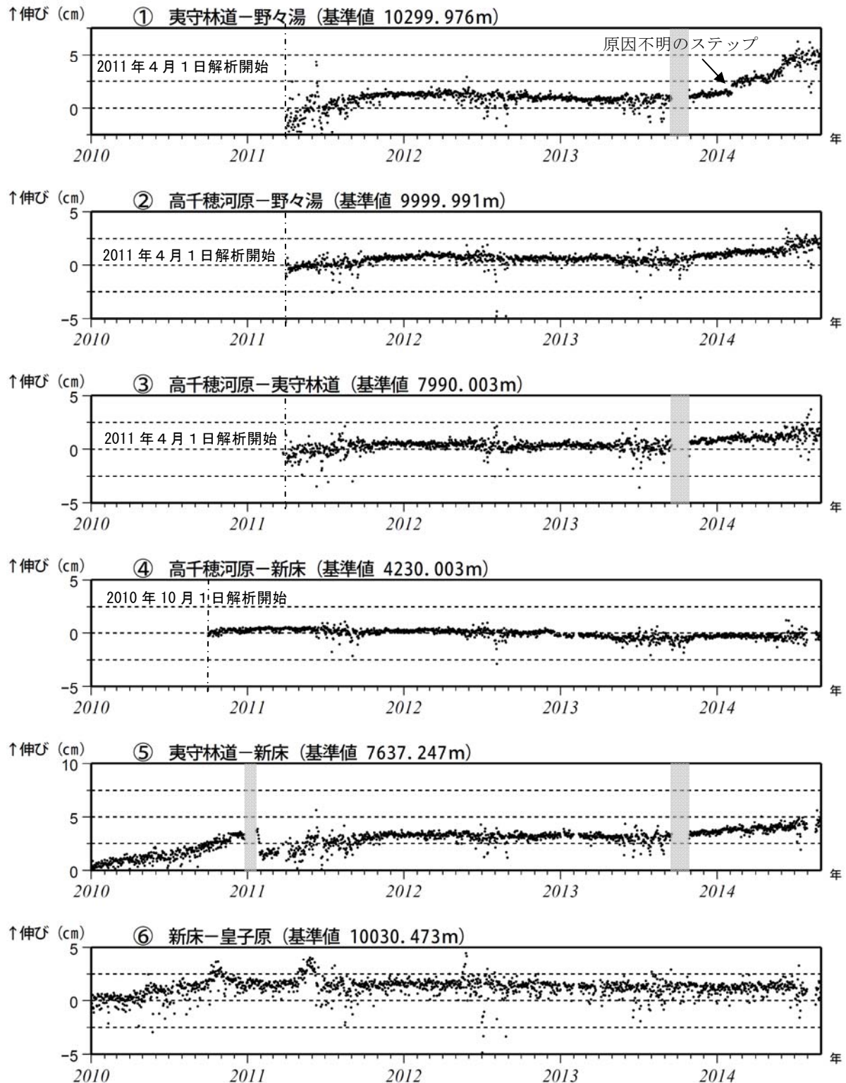
図 6-1 霧島山 GNSS 連続観測による基線長変化 (2010 年 1 月～2014 年 8 月)
