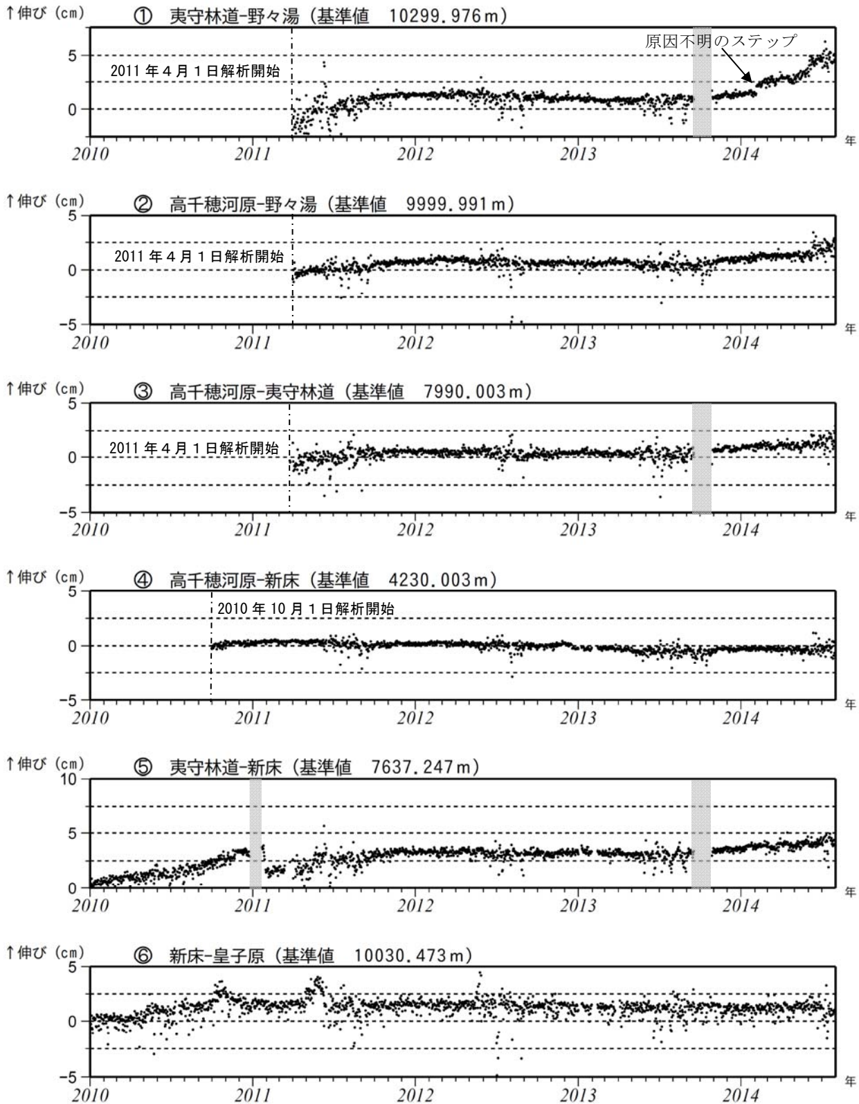
図 6-1 霧島山 GNSS 連続観測による基線長変化（2010 年 1 月～2014 年 7 月）
