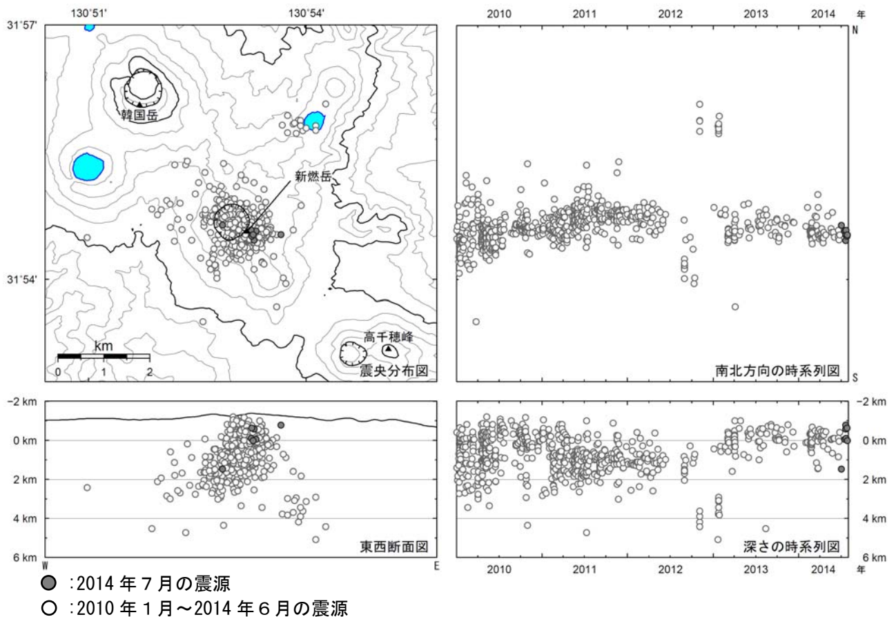
図 2 霧島山（新燃岳） 震源分布図（2010 年 1 月～2014 年 7 月）
