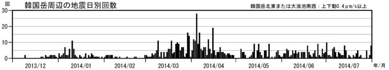
図9 霧島山（韓国岳周辺、大浪池付近） 地震日別回数（2013年12月～2014年7月）
