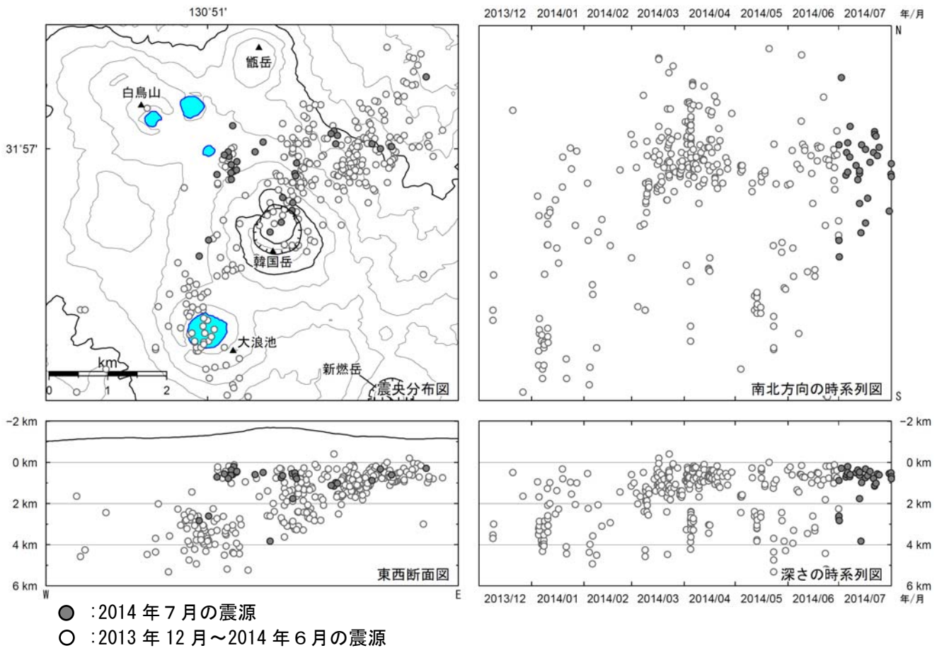
図10 霧島山（韓国岳周辺、大浪池付近） 震源分布図（2013年12月～2014年7月）
