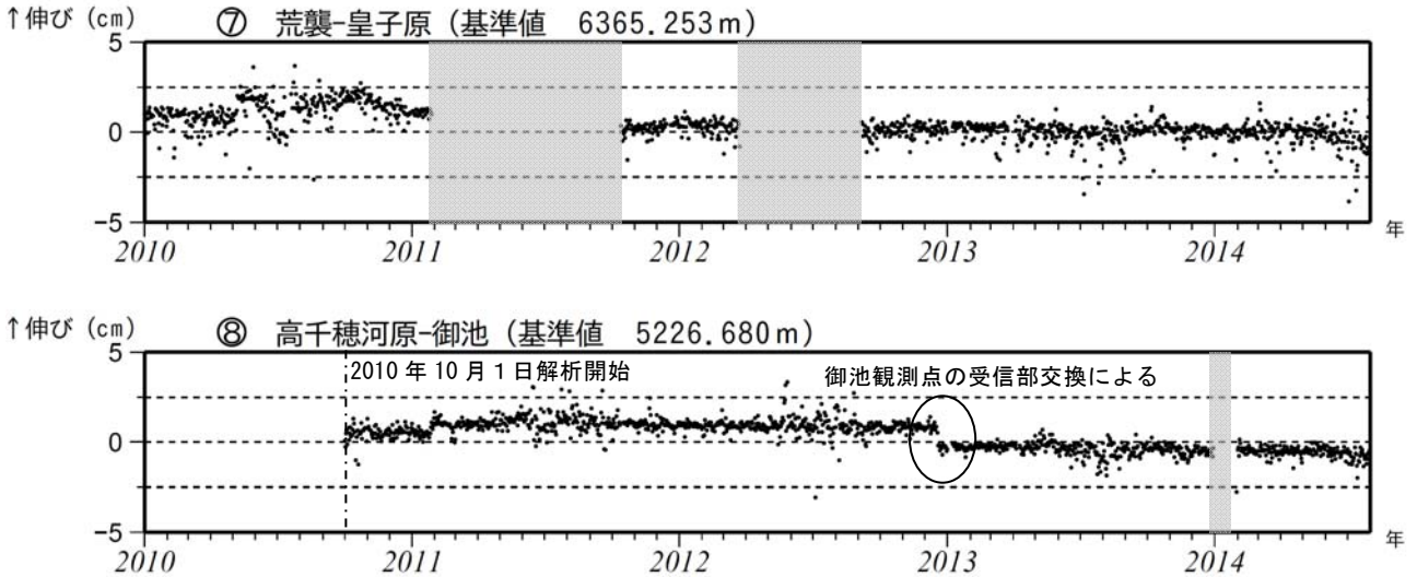
図 6-2 霧島山 GNSS 連続観測による基線長変化（2010 年 1 月～2014 年 7 月）
