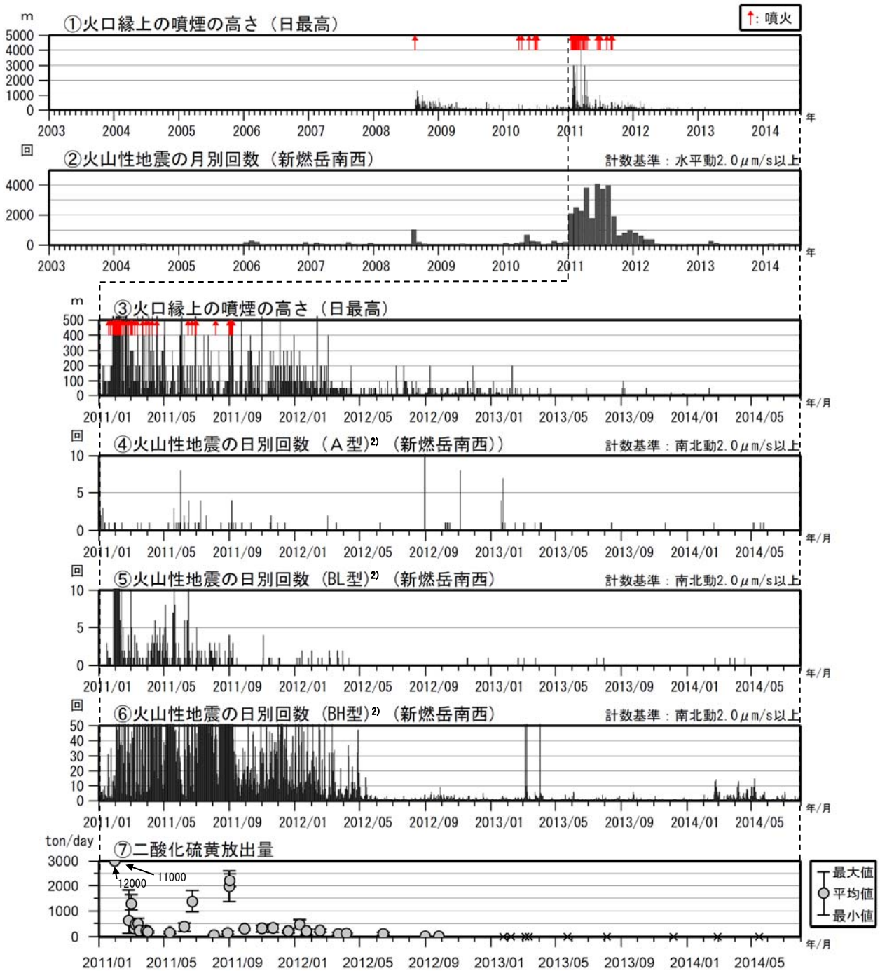
図3 霧島山（新燃岳） 火山活動経過図（2003年1月～2014年7月）
