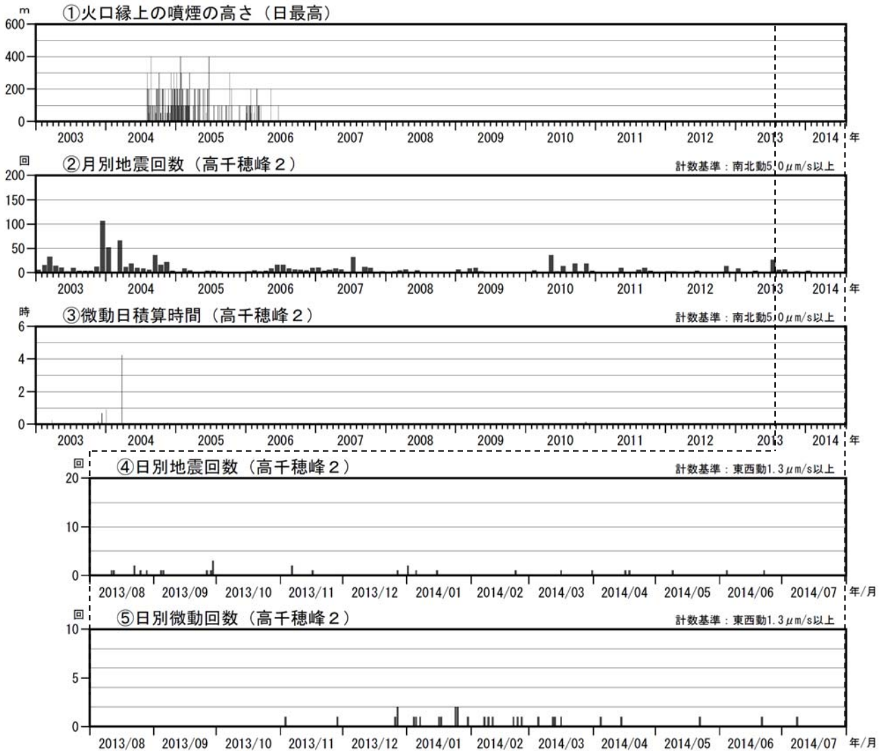
図 12 霧島山（御鉢） 火山活動経過図（2003 年 1 月～2014 年 7 月）
