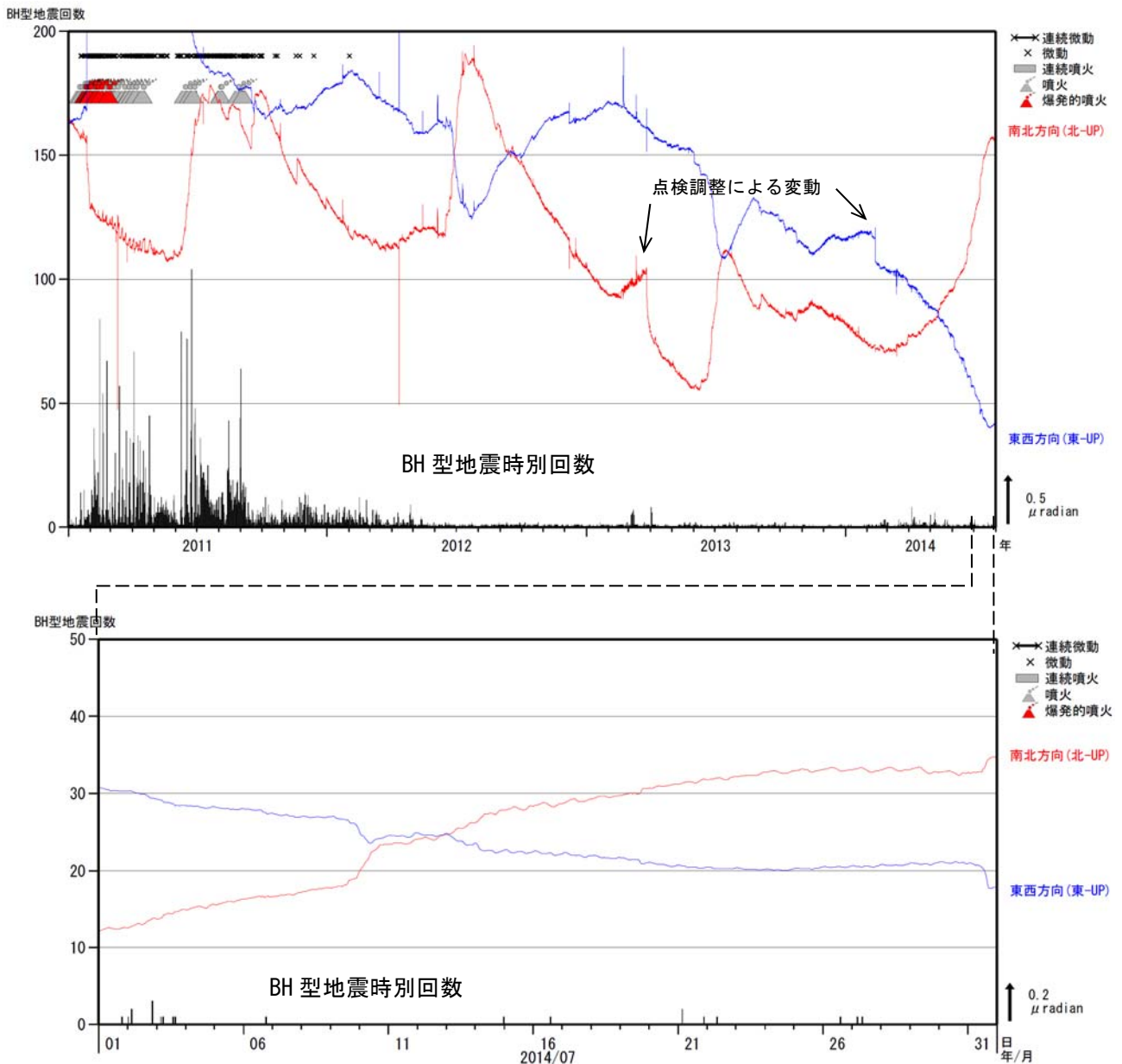
図4 霧島山（新燃岳） BH型地震の時間別回数と高千穂河原傾斜計の傾斜変動（2011年1月～2014年7月）
