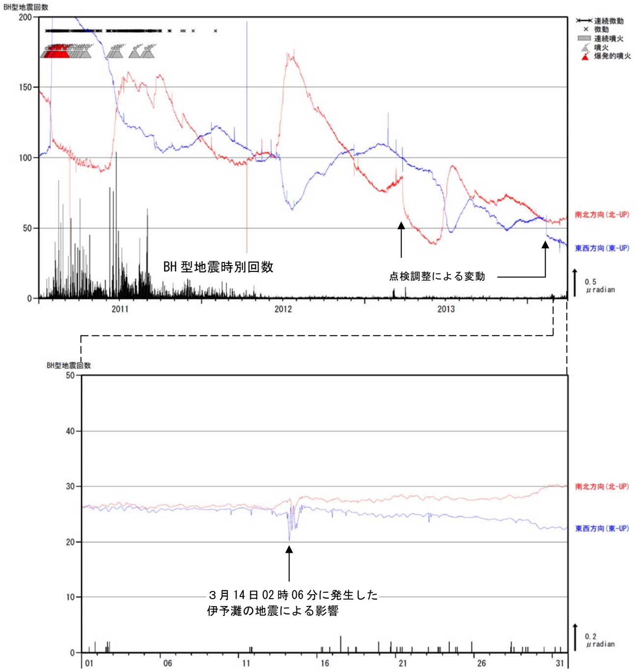
図4 霧島山（新燃岳）BH型地震の時間別回数と高千穂河原傾斜計の傾斜変動（2011年1月～2014年3月）
