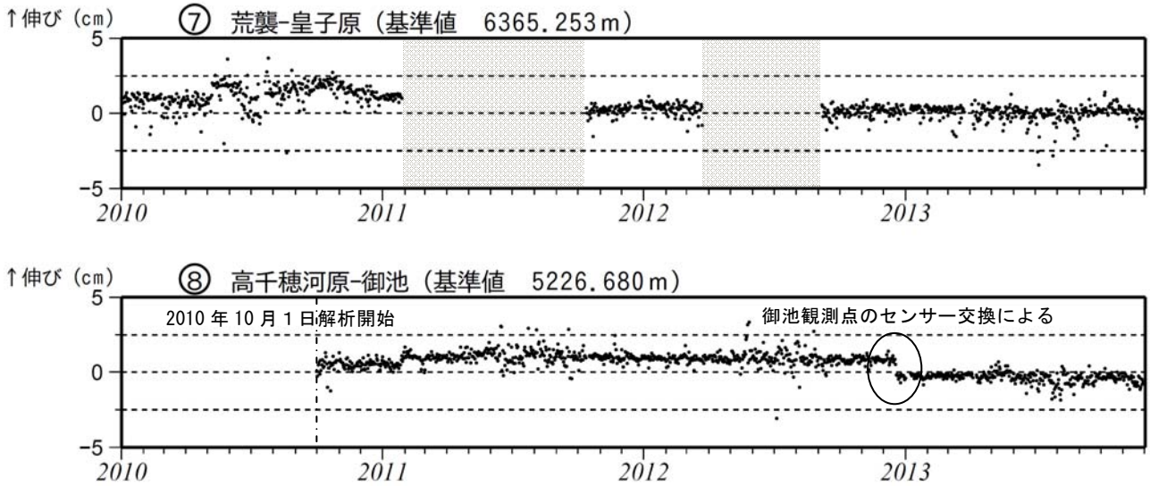
図 6-2 霧島山 GPS 連続観測による長期の基線長変化（2010 年 1 月～2013 年 11 月）
