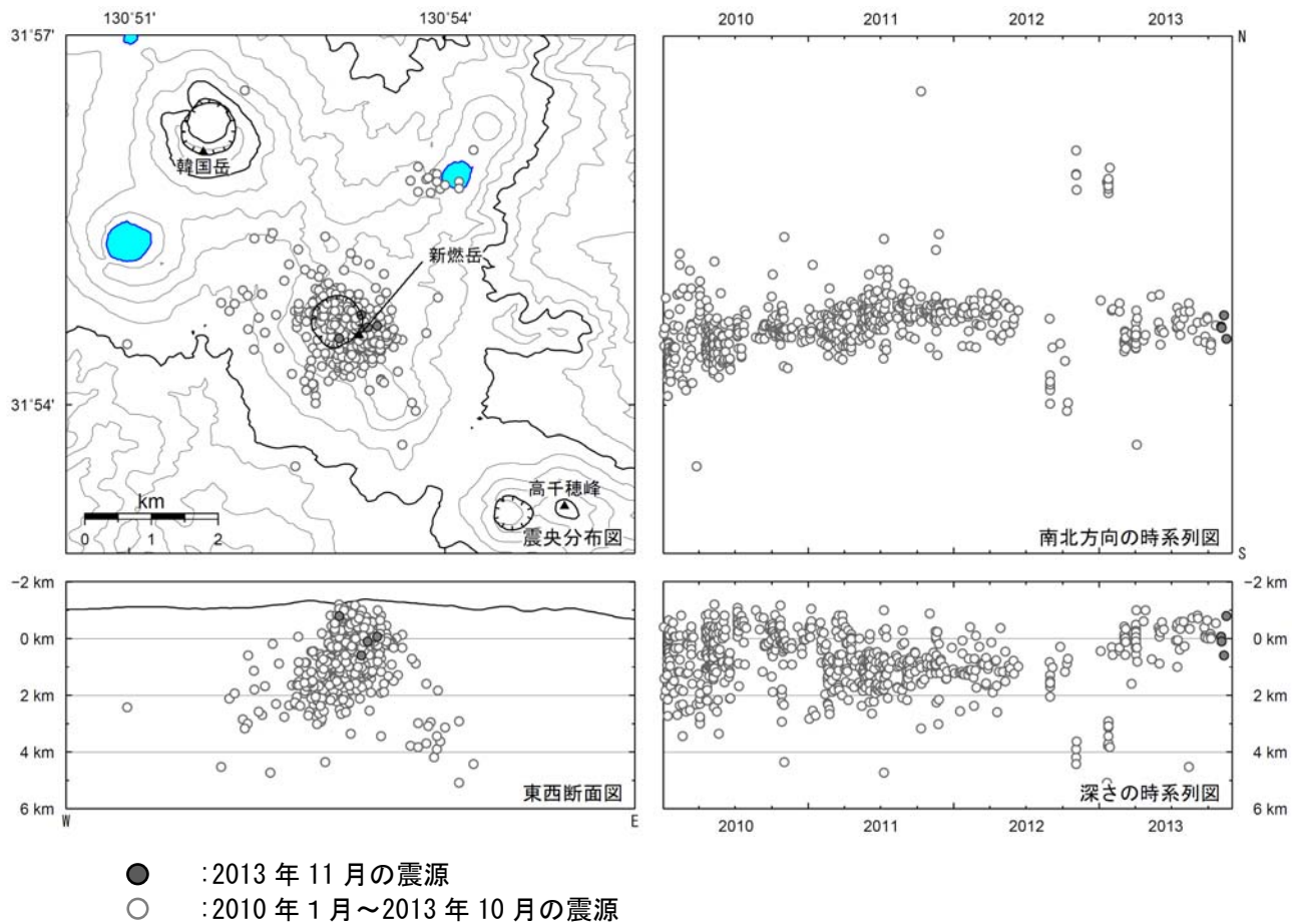
図 2 霧島山（新燃岳） 震源分布図（2010 年 1 月～2013 年 11 月）
