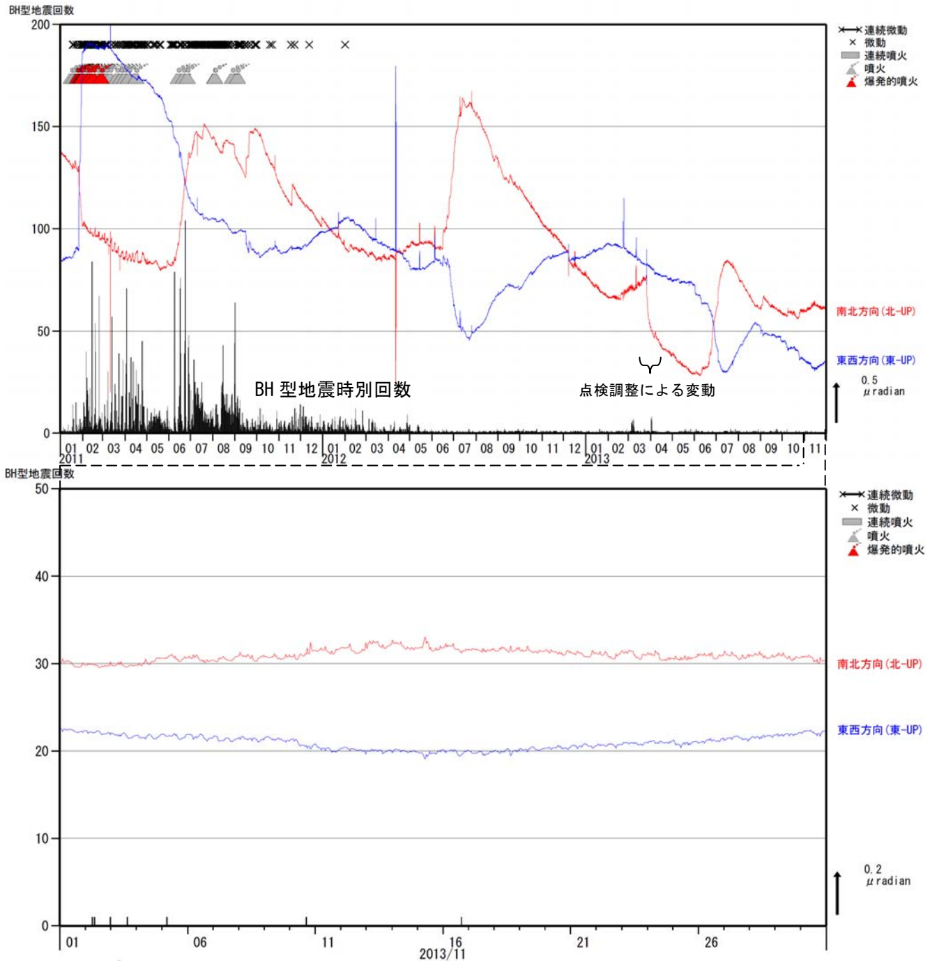
図4 霧島山（新燃岳） BH型地震の時間別回数と高千穂河原傾斜計の傾斜変動 （2011年1月～2013年11月）
