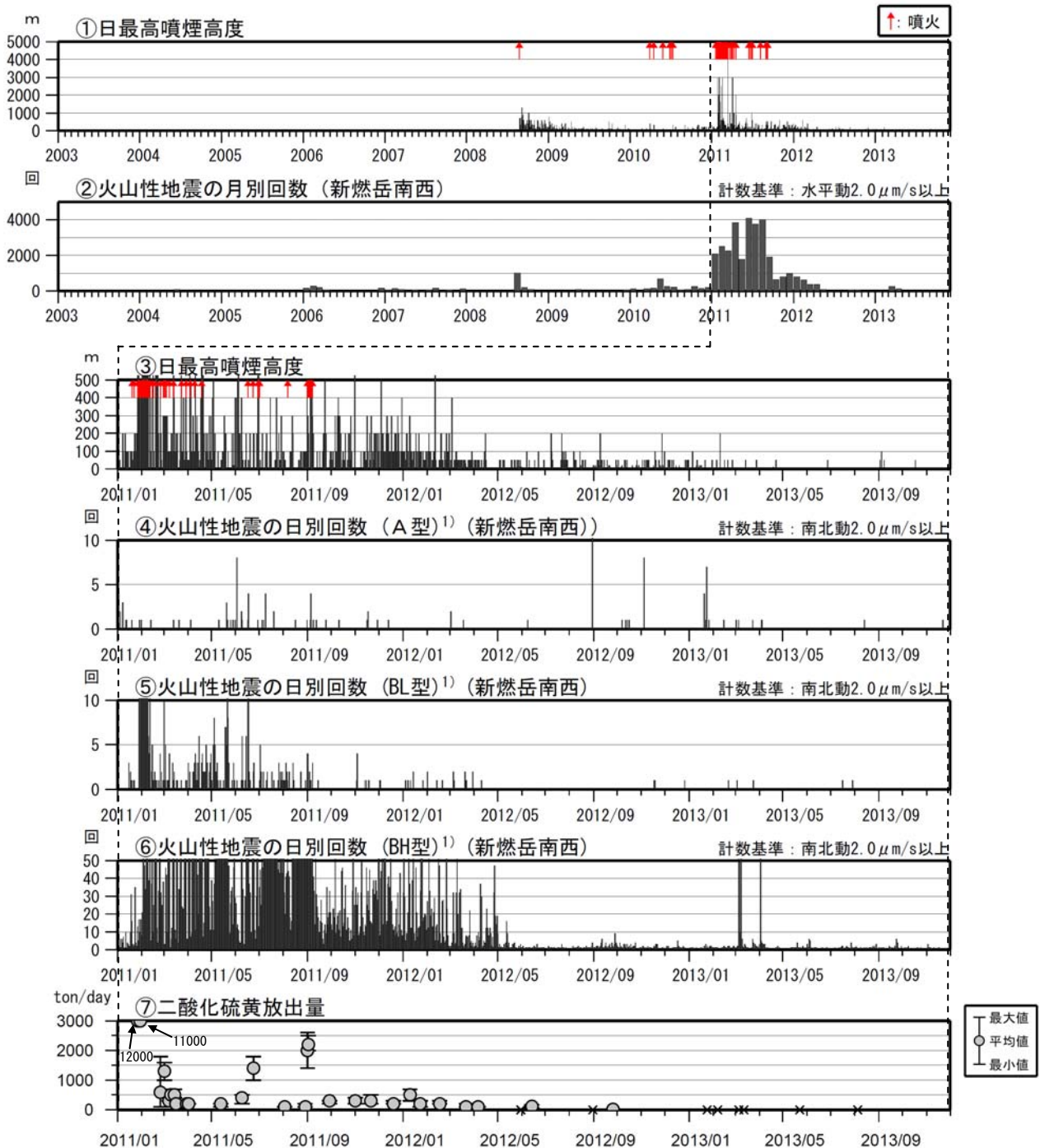
図3 霧島山（新燃岳） 火山活動経過図（2003年1月～2013年11月） <11月の状況>
