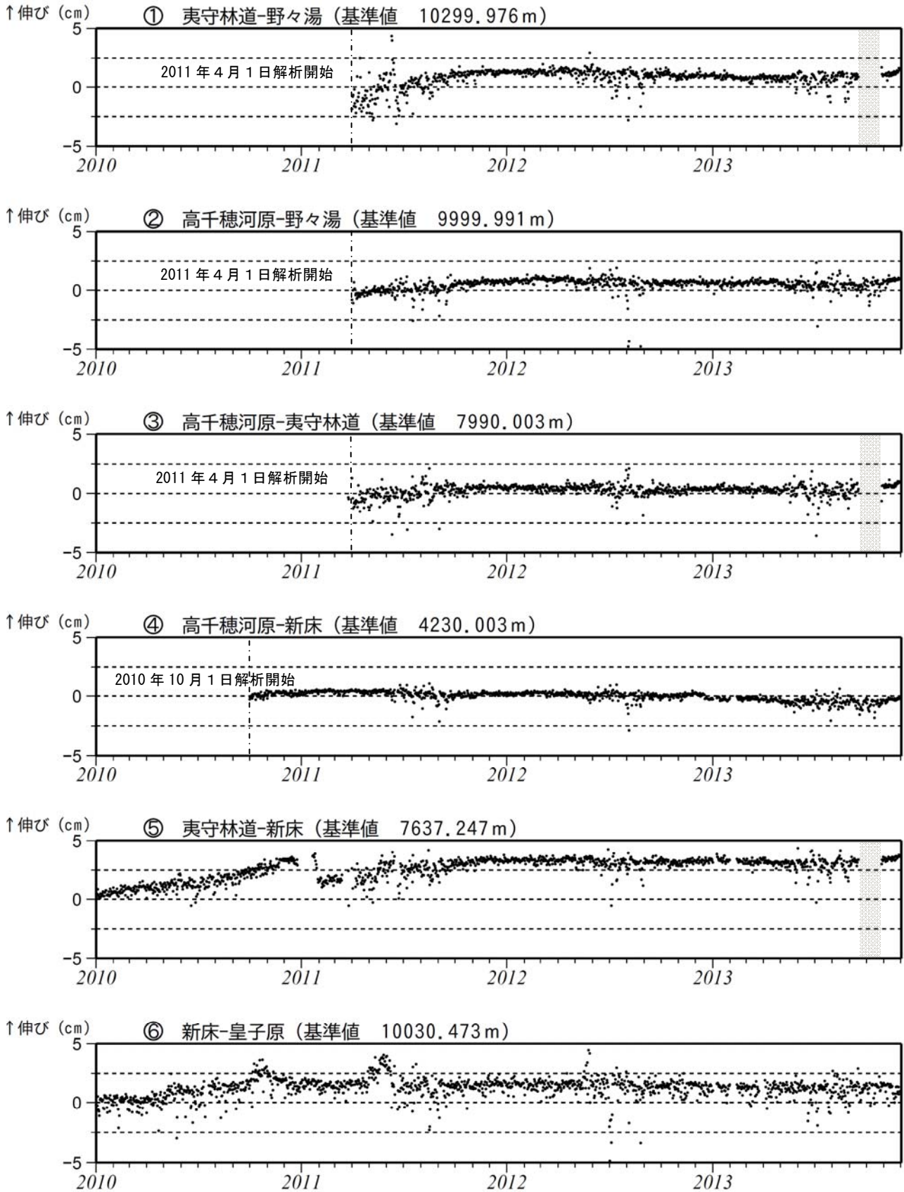
図 6-1 霧島山 GPS 連続観測による長期の基線長変化（2010 年 1 月～2013 年 11 月） GPS 連続観測では、新燃岳周辺の基線で火山活動によると考えられる変化は認められませんでした。
