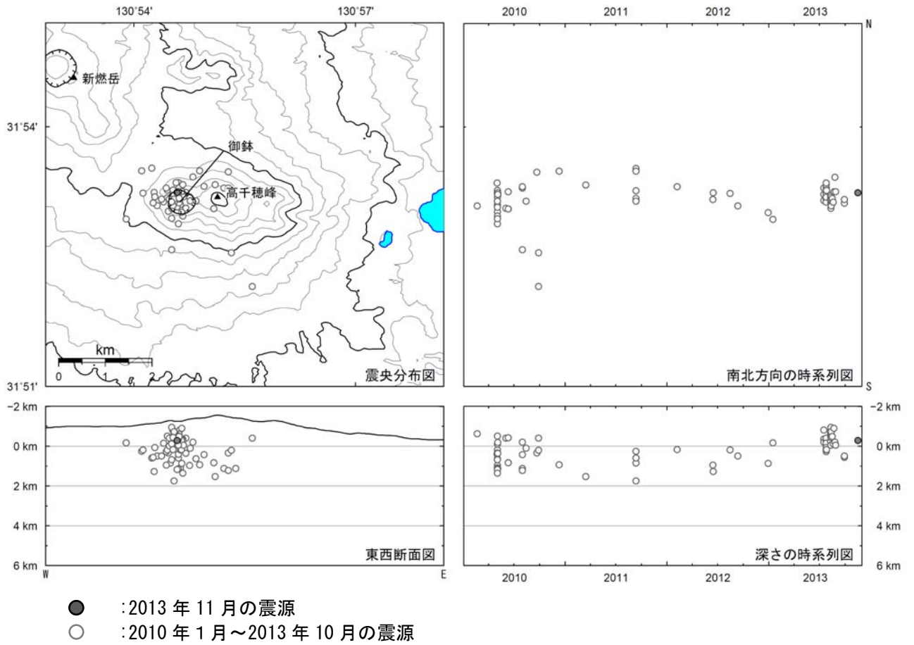
図 10 霧島山（御鉢） 震源分布図（2010 年 1 月～2013 年 11 月）
