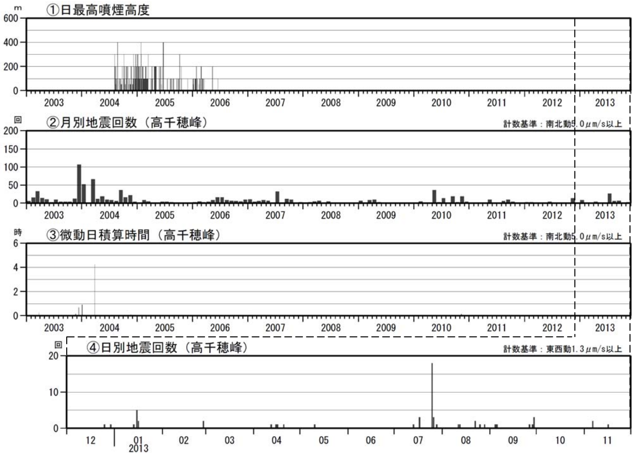
図 11 霧島山（御鉢） 火山活動経過図（2003 年 1 月～2013 年 11 月）
