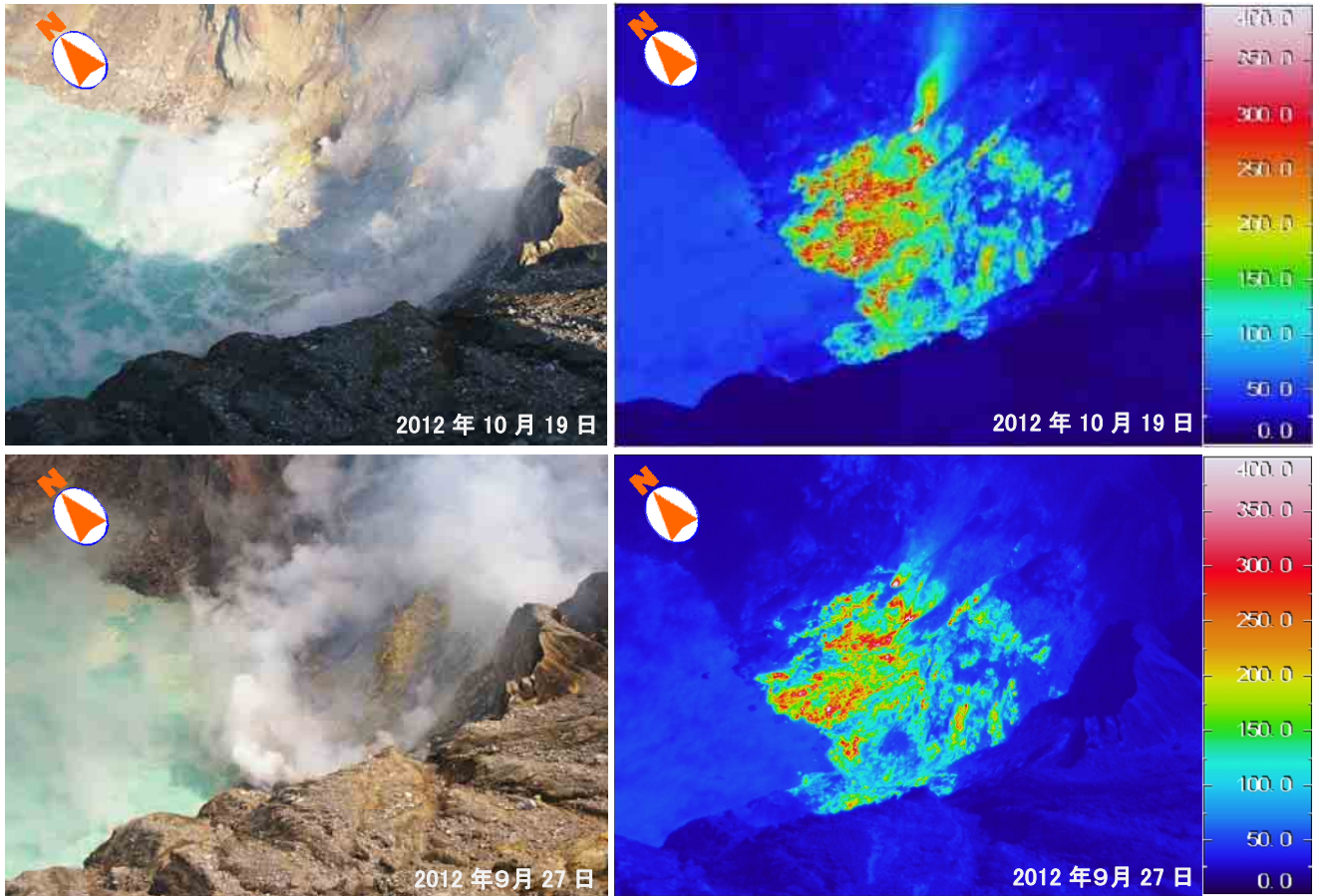
図 13 阿蘇山 赤外熱映像装置による中岳第一火口南側火口壁の地表面温度分布 （左：可視画像 右：赤外画像） （上段：10月19日撮影 下段：9月27日撮影） 温度分布に、特段の変化はありませんでした。
