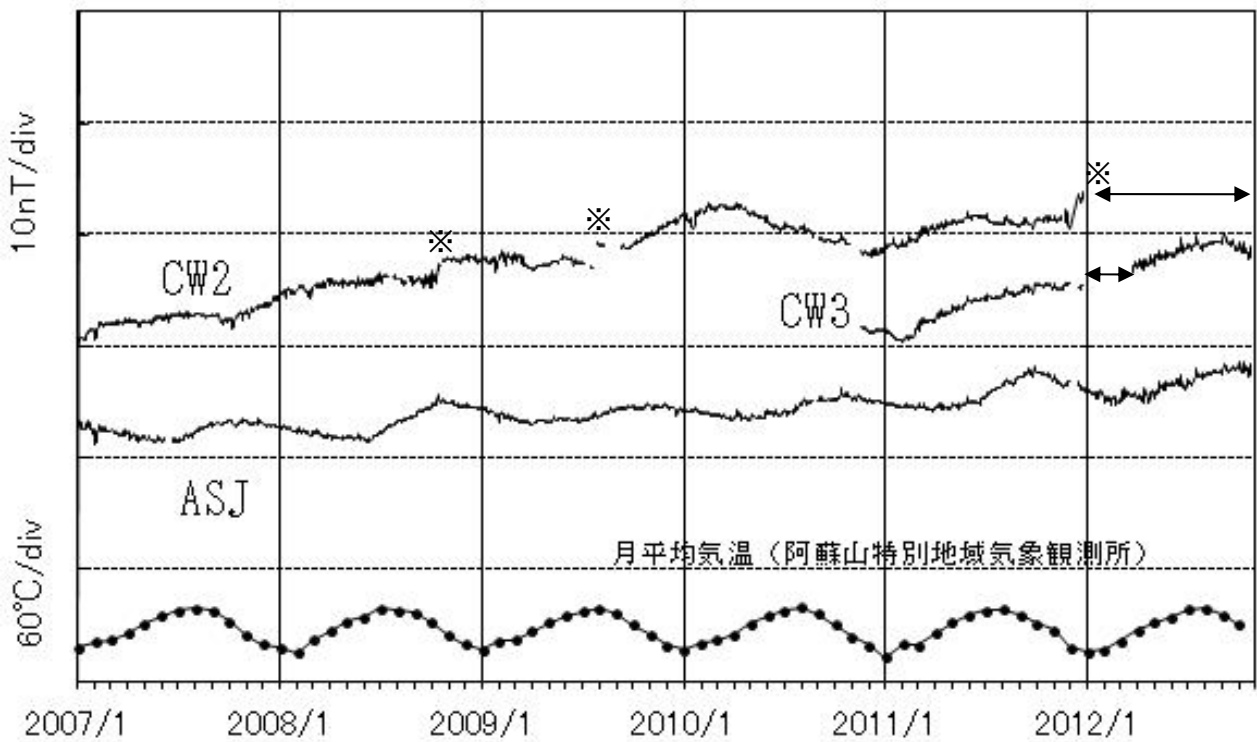
図 10 阿蘇山 阿蘇山麓 (AHK) を基準とした阿蘇中岳火口周辺の全磁力変化、及び阿蘇山特別地域気象観測所における月平均気温 (2007 年 1 月～2012 年 10 月)
