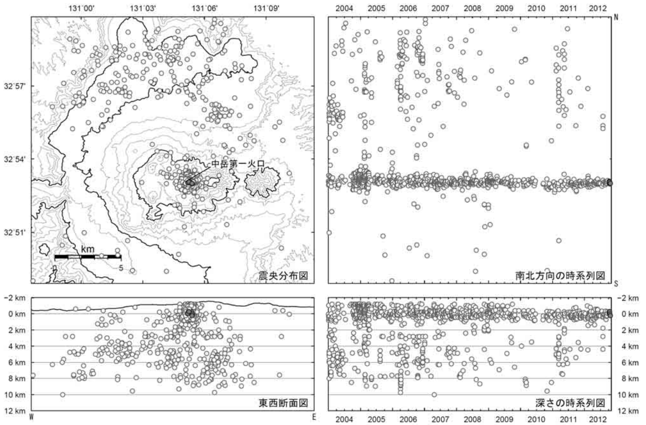
図 6※ 阿蘇山 震源分布図（2004 年 1 月～2012 年 10 月）
