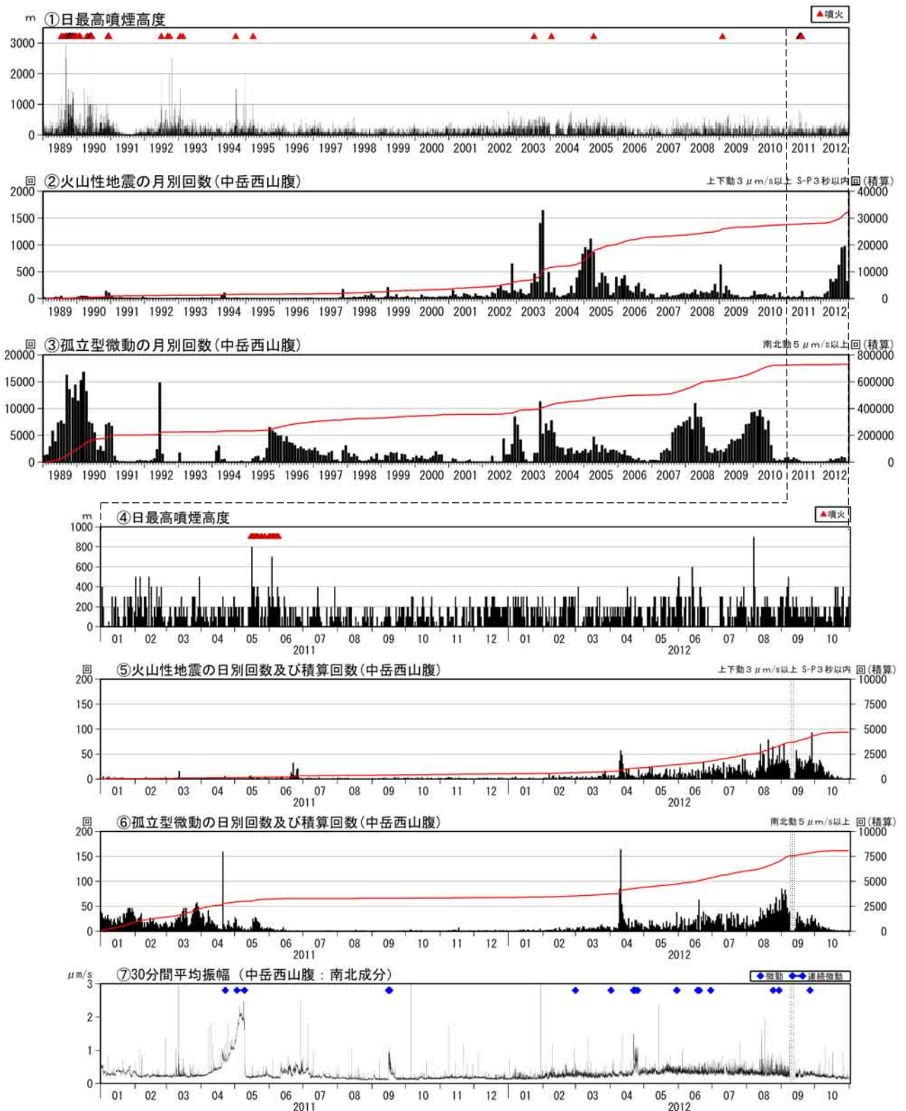
図4 阿蘇山 火山活動経過図（1989年1月～2012年10月） 緩やかな増加傾向を示していた孤立型微動および火山性地震は2012年9月中旬以降減少しています。 <10月の状況> ・噴煙活動に特段の変化はなく、白色の噴煙が概ね火口縁上 200mで経過し、最高で火口縁上 400mまで上がりました。 ・孤立型微動は、月回数が152回（9月：867回）と減少しました。 ・火山性地震は、月回数が324回（9月：978回）と減少しました。 ・火山性微動は発生しませんでした（9月：1回）。
