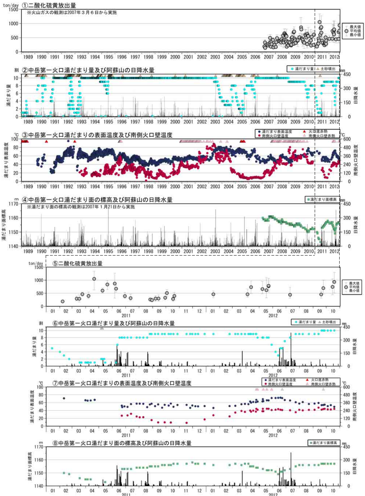
図5※ 阿蘇山 湯だまり、火口壁、二氧化硫黄放出量の状況（1989年1月～2012年10月） <10月の状況>
