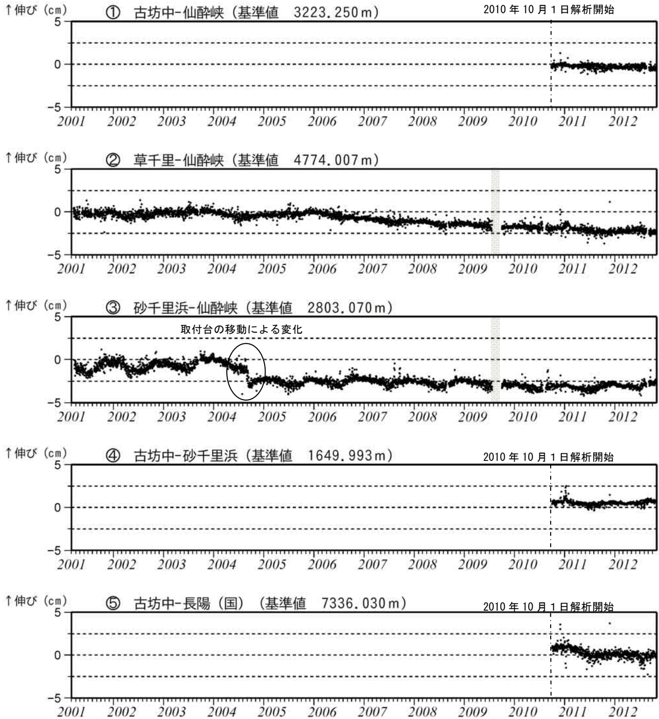
図 8※ 阿蘇山 GPS連続観測による基線長変化（2001 年 3 月～2012 年 10 月）
