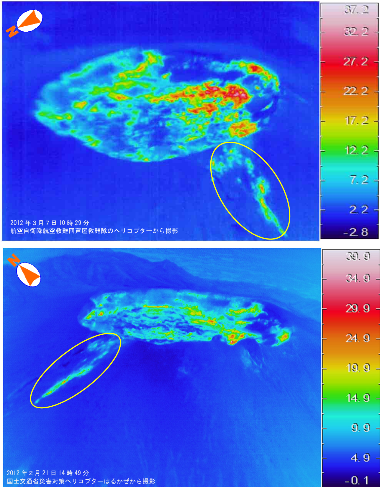
図2 霧島山（新燃岳） 赤外熱映像装置による火口付近の地表面温度分布 ・ 前回（2月21日）と比較して地表面温度分布に大きな変化はなく、火口内に蓄積された溶岩の縁辺部が比較的高温でした。 ・ 西側斜面の割れ目の一部（黄丸）では、前回の調査と同様にやや温度の高い部分が認められました。
