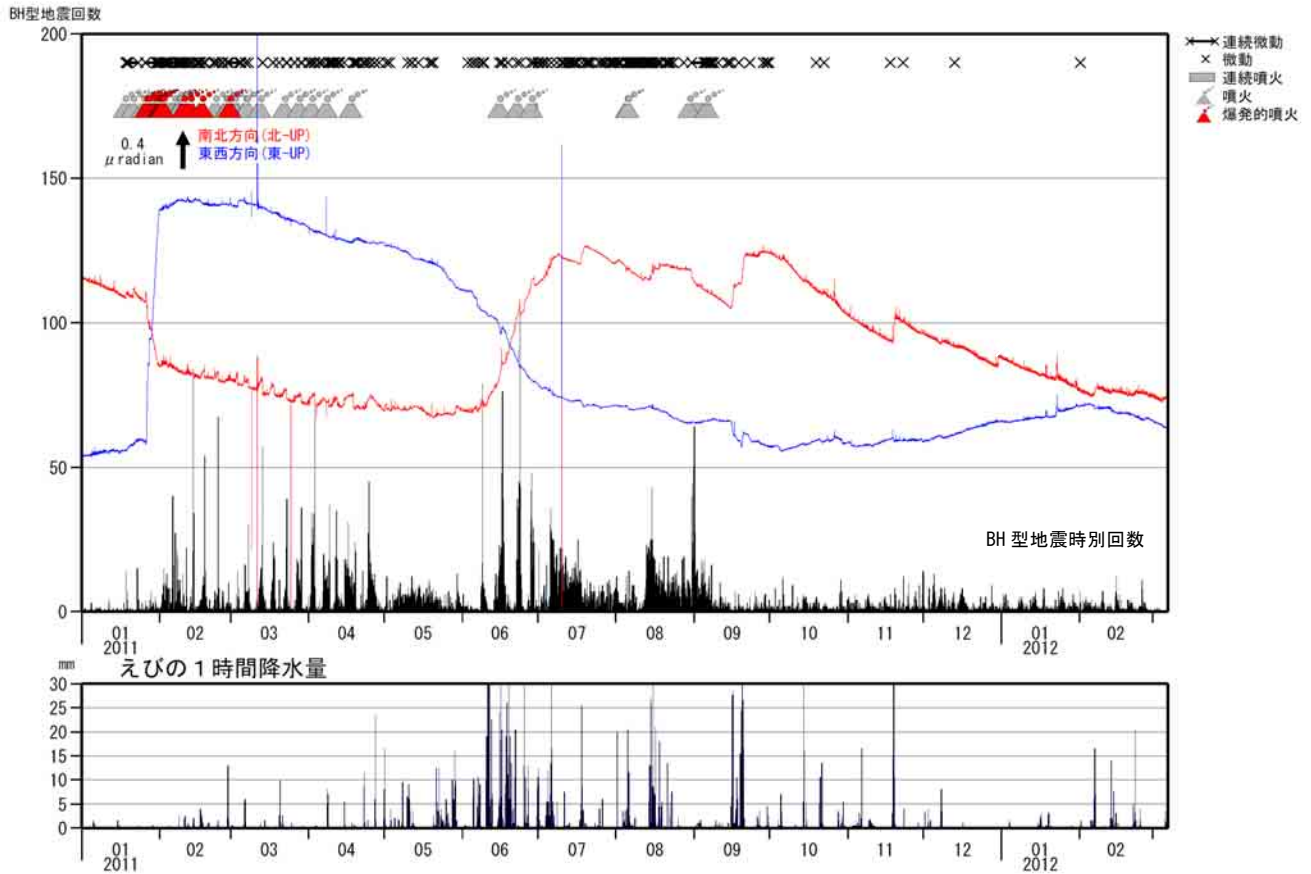
図3 霧島山（新燃岳） BH型地震 2) の時間別回数と高千穂河原傾斜計（新燃岳の南東約3 km）の変化（2011年1月～2012年3月6日）
