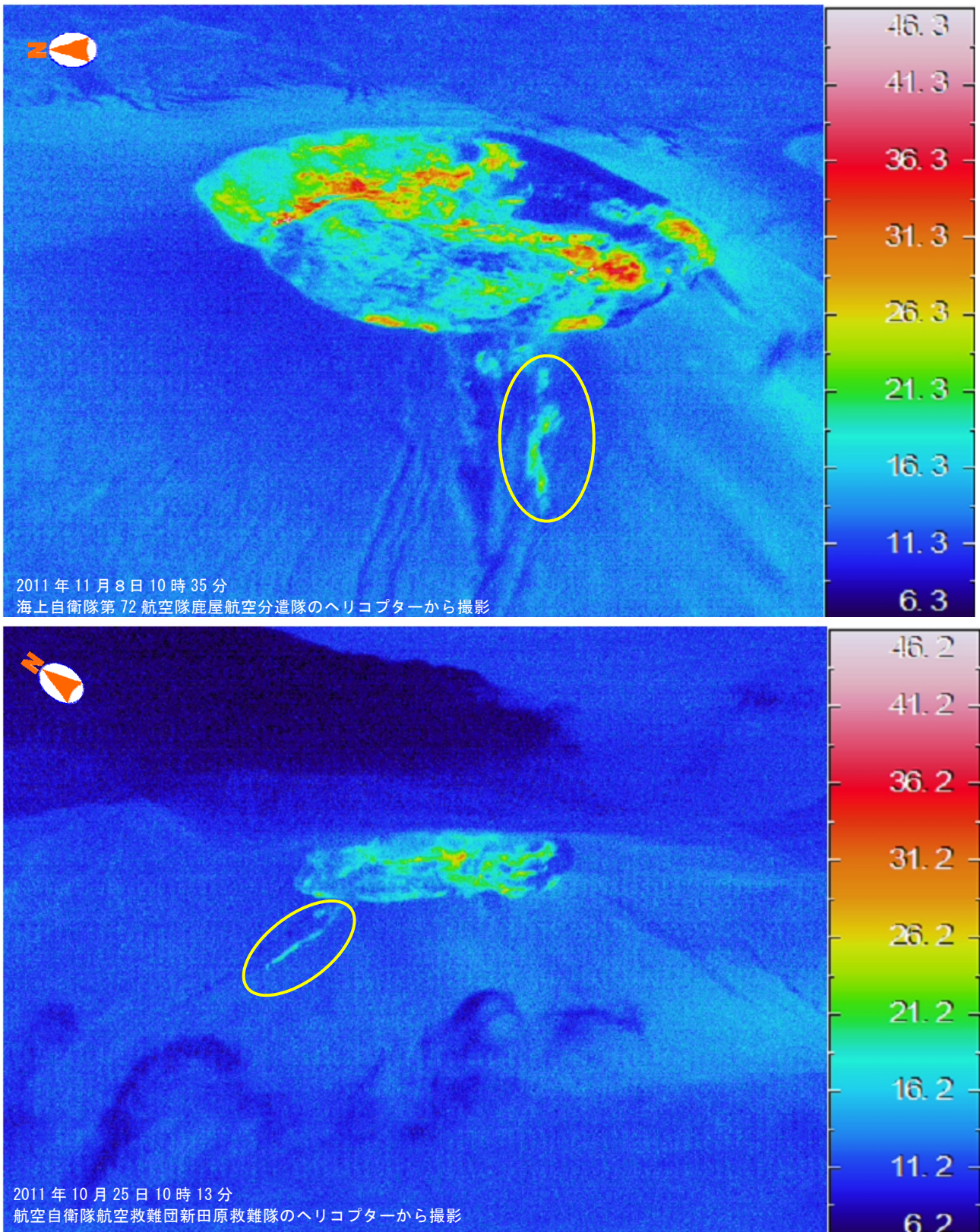
図 2 霧島山（新燃岳） 赤外熱映像装置による火口付近の地表面温度分布 10 月 25 日と比較して地表面温度分布に大きな変化はなく、火口内に蓄積された溶岩の縁辺部が比較的高温でした。また、2008 年 8 月の噴火時に形成された西側斜面の割れ目（図 2 の黄丸）の一部にも、10 月 25 日の調査と同様にやや温度の高い部分が認められました。
