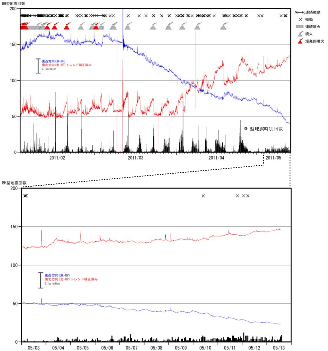
図3 霧島山（新燃岳） BH型地震 2) の時間別回数と高千穂河原傾斜計の変化 (2011年2月1日00時00分～5月13日13時00分) 5月4日0時頃から新燃岳側がわずかに隆起する変化が観測されていましたが、噴火は発生せず、4日11時頃沈降に転じ、その後停滞しています。
