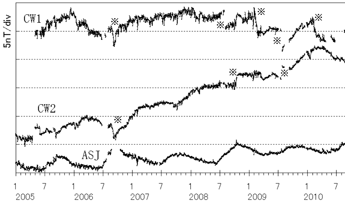
図 6 阿蘇山 全磁力連続観測による阿蘇山麓 (AHK) を基準とした中岳第一火口周辺の全磁力変化 (2005 年 1 月～2010 年 8 月)
