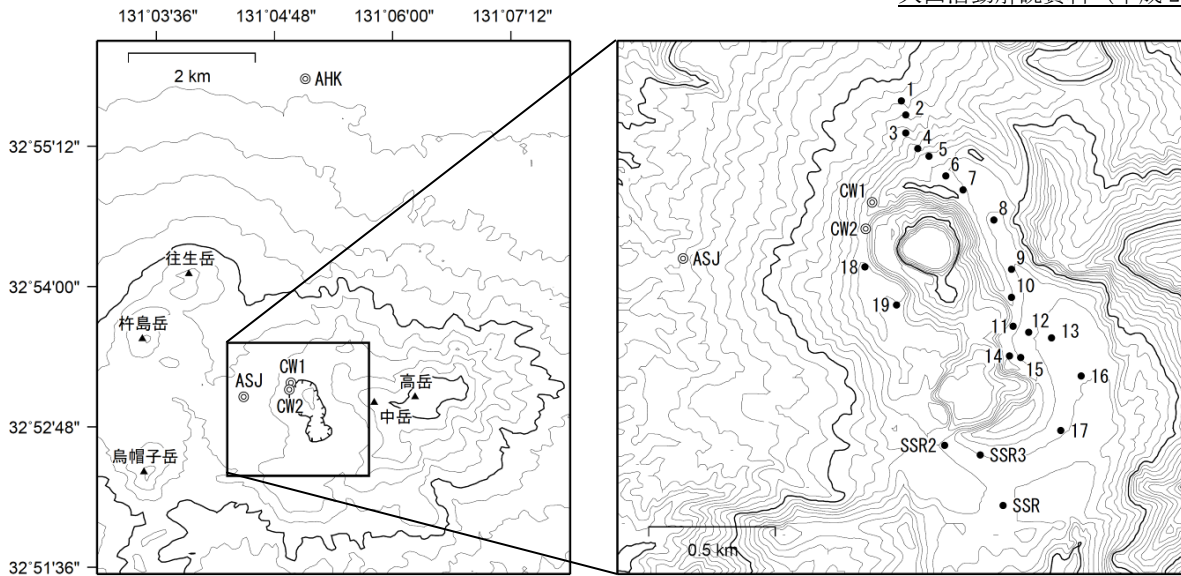
図 5 阿蘇山 全磁力観測点配置図 (◎：連続観測点 ●：繰返し観測点)
