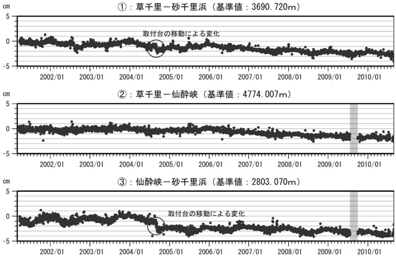
図 4 阿蘇山 GPS連続観測による基線長変化（2001年3月～2010年8月）
