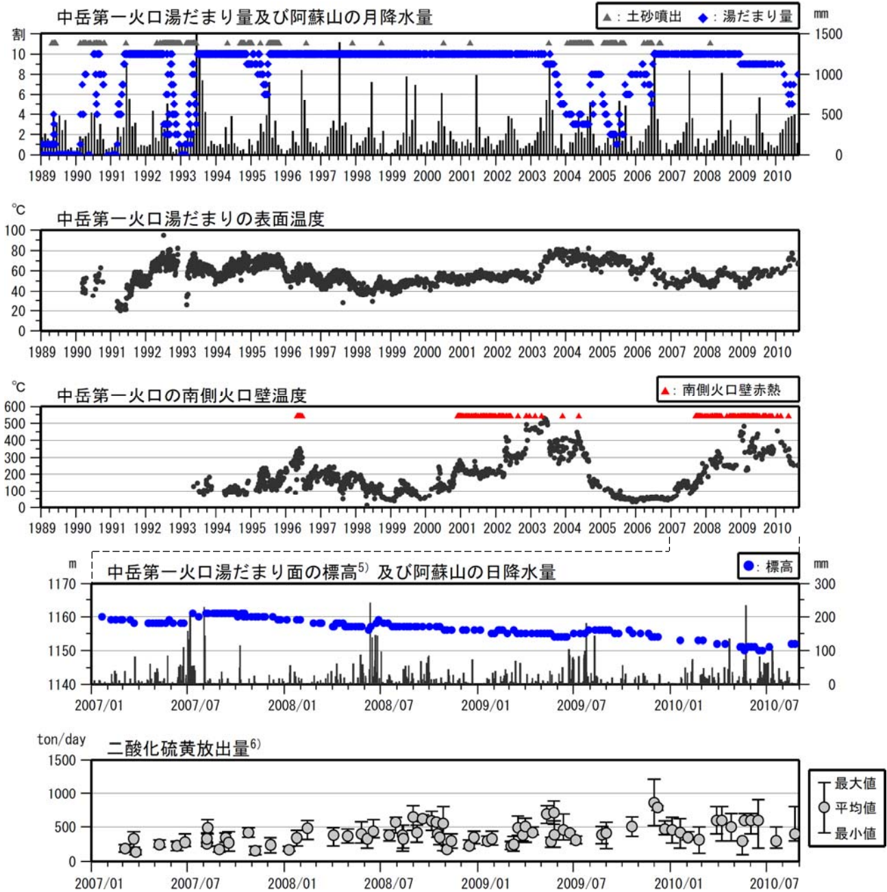
図 3※ 阿蘇山 湯だまり、火口壁、二氧化硫黄放出量の状況（1989 年 1 月～2010 年 8 月） 湯だまり面の標高は、2007 年 10 月頃から緩やかに低下しています。
