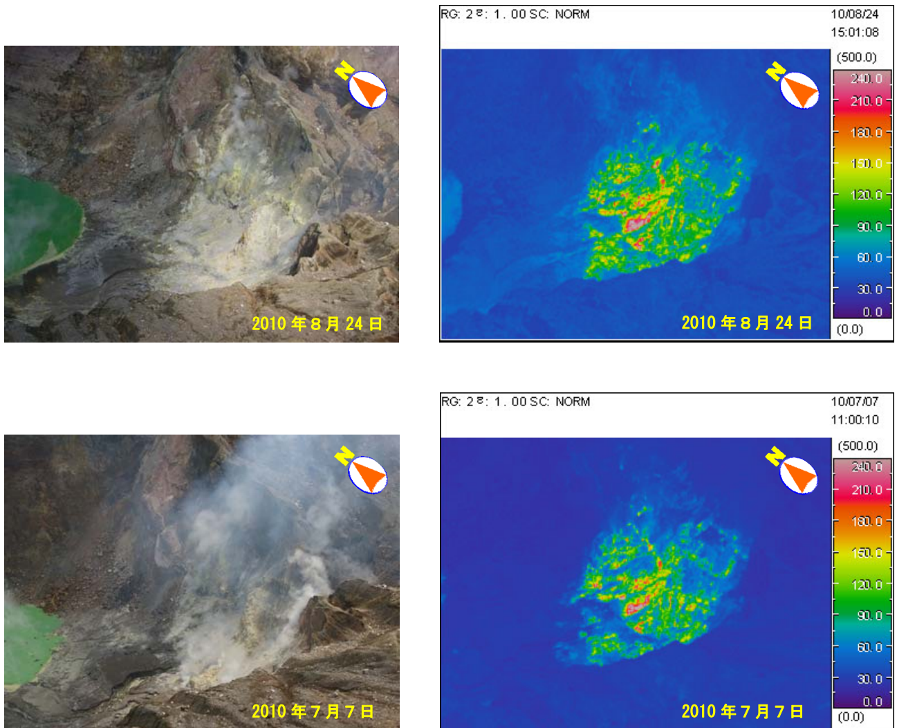
図 7 阿蘇山 赤外熱映像装置 7) による中岳第一火口南側火口壁の地表面温度分布 熱異常域の分布は前期間と比べて特段の変化はありませんでした。
