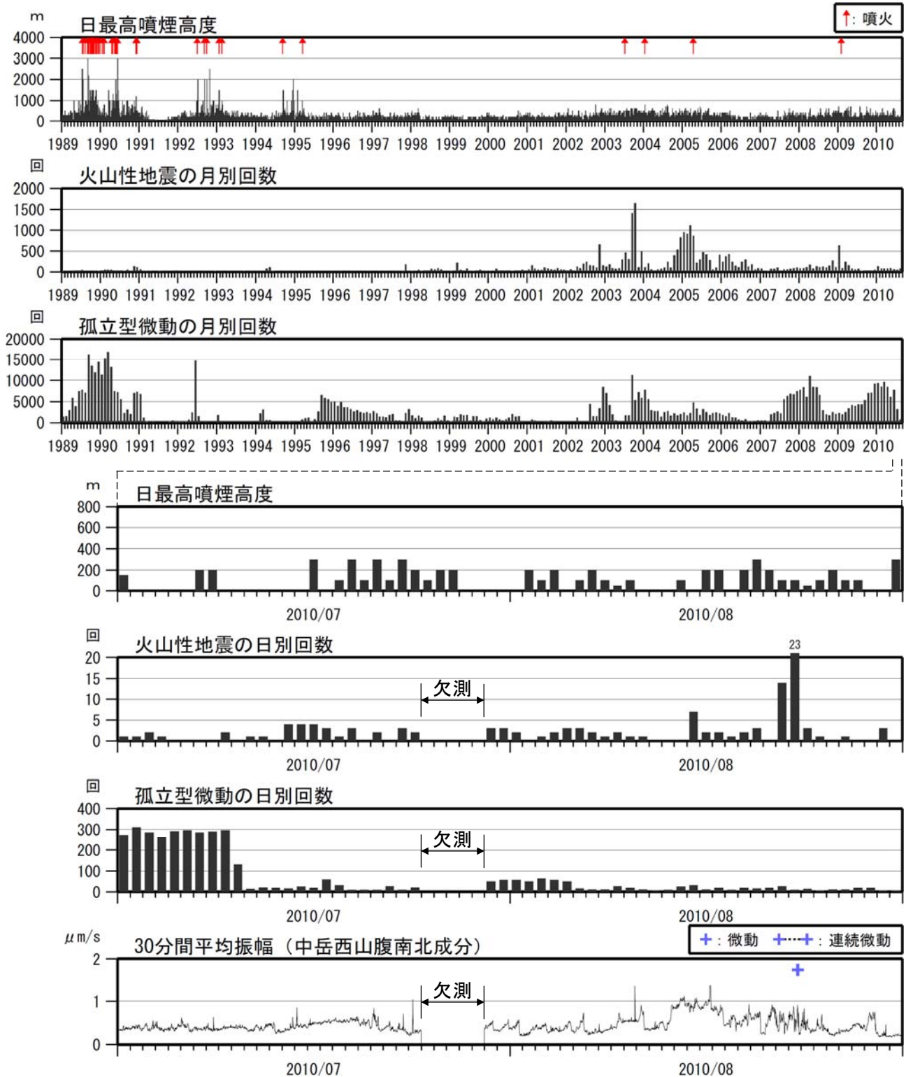
図 2 阿蘇山 噴煙、火山性地震、孤立型微動の状況（1989 年 1 月～2010 年 8 月）
