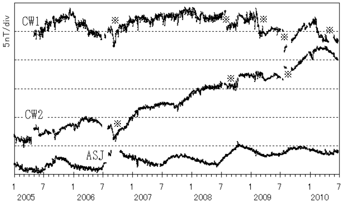
図 7 阿蘇山 全磁力連続観測による阿蘇山麓 (AHK) を基準とした中岳第一火口周辺の全磁力変化 (2005 年 1 月～2010 年 6 月)
