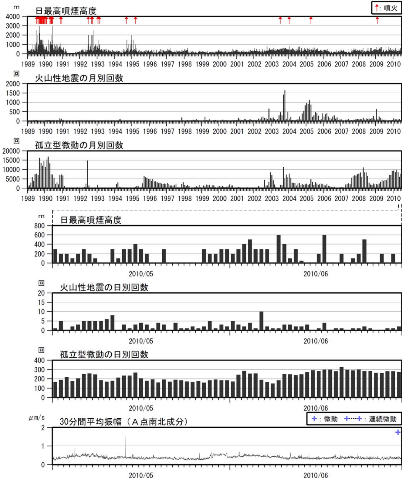
図 2 阿蘇山 噴煙、孤立型微動、火山性地震の状況（1989 年 1 月～2010 年 6 月）
