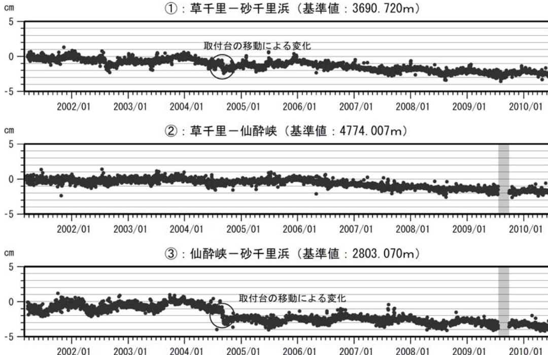
図 5 阿蘇山 GPS連続観測による基線長変化（2001 年 3 月～2010 年 6 月）
