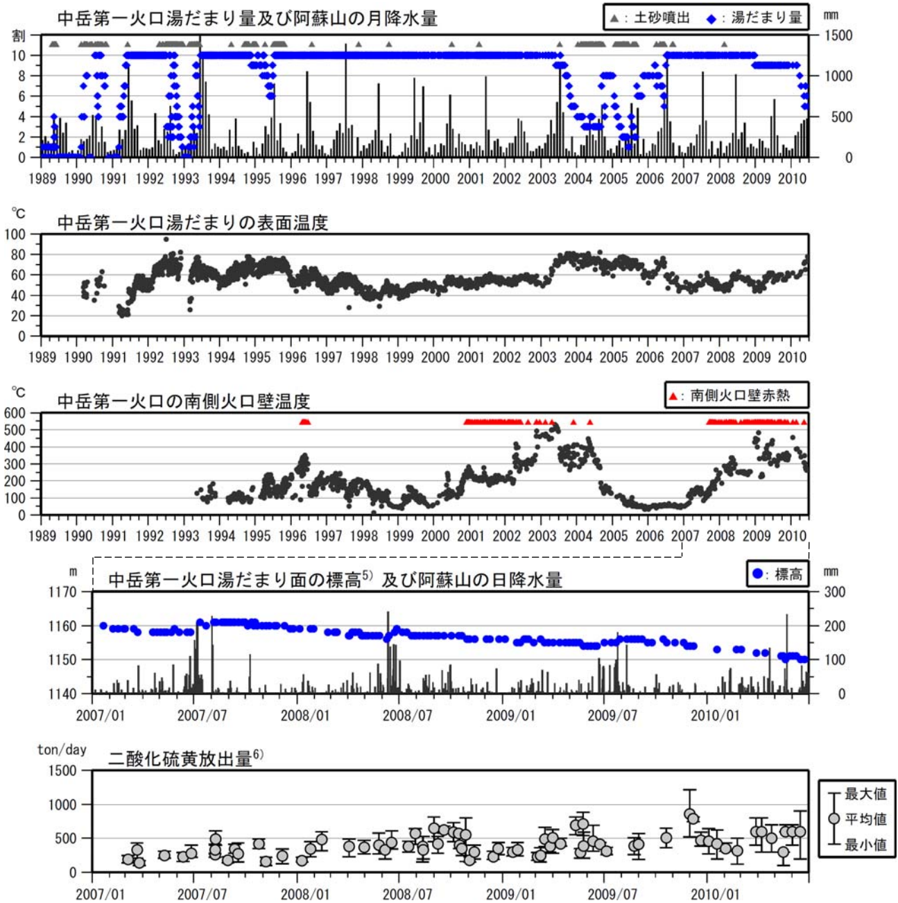
図 3※ 阿蘇山 湯だまり、火口壁、二氧化硫黄放出量の状況（1989 年 1 月～2010 年 6 月）
