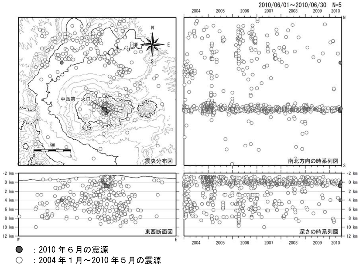
図 4※ 阿蘇山 震源分布図（2004 年 1 月～2010 年 6 月）
