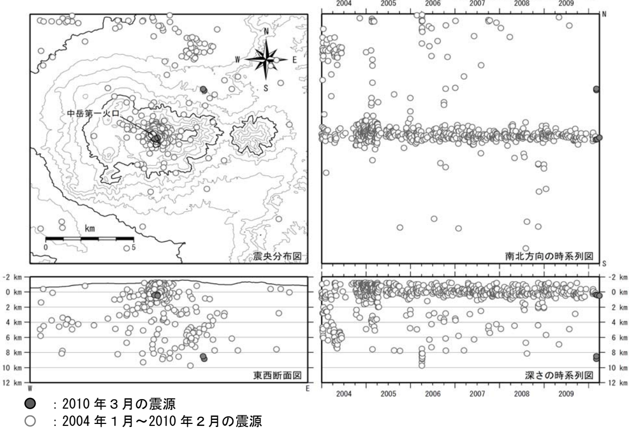
図 4※ 阿蘇山 震源分布図 (2004 年 1 月~2010 年 3 月)
