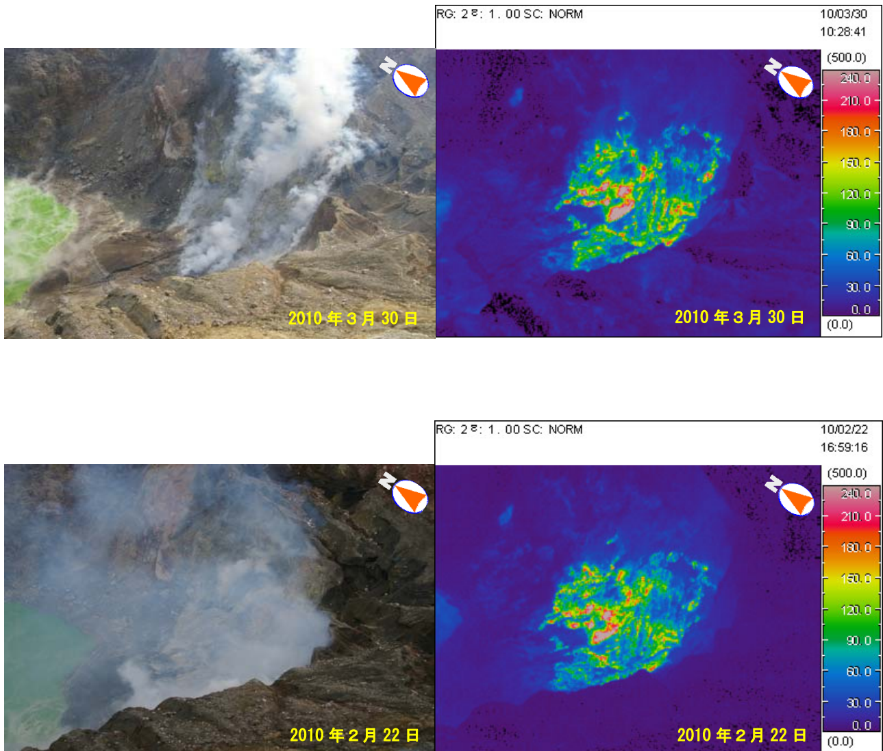
図 8 阿蘇山 赤外熱映像装置 9) による中岳第一火口南側火口壁の地表面温度分布 < 3 月の状況 >
