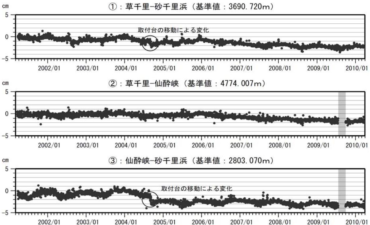
図 5 阿蘇山 GPS連続観測による基線長変化 (2001 年 3 月~2010 年 3 月)
