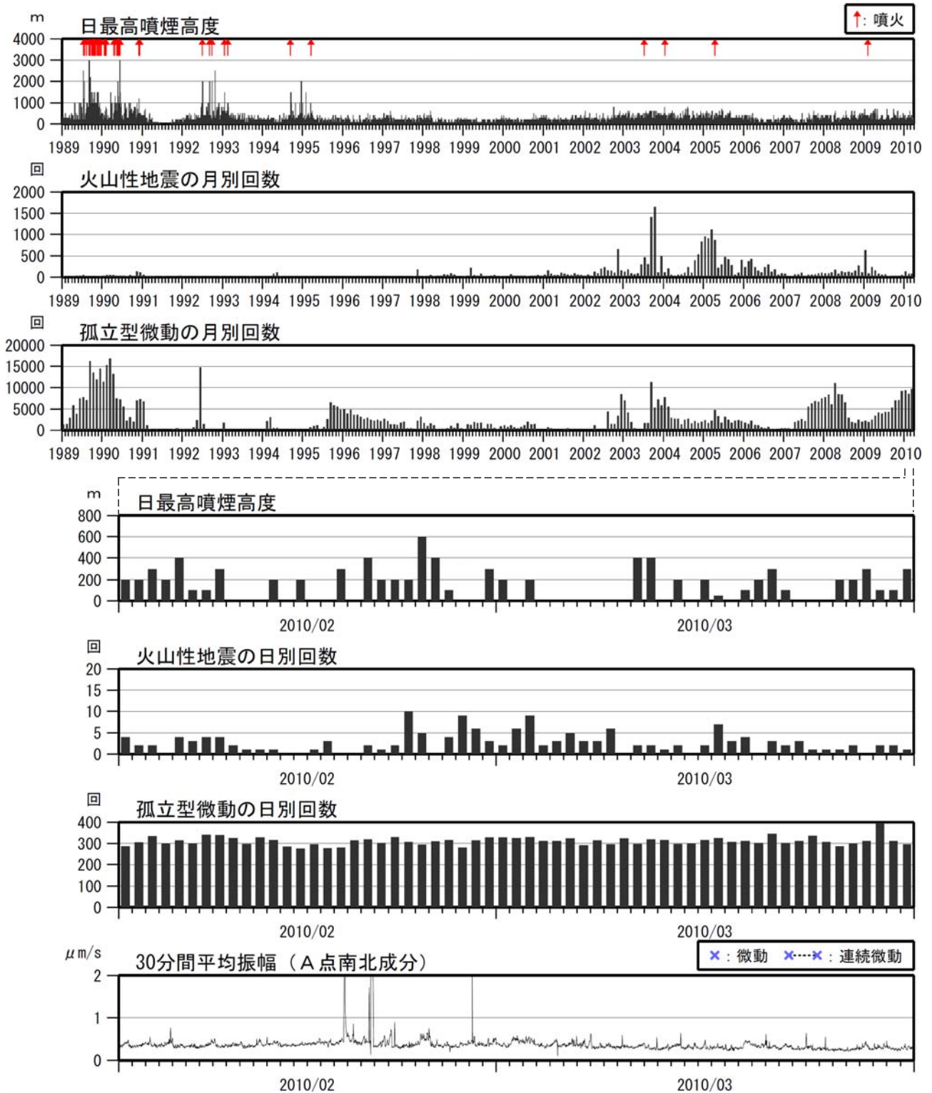
図 2 阿蘇山 火山活動経過図（1989 年 1 月～2010 年 3 月）
