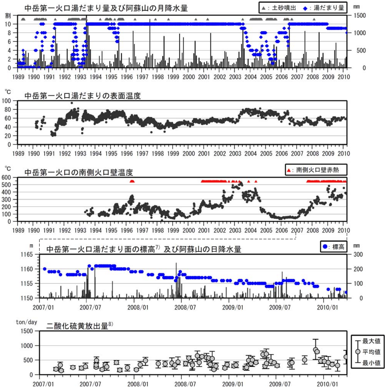
図3 阿蘇山 火山活動経過図（1989年1月～2010年3月）
