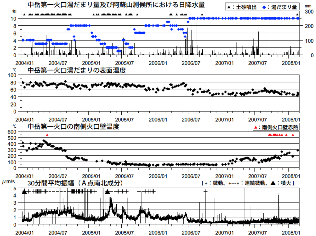
図3 阿蘇山 火山活動経過図(2004年1月1日~2008年2月29日)
