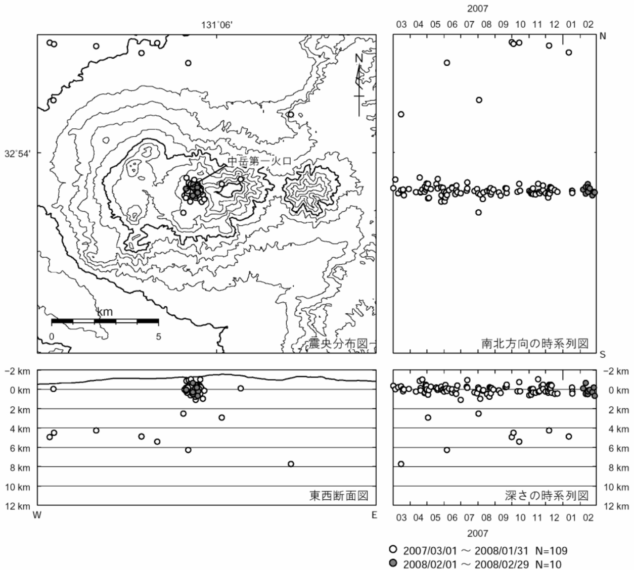
図1 阿蘇山 震源分布図
