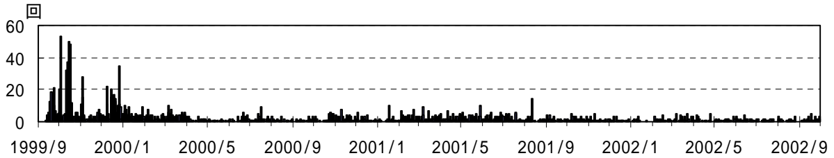
図1 A型地震日別地震回数(1999年9月12日～2002年9月30日)
