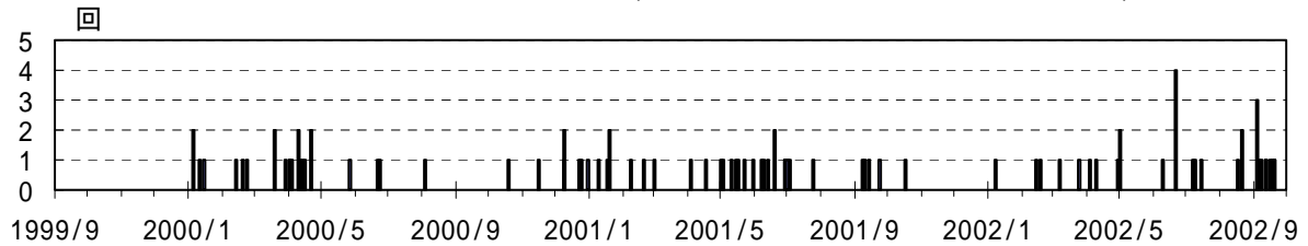
図2 B型地震日別地震回数(1999年9月12日～2002年9月30日)
