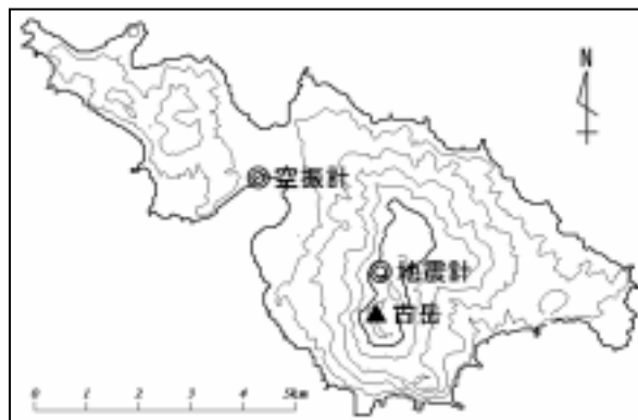
図5 観測点位置図
