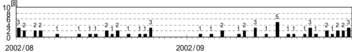
図3 A型地震日別地震回数(2002年8月1日～2002年9月30日)
