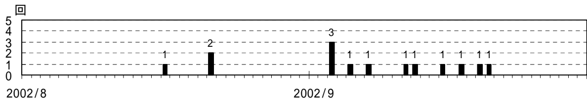
図4 B型地震日別地震回数(2002年8月1日～2002年9月30日)
