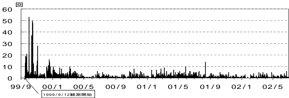
図2 日別地震回数(1999年9月12日～2002年6月30日)
