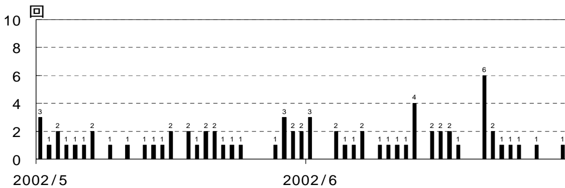
図1 日別地震回数(2002年5月1日～6月30日)
