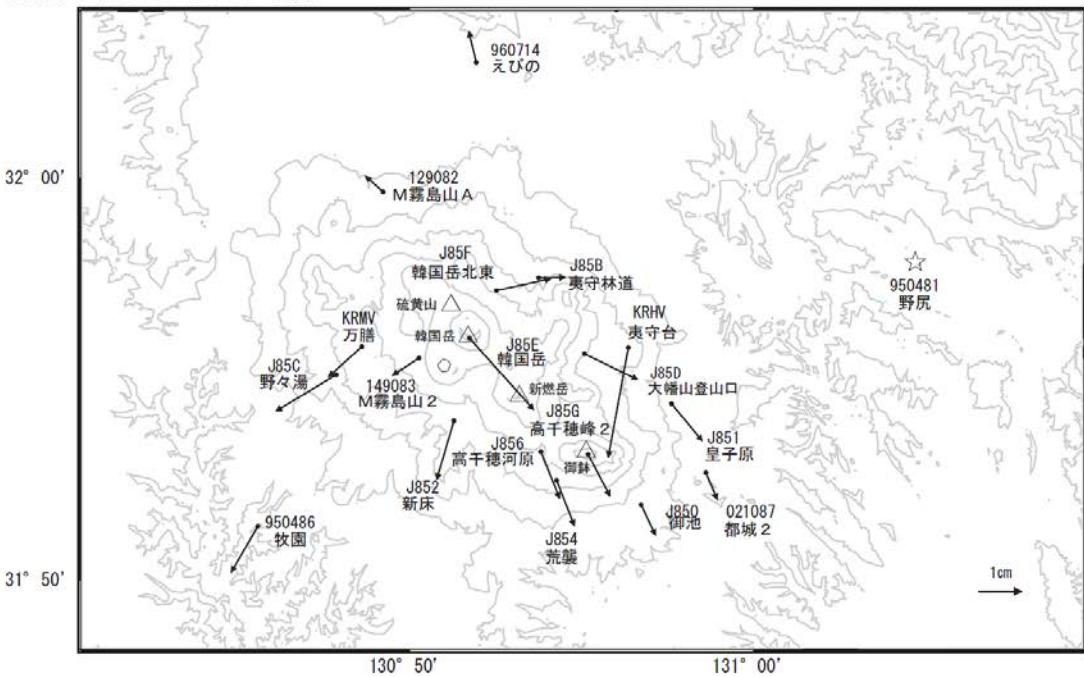
第4図 霧島山周辺の電子基準点・気象庁・防災科学技術研究所 GNSS 観測点の統合解析による水平変動ベクトル図(上段:2018年6月~2018年9月、下段:2017年9月~2018年9月)
