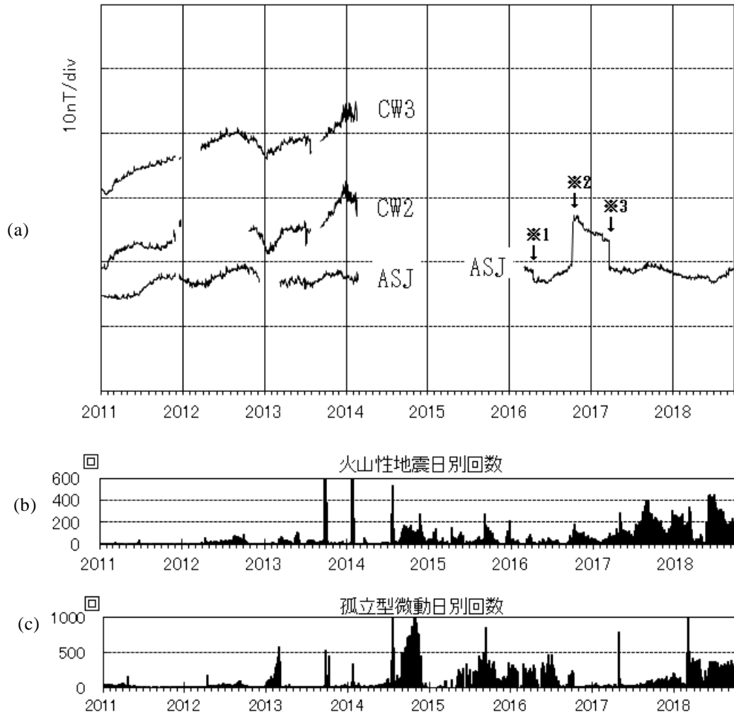
第2図 2011年1月から2018年9月までの連続観測点CW2、CW3、ASJにおける全磁力日平均値と参照点AHKの日平均値との差(a)、火山性地震日別回数(b)、孤立型微動日別回数(c)
