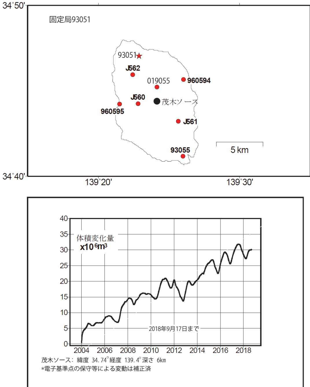
第 6-1 図 時間依存インバージョンの手法による伊豆大島の変動源の体積変化推定 (上段: 推定に用いた観測点 (赤点)、固定点 (星印) の配置と茂木ソースの位置 (黒丸)、 下段: 推定された茂木ソース体積の時間変化)
