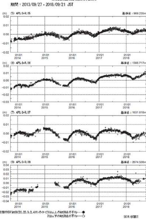
第4図 伊豆大島の光波測距観測結果
