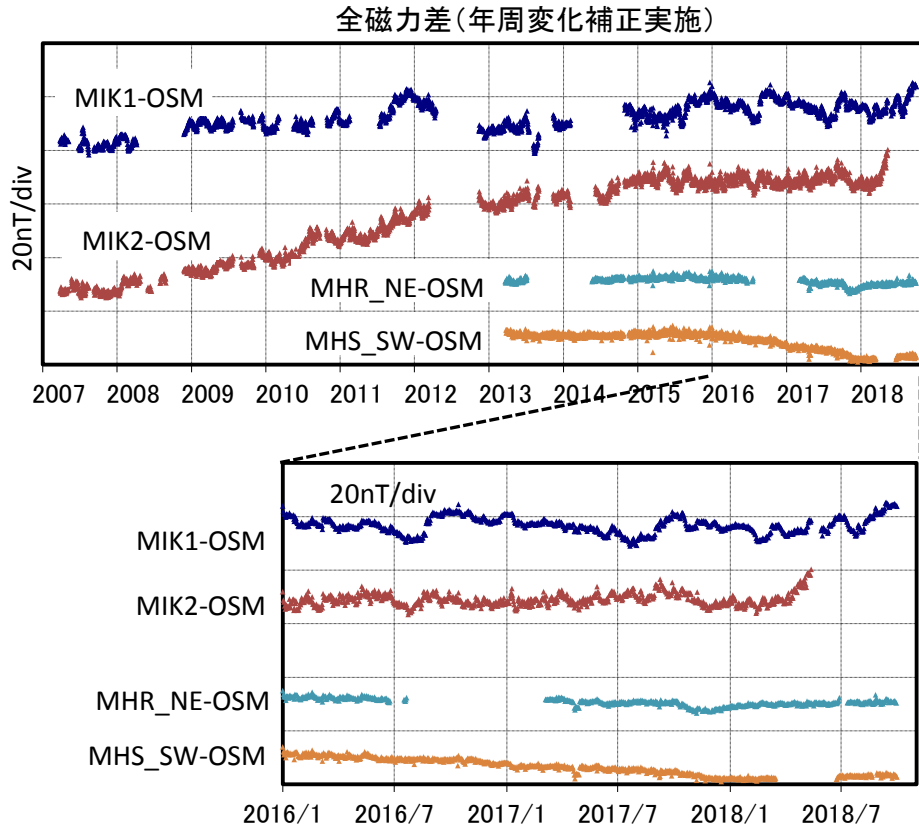
第3図 年周変化補正後の全磁力日平均値差 (上図：2007年3月～2018年9月、下図：2016年1月～2018年9月)
