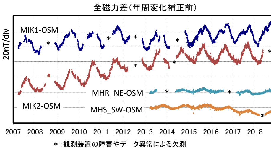
第2図 各連続観測点と参照点OSMの全磁力日平均値差(2007年3月～2018年9月)
