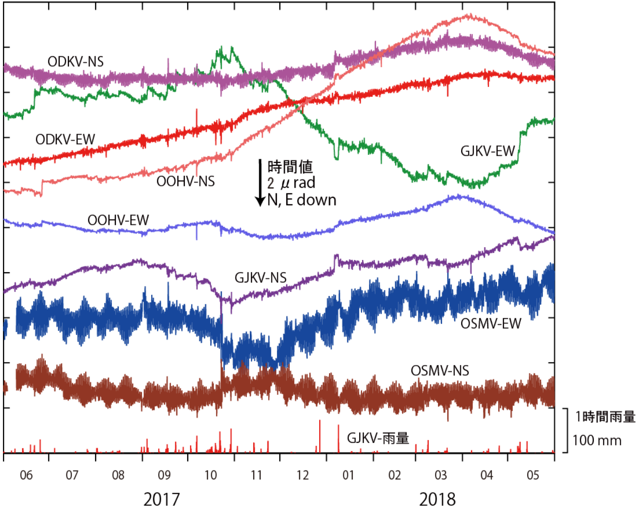
第2図 防災科学技術研究所・伊豆大島火山活動観測網による傾斜変動観測結果。表示期間は2017年6月1日～2018年5月31日で、表示データは時値（毎正時の値）。
