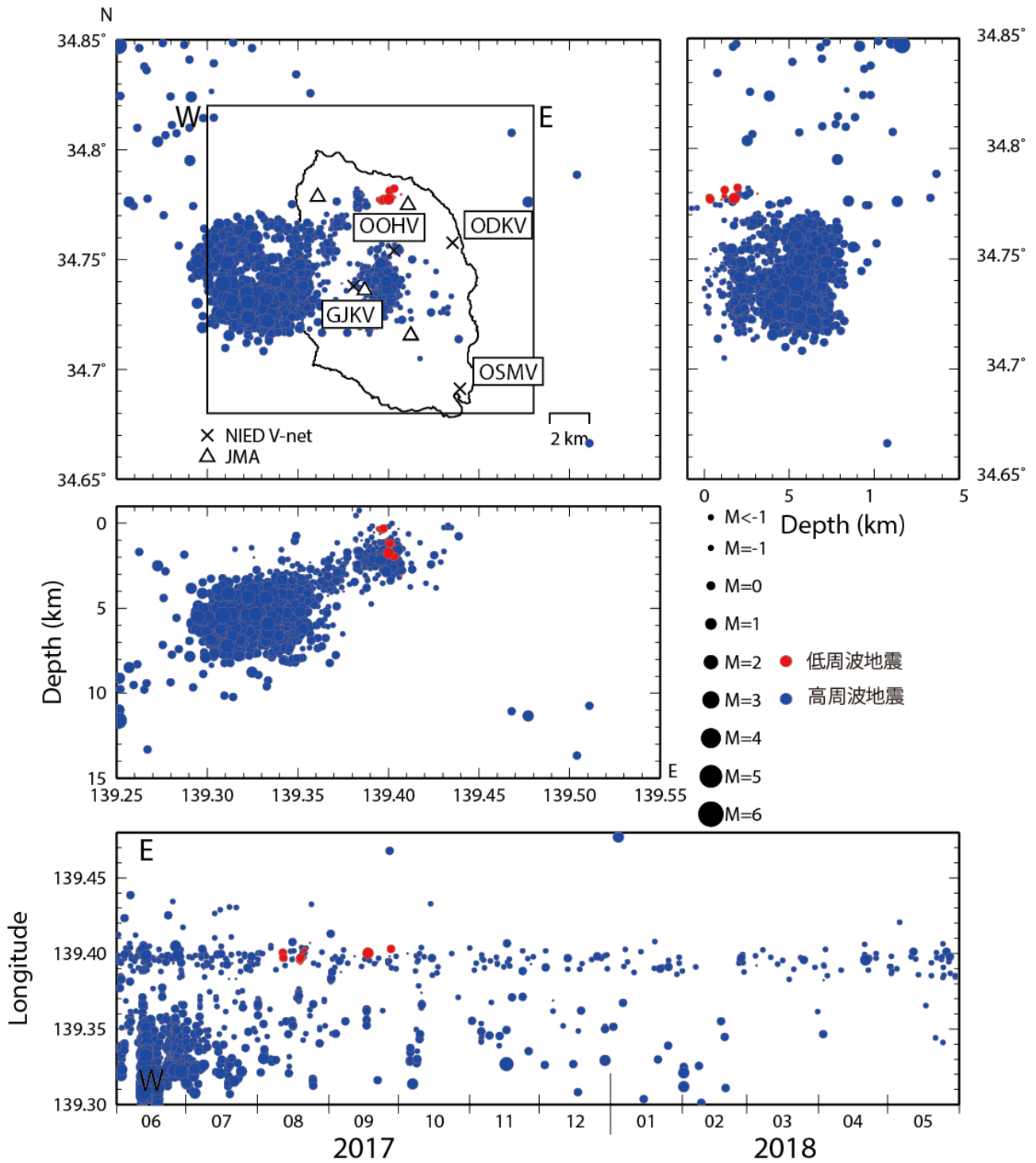
第1図 伊豆大島の震源分布および時空間分布図。表示期間は2017年6月1日～2018年5月31日。 Fig. 1 Hypocenter distribution around Izu-Oshima for the period from Jun 1, 2017 to May 31, 2018.
